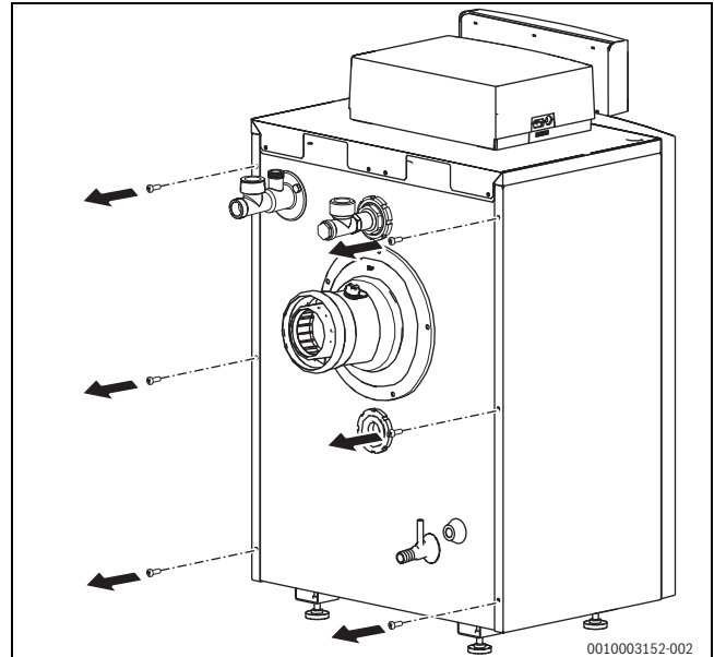
Bild 70 Befestigungsschrauben lösen
