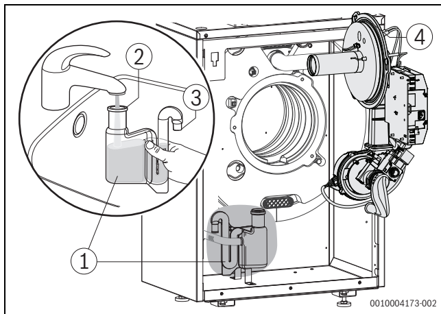
Bild 69 Siphon reinigen
