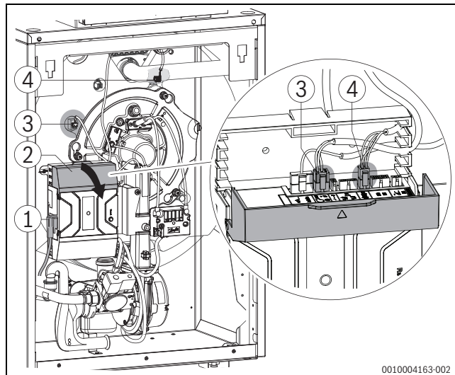
Bild 59 Steckverbinder lösen
