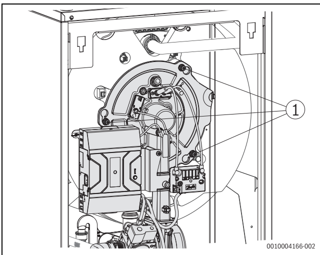
Bild 62 Befestigungsmuttern lösen
