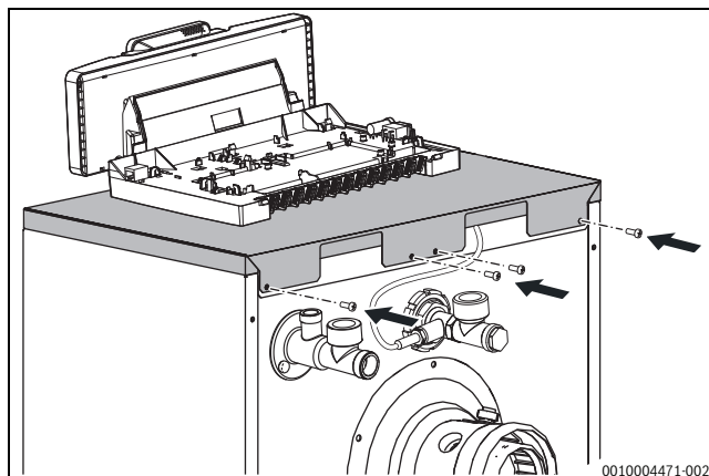
Bild 22 Elektrische Leitungen verlegen
