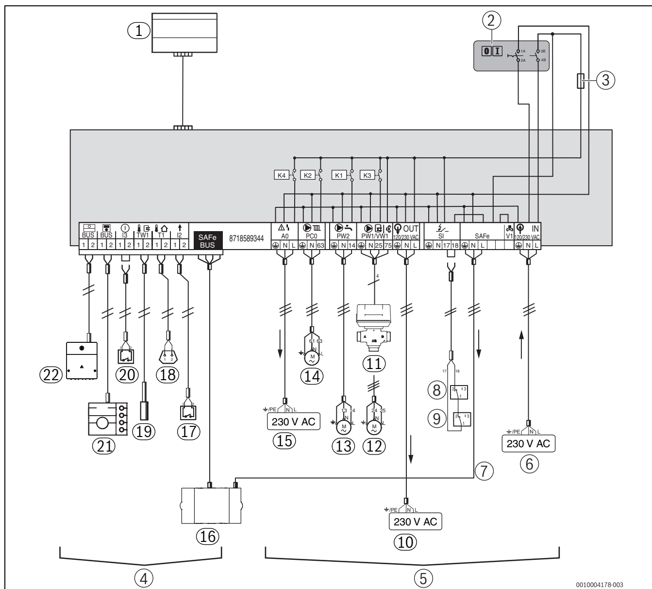
Bild 83 Anschlussplan Regelgerät MX25
