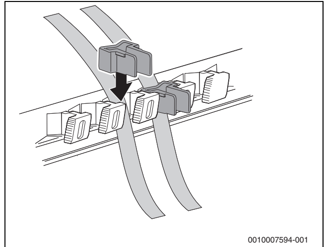
Bild 28 Elektrische Leitungen mit Zugentlastung sichern
