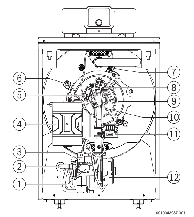
Bild 89 Vorderansicht
