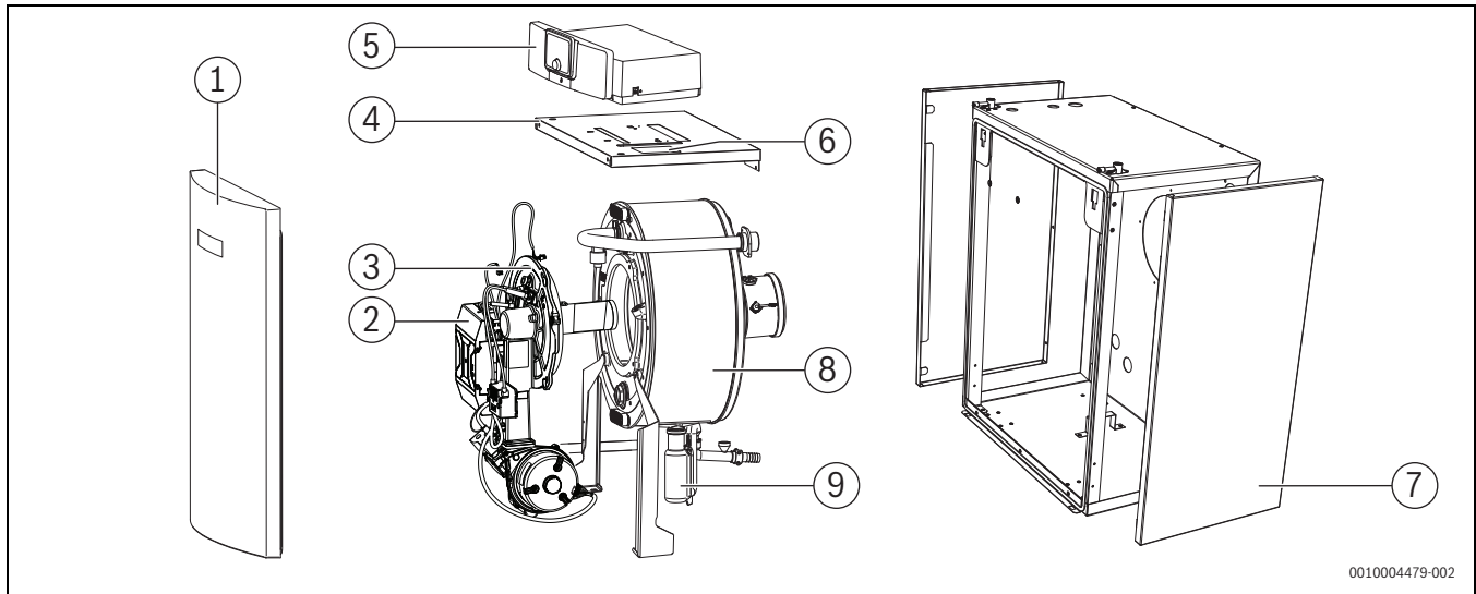
Bild 1 GC7000F 15...50 – Hauptbestandteile
