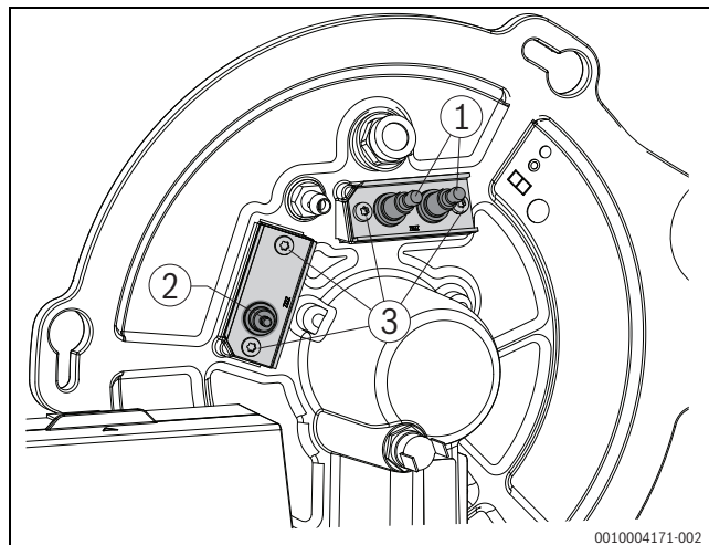
Bild 67 Elektrodenposition
