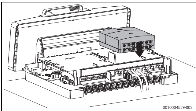
Bild 27 Funktionsmodule einstecken
