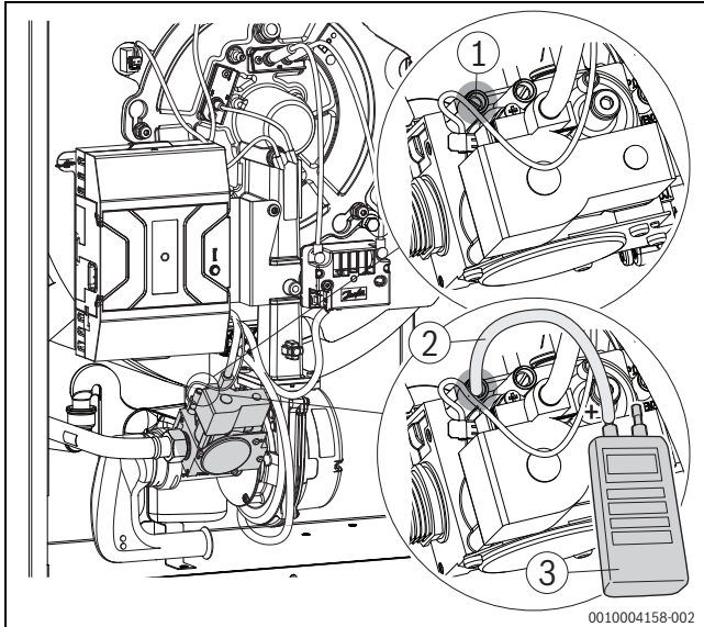
Bild 48 Gas-Anschlussdruck messen
