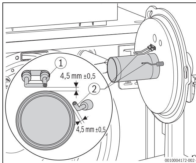
Bild 68 Abstände Elektroden
