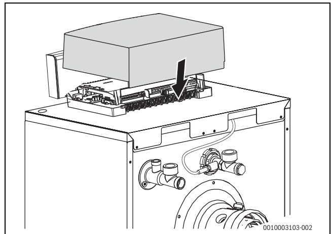
Bild 29 Abdeckhaube montieren
