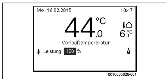
Bild 50 Schornsteinfegerbetrieb aktiv
