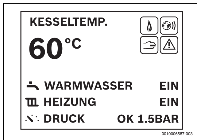
Bild 244 Standardanzeige
