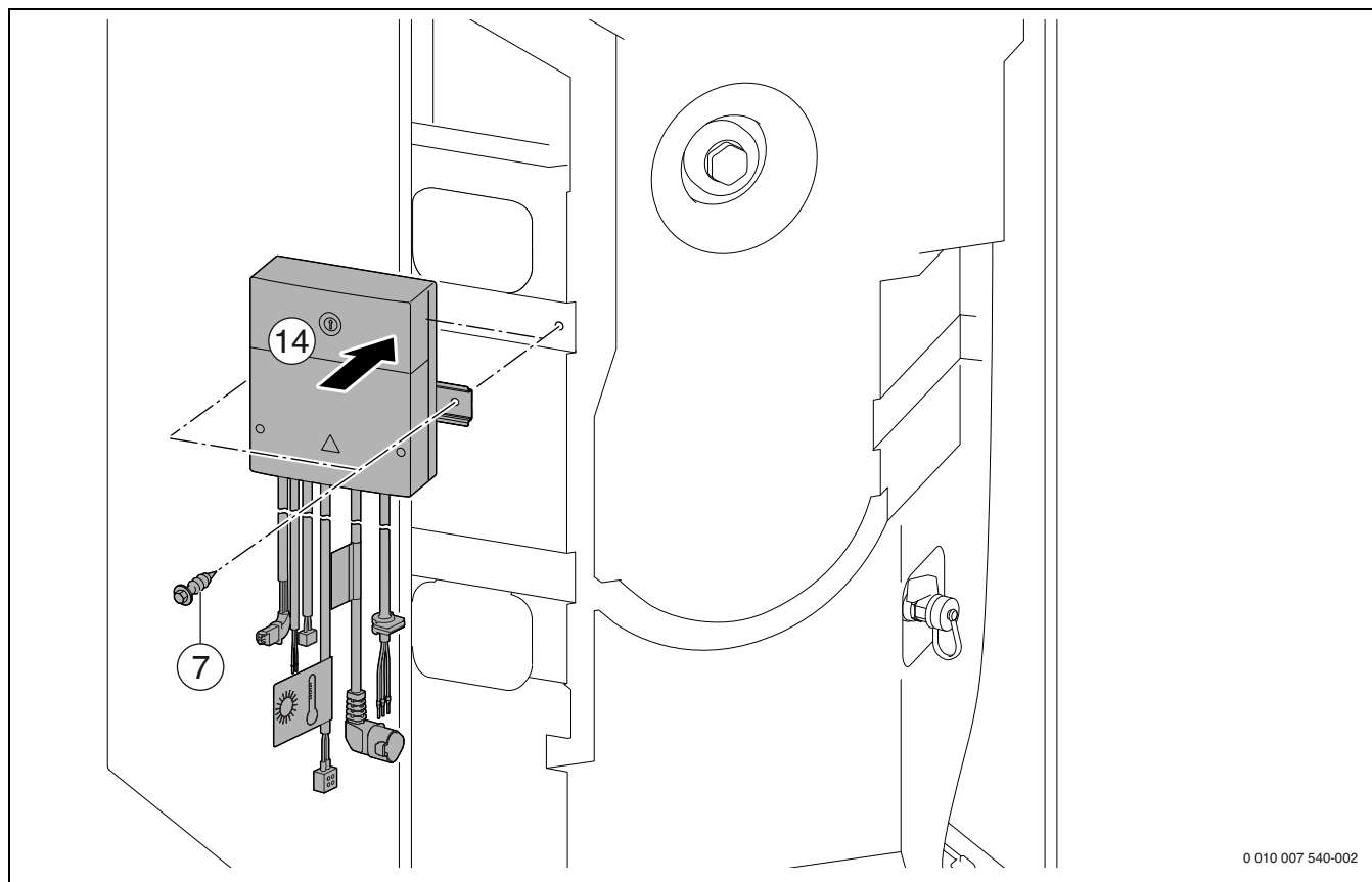
Bild 174 GC9000iWM../150-Geräte
