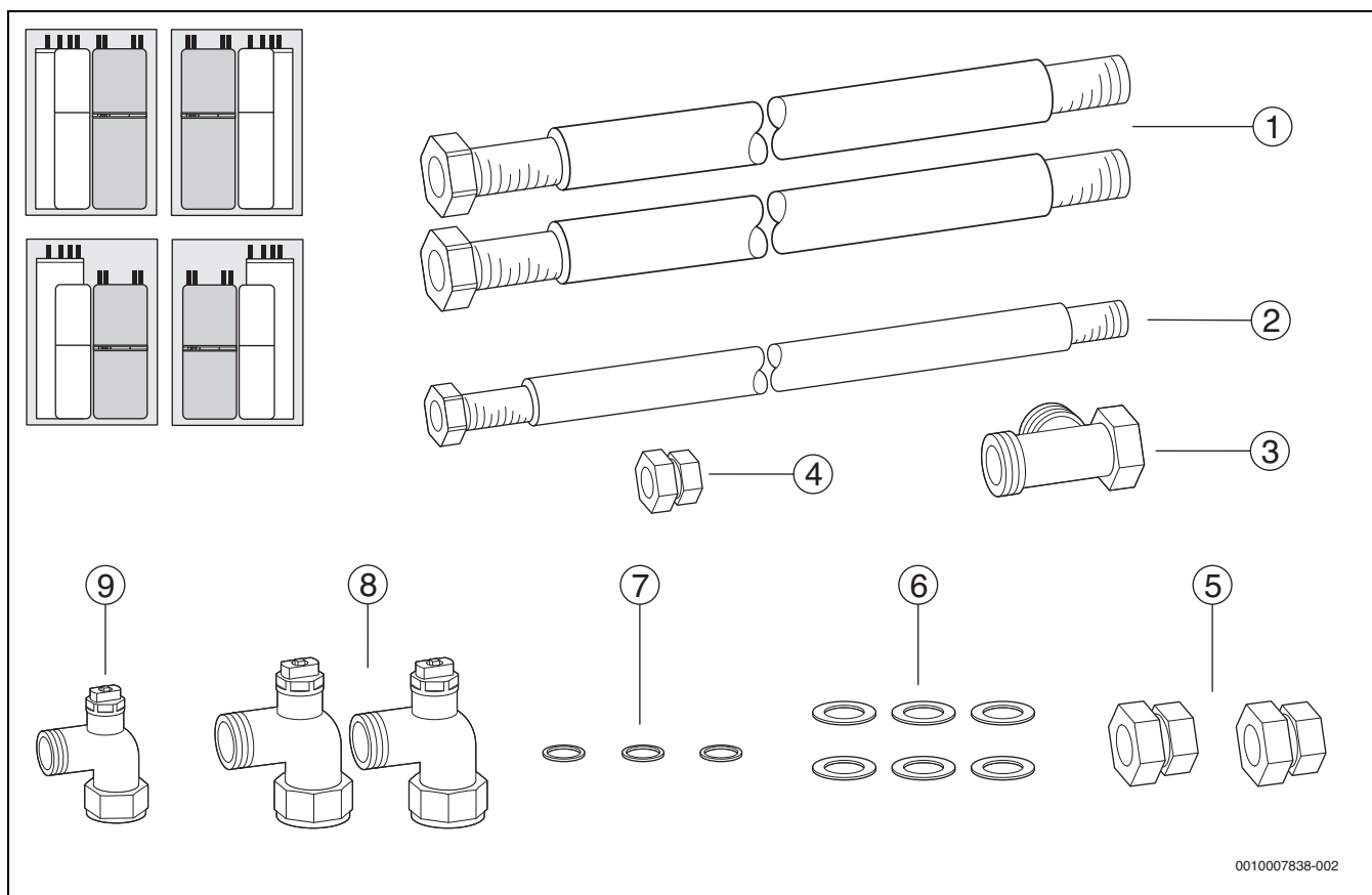
Bild 211 Lieferumfang
