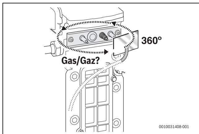
Bild 253 Dichtheit kontrollieren
