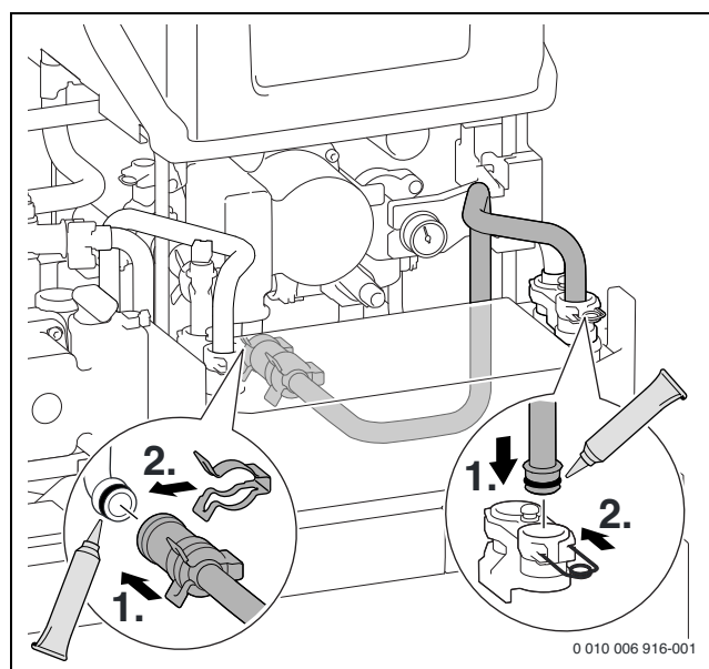
Bild 61 Rohrverbindung zwischen Plattenwärmetauscher und Wärmeblock erstellen (Rücklauf)
