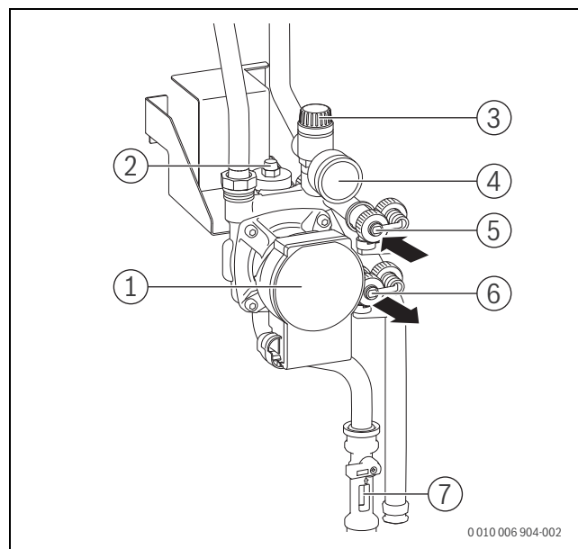
Bild 236 Übersicht Solargruppe
