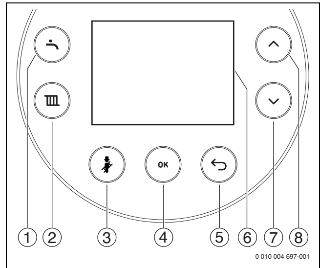
Bild 243 Bedienfeld
