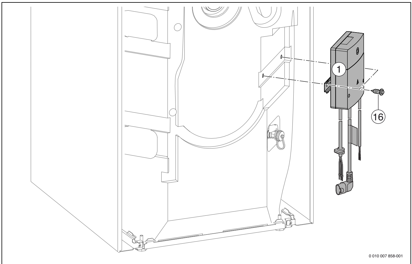
Bild 109 GC9000iWM../150-Geräte
