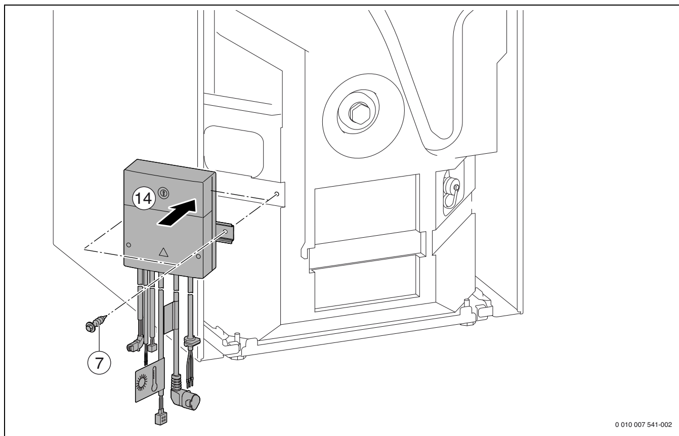
Bild 175 GC9000iWM../100-Geräte
