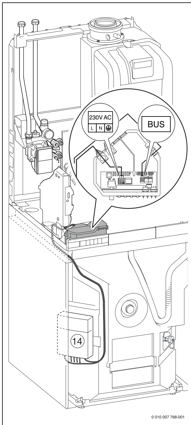
Bild 179 GC9000iWM../100-Geräte
