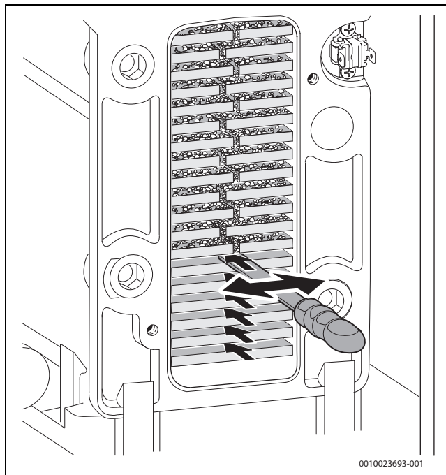
Bild 209 Reinigungsmesser
