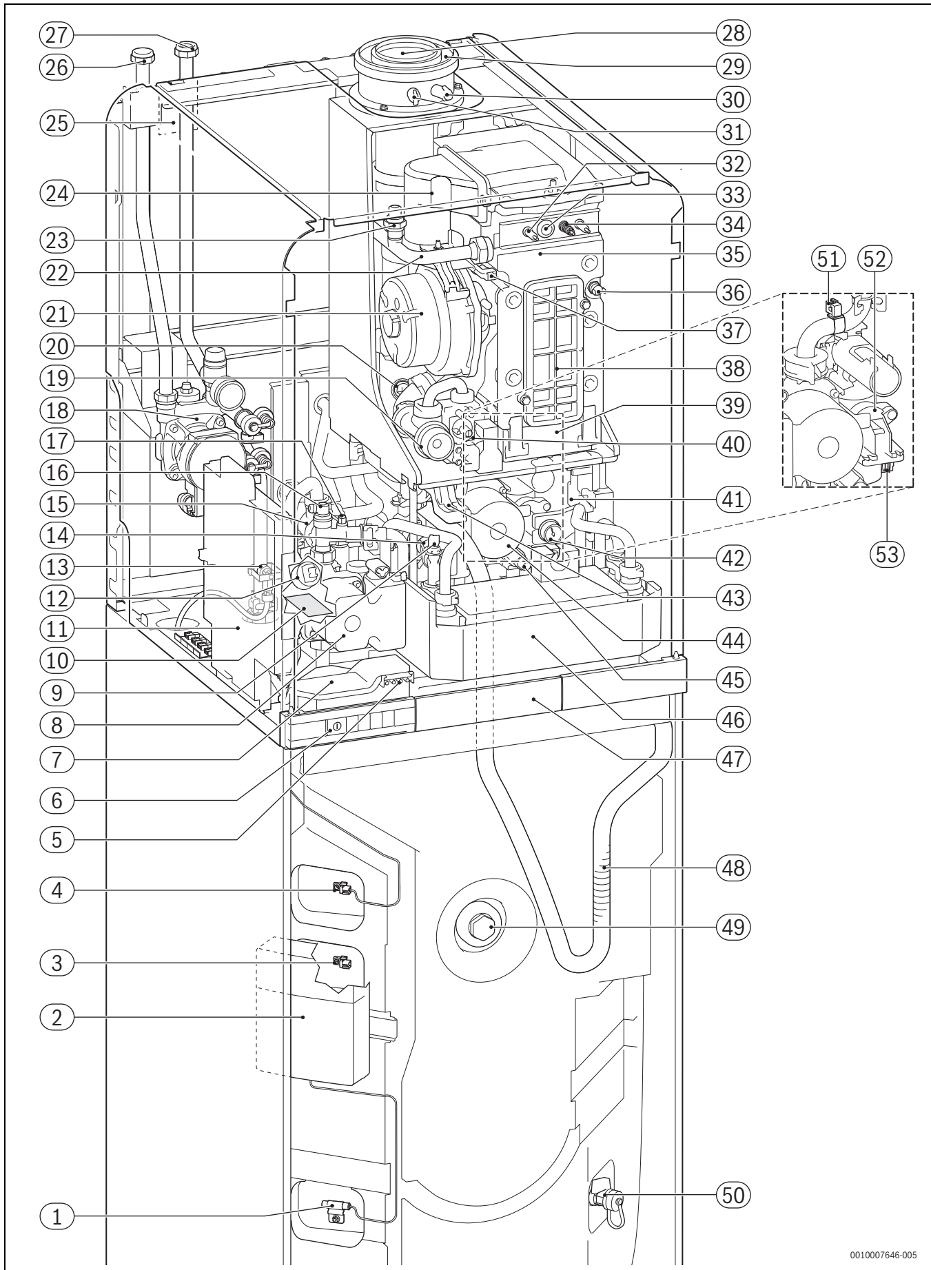
Bild 12 GC9000iWM.../210 S-Geräte
