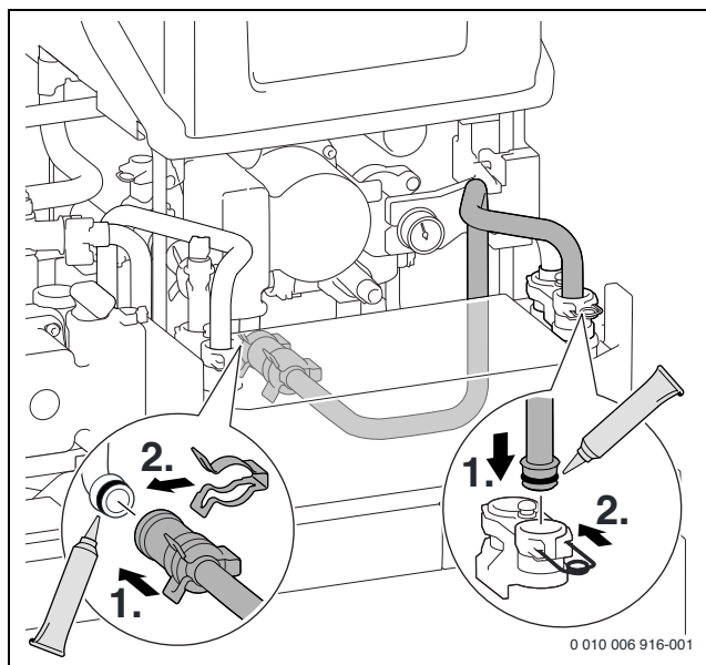
Bild 54 Rohrverbindung zwischen Plattenwärmetauscher und Wärmeblock erstellen (Rücklauf)
