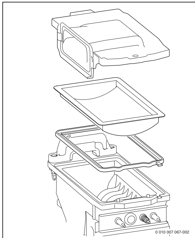
Bild 207 Brenner
