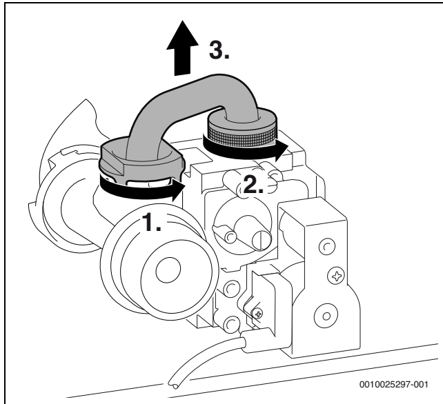
Bild 219 Gasrohr ausbauen
