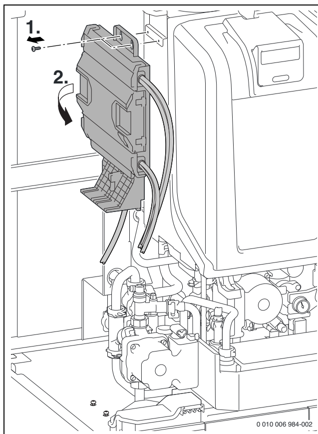
Bild 55 Steuergerät abnehmen
