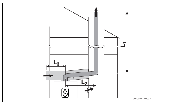
Bild 22 Starre Abgasführung nach C 53x im Schacht und Luft-Abgas-Führung mit separater Luftzufuhr und konzentrischer Abgasableitung im Aufstellraum
