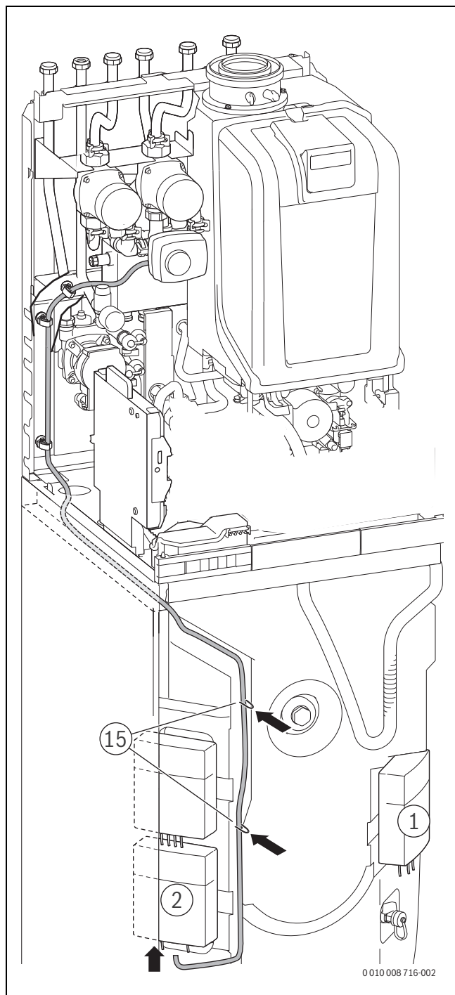
Bild 138 Anschluss Mischermotor
