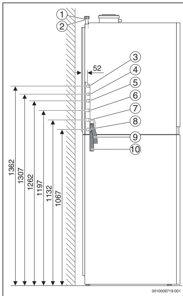
Bild 4 Anschlussmaße des Zubehörs CS 10 - Horizontales Anschluss-Set (Maße in mm)
