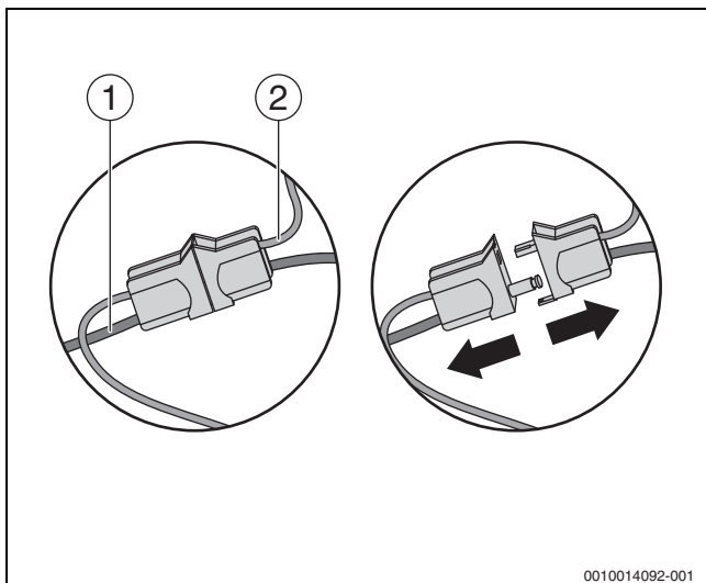
Bild 43 Steckverbinder trennen
