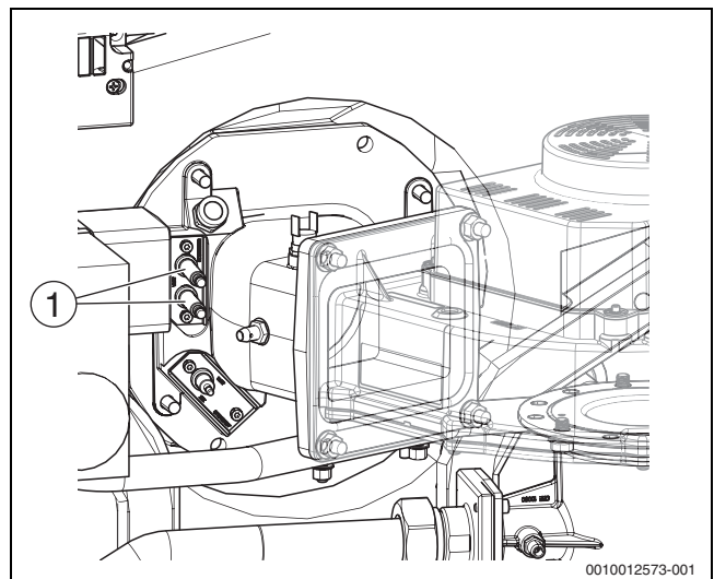
Bild 42 Zündelektroden
