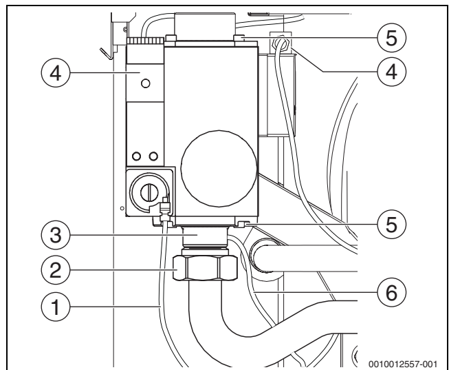
Bild 62 Anschlüsse Gasarmatur (150 ... 300 kW) lösen
