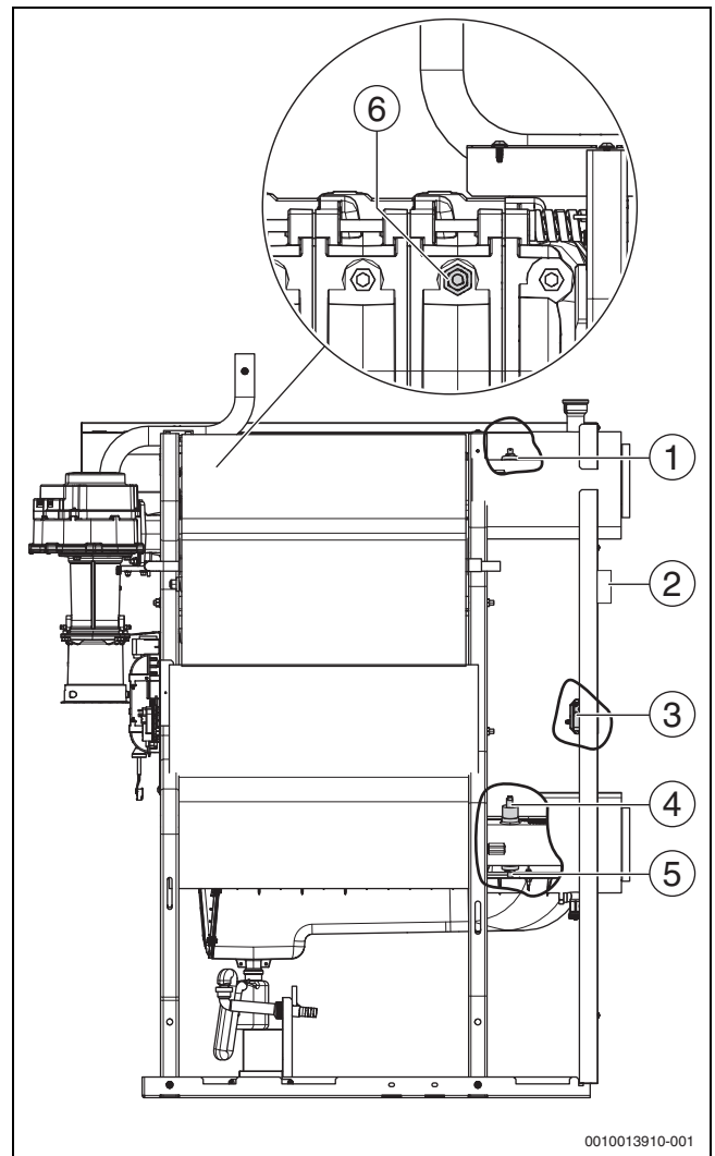
Bild 38 Detail-Übersicht: Position der Fühler
