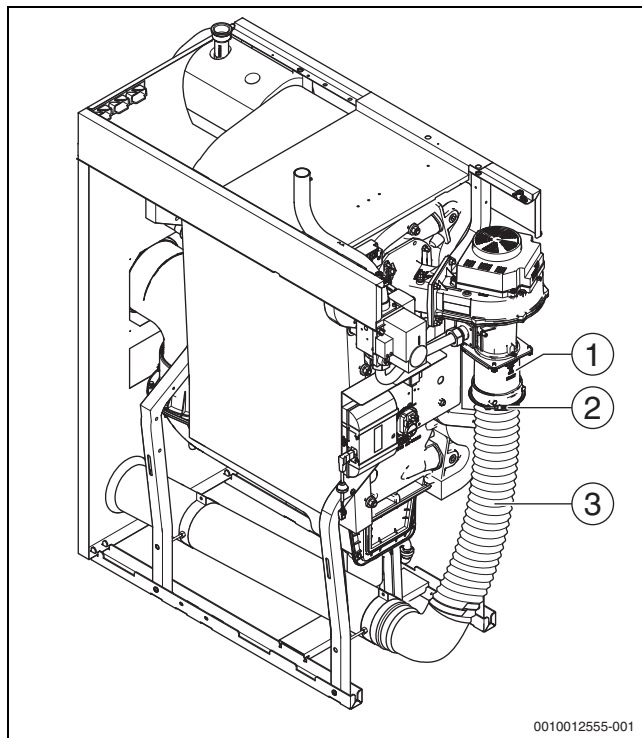
Bild 45 Zuluftleitung
