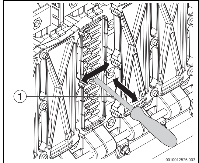
Bild 56 Wärmetauscher waagrecht reinigen
