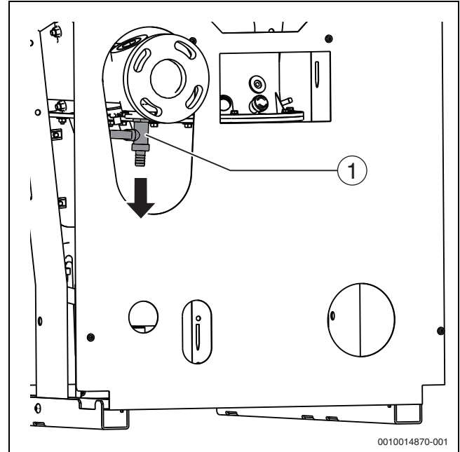
Bild 16 Demontage Entleerhahn (Dargestellt: Kessel mit Flanschanschluss, Ausführung rechts)
