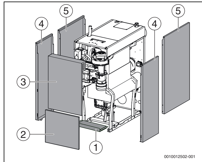
Bild 35 Verkleidungsteile montieren
