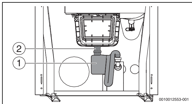
Bild 50 Siphon demontieren
