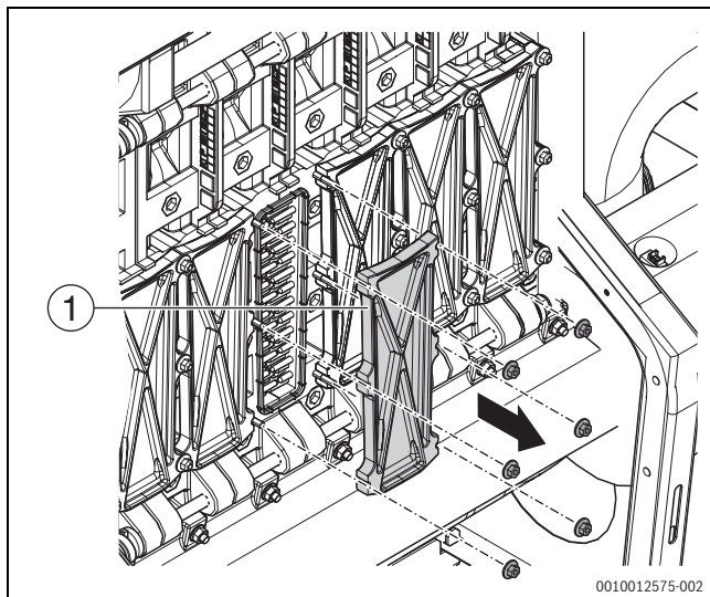
Bild 55 Reinigungsdeckel abnehmen
