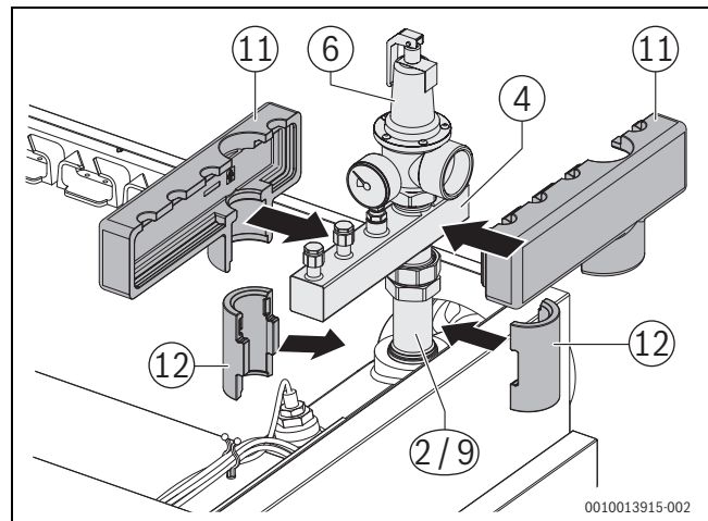
Bild 20 Sicherheits-Set 4 bis 6 bar (Dargestellt: alternative Montage-möglichkeit)
