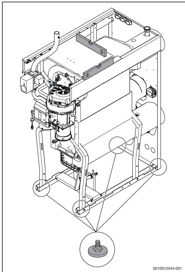
Bild 12 Heizkessel ausrichten
