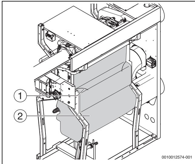
Bild 54 Wärmeschutz am Wärmetauscher
