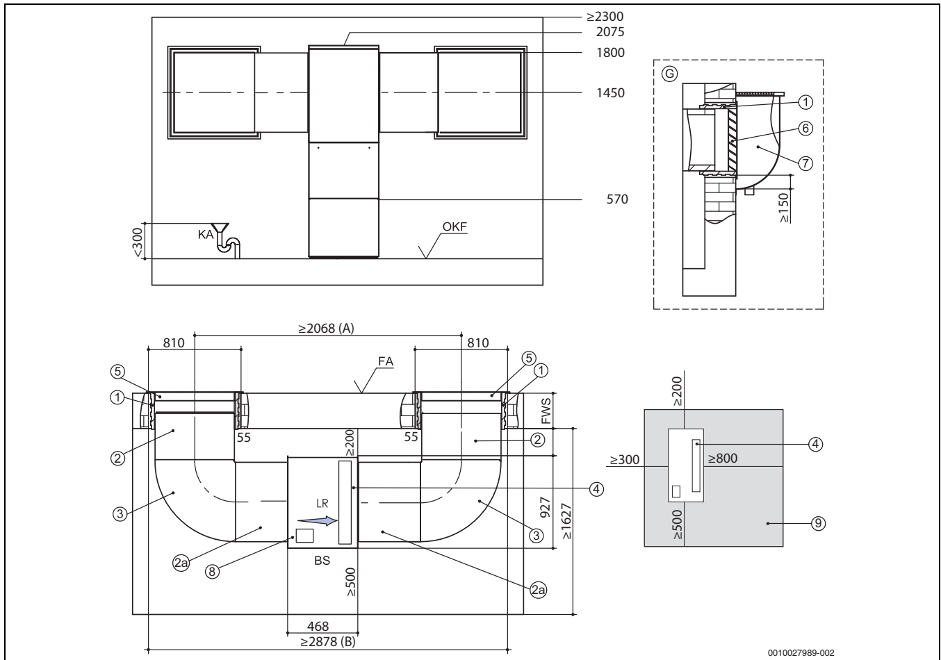
Bild 42 Kanalpläne Variante 3
