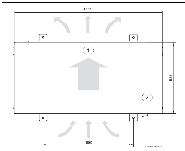
Bild 7 Abmessungen der Wärmepumpenmodelle 13–17, Ansicht von oben
