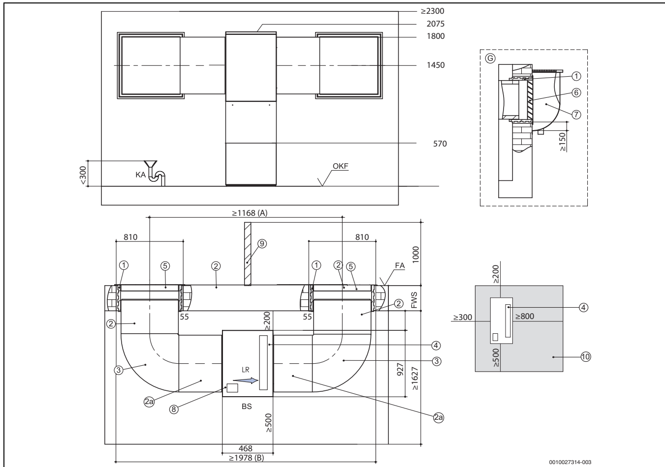
Bild 41 Kanalpläne Variante 2
