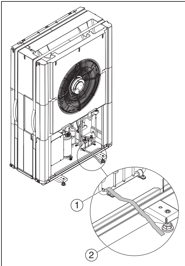
Bild 12 Transportsicherung
