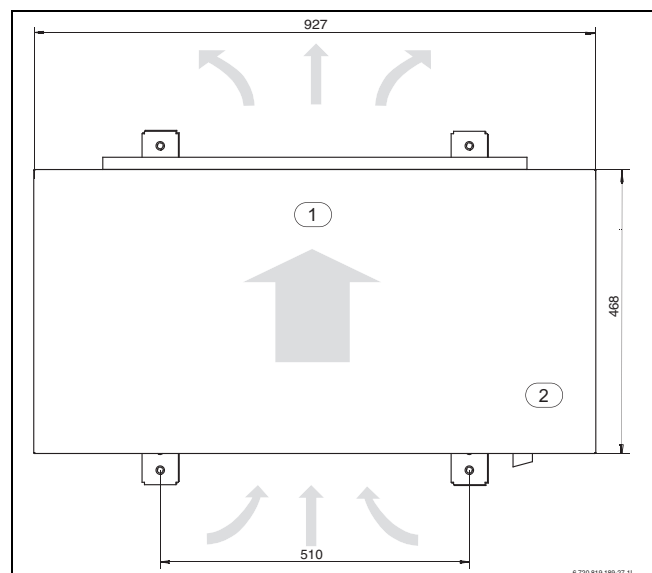
Bild 5 Abmessungen der Wärmepumpenmodelle 7–9, Ansicht von oben
