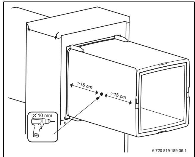
Bild 29 Fühler montieren
