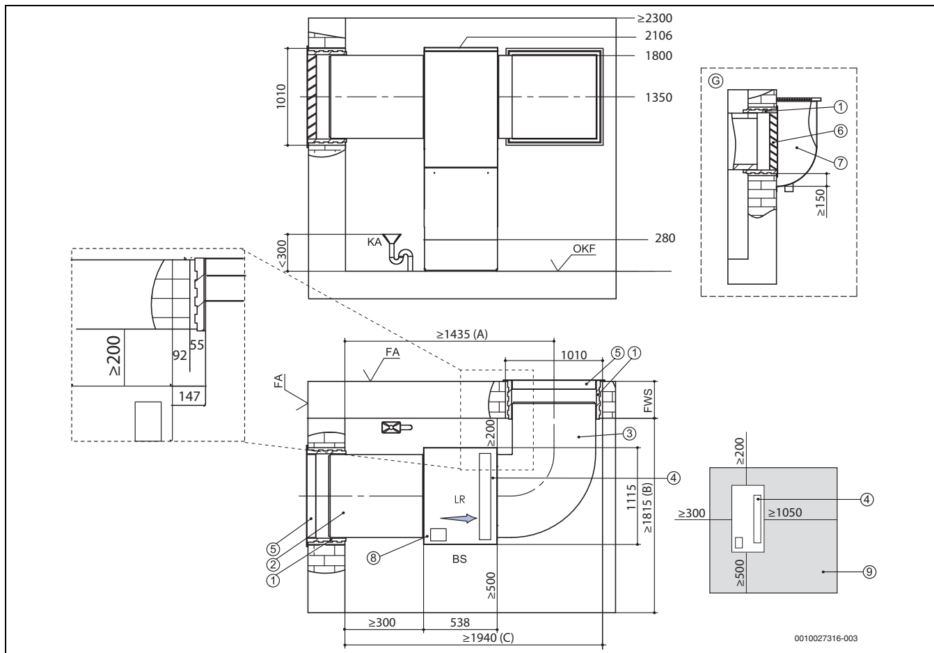
Bild 43 Kanalpläne Variante 1
