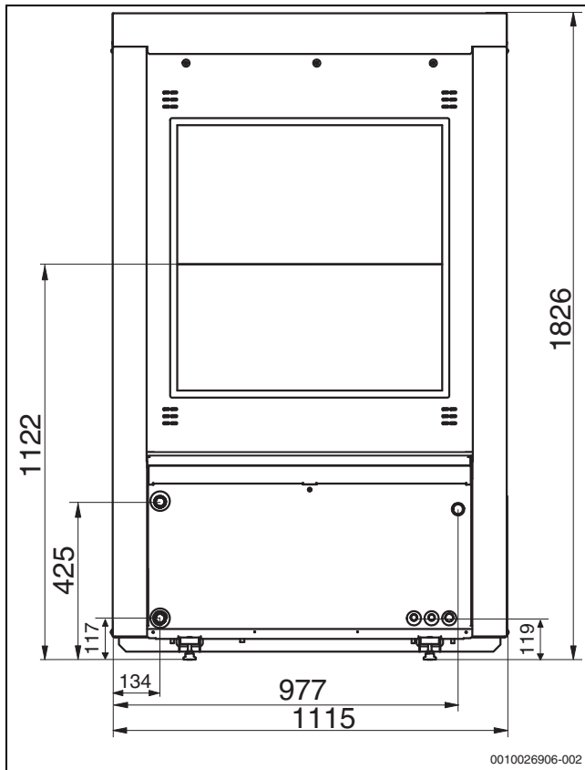
Bild 6 Abmessungen und Anschlüsse der Wärmepumpenmodelle 13–17, Rückseite
