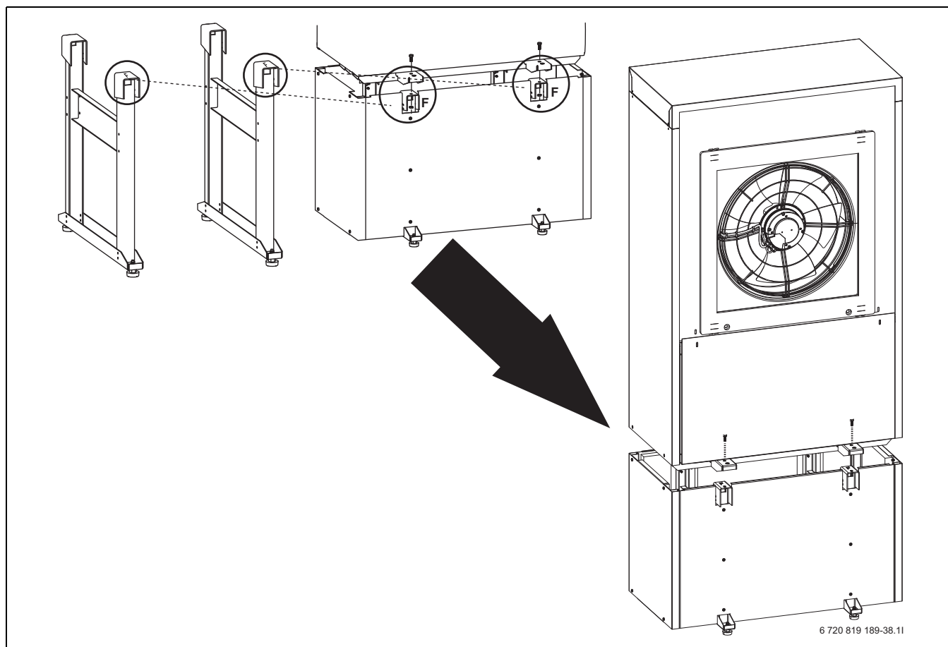
Bild 35 Gestell
