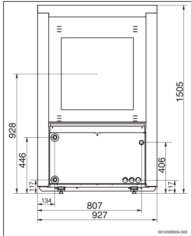
Bild 4 Abmessungen und Anschlüsse der Wärmepumpenmodelle 7–9, Rückseite
