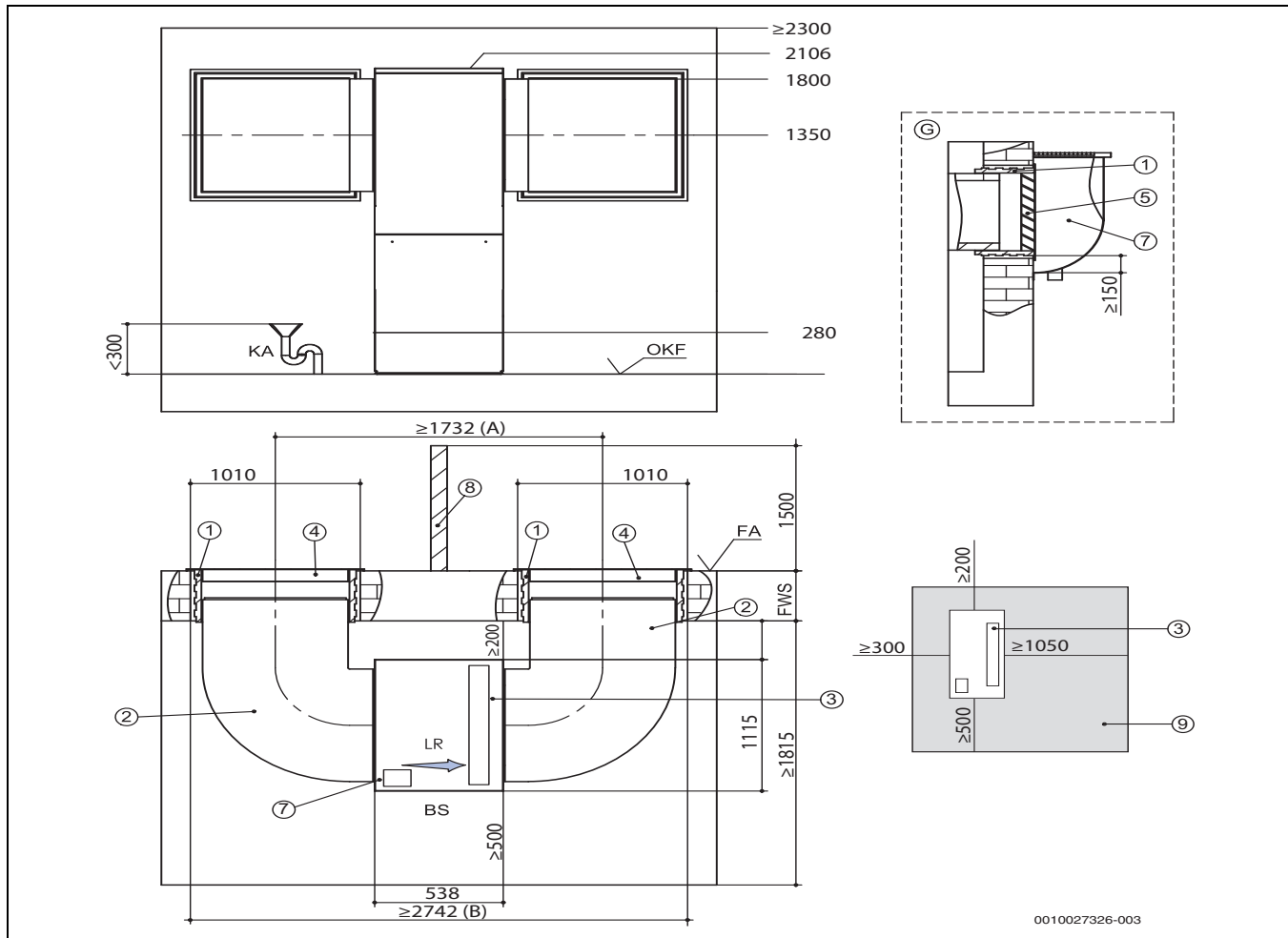
Bild 45 Kanalpläne Variante 3
