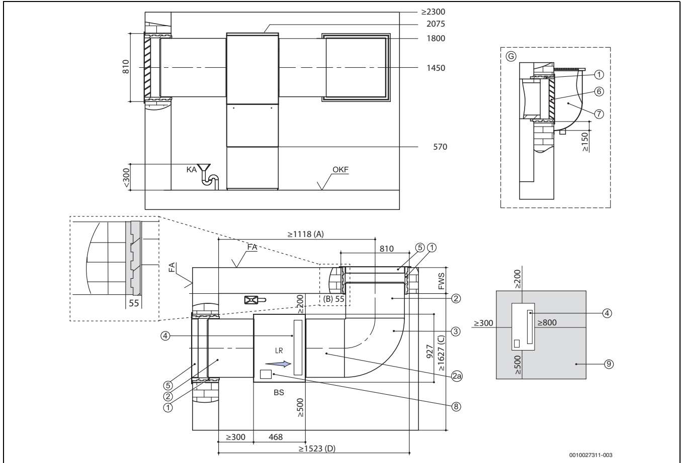
Bild 40 Kanalpläne Variante 1
