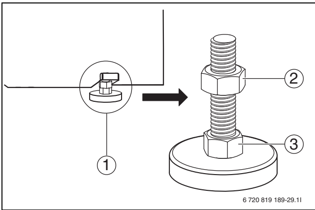
Bild 13 Stellfüße montieren
