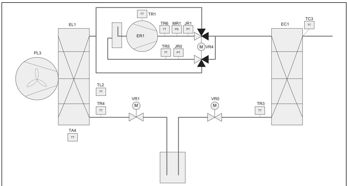
Bild 37 Kältemittelkreis
