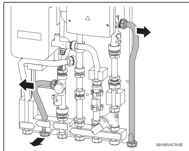
Bild 23 Vor- und Rücklaufrohr demontieren
