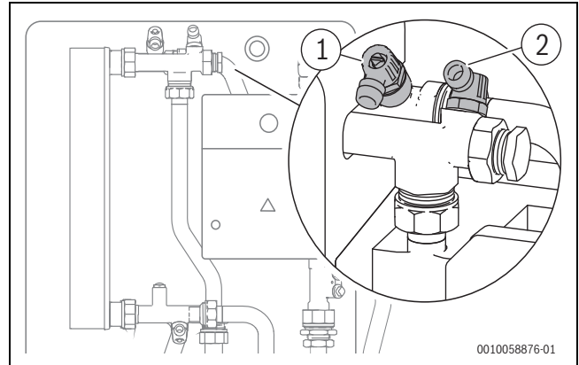
Bild 43 Warmwasser- und Heizkreis/Primärkreis entlüften
