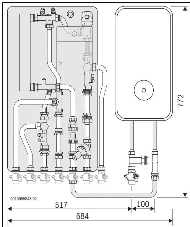
Bild 5 Abstände Station und elektrischer Durchlauferhitzer
