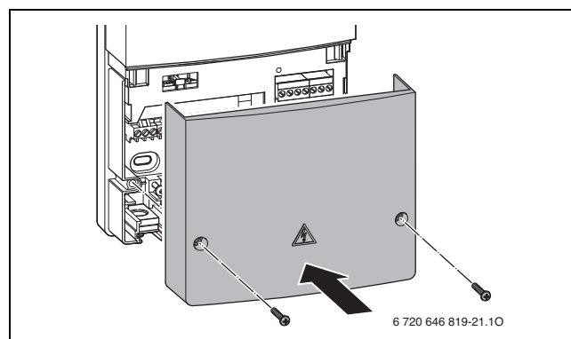
Bild 42 Abdeckung montieren
