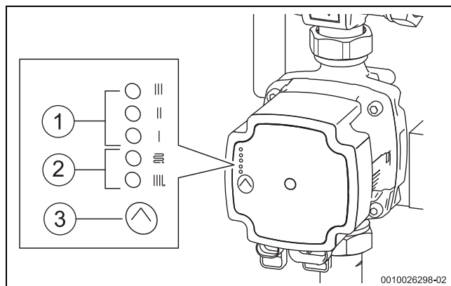
Bild 54 Statusanzeigen der integrierten Heizungspumpe
