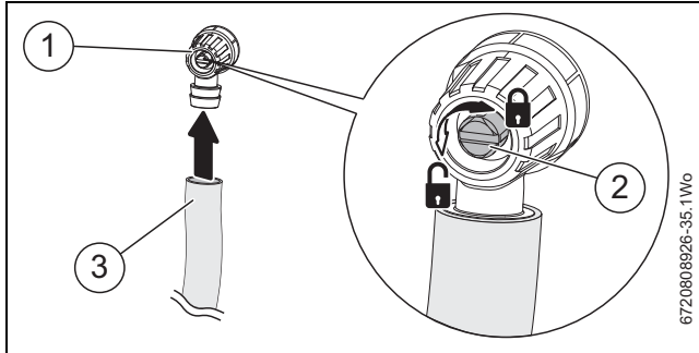
Bild 57 Entleerungsanschluss
