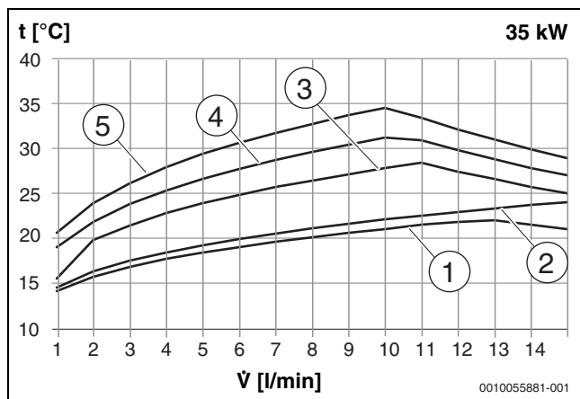
Bild 11 35 kW - Primäre Rücklauftemperatur in Abhängigkeit der primären Vorlauftemperatur und Zapfrate (l/min)
