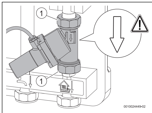
Bild 61 Differenzdruckregler
