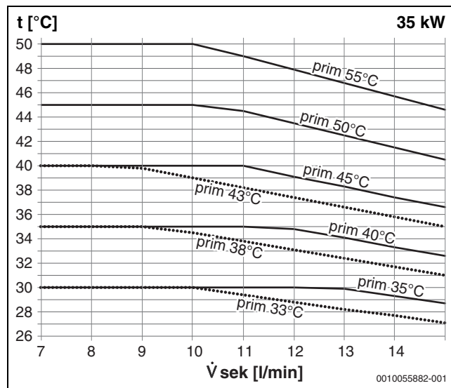
Bild 12 35 kW - Warmwassertemperatur in Abhängigkeit der primären Vorlauftemperatur und Zapfrate (l/min)
