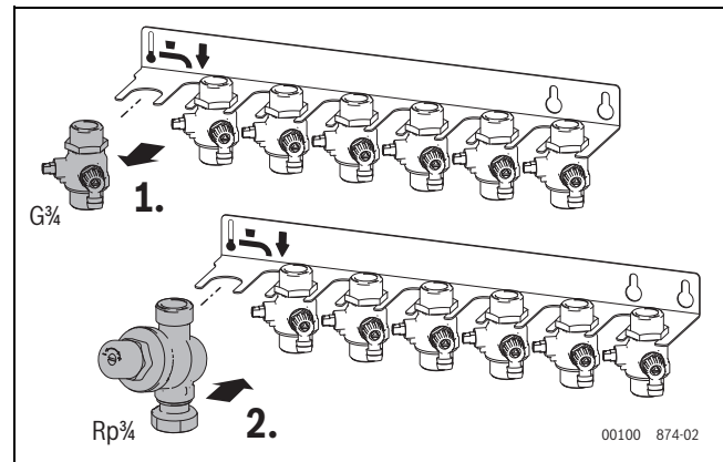
Bild 22 Druckminderer montieren
