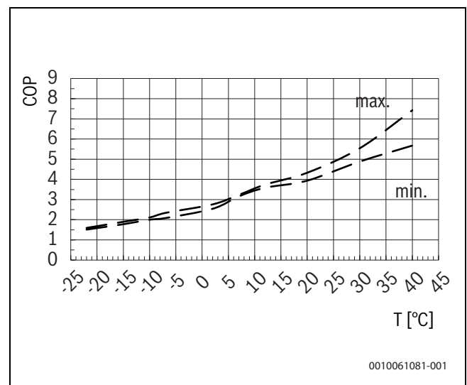
Bild 74 Leistungszahl
