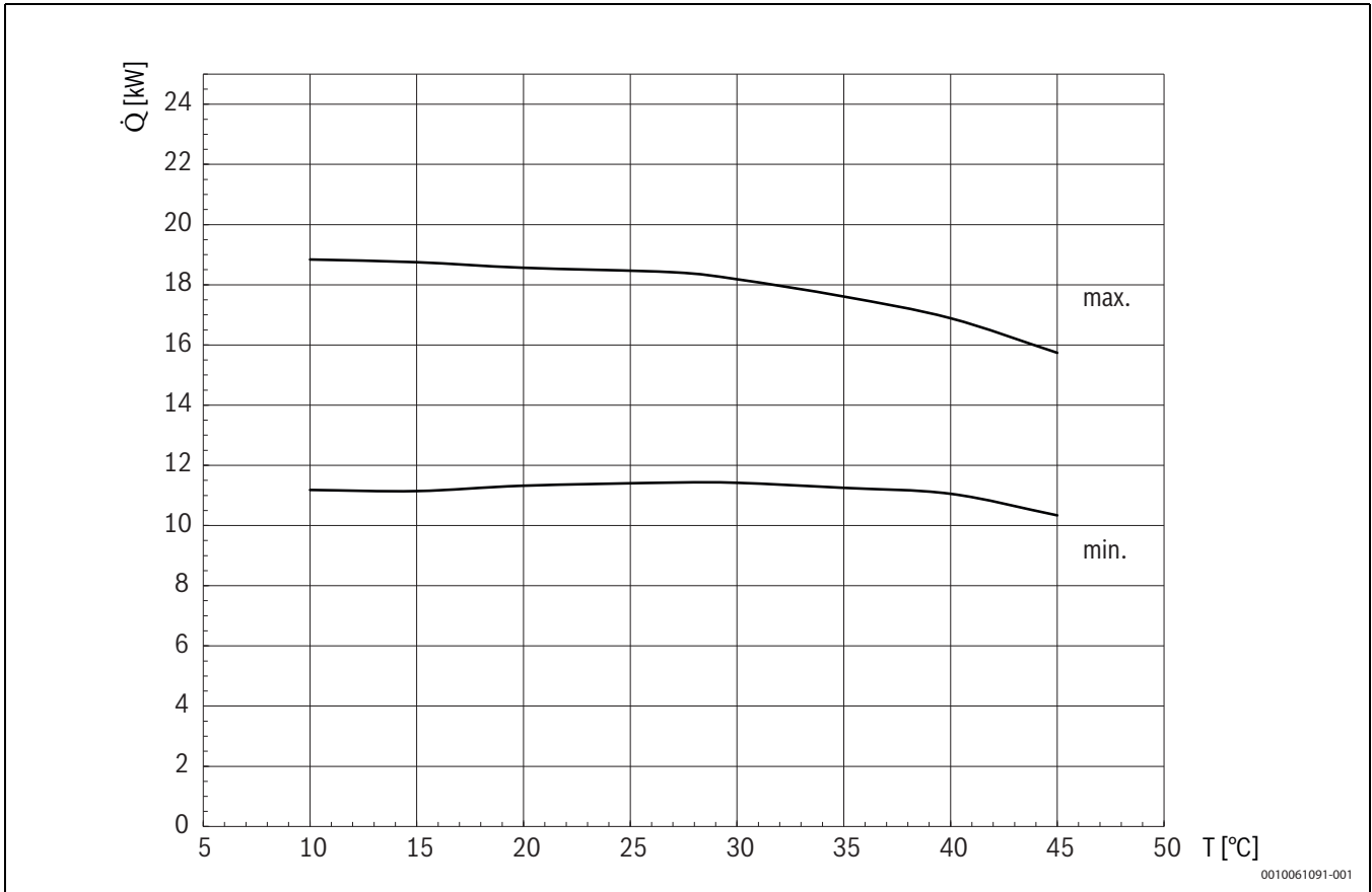
Bild 84 Kühlleistung
