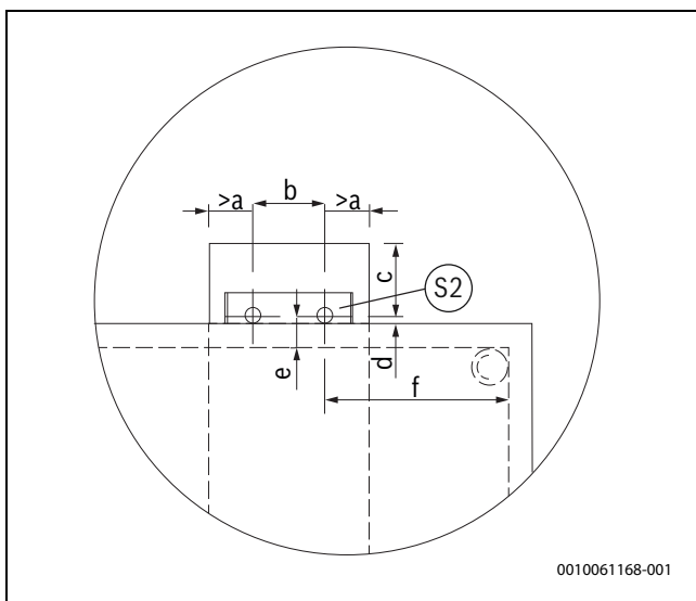
Bild 36 Detail C
