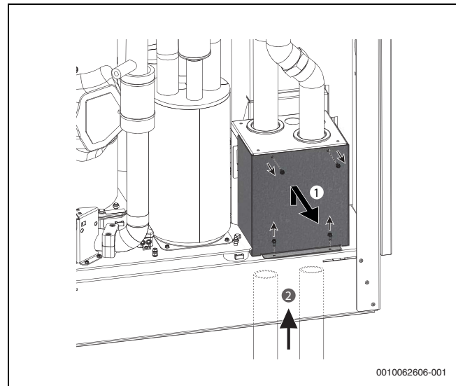
Bild 58 Wasseranschluss installieren
