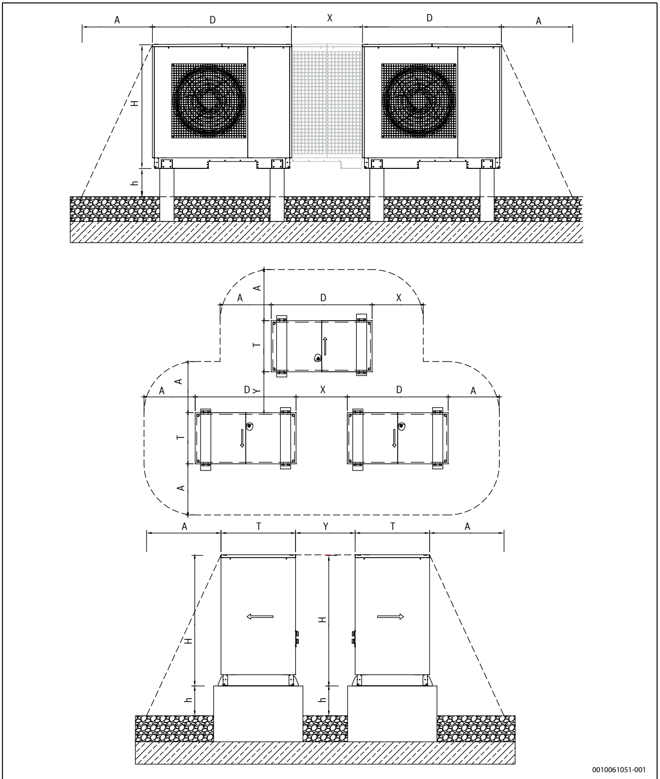
Bild 25 Variante 3 (Legende → Tabelle 8, Seite 21)
