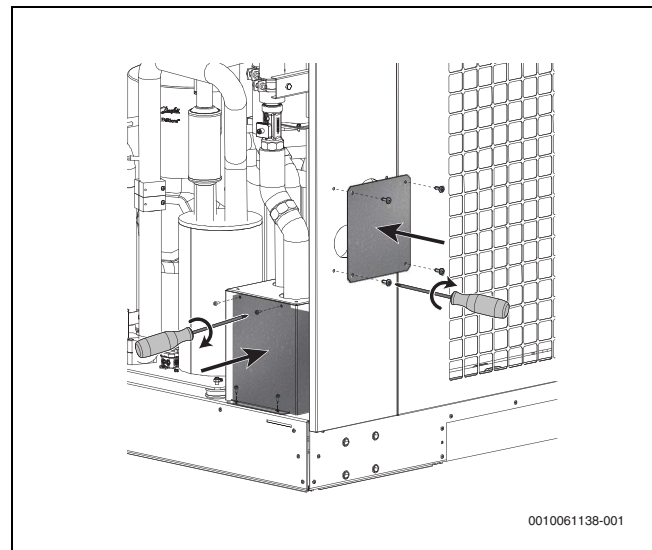
Bild 59 Bleche montieren
