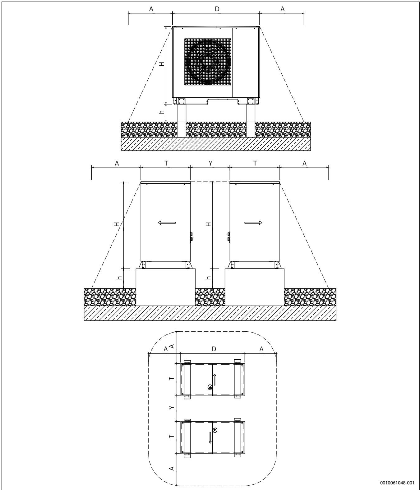
Bild 24 Variante 2 (Legende → Tabelle 8, Seite 21)
