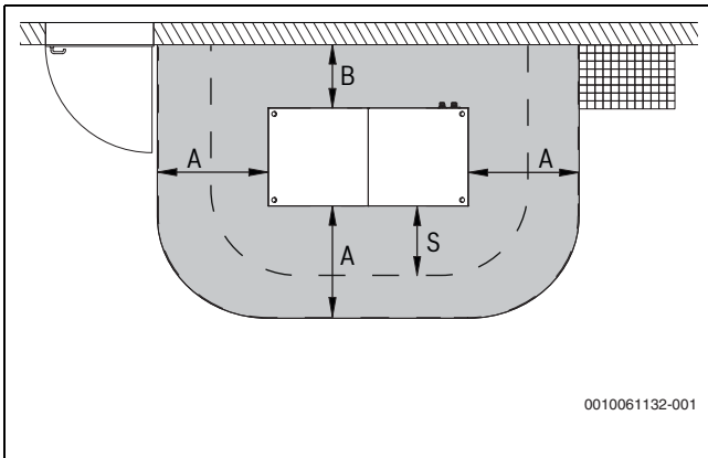
Bild 12 Schutzbereich bei wandnaher Aufstellung mit erhöhter Aufstellung
