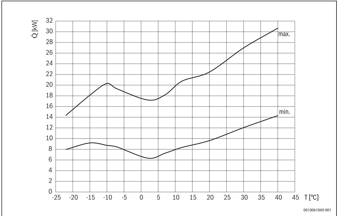
Bild 68 Heizleistung
