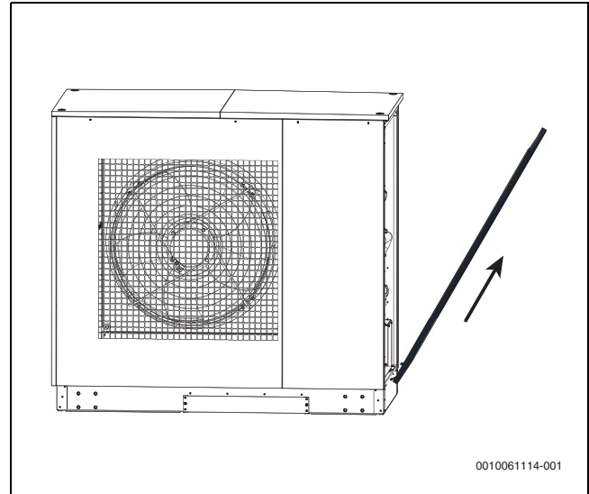
Bild 50 Blechteil entfernen
