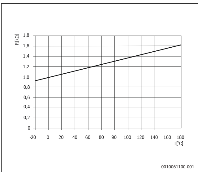
Bild 63 Fühlerkennlinie PT1000
