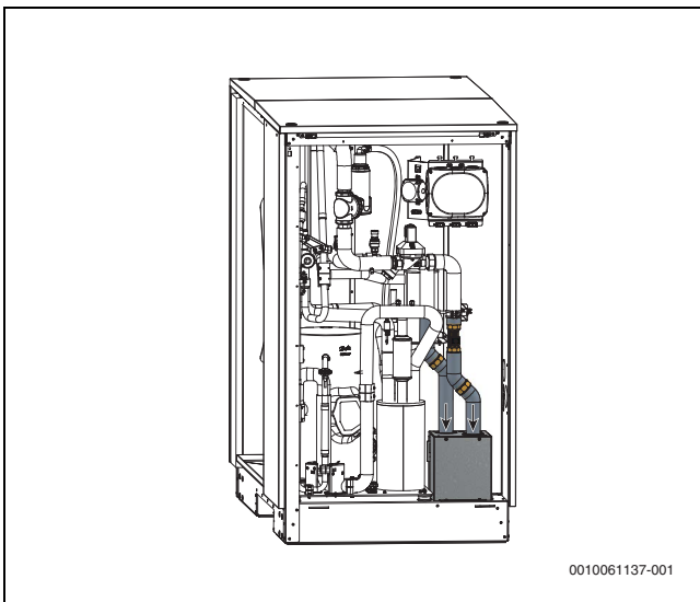
Bild 57 Wasserrohre anschließen
