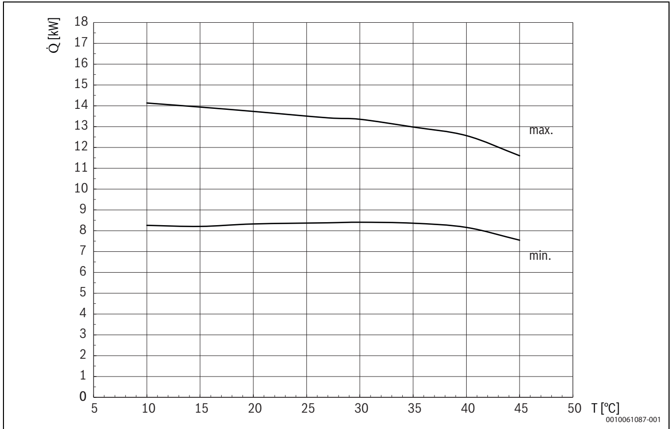
Bild 80 Kühlleistung
