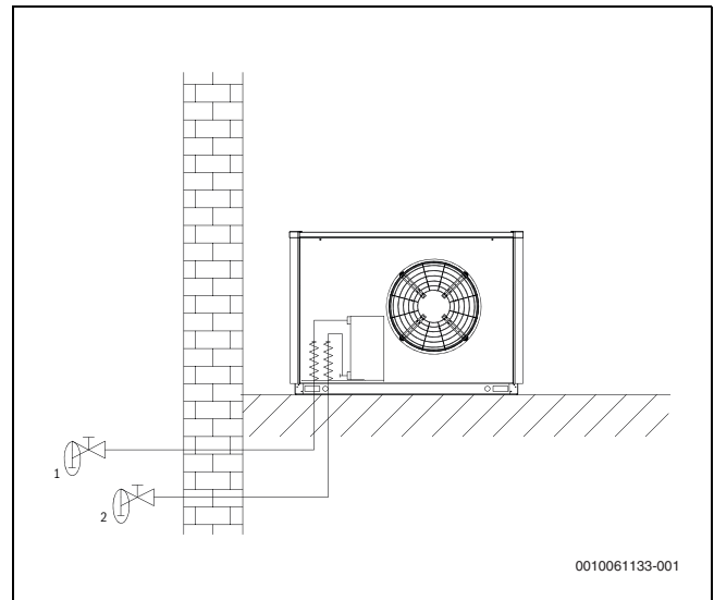
Bild 60 Frostschutz
