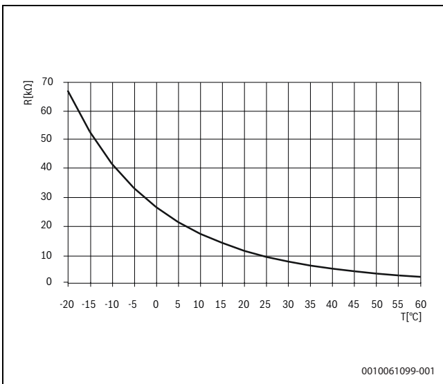
Bild 62 Fühlerkennlinie NTC-10
