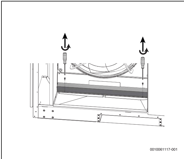
Bild 51 Schraub-Blindniete entfernen
