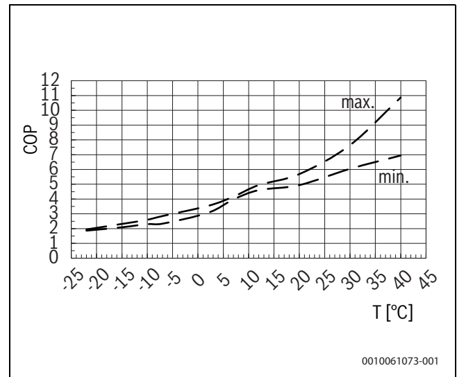
Bild 70 Leistungszahl
