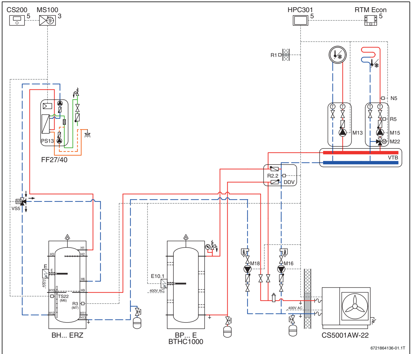
Bild 91 Hydraulische Einbindungsschemata
