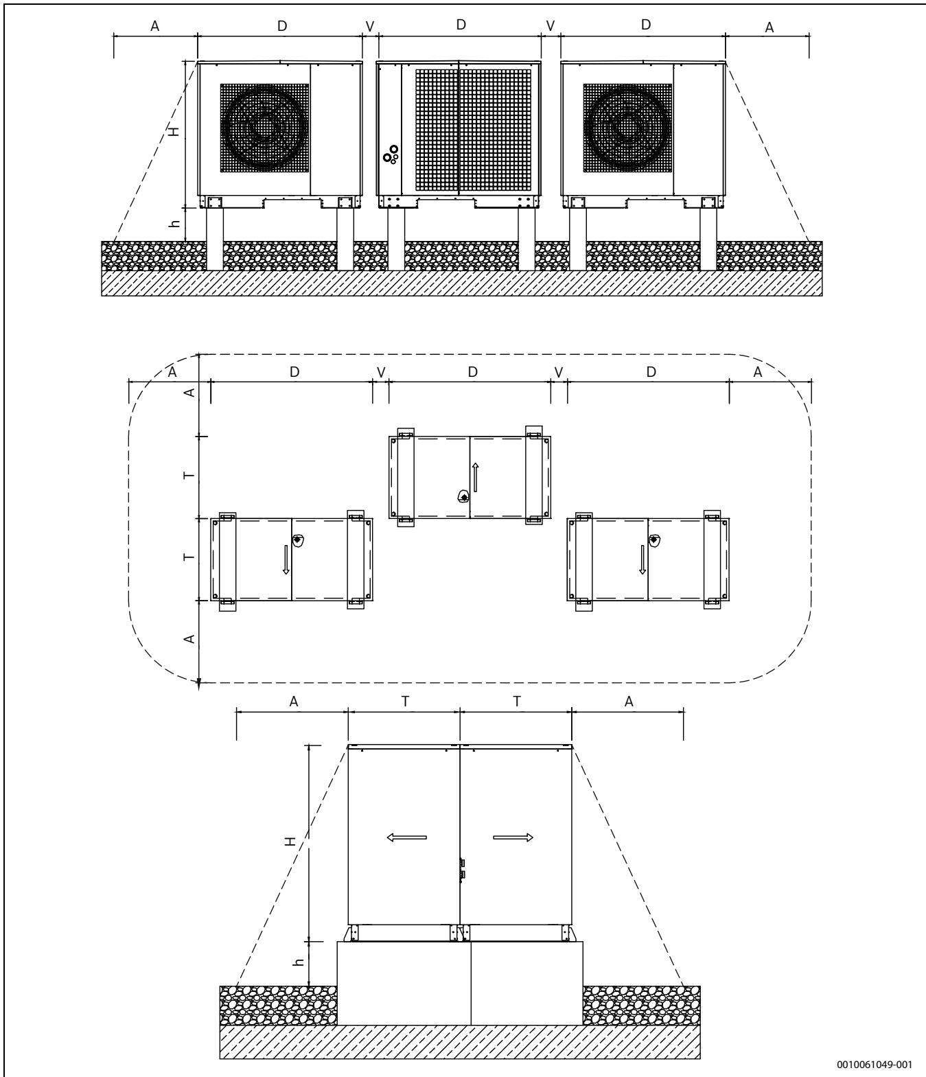
Bild 26 Variante 4 (Legende → Tabelle 8, Seite 21)
