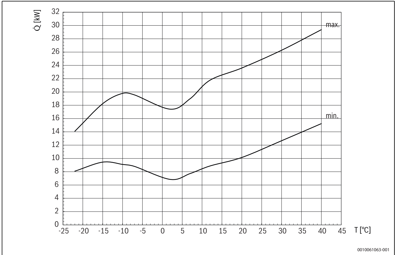
Bild 64 Heizleistung
