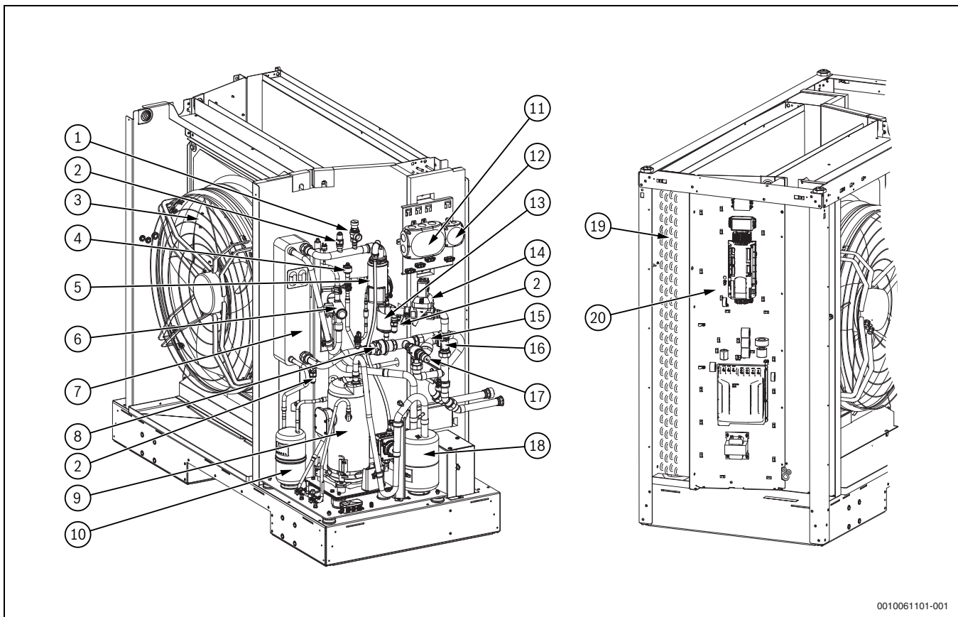
Bild 1 Lieferumfang Wärmepumpe WLW 286.2
