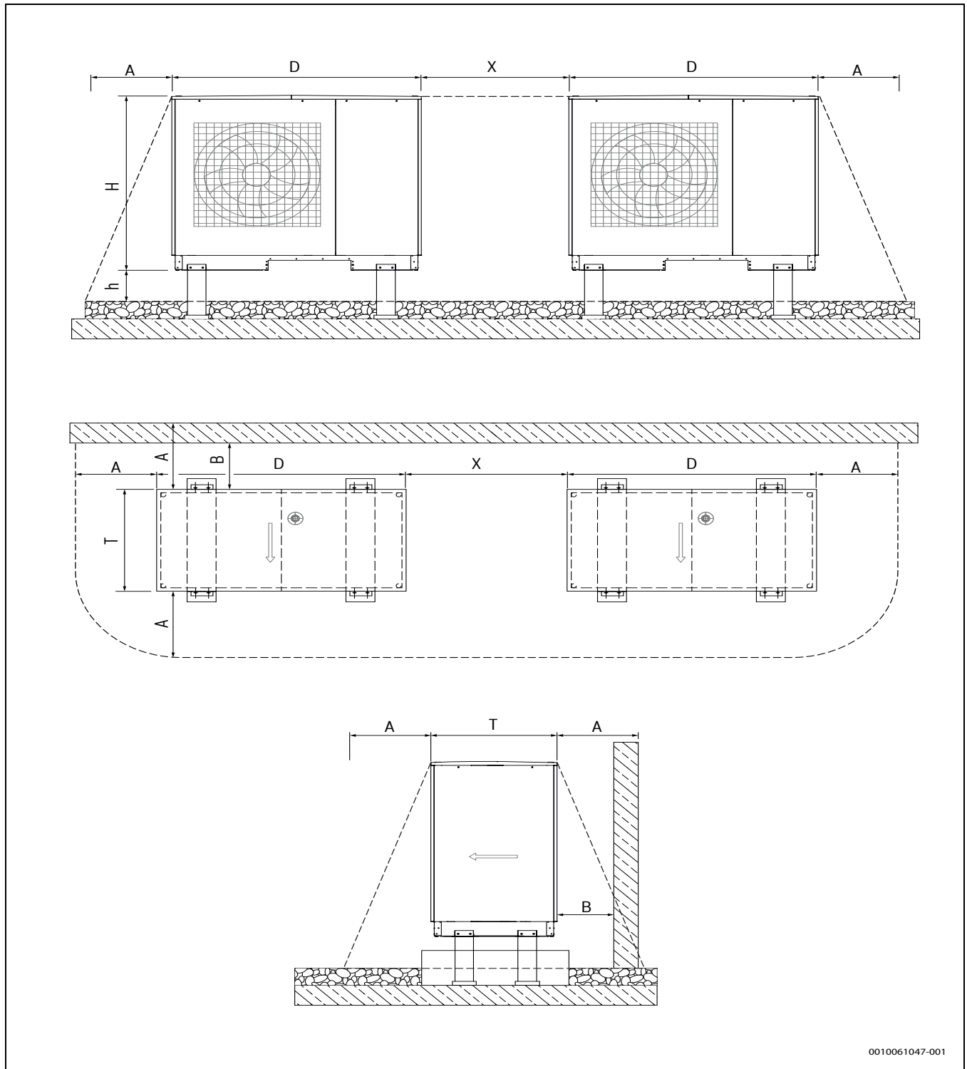
Bild 23 Variante 1 (Legende → Tabelle 8, Seite 21)
