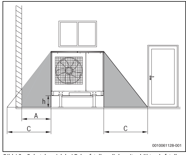
Bild 16 Schutzbereich bei Eckaufstellung links mit erhöhter Aufstellung
