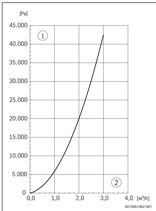
Bild 75 Druckverlust über den Plattenwärmetauscher
