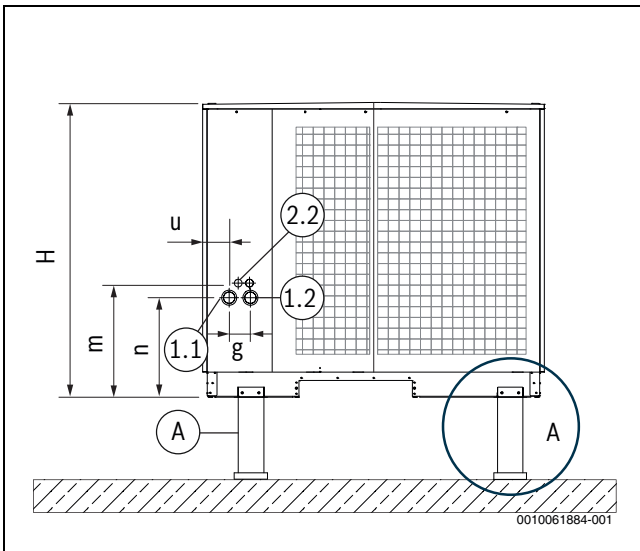
Bild 28 Montagesockel Rückseite
