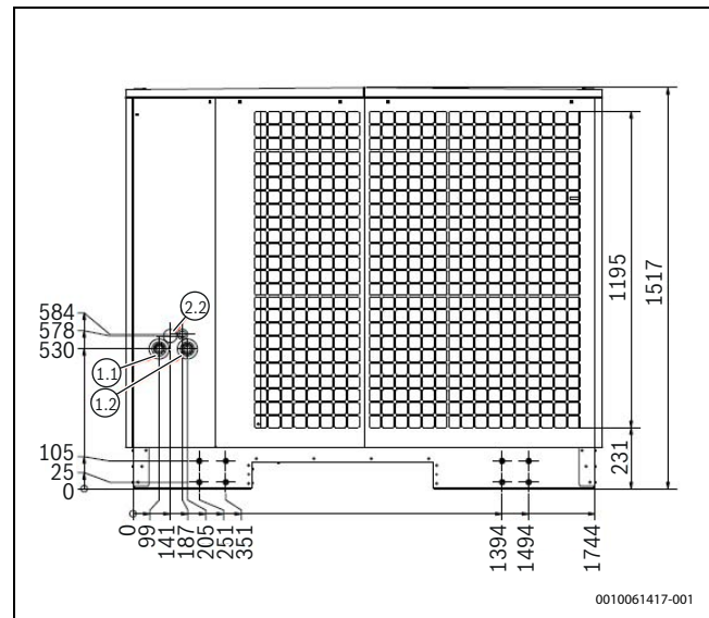
Bild 4 Rückansicht (Maße in [mm])
