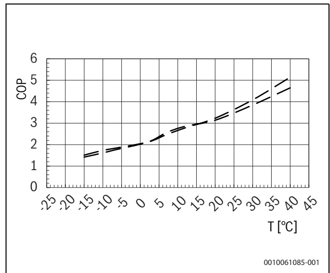
Bild 78 Leistungszahl
