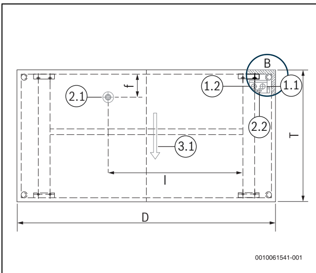
Bild 29 Montagesockel Draufsicht
