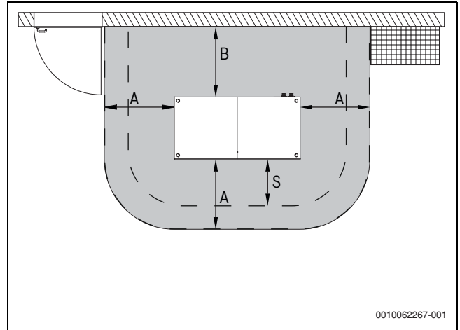
Bild 13 Schutzbereich bei wandnaher Aufstellung mit Bodenaufstellung
