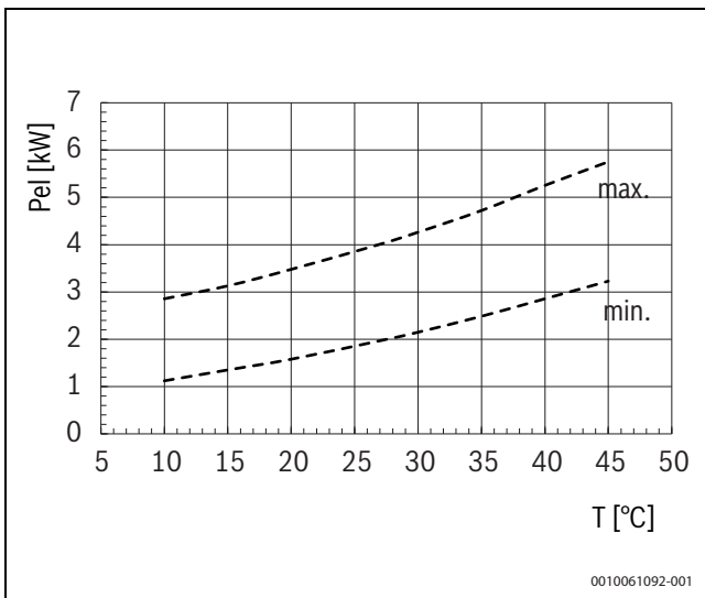
Bild 85 Leistungsaufnahme
