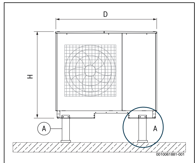
Bild 27 Montagesockel Vorderseite
