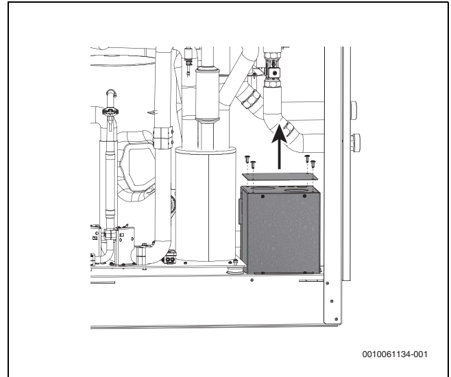
Bild 54 Deckelblech entfernen
