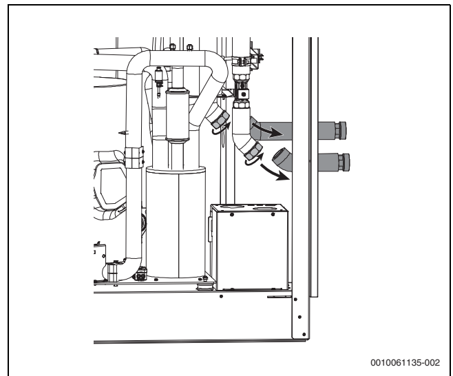
Bild 55 Wasserverrohrung lösen
