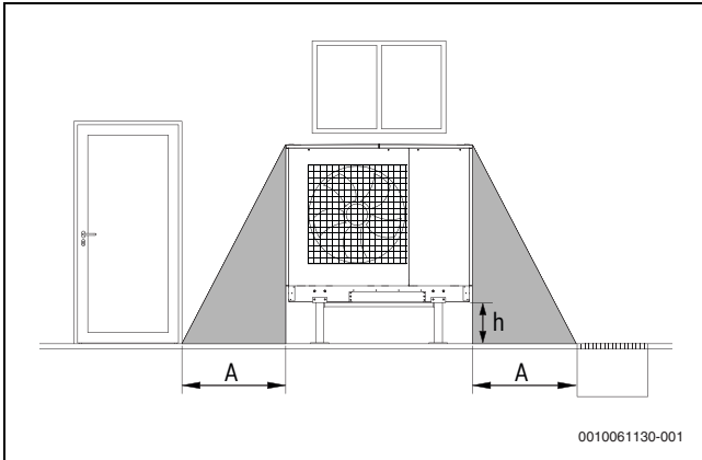
Bild 11 Schutzbereich bei wandnaher Aufstellung
