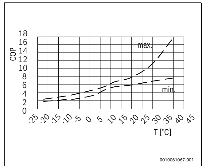
Bild 66 Leistungszahl
