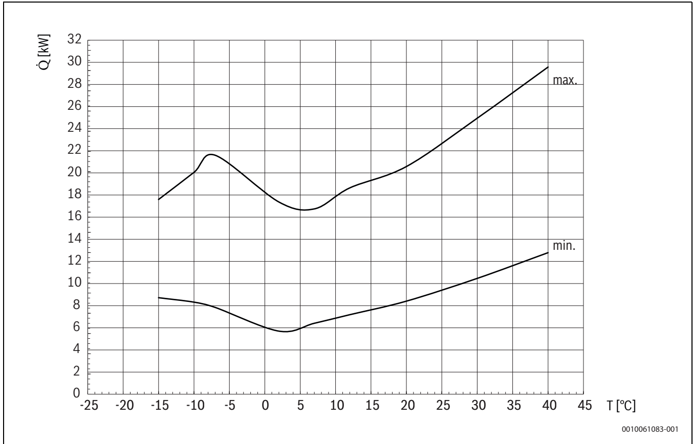
Bild 76 Kennlinie Heizleistung
