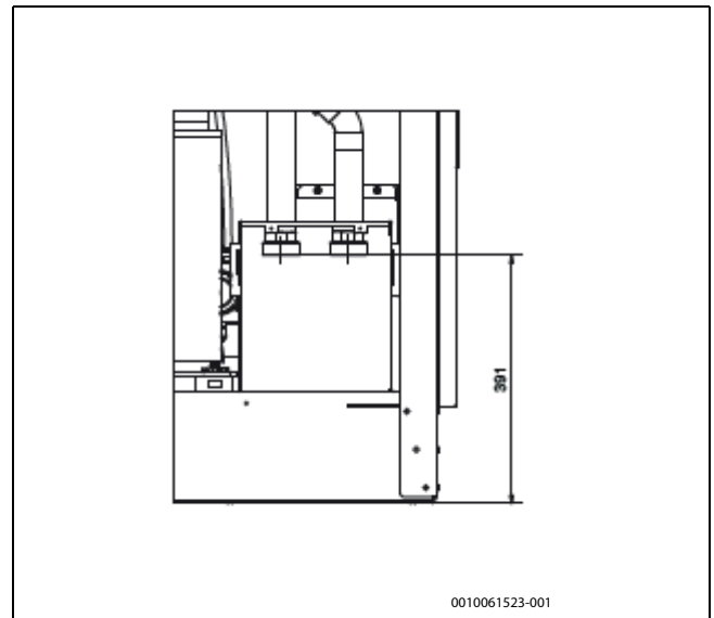
Bild 7 Seitenansicht- Anschluss von unten (Maße in [mm])
