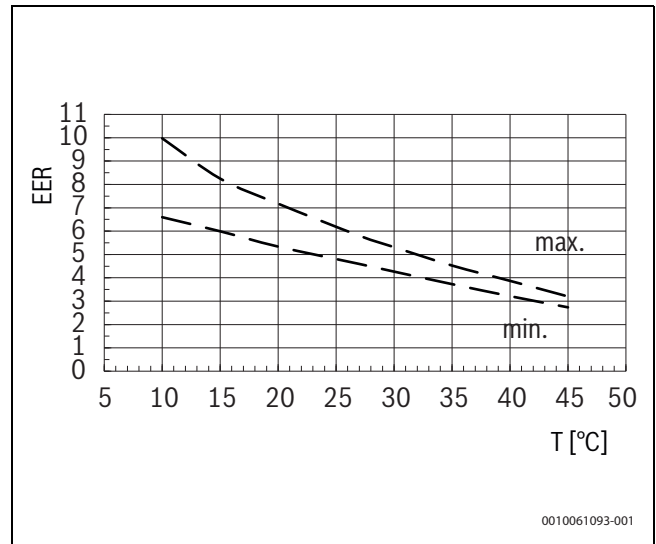
Bild 86 Leistungszahl
