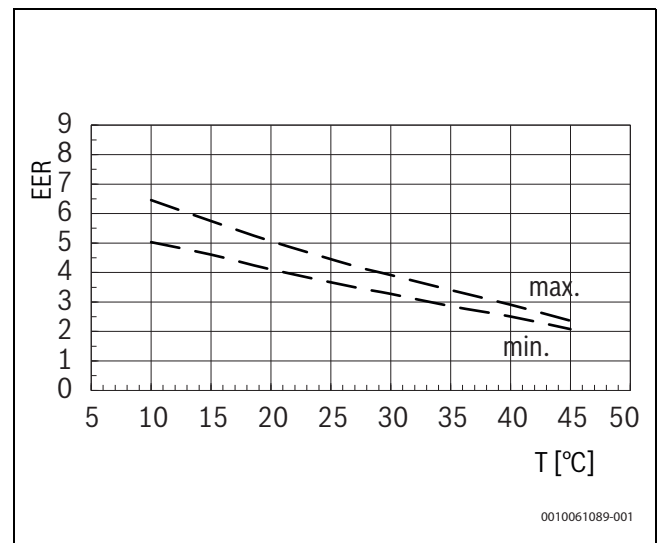
Bild 82 Leistungszahl
