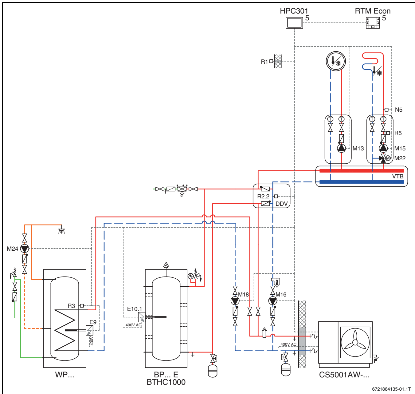
Bild 92 Hydraulische Einbindungsschemata
