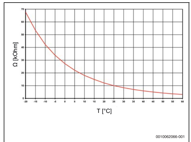
Bild 4 Fühlerkennlinie NTC-10
