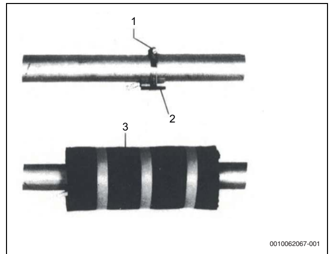
Bild 6 Rohranlegefühler montieren
