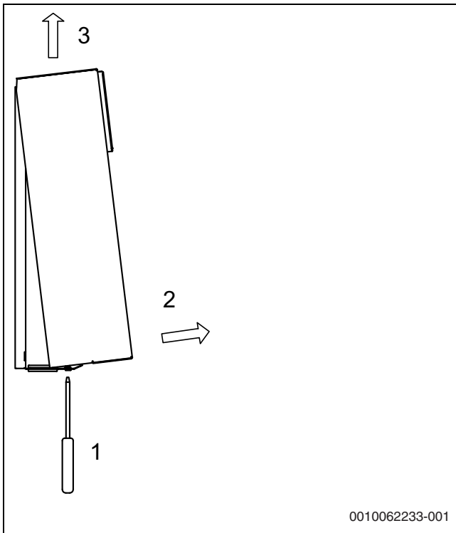
Bild 3 Wandmontage
