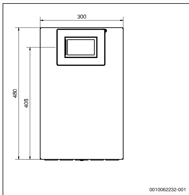
Bild 2 Frontansicht (mm)
