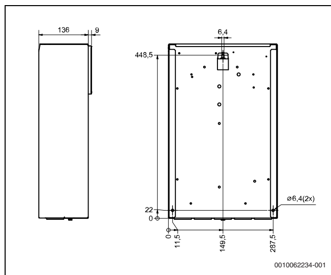
Bild 1 Seitenansicht (mm)
