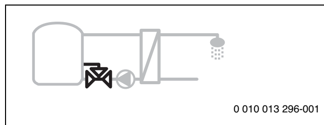
Bild 30 Ventil Rücklauf
