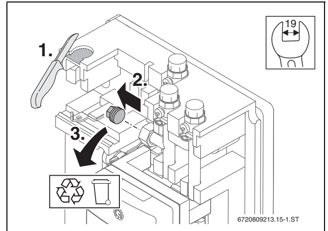
Bild 23 Montage vorbereiten
