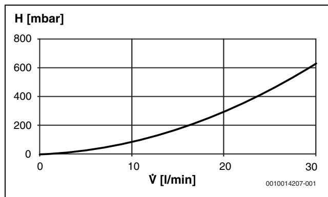
Bild 7 Druckverlust Sekundärseite
