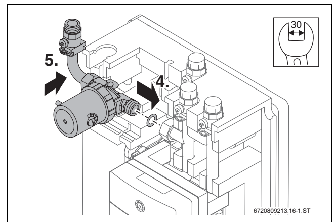
Bild 24 Montage vorbereiten
