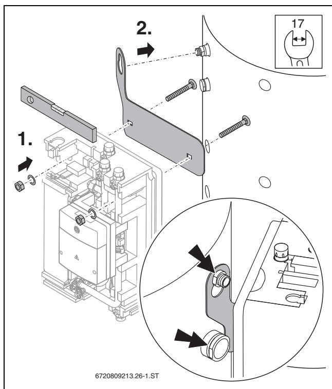
Bild 14 Halblech montieren
