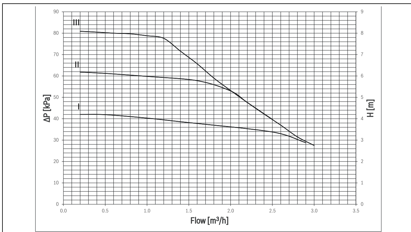
Bild 45 Restförderhöhe Heizkreispumpe für den Anschluss an den ungemischten Heizkreis für PC1 im Betrieb mit konstantem Druck
