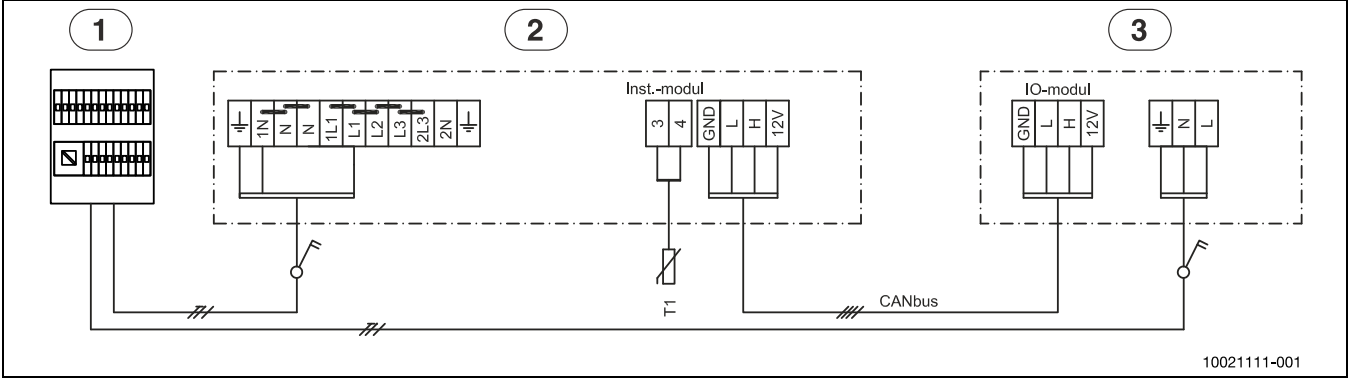
Bild 52 Schaltplan 1N~ 1)
