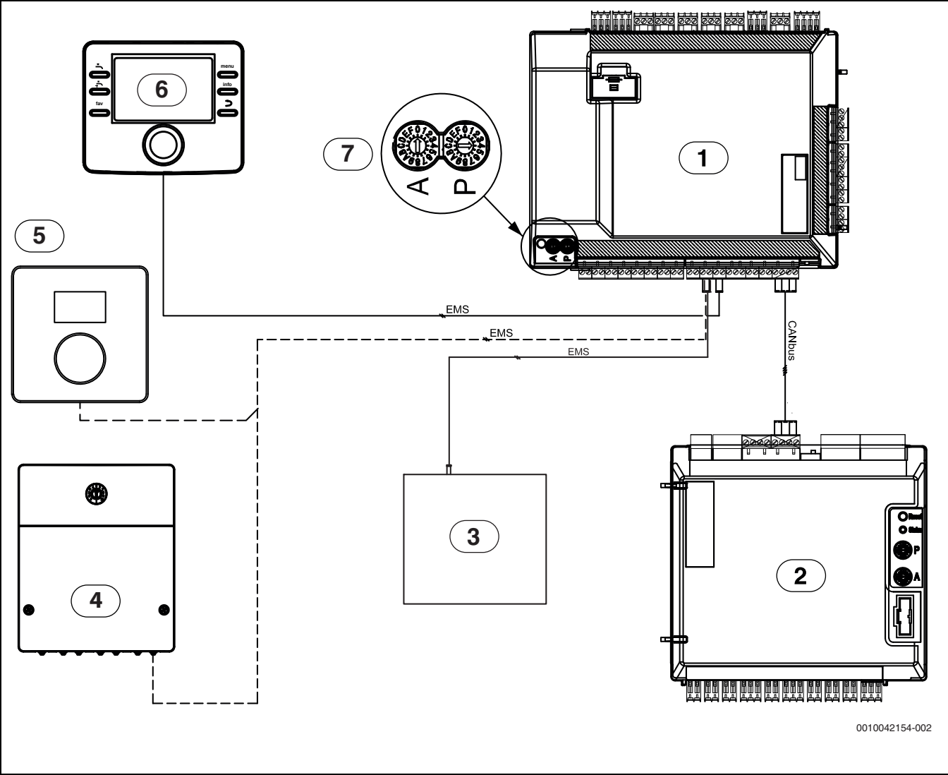
Bild 56 Schaltplan/Inneneinheit
