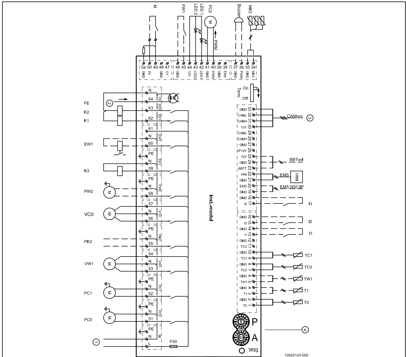
Bild 55 Schaltplan Installationsmodul
