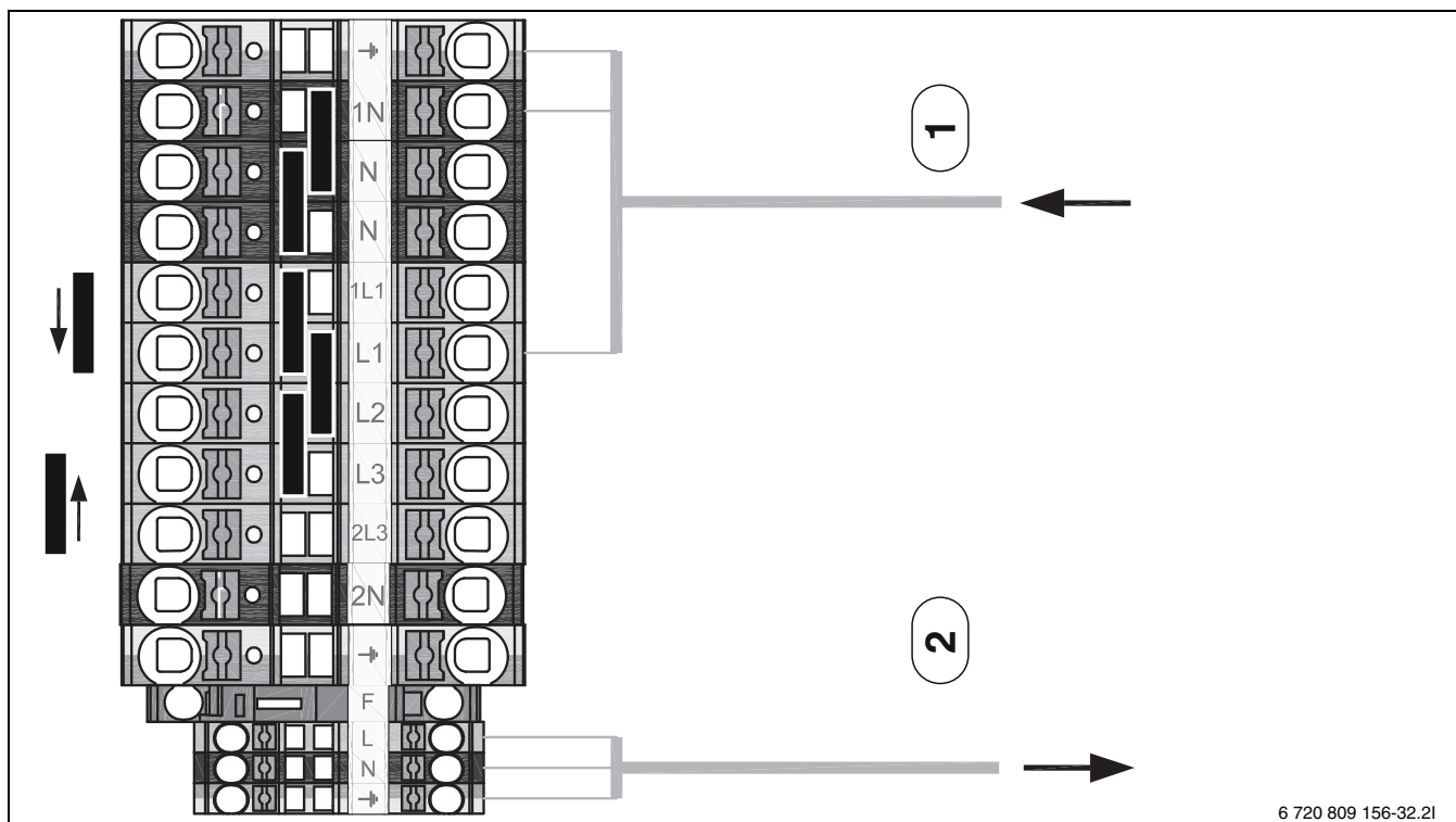
Bild 25 Klemmenbelegung im Klemmenkasten
