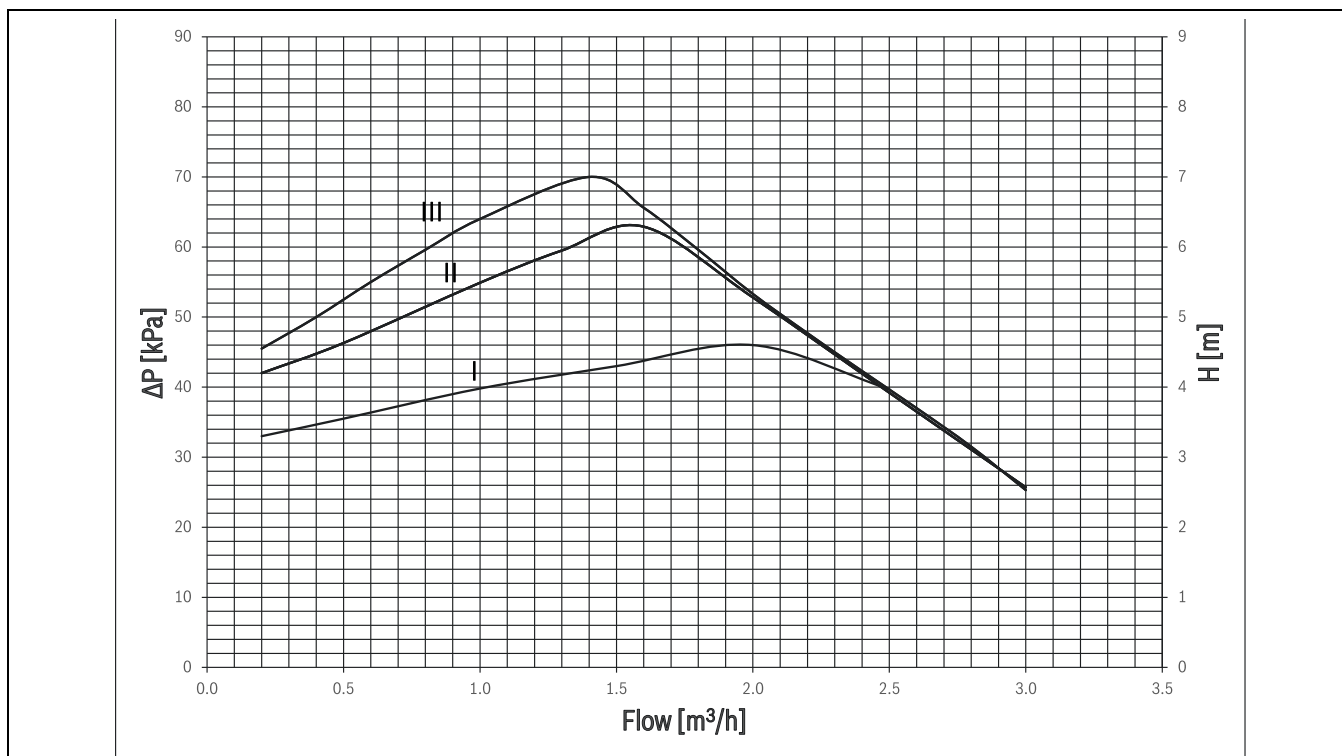
Bild 44 Restförderhöhe Heizkreispumpe für den Anschluss an den ungemischten Heizkreis für PC1 im Betrieb mit proportionalem Druck
