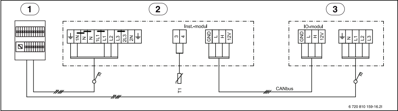
Bild 51 Schaltplan 3 N~
