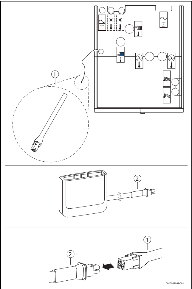
Bild 18 Anschluss des Funkmodul.
