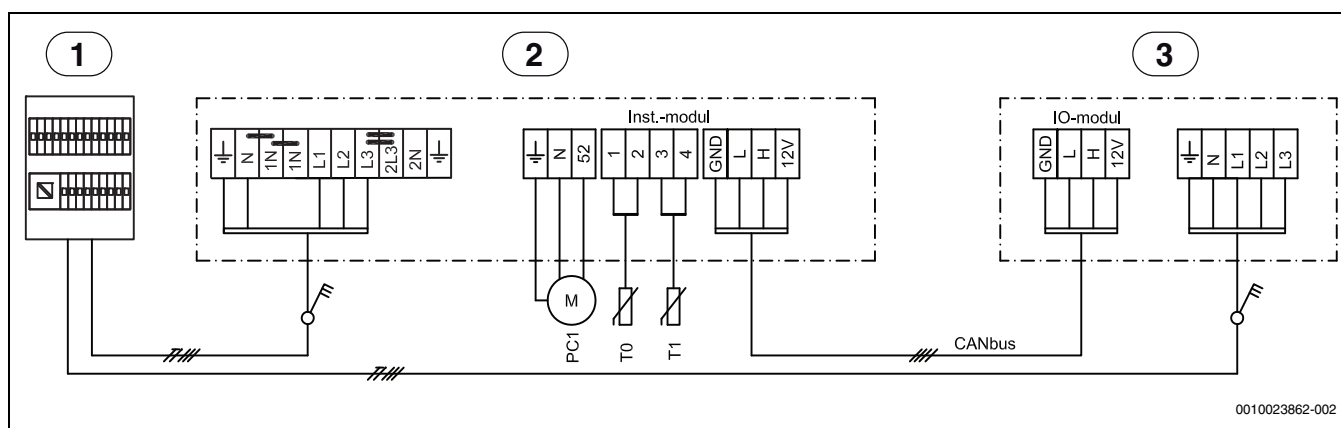
Bild 30 Anschlussplan 9 kW (Drehstrom)
