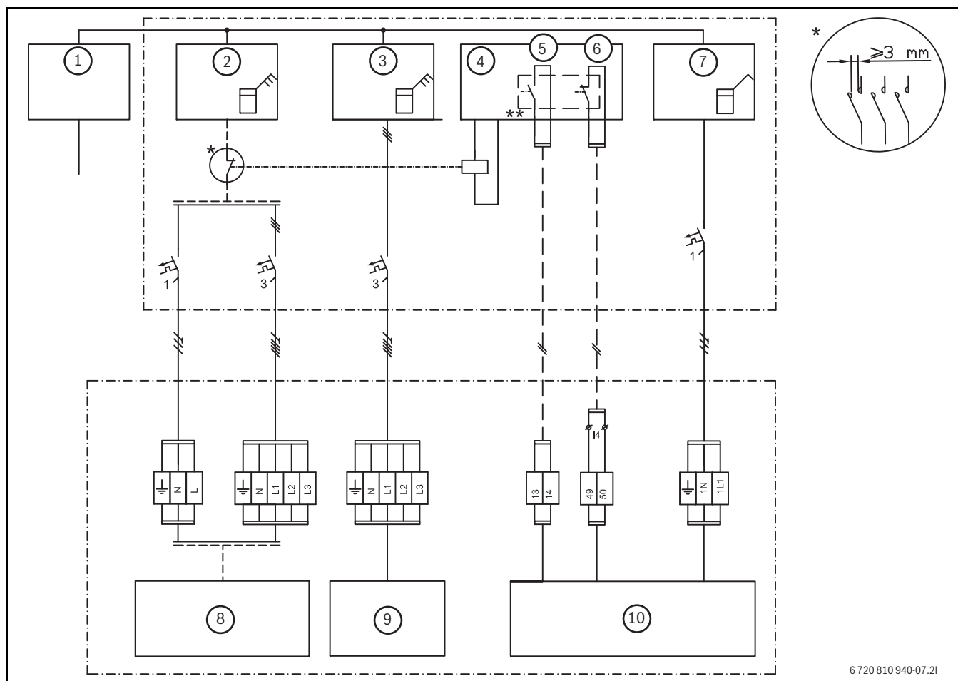
Bild 39 EVU Typ 2
