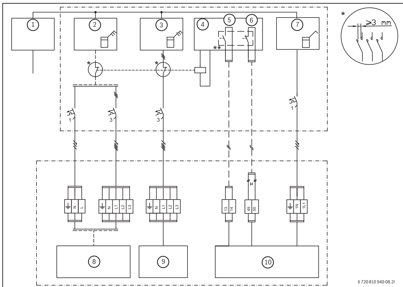
Bild 38 EVU Typ 1
