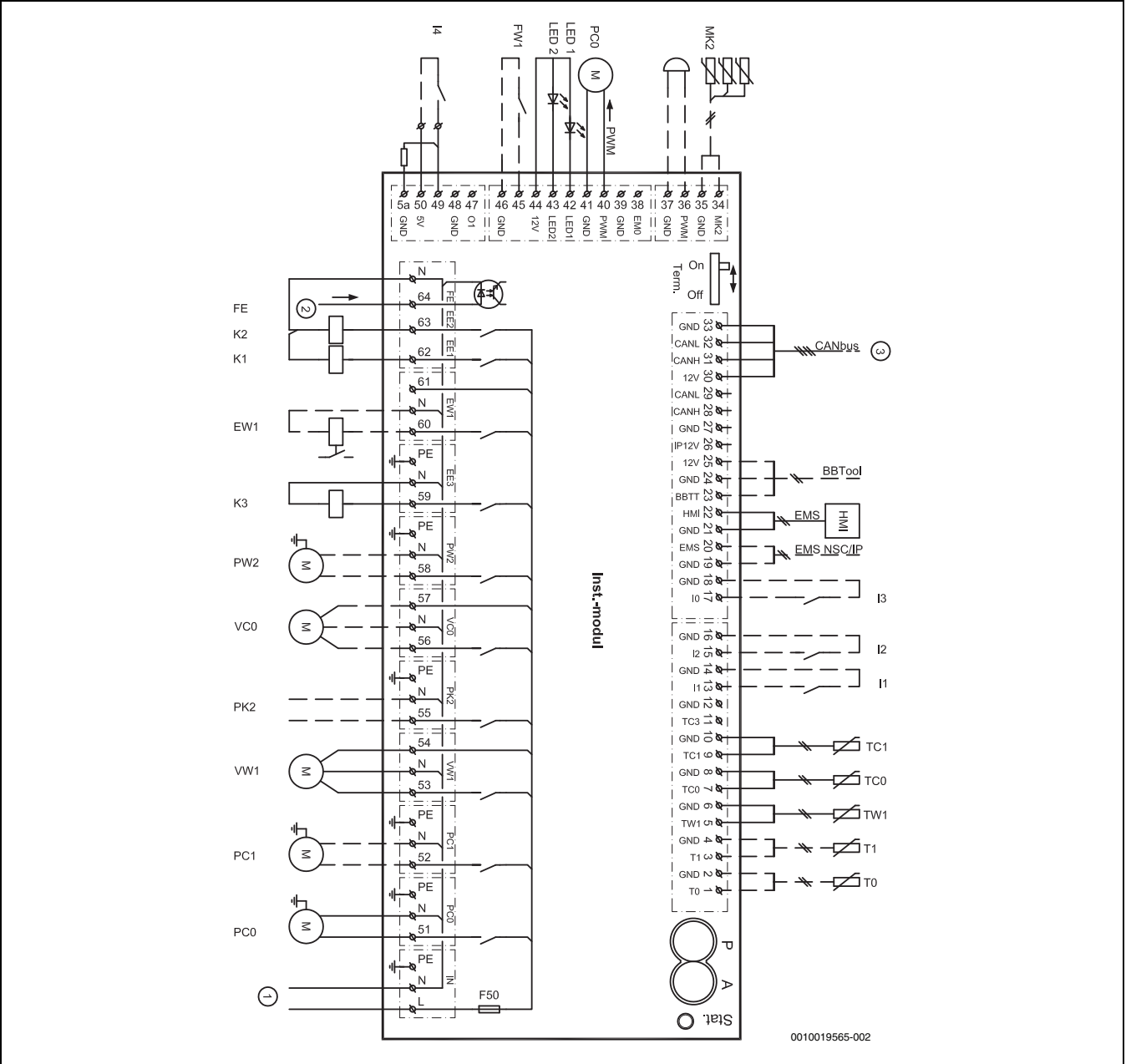
Bild 32 Schaltplan, Installationsmodul
