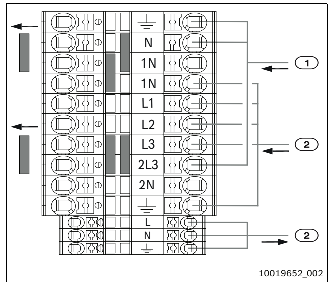
Bild 35 Klemmenanschlüsse und Anordnung der Brücken
