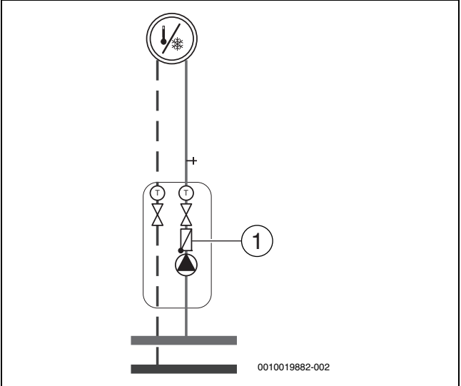
Bild 28 Heizkreis
