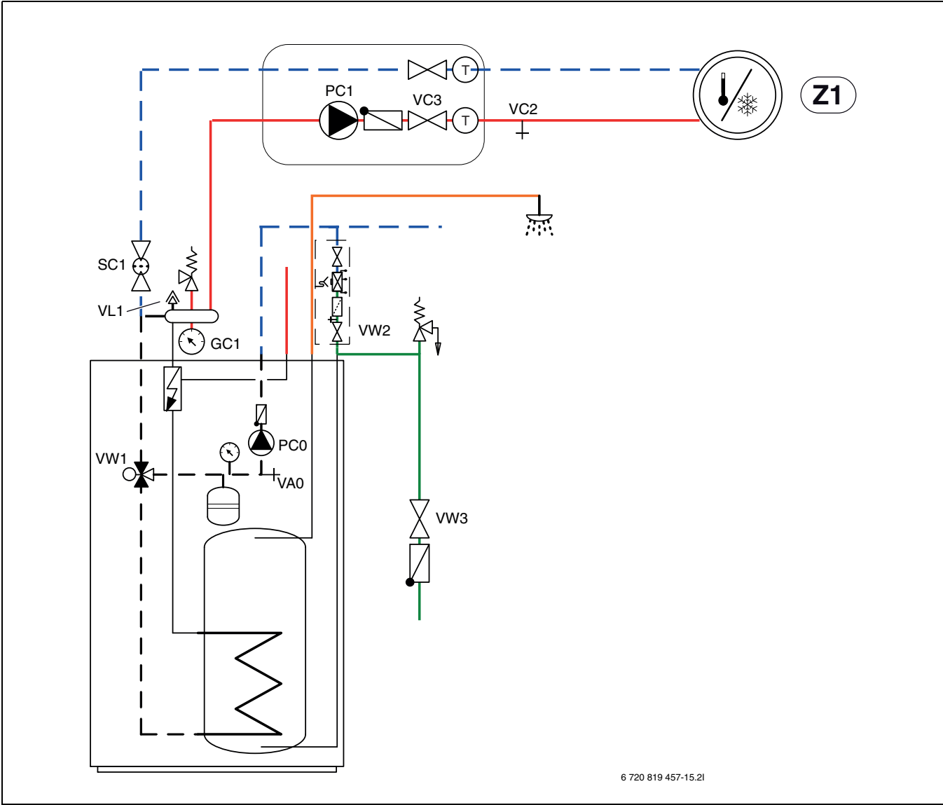
Bild 22 Inneneinheit und Heizungsanlage
