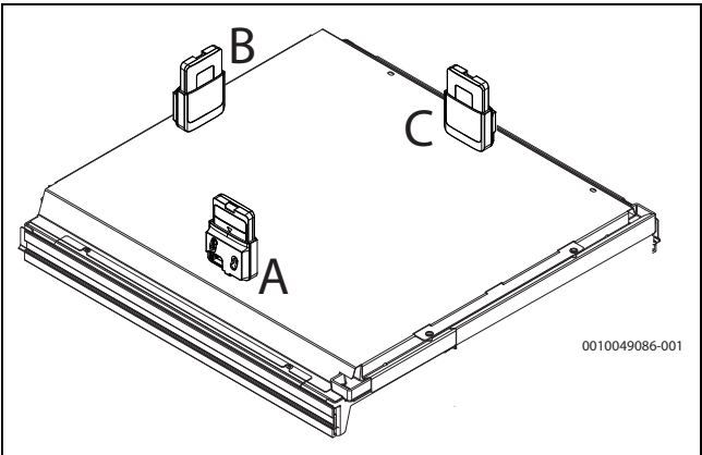
Bild 19 Befestigung des Halters an der oberen Abdeckung der Inneneinheit. Neben dem Halter zeigt die Abbildung auch das im Halter sitzende Funkmodul
