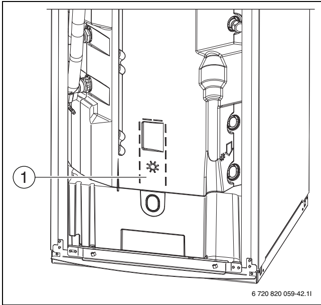
Bild 25 Anordnung von Temperaturfühler TW1 und ggf. TS2
