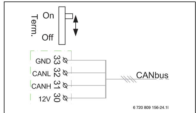
Bild 13 CAN-BUS-Terminierung
