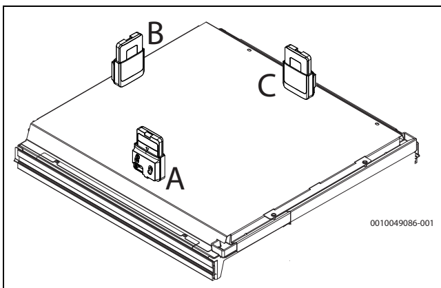
Bild 17 Befestigung des Halters an der oberen Abdeckung der Inneneinheit. Neben dem Halter zeigt die Abbildung auch das im Halter sitzende Funkmodul
