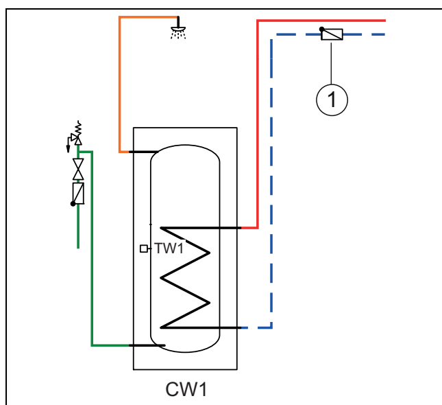
Bild 24 Warmwasserspeicher
