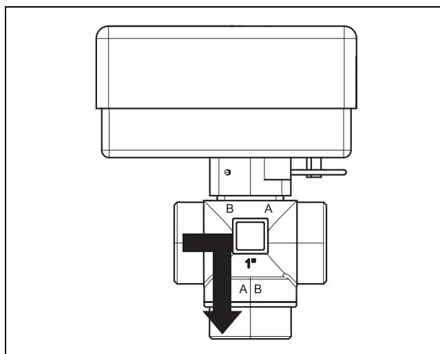
Bild 27 Kontakt offen, Anschluss B offen
