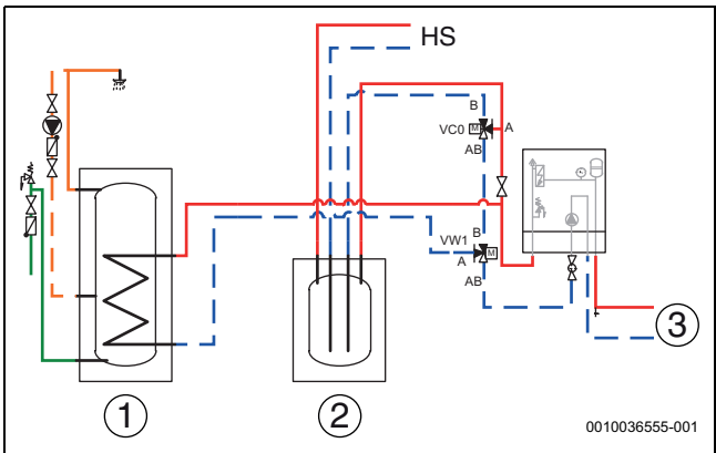
Bild 30 Puffer, VC0-Bypassventil
