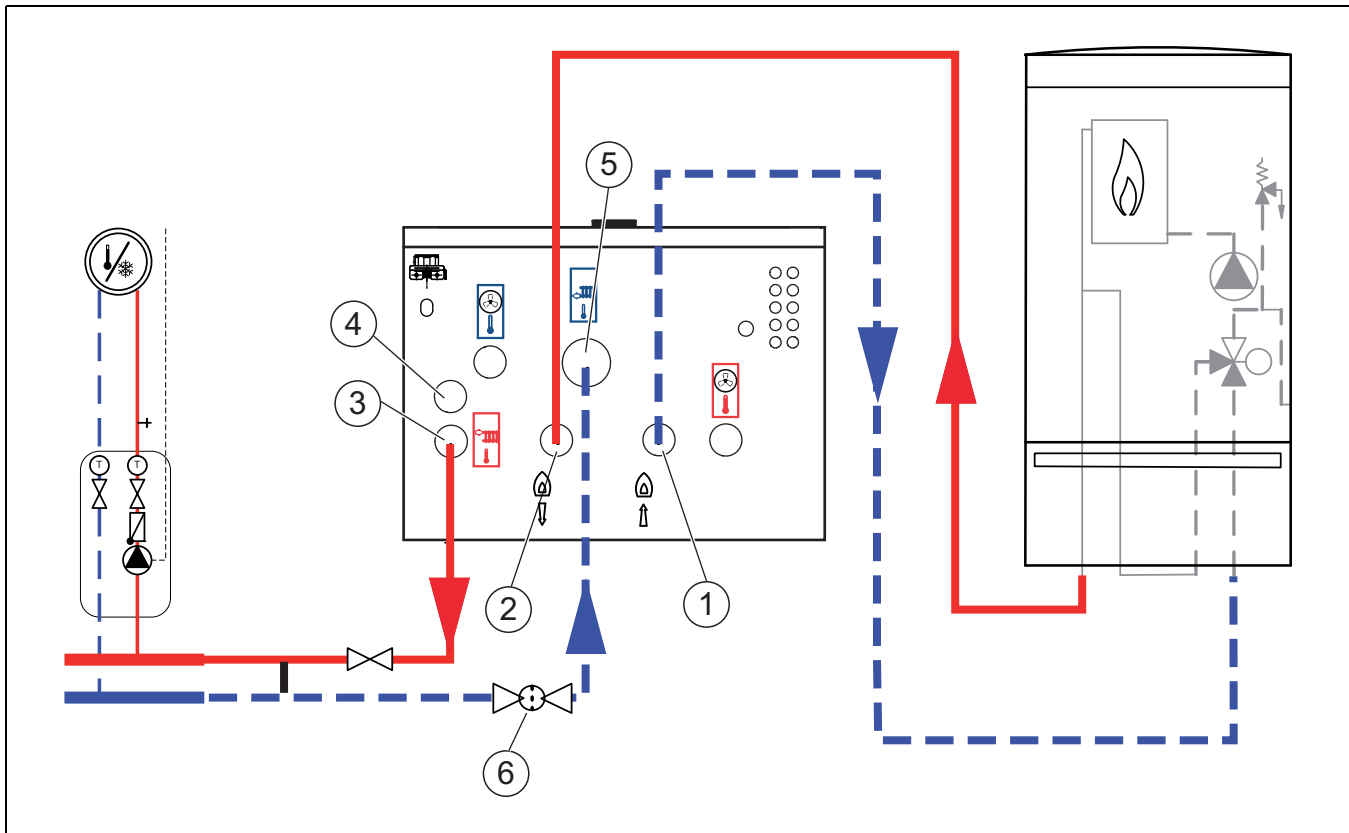
Bild 8 Anschluss der Inneneinheit mit Mischer für externen Zuheizer an die Heizungsanlage und den Zuheizer
