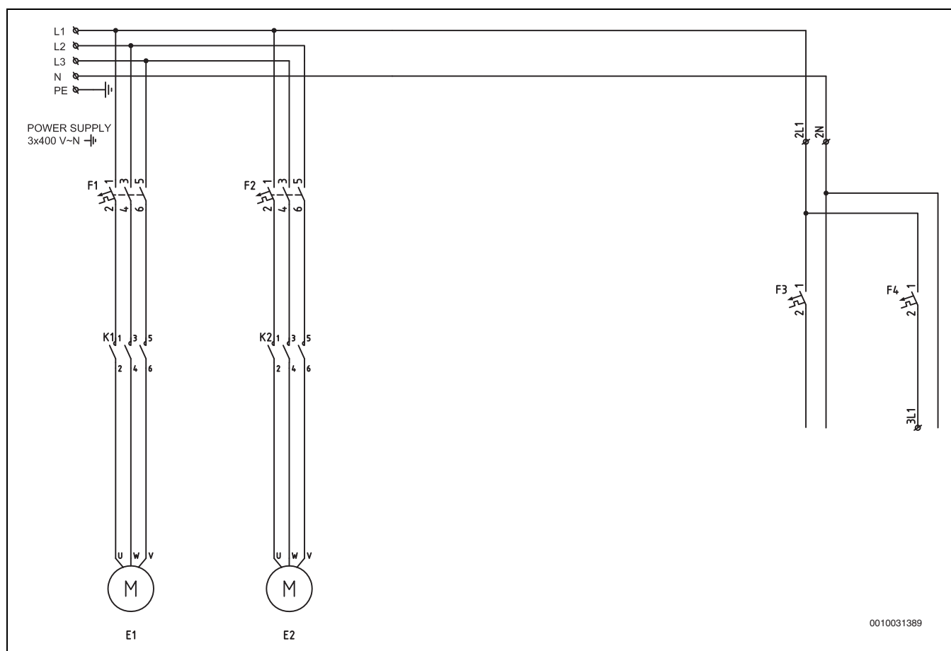
Bild 24 Betriebsschaltplan mit Schütz
