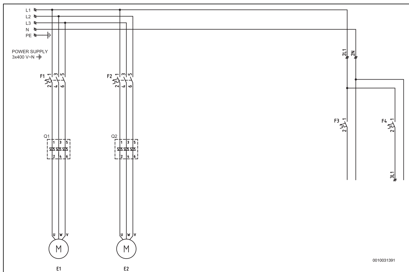
Bild 25 Betriebsschaltplan, Anlaufstrombegrenzer
