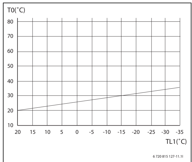
Bild 3 Fußbodenheizung
