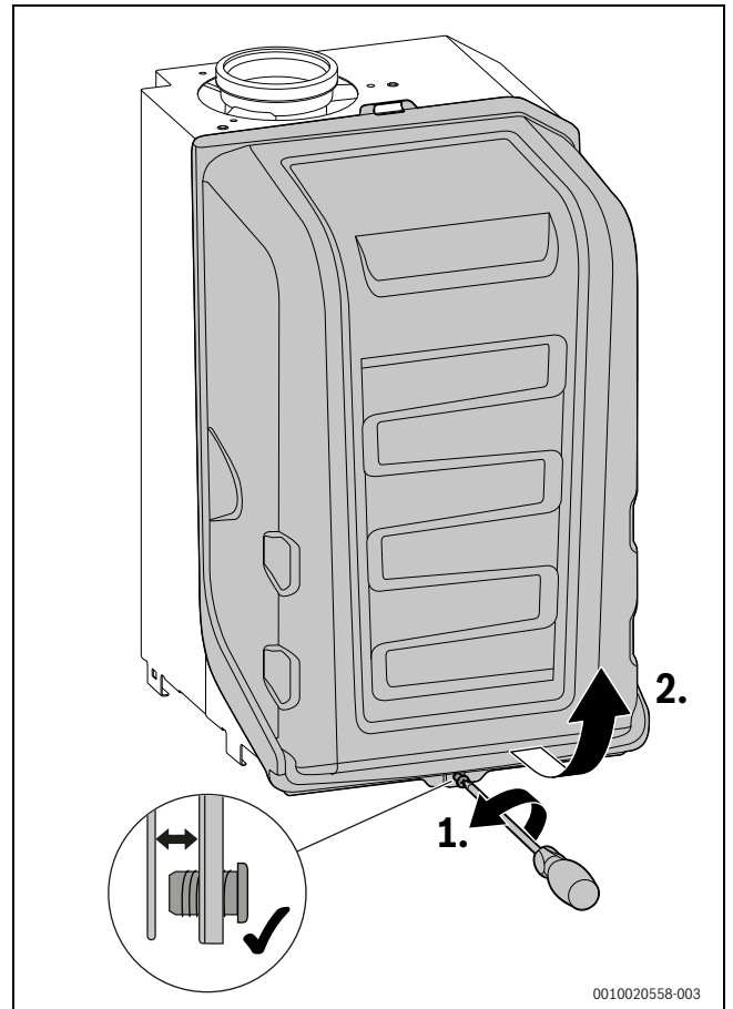
Bild 117 Brennerhaube abnehmen
