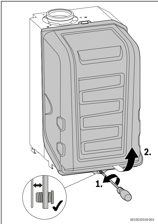
Bild 90 Brennerhaube abnehmen
