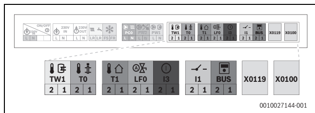
Bild 99 Niederspannungsbereich: Klemmleiste
