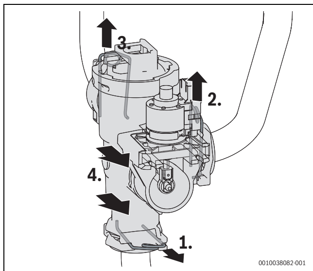
Bild 170 Federn lösen
