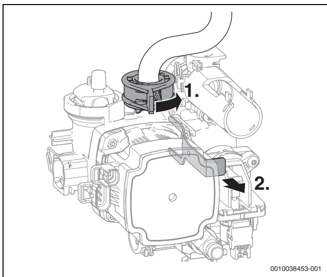
Bild 150 Heizpumpe entriegeln
