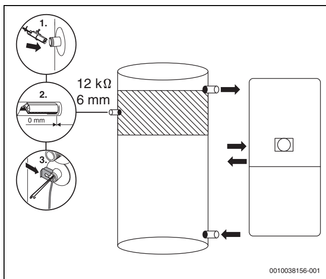
Bild 85 Pufferspeicher-Temperaturfühler einsetzen
