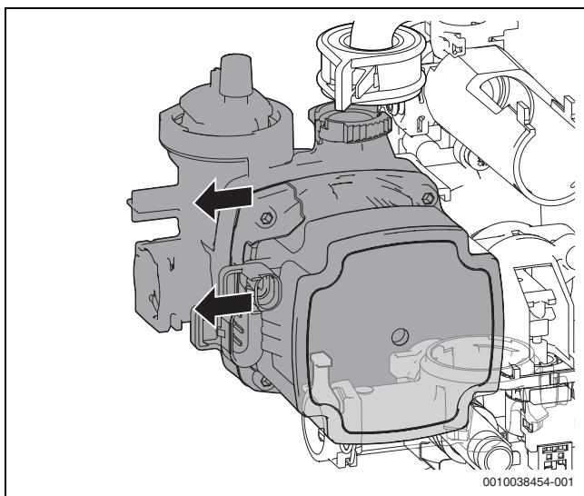
Bild 151 Heizpumpe aus dem Gerät nehmen
