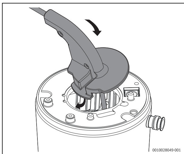
Bild 140 Bürste in den Wärmeblock einsetzen
