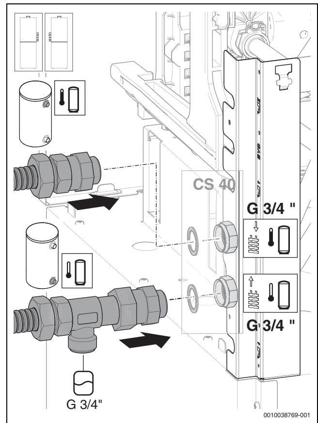
Bild 53 Ausdehnungsgefäß anschließen
