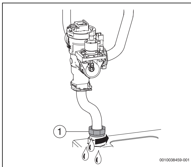
Bild 169 Wasser aus dem Wärmetauscher ablassen
