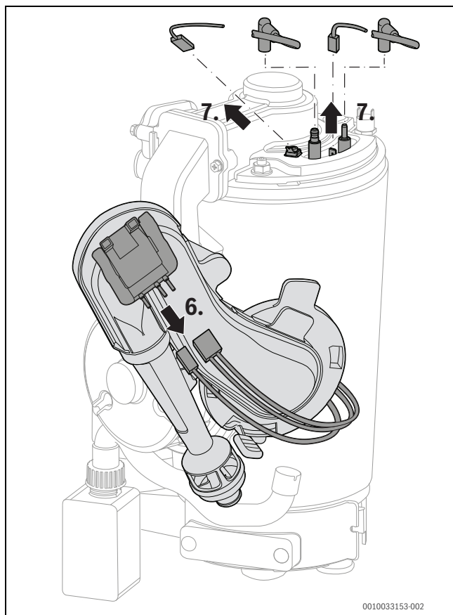
Bild 133 Kabel abziehen
