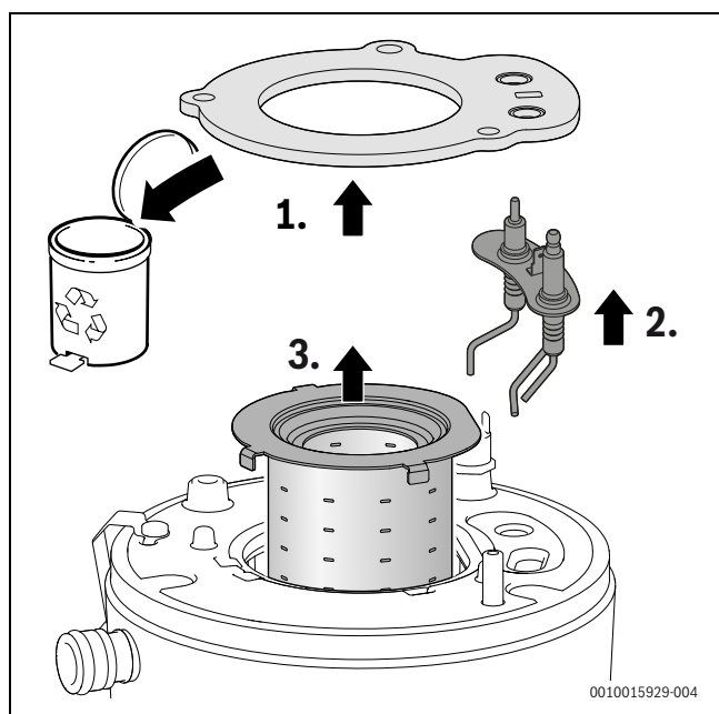
Bild 137 Brenner herausnehmen
