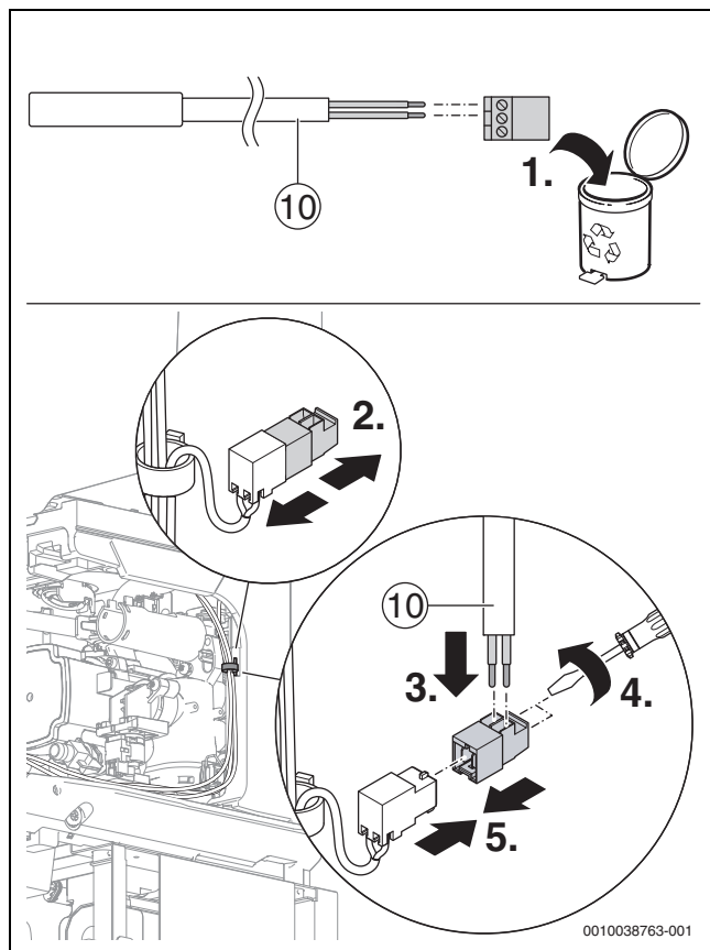
Bild 101 Pufferspeicher-Temperaturfühler anschließen
