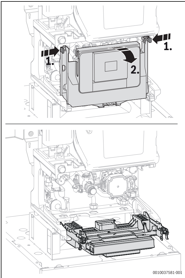
Bild 128 Steuergerät herunterklappen
