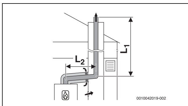
Bild 40 Starre Abgasführung im Schacht nach B 53p /B 53s mit raumluftabhängiger Luftzufuhr über die konzentrische Luft-Abgas-Führung im Aufstellraum
