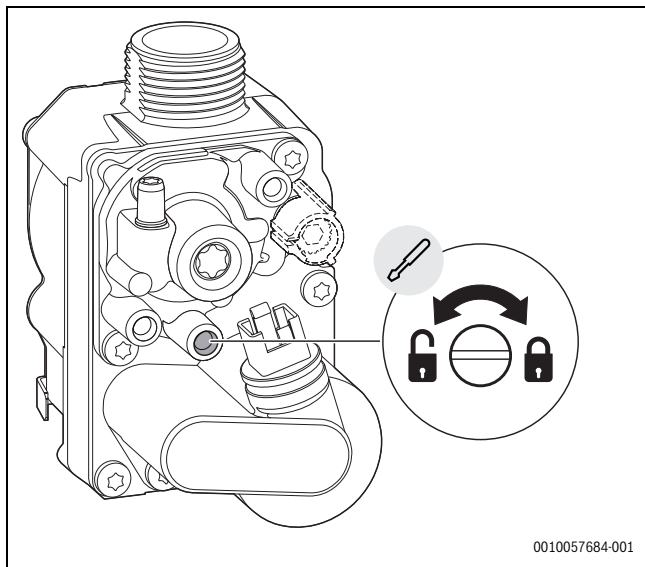
Bild 118 Gas-Anschlussdruck messen
