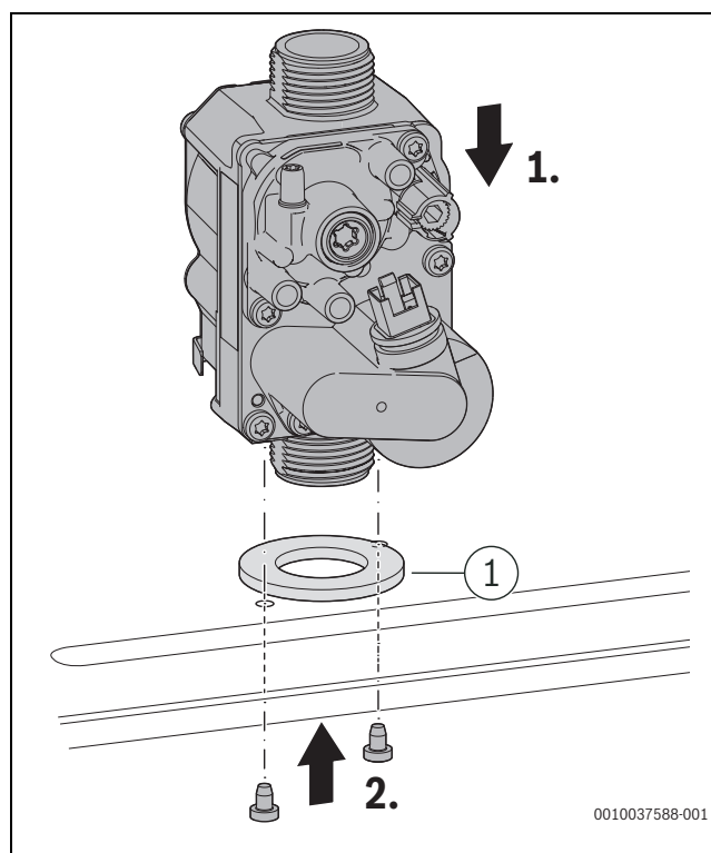
Bild 156 Gasarmatur einbauen
