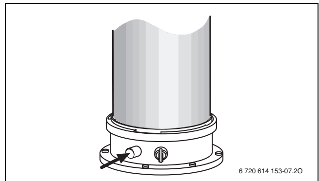
Bild 119 Stopfen abnehmen
