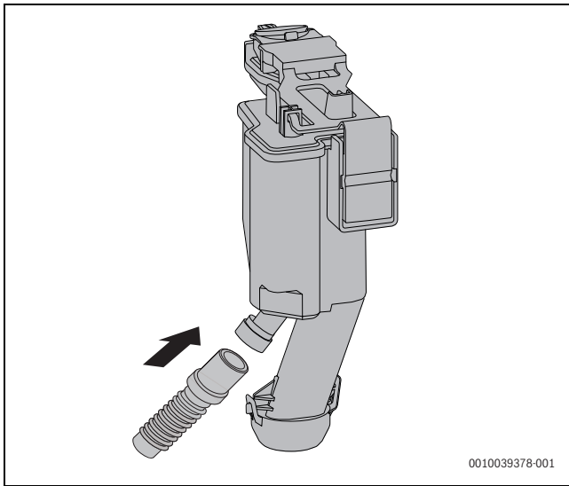
Bild 81 Schlauch am Kondensatsiphon anschließen
