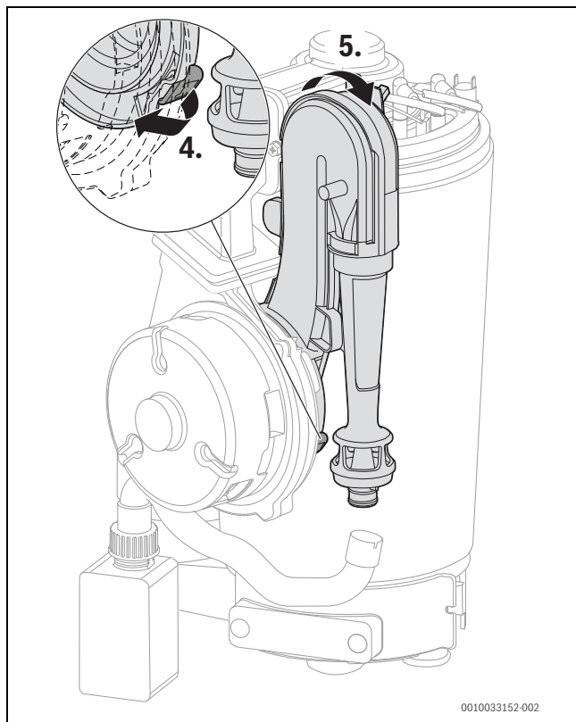
Bild 132 Venturirohr abnehmen
