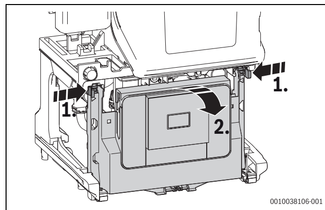
Bild 70 Steuergerät herunterklappen
