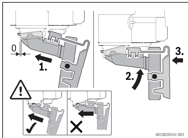
Bild 164 Kondensatsiphon einbauen
