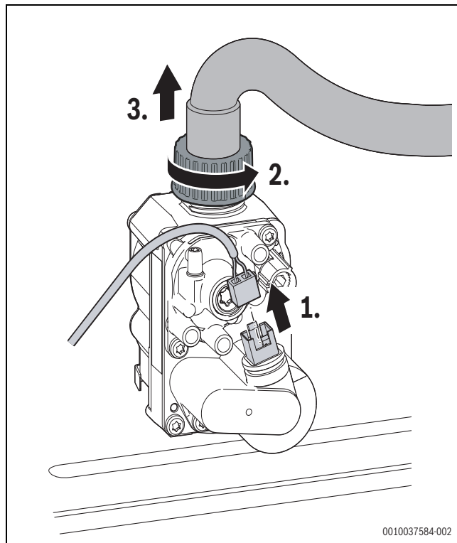
Bild 152 Stecker an der Gasarmatur abziehen und Überwurfmutter mit Gasschlauch abnehmen
