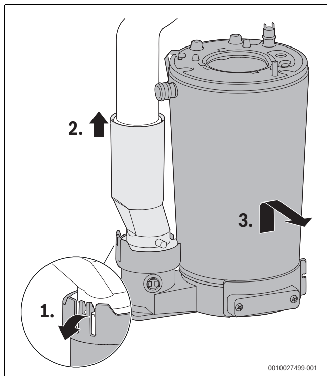
Bild 147 Wärmeblock ausbauen
