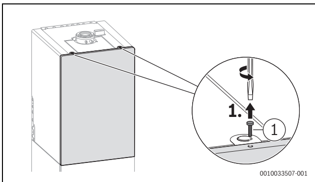
Bild 125 Sicherungsschraube lösen
