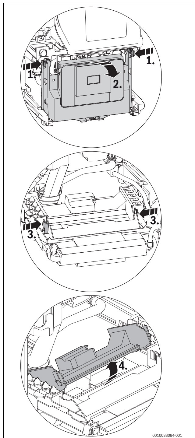
Bild 94 Abdeckung öffnen
