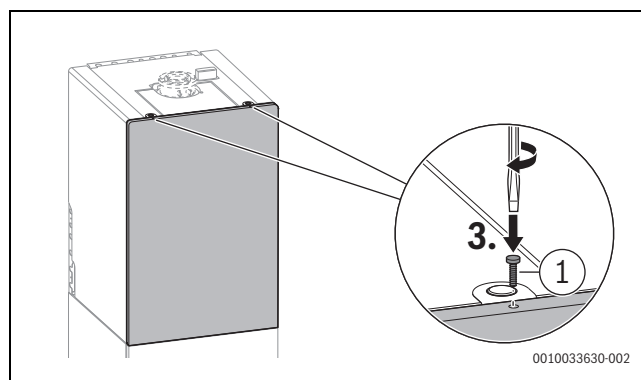
Bild 107 Vorderteil der Geräteverkleidung mit Schraube aus Lieferumfang sichern
