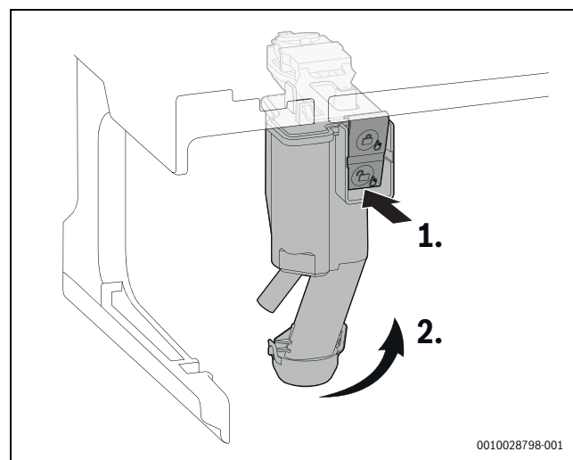
Bild 71 Kondensatsiphon herausnehmen
