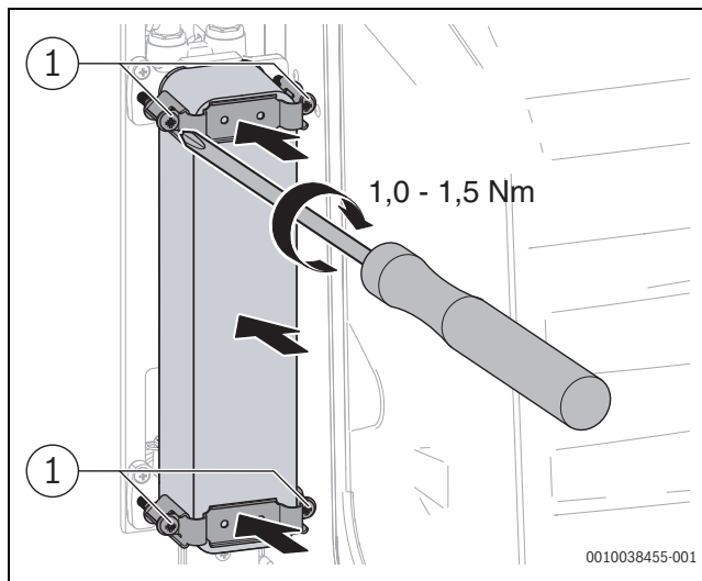
Bild 168 Plattenwärmetauscher einbauen
