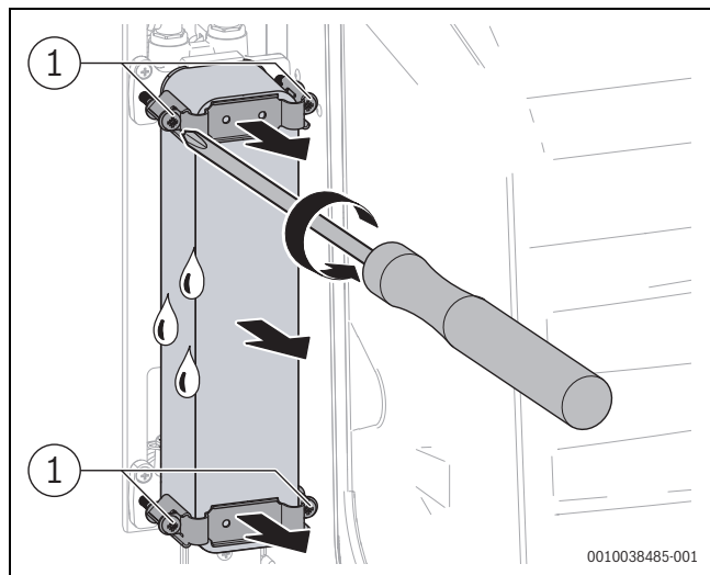
Bild 166 Plattenwärmetauscher ausbauen
