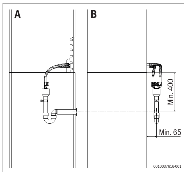
Bild 22 A: Ansicht von der rechten Seite (Maße in mm) B: Ansicht von vorn (Maße in mm)
