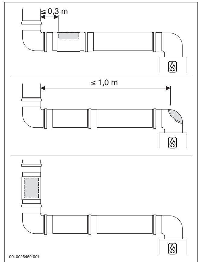
Bild 25 Anordnung der unteren Prüföffnung
