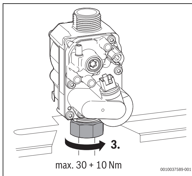
Bild 157 Anzugsdrehmoment beachten
