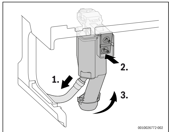
Bild 161 Kondensatsiphon ausbauen
