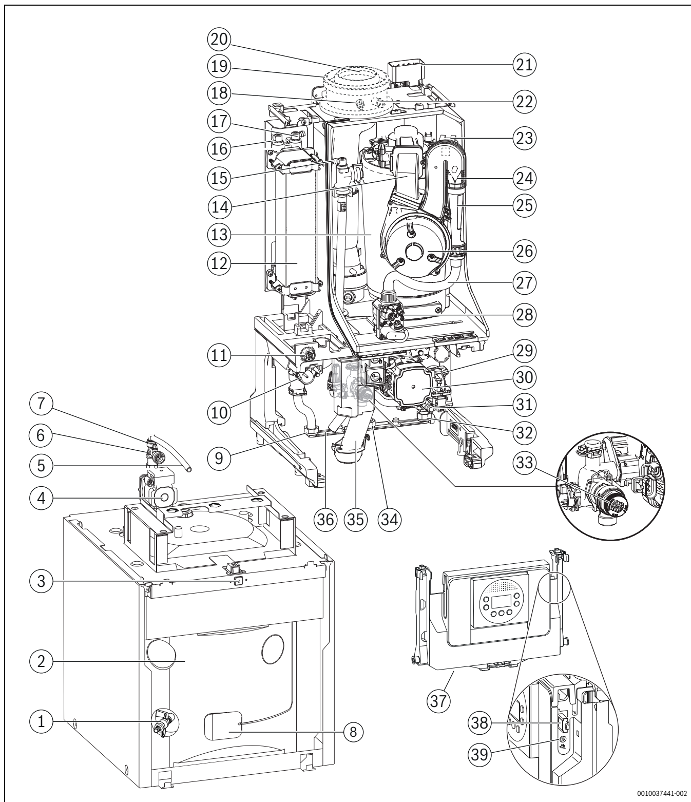
Bild 5 Produktübersicht
