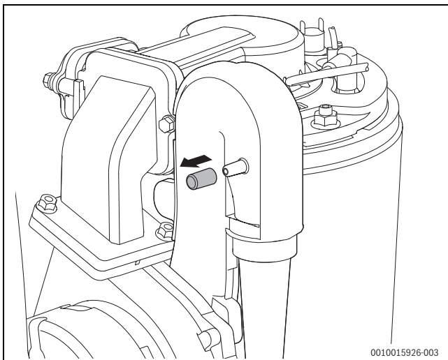
Bild 129 Messstutzen an der Mischeinrichtung
