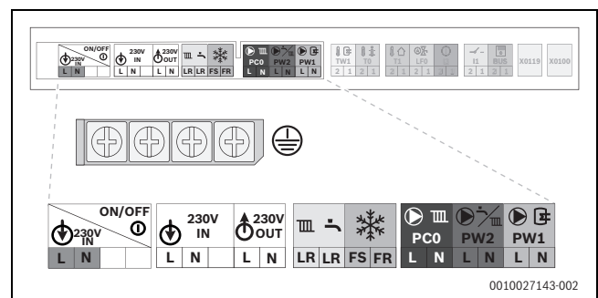
Bild 98 Netzspannungsbereich: Klemmleiste
