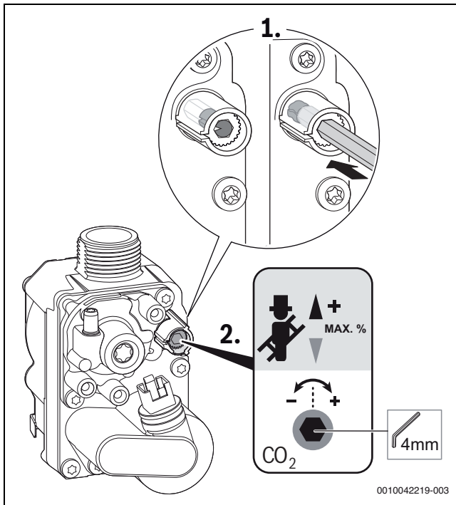
Bild 120 \text{CO}_2/\text{O}_2 -Gehalt bei maximaler Nennwärmeleistung einstellen
