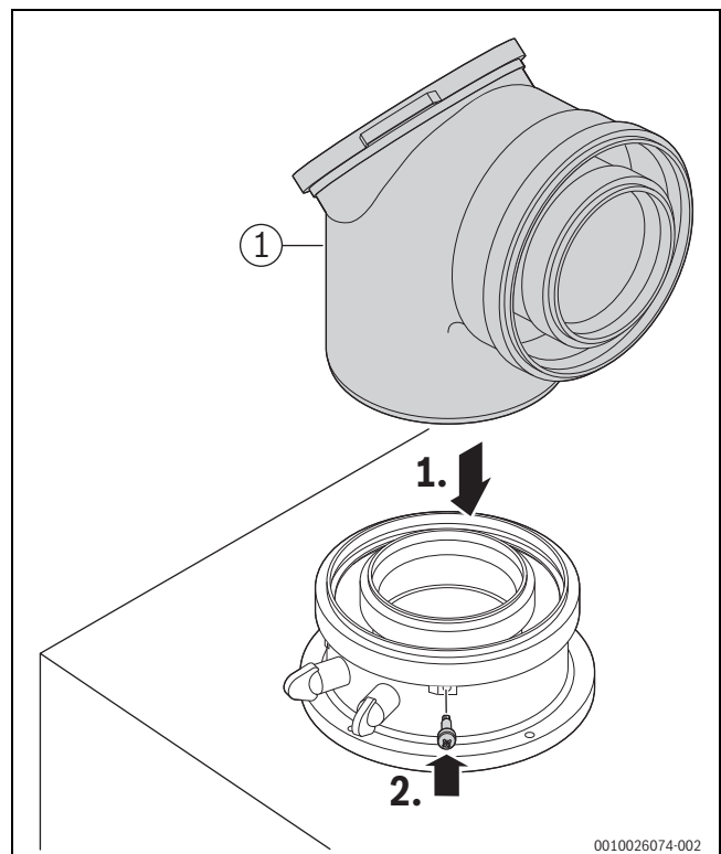
Bild 84 Abgaszubehör einsetzen und mit Schraube sichern
