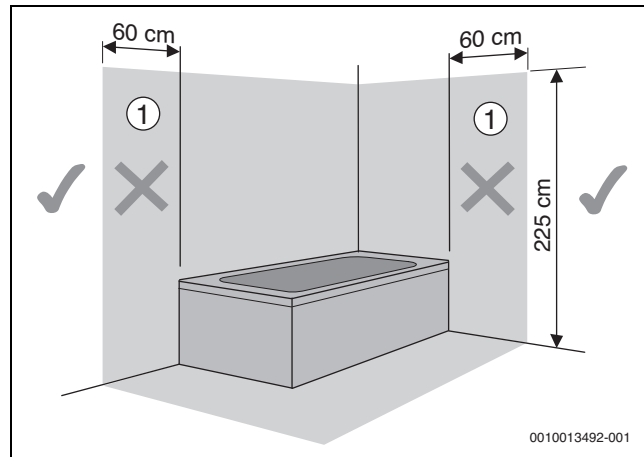
Bild 50 Schutzbereiche
