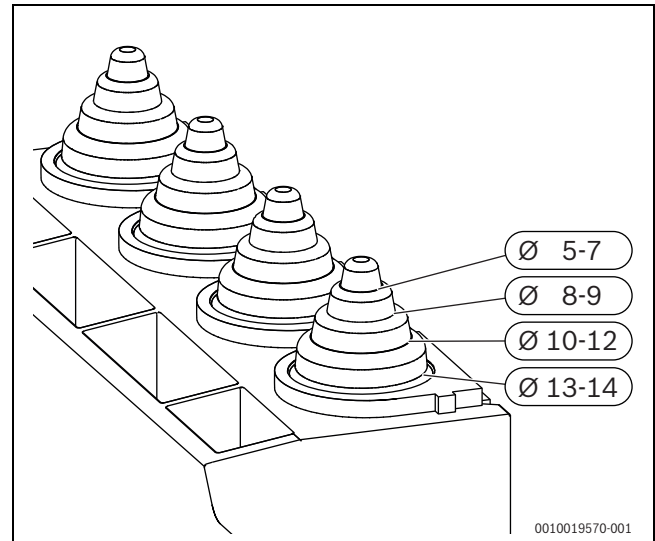
Bild 97 Zugentlastung an Kabeldurchmesser anpassen
