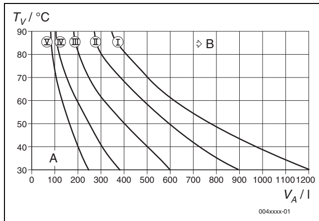
Bild 52 Größe des Ausdehnungsgefäßes für Pufferspeicher mit maximal 400 l Inhalt bestimmen
