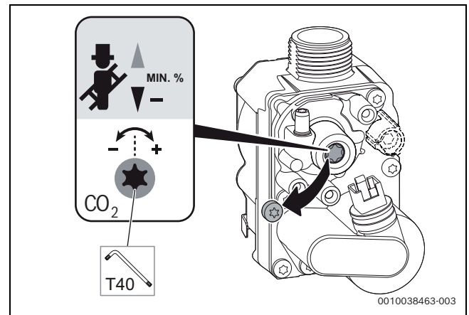
Bild 121 \text{CO}_2/\text{O}_2 -Gehalt bei minimaler Nennwärmeleistung einstellen
