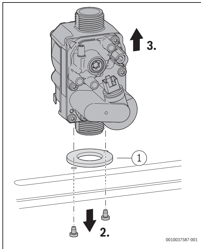
Bild 155 Gasarmatur ausbauen
