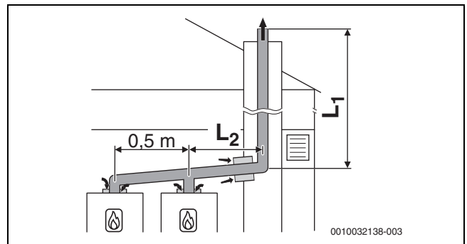
Bild 48 Kaskade mit 2 Geräten:
