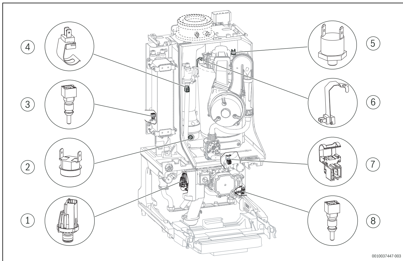
Bild 6 Fühler und Sensoren im Gerät
