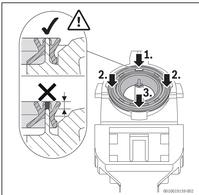
Bild 163 Dichtung andrücken
