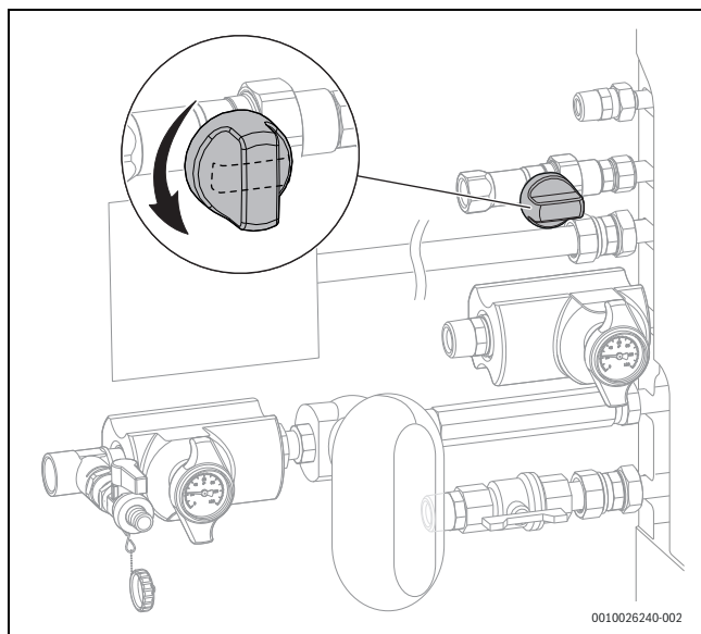
Bild 5 Gashahn öffnen
