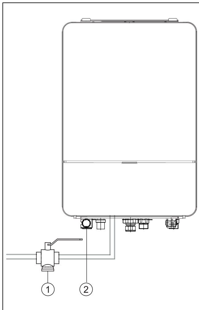
Bild 7 Inneneinheit AWE
