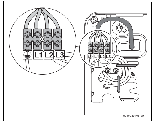
Rys. 43 Podłączenie od góry
