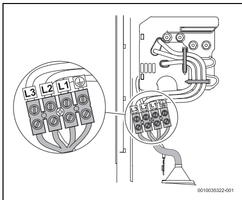
Fig. 44 Raccord inférieur
