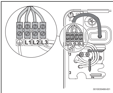
Fig. 43 Raccord supérieur
