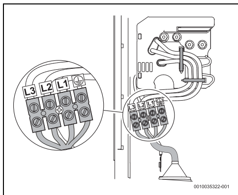
Bild 45 Anschluss unten
