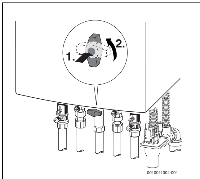
Bild 6 Gashahn öffnen
