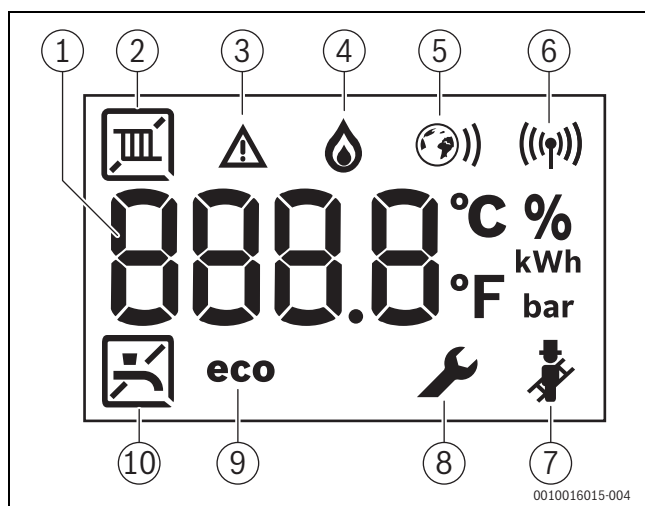
Bild 3 Displayanzeigen
