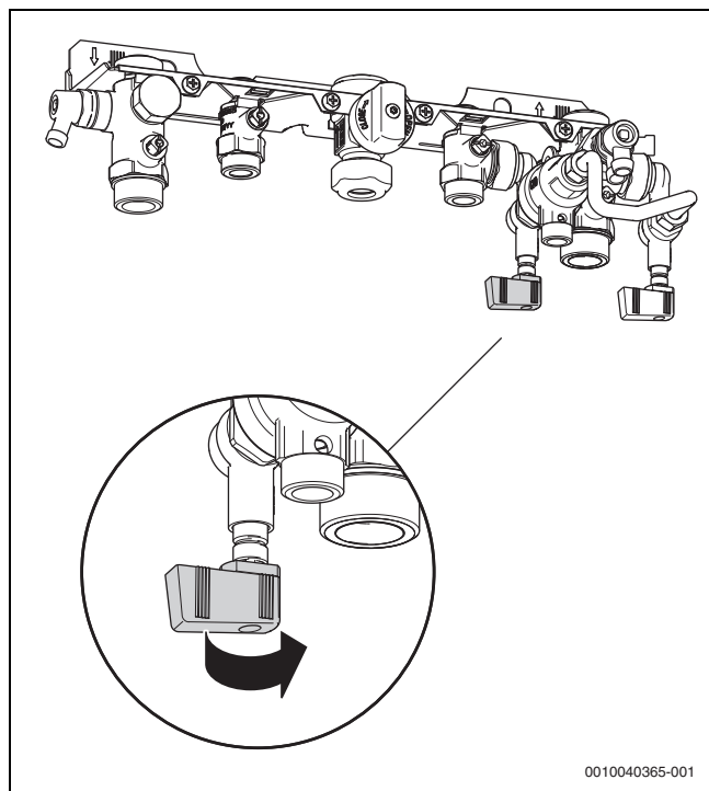
Bild 7 Fülleinrichtung öffnen
