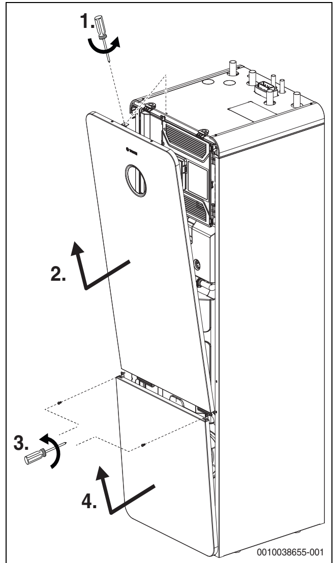
Bild 16 Front abnehmen
