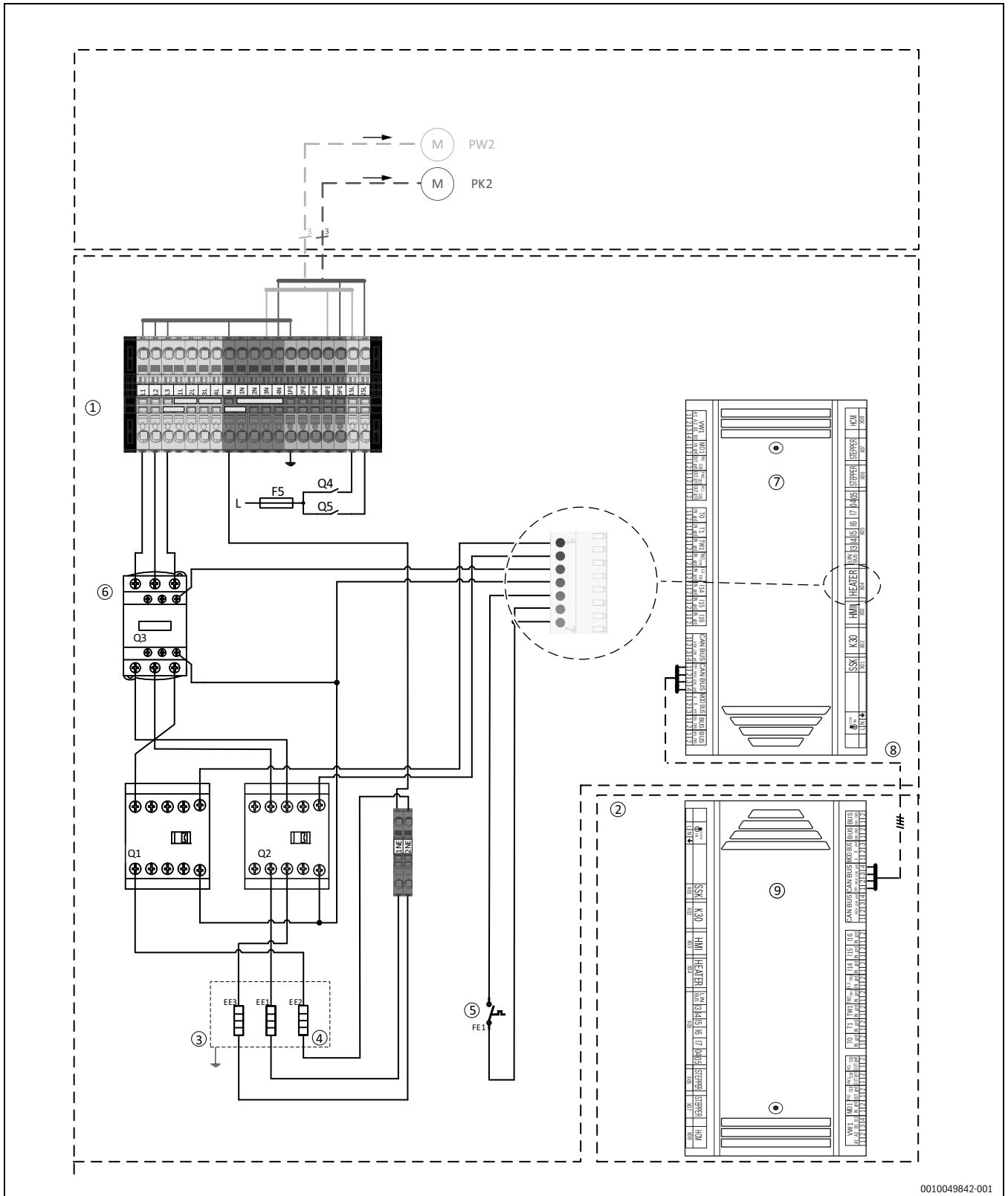
Bild 50 Spannungsversorgung Inneneinheit
