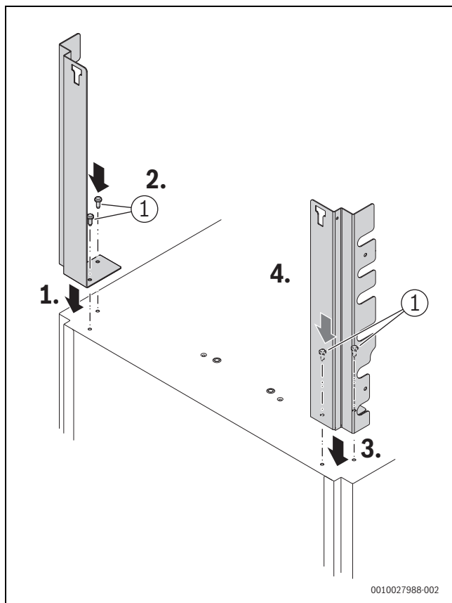
Bild 56 Basismodul (Zubehör CS 35) montieren – Schritt 1
