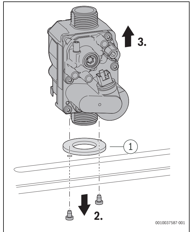
Bild 151 Gasarmatur ausbauen
