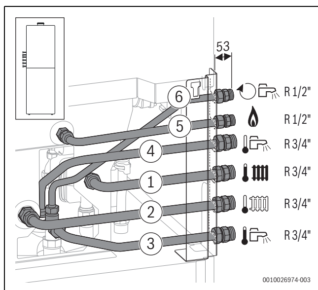
Bild 61 Zubehör CS 10 auf der linken Seite montiert
