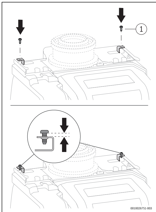
Bild 64 Schrauben für die Oberseite der Geräteverkleidung locker eindrehen
