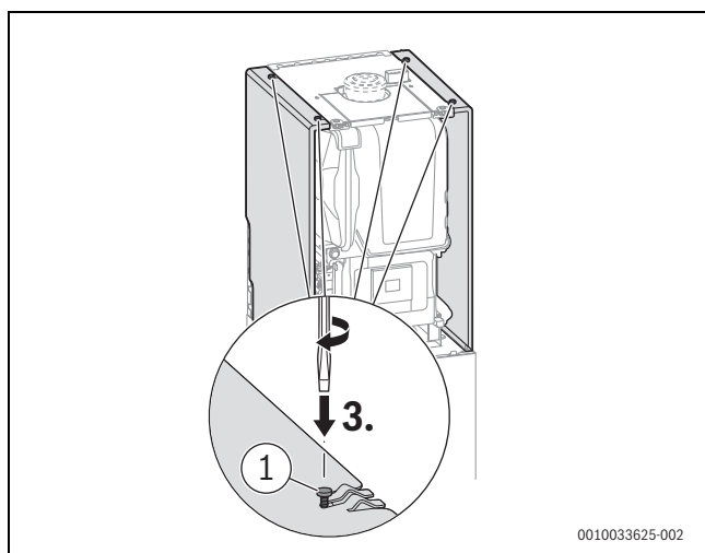
Bild 101 Seitenteile der Geräteverkleidung befestigen
