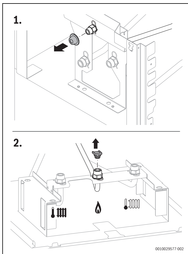
Bild 60 Schutzkappe und Stopfen vom Gasrohr abnehmen
