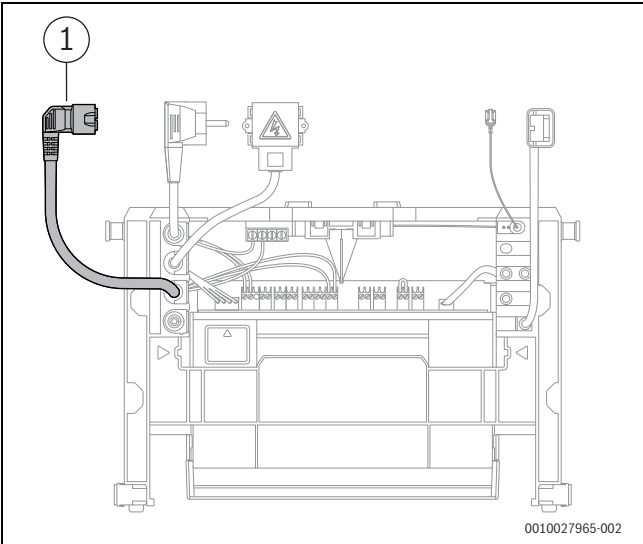
Bild 93 Steckplatz für das Anschlusskabel der Schichtladepumpe
