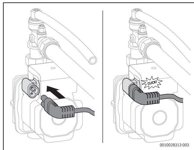
Bild 97 Schichtladepumpe elektrisch anschließen
