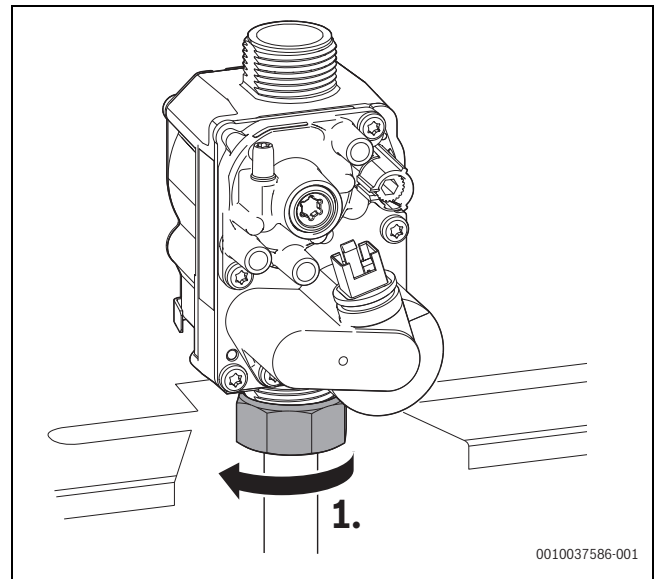
Bild 150 Überwurfmutter lösen
