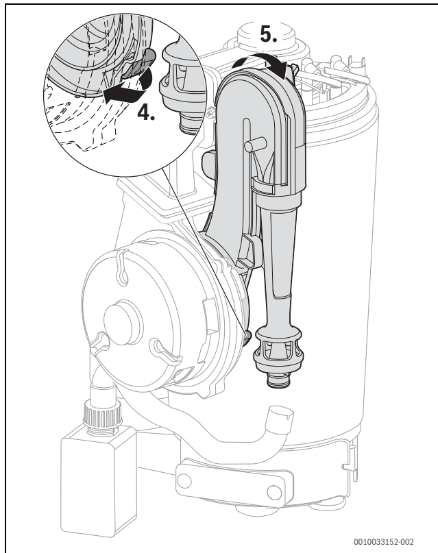
Bild 128 Venturirohr abnehmen
