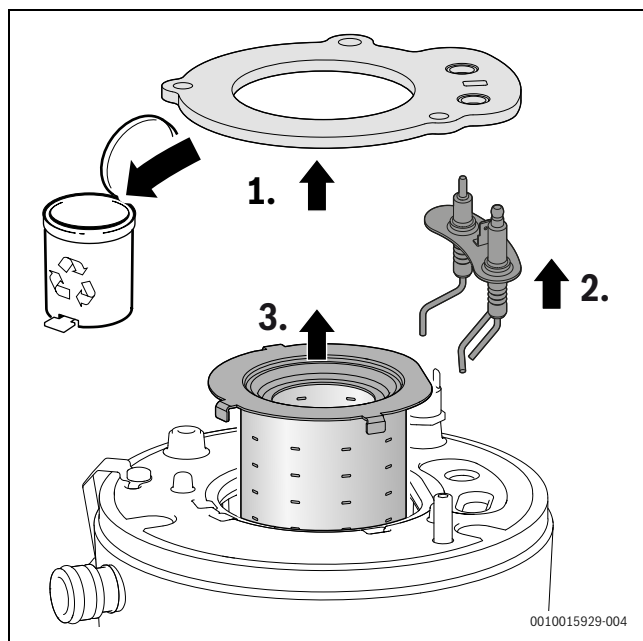
Bild 133 Brenner herausnehmen
