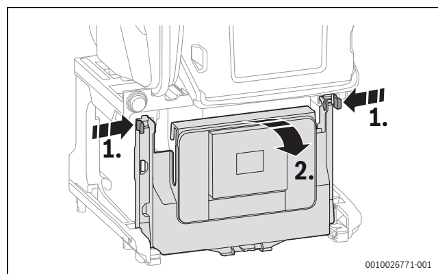
Bild 68 Steuergerät herunterklappen
