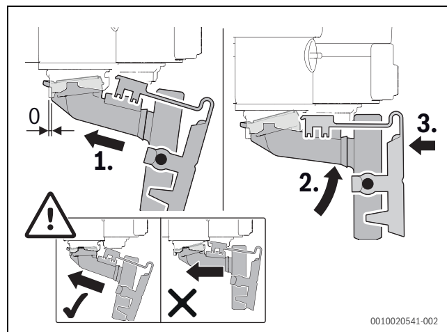
Bild 73 Kondensatsiphon wieder einsetzen und auf festen Sitz prüfen
