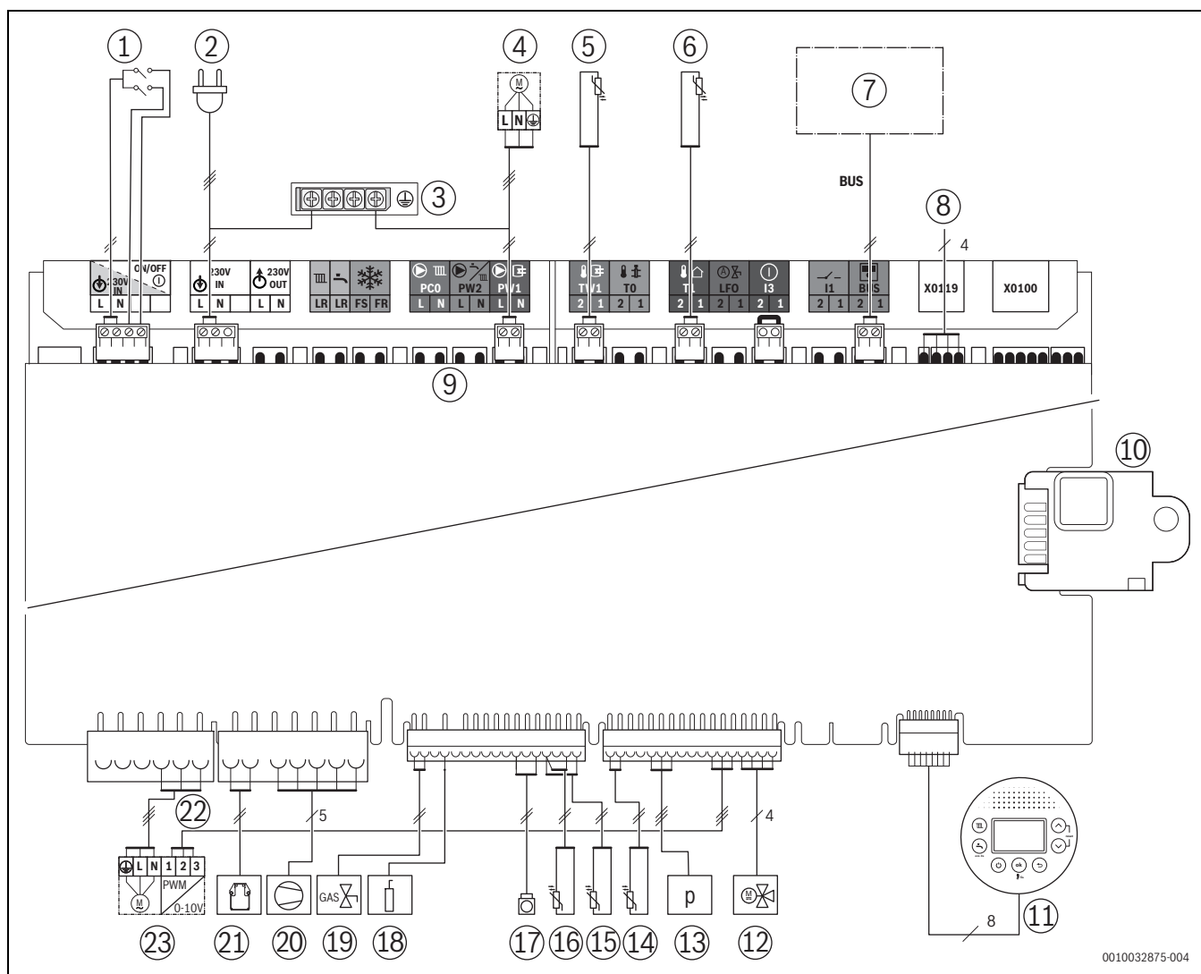
Bild 165 Elektrische Verdrahtung
