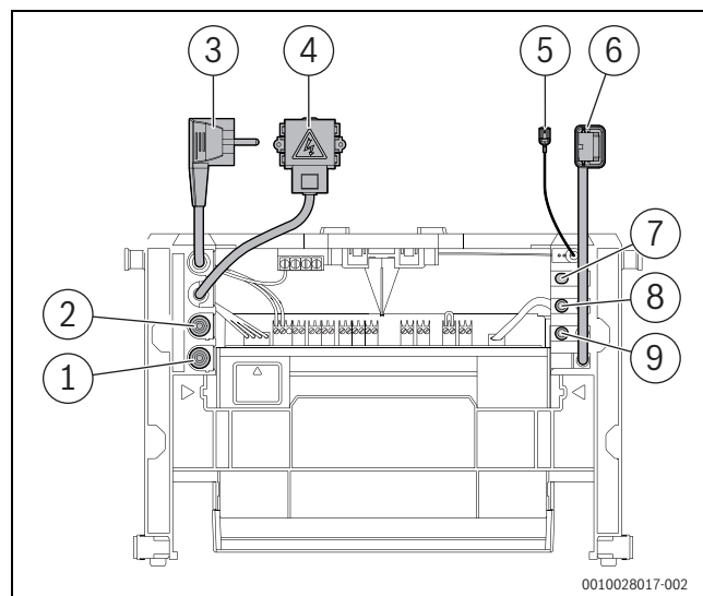
Bild 92 Lieferzustand des Steuergeräts mit angeschlossenen Komponenten
