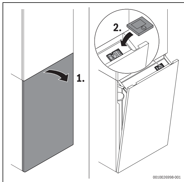
Bild 84 Bedieneinheit CW 400 einsetzen
