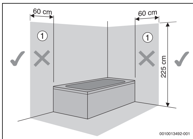
Bild 47 Schutzbereiche
