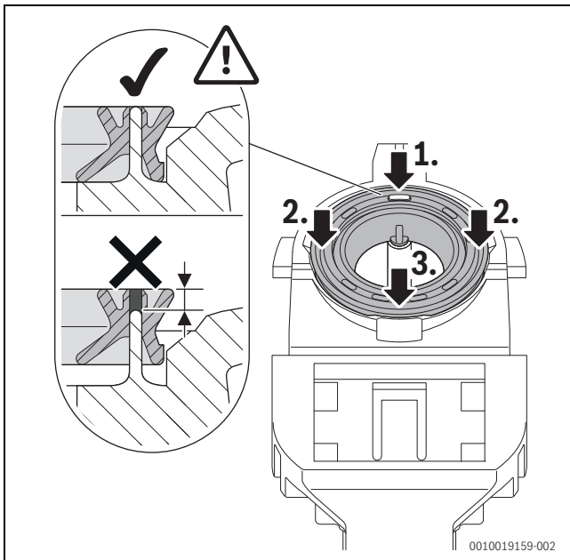
Bild 159 Dichtung andrücken
