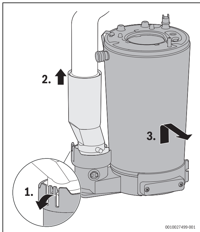
Bild 143 Wärmeblock ausbauen
