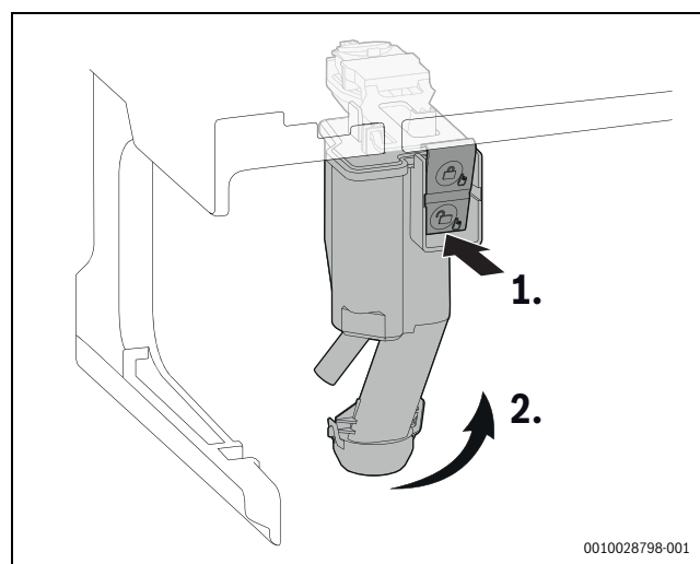
Bild 69 Kondensatsiphon herausnehmen
