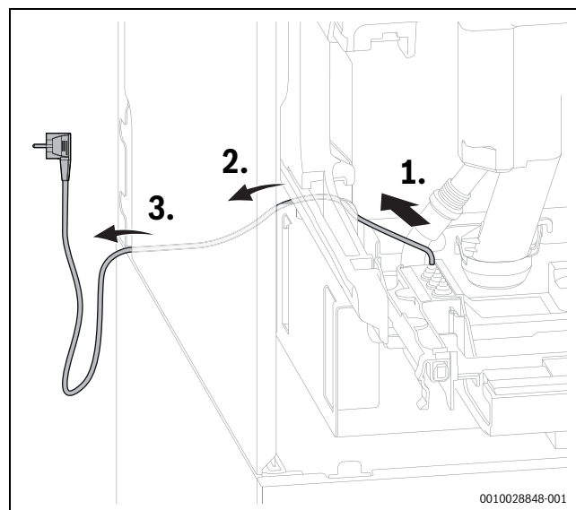
Bild 98 Kabelführung des Netzkabels
