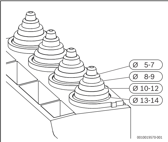
Bild 94 Zugentlastung an Kabeldurchmesser anpassen
