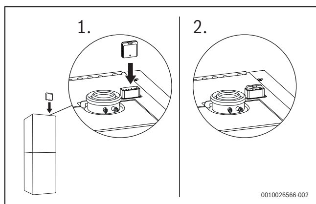
Bild 83 Control Key in den Key-Halter einstecken
