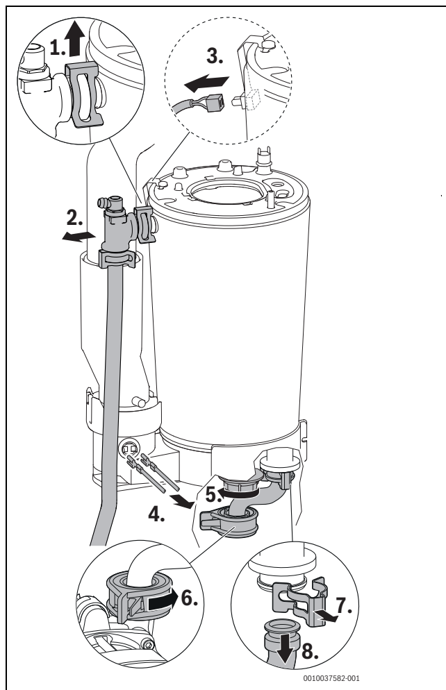
Bild 142 Vorlaufrohr lösen, Kabel abziehen und Rücklaufrohr lösen
