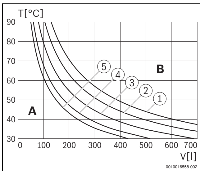
Bild 49 Kennlinien für Ausdehnungsgefäß (12 l)
