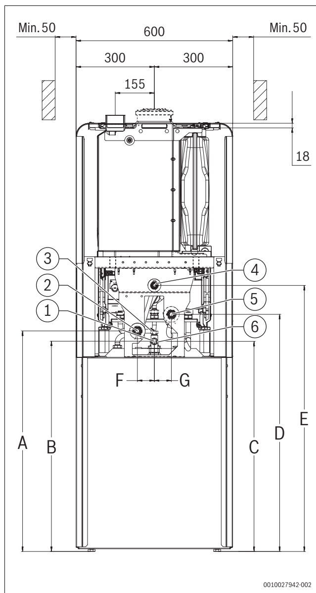
Bild 9 Ansicht von der Rückseite (Maße in mm)
