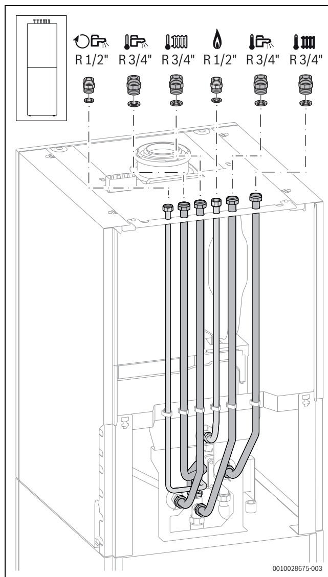
Bild 63 Zubehör CS 33 montiert
