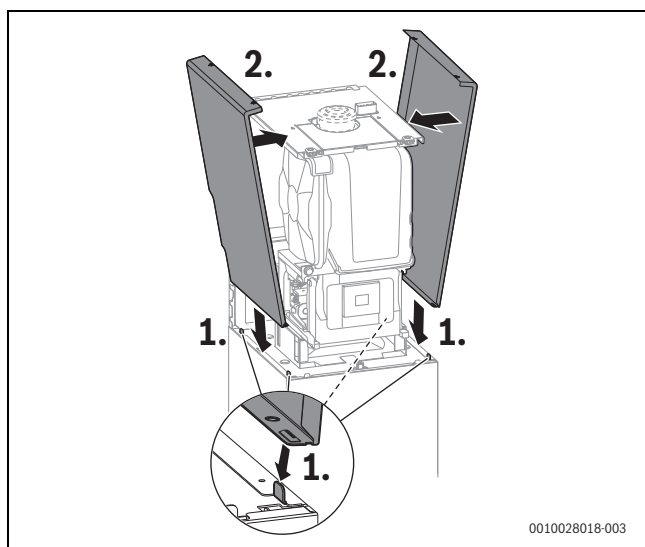
Bild 100 Seitenteile der Geräteverkleidung einsetzen
