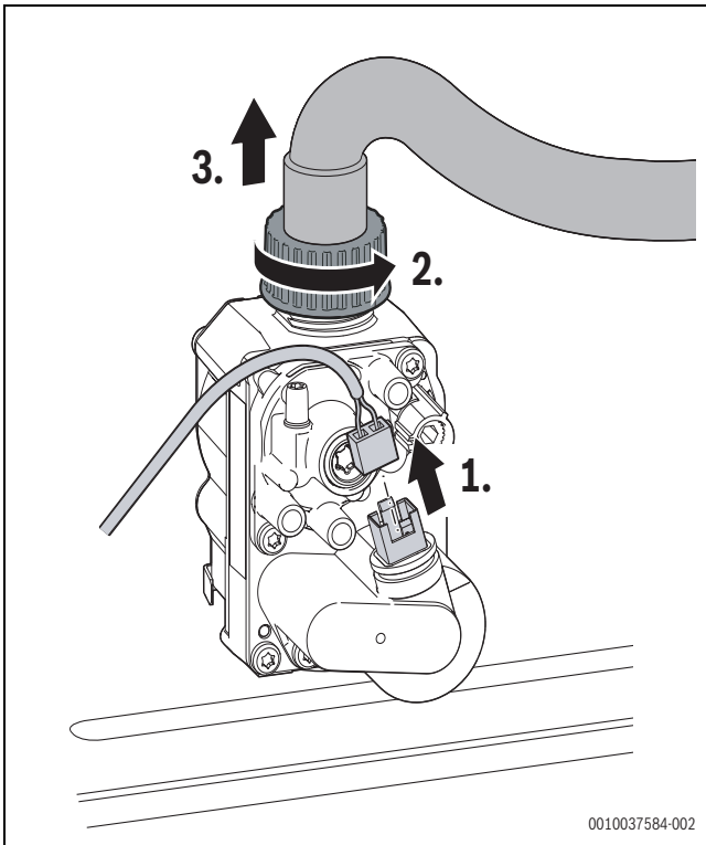
Bild 148 Stecker an der Gasarmatur abziehen und Überwurfmutter mit Gasschlauch abnehmen
