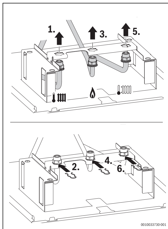
Bild 59 Heizungsanlauf, Gasrohr und Heizungsanlauf vorn einsetzen (Zubehör CS 35)
