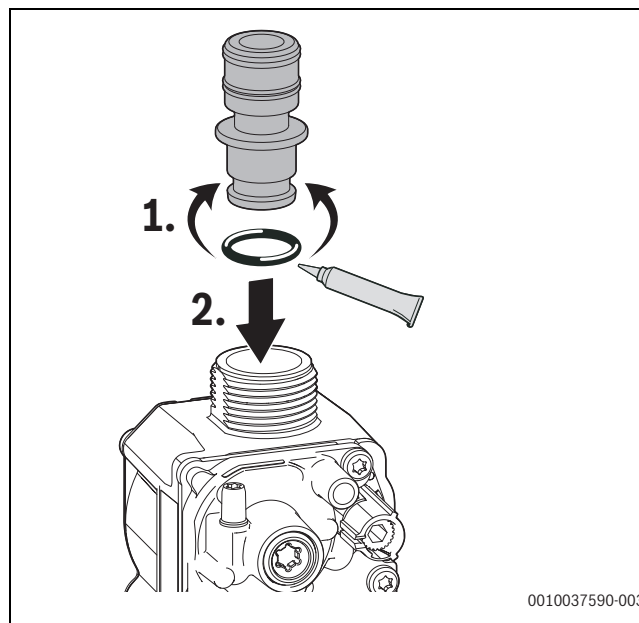
Bild 154 Gasdüse einsetzen
