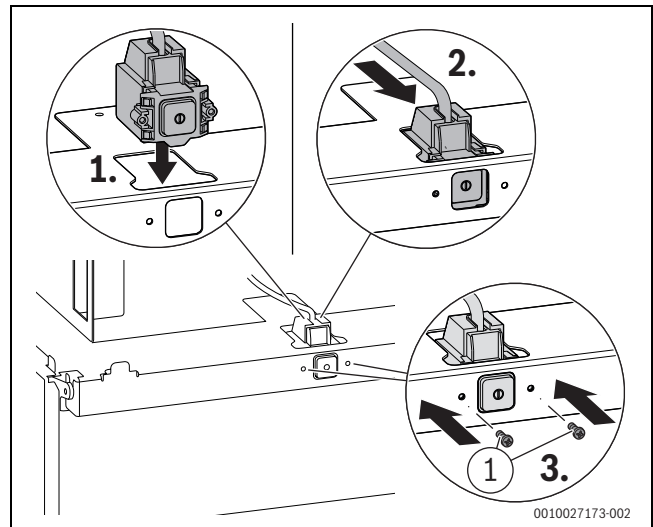
Bild 89 Schalter Ein/Aus befestigen
