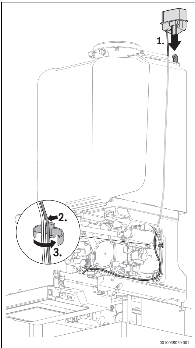
Bild 75 Key-Halter in den Steckplatz einsetzen und Kabel im Kabelhalter befestigen
