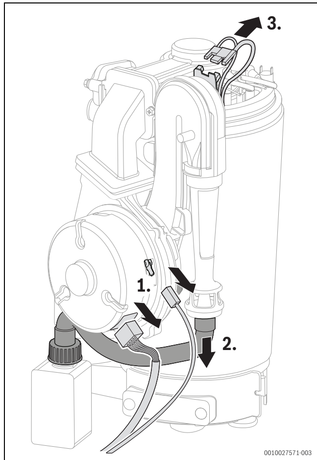
Bild 127 Stecker und Gasschlauch abziehen
