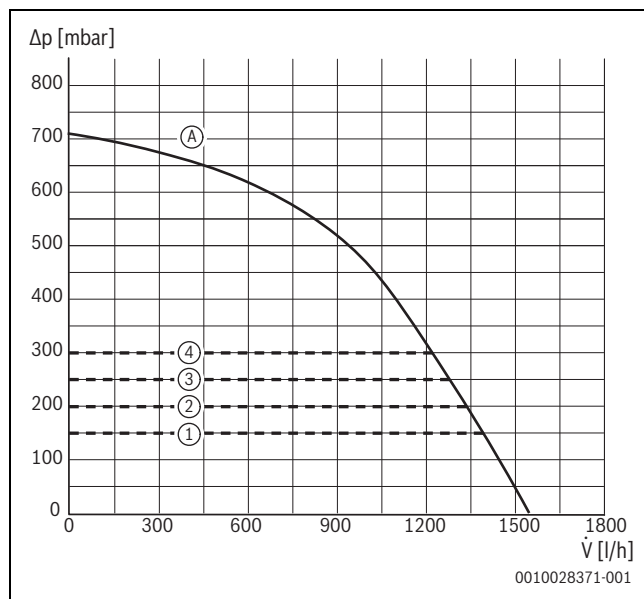
Bild 166 Pumpenkennfelder und Pumpenkennlinie (17/24 kW)
