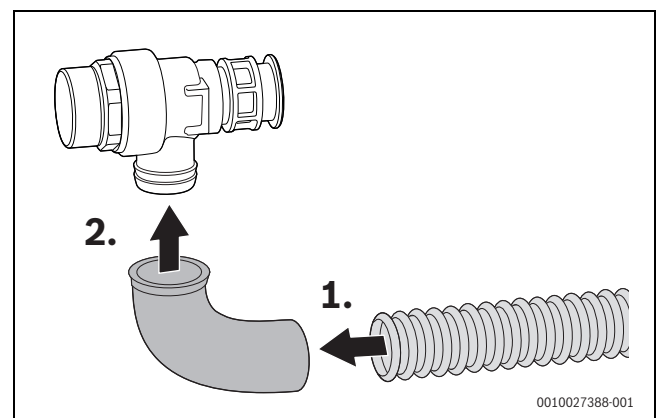
Bild 78 Schlauch am Sicherheitsventil anschließen
