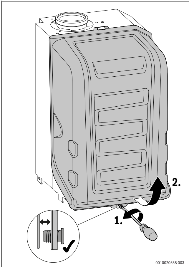
Bild 113 Brennerhaube abnehmen
