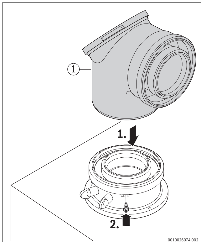
Bild 82 Abgaszubehör einsetzen und mit Schraube sichern
