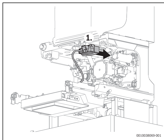
Bild 74 Key-Halter auf die Rückseite des Geräts führen
