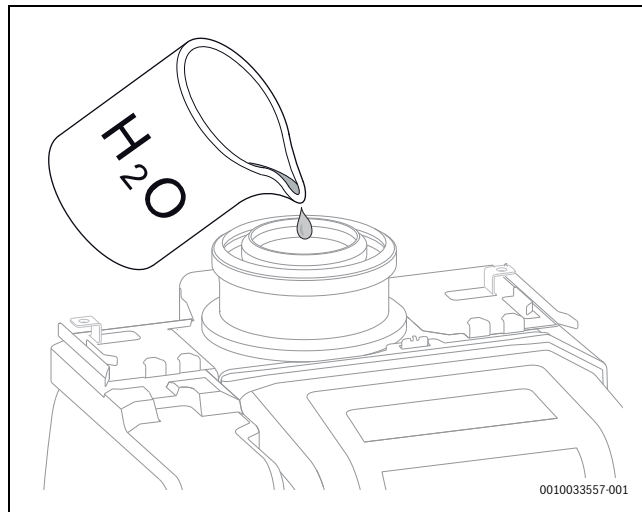
Bild 81 Kondensatsiphon mit Wasser füllen
