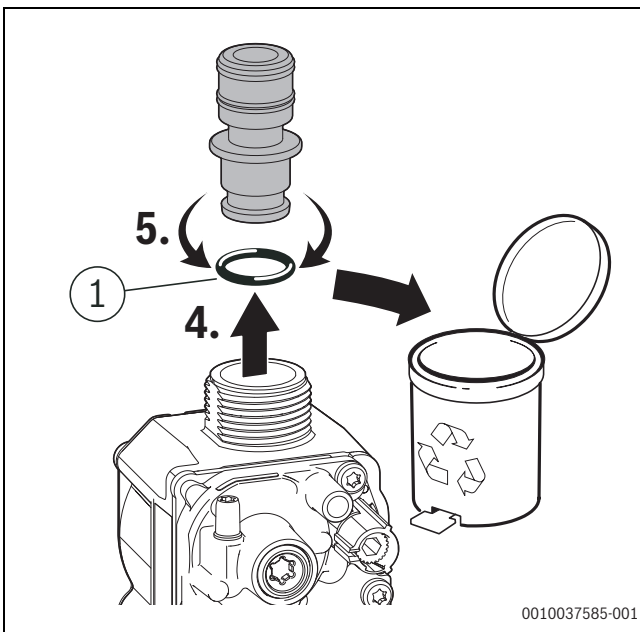
Bild 149 Gasdüse abnehmen
