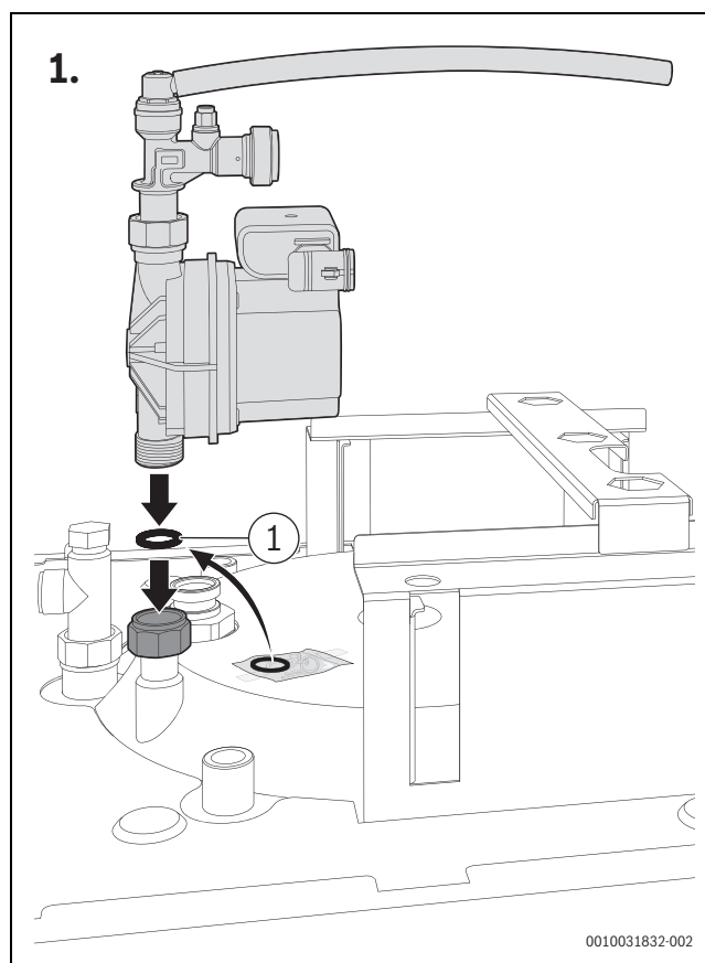
Bild 54 Schichtladepumpe einsetzen
