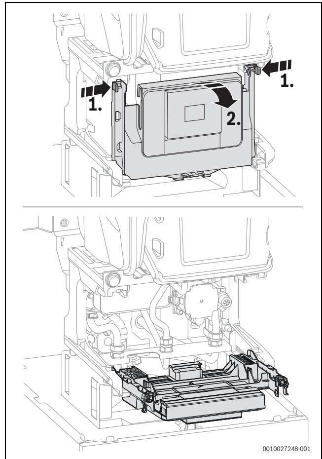
Bild 124 Steuergerät herunterklappen
