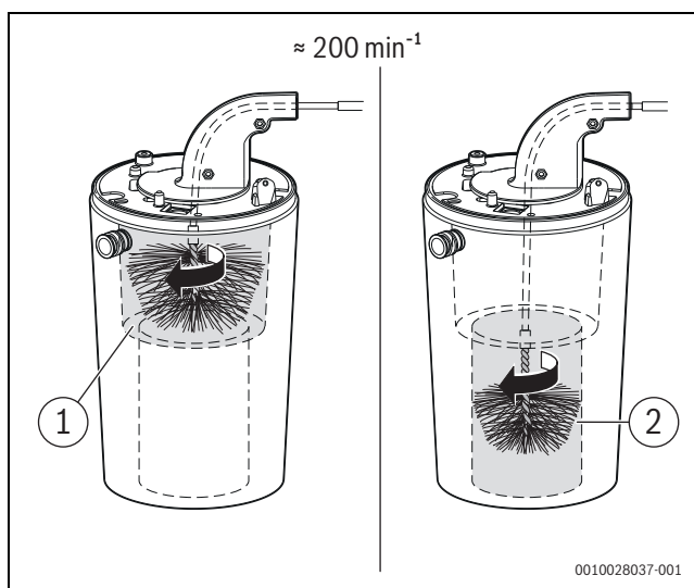
Bild 138 Wärmeblock reinigen (ca. 200 min -1 , nur Rechtslauf)
