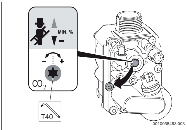
Bild 117 CO 2 /O 2 -Gehalt bei minimaler Nennwärmeleistung einstellen
