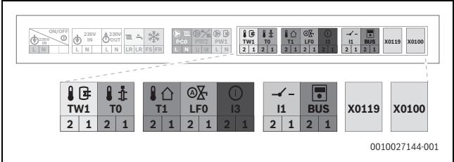
Bild 96 Niederspannungsbereich: Klemmleiste
