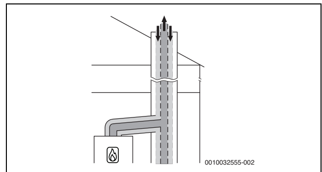
Bild 30 Konzentrische Luft-Abgas-Führung nach C 43x im Aufstellraum
