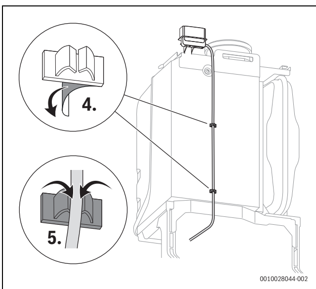
Bild 76 Kabelhalter an der Rückseite des Geräts anbringen und Kabel befestigen
