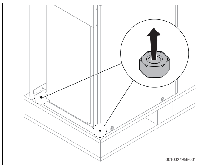
Bild 52 Transportsicherung unten an der Rückseite des Speichers entfernen
