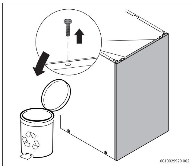
Bild 53 Transportsicherung am Vorderteil der Speicherverkleidung entfernen
