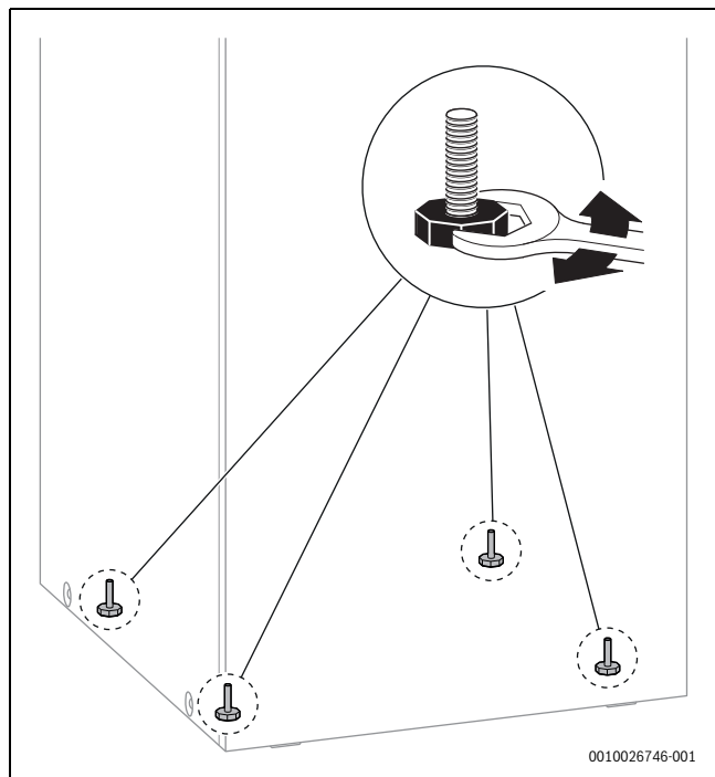
Bild 106 Am endgültigen Aufstellort Unebenheiten des Fußbodens mit den Stellfüßen ausgleichen
