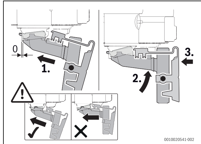
Bild 160 Kondensatsiphon einbauen
