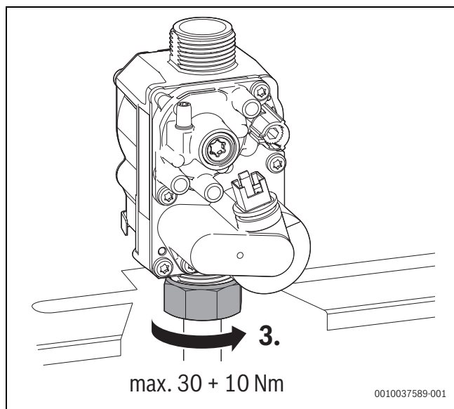
Bild 153 Anzugsdrehmoment beachten
