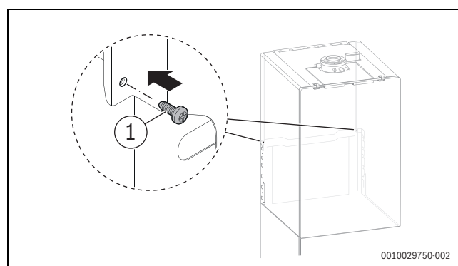
Bild 104 Seitenteile der Geräteverkleidung auf der linken und rechten Seite festschrauben
