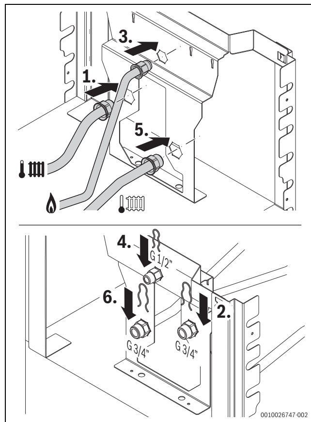
Bild 58 Heizungsanlauf, Gasrohr und Heizungsanlauf hinten einsetzen (Zubehör CS 35)
