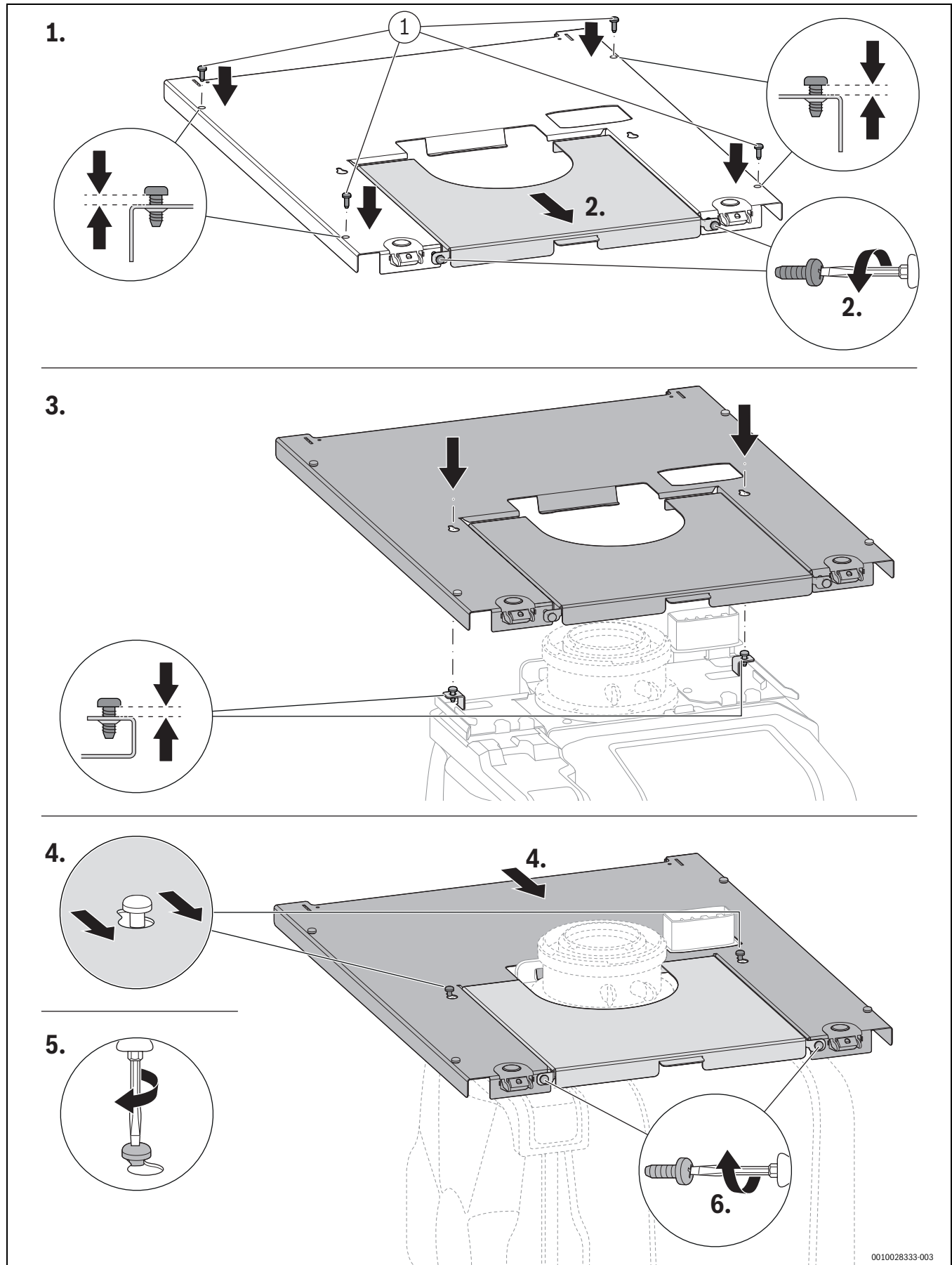
Bild 99 Oberteile der Geräteverkleidung befestigen. Wenn erforderlich können beide Teile der Verkleidung nacheinander eingesetzt werden.
