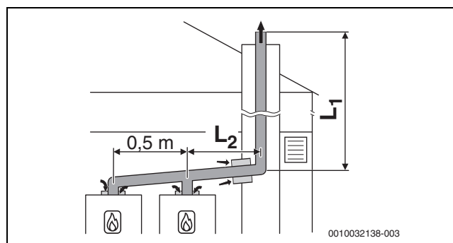
Bild 45 Kaskade mit 2 Geräten:
