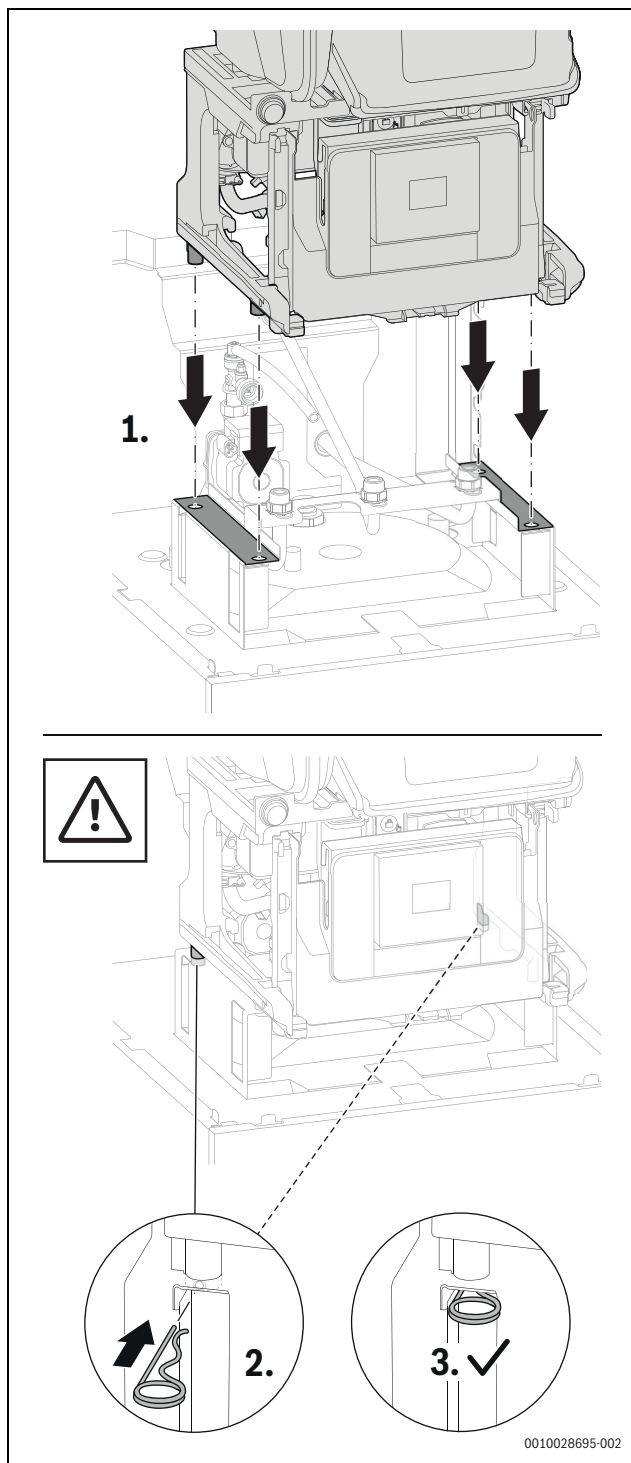
Bild 67 Gerät auf den Speicher aufsetzen und mit 2 Splinten sichern
