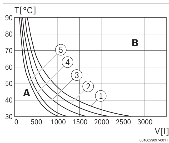
Bild 51 Kennlinien für Ausdehnungsgefäß (29 l)
