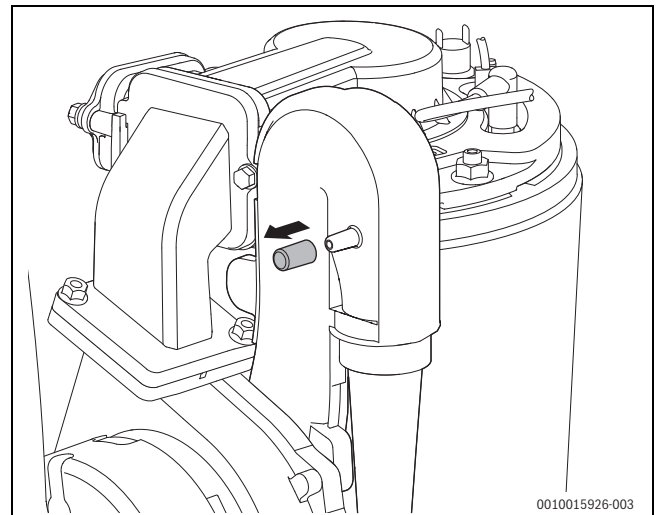
Bild 125 Messstutzen an der Mischeinrichtung
