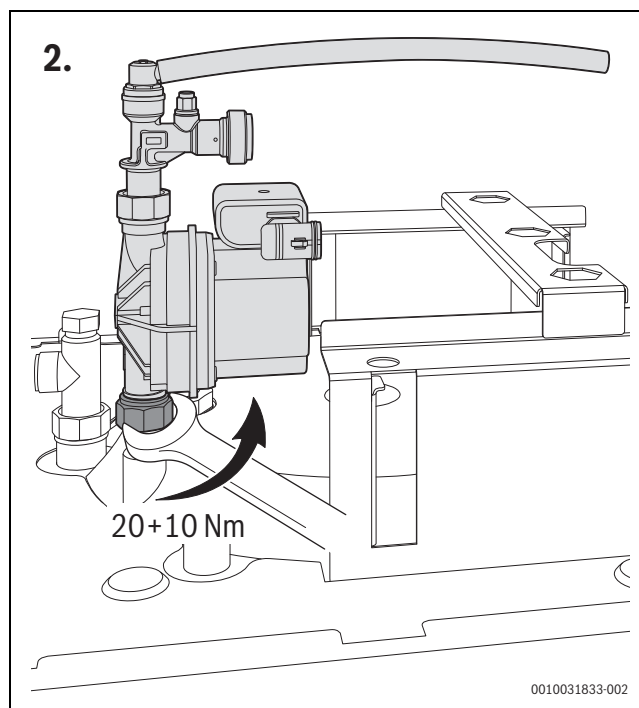
Bild 55 Anzugsdrehmoment beachten
