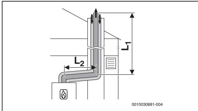
Bild 28 Konzentrische Luft-Abgas-Führung nach C 33x im Schacht
