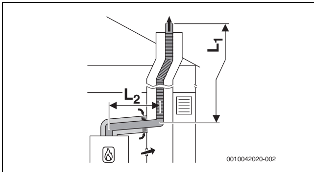
Bild 39 Flexible Abgasführung im Schacht nach B 53p /B 53s mit raumluftabhängiger Luftzufuhr über die konzentrische Luft-Abgas-Führung im Aufstellraum
