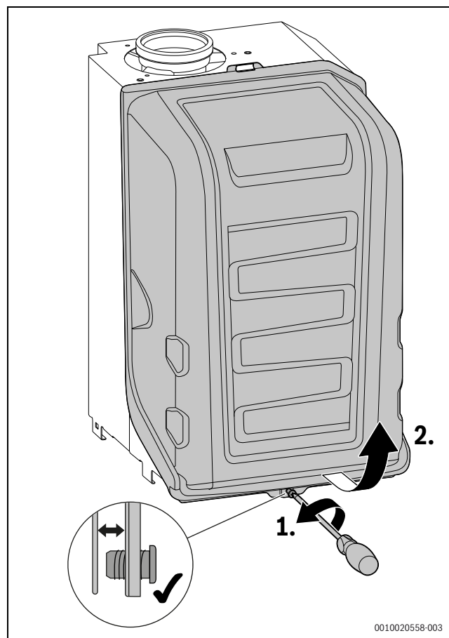
Bild 86 Brennerhaube abnehmen
