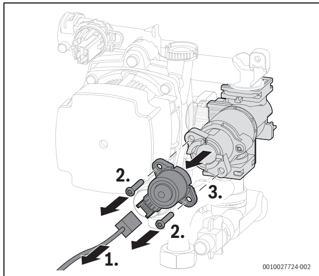
Bild 162 Motor am 3-Wege-Ventil ausbauen
