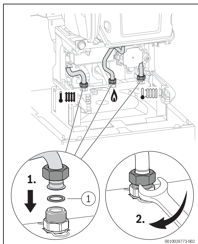
Bild 70 Heizungsvorlauf, Gas, Heizungsrücklauf anschließen
