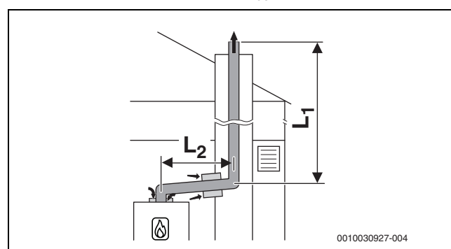
Bild 36 Starre Abgasführung im Schacht nach B 53p mit raumluftabhängiger Luftzufuhr am Gerät und konzentrischem Verbindungsstück zwischen Aufstellraum und Schacht
