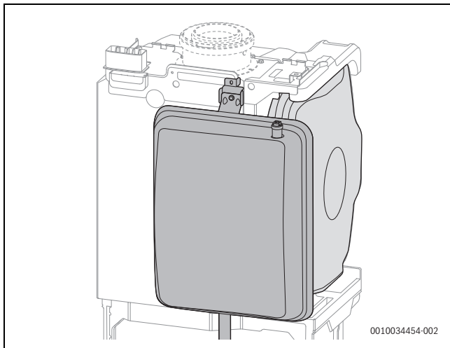
Bild 50 2 Ausdehnungsgefäße im Gerät montiert
