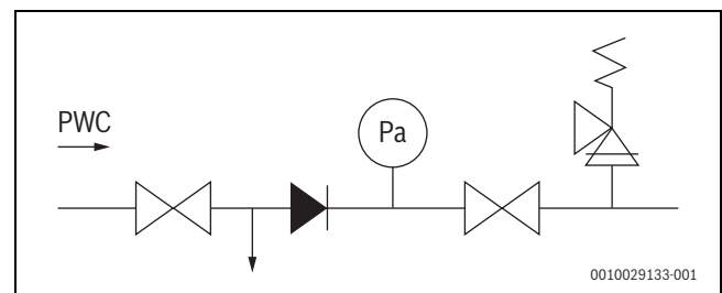
Bild 77 Beispiel: Sicherheitsgruppe für Expansionswasser nach EN 1488
