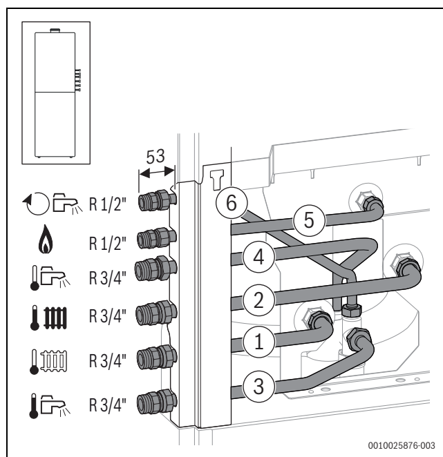
Bild 62 Zubehör CS 10 auf der rechten Seite montiert
