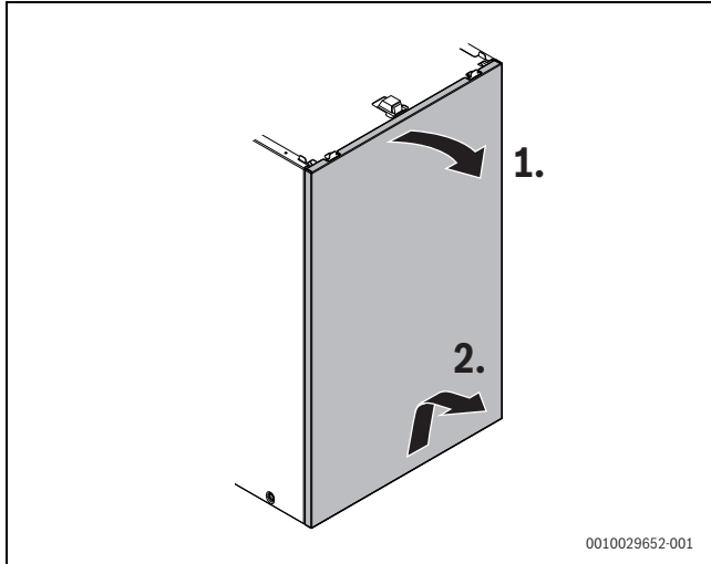
Bild 163 Vorderteil der Speicherverkleidung abnehmen und sicher abstellen
