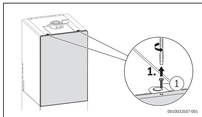
Bild 121 Sicherungsschraube lösen
