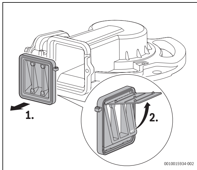
Bild 132 Rückströmsicherung in der Mischeinrichtung
