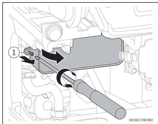
Bild 161 Plattenwärmetauscher ausbauen
