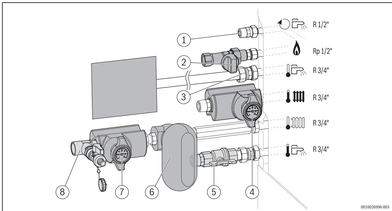
Bild 85 Armaturen-Set Zubehör CS 28-1 – Beispiel: Anschlüsse horizontal auf der linken Seite
