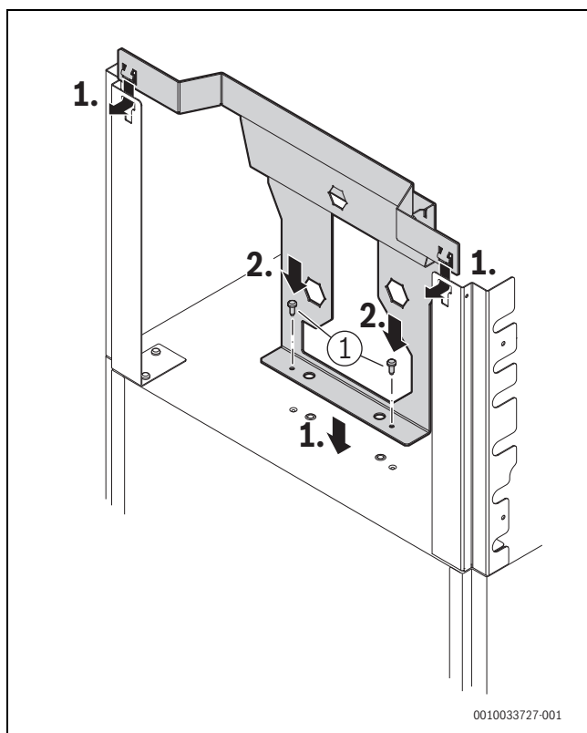
Bild 57 Basismodul (Zubehör CS 35) montieren – Schritt 2
