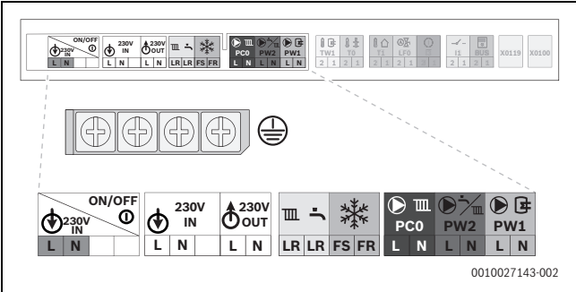
Bild 95 Netzspannungsbereich: Klemmleiste
