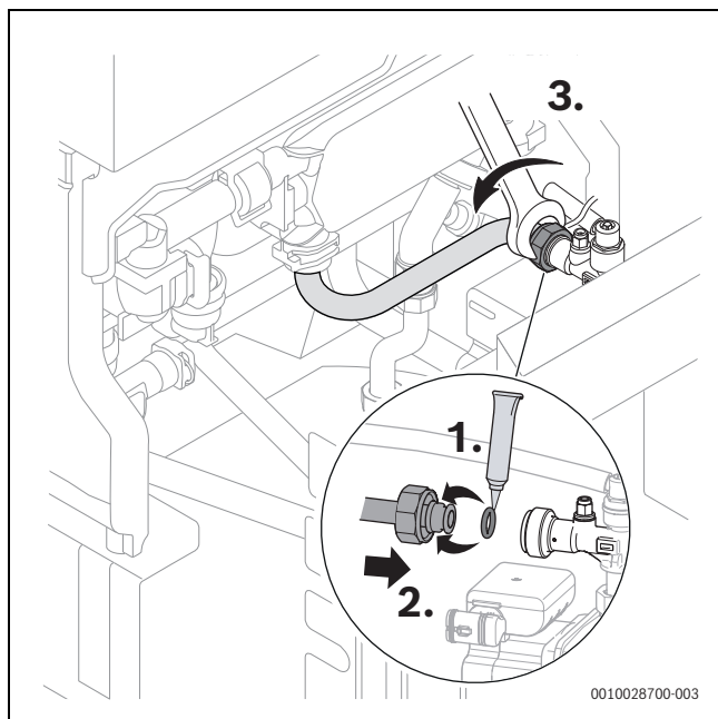
Bild 71 Kaltwasserrohr des Speicherladekreises anschließen
