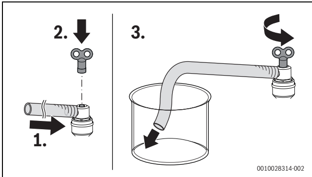
Bild 87 Warmwasserkreis und Heizkreis entlüften
