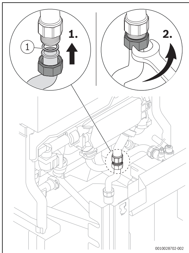
Bild 72 Warmwasserrohr des Speicherladekreises am Speicher anschließen
