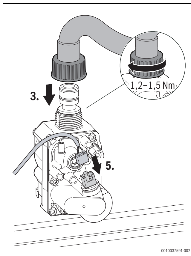
Bild 155 Gasschlauch und Stecker anschließen – Anzugsdrehmoment beachten
