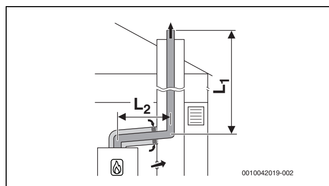
Bild 37 Starre Abgasführung im Schacht nach B 53p /B 53s mit raumluftabhängiger Luftzufuhr über die konzentrische Luft-Abgas-Führung im Aufstellraum
