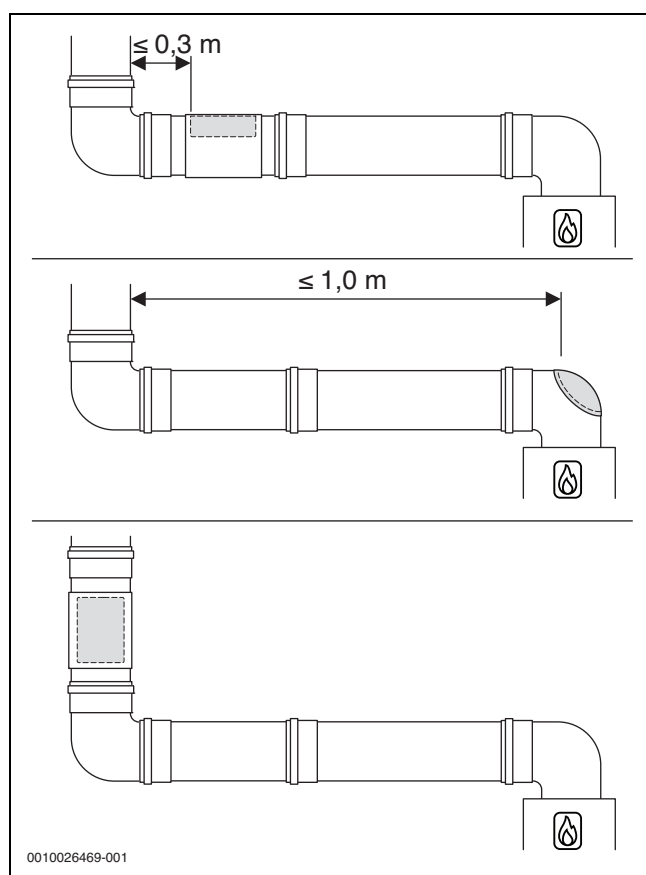
Bild 22 Anordnung der unteren Prüfföffnung
