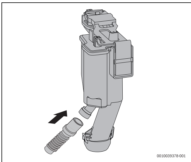
Bild 79 Schlauch am Kondensatsiphon anschließen
