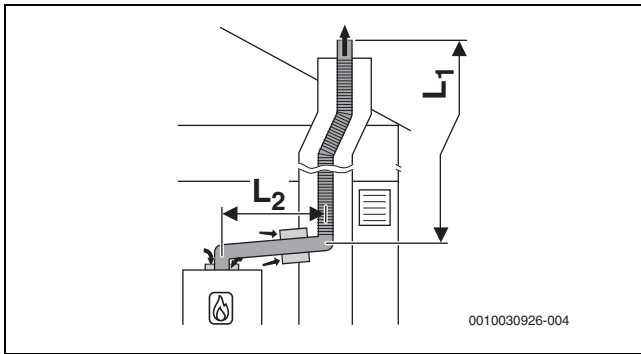
Bild 38 Flexible Abgasführung im Schacht nach B 53p mit raumluftabhängiger Luftzufuhr am Gerät und konzentrischem Verbindungsstück zwischen Aufstellraum und Schacht
