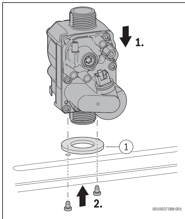
Bild 152 Gasarmatur einbauen
