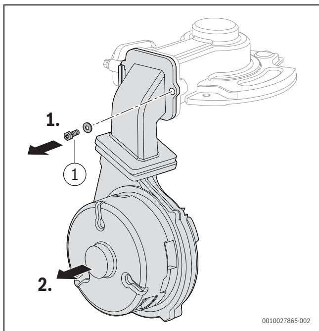
Bild 131 Mischeinrichtung und Gebläse ausbauen
