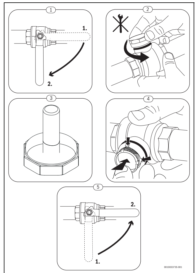
Bild 14 Reinigen des Partikelfilters
