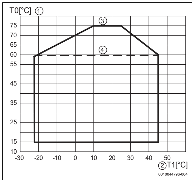
Bild 4 Wärmepumpe im Heizbetrieb ohne Zuheizer
