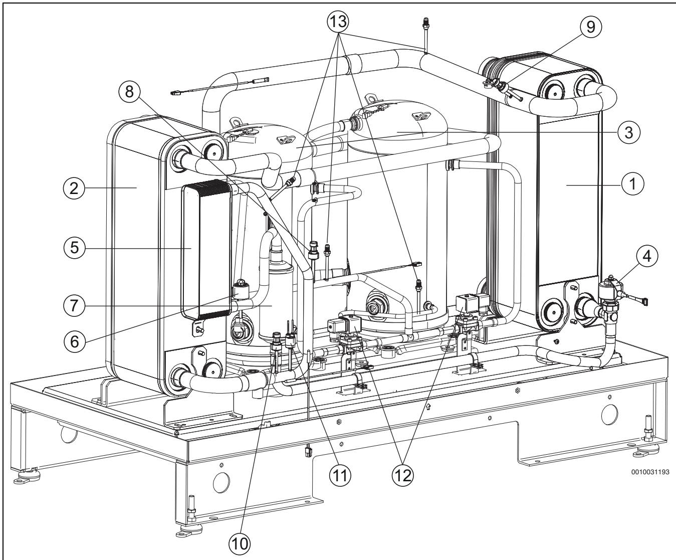
Bild 3 Produktübersicht
