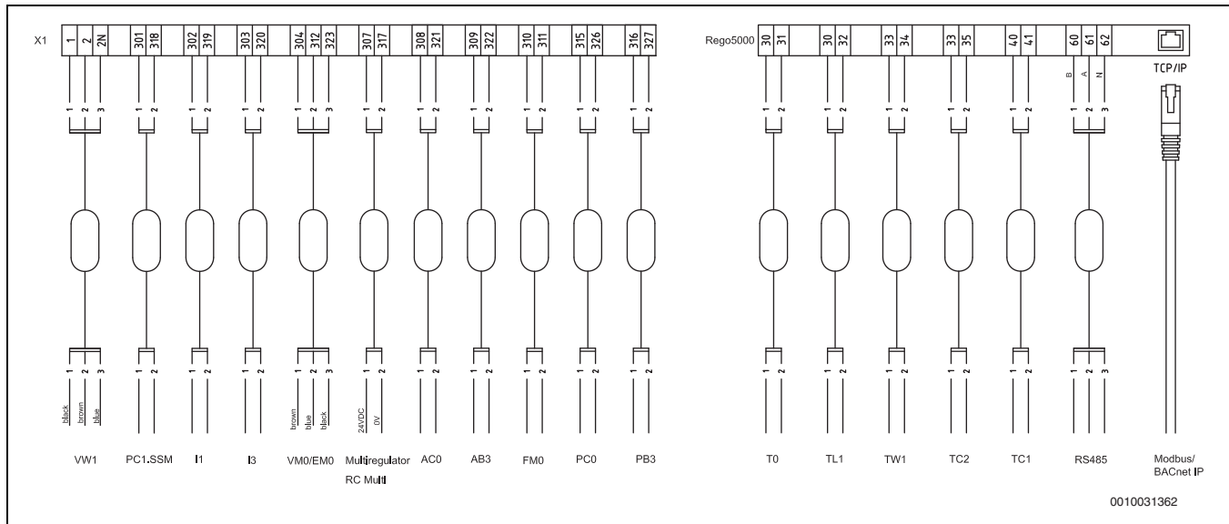
Bild 24 Anschlussplan der externen Anschlüsse
