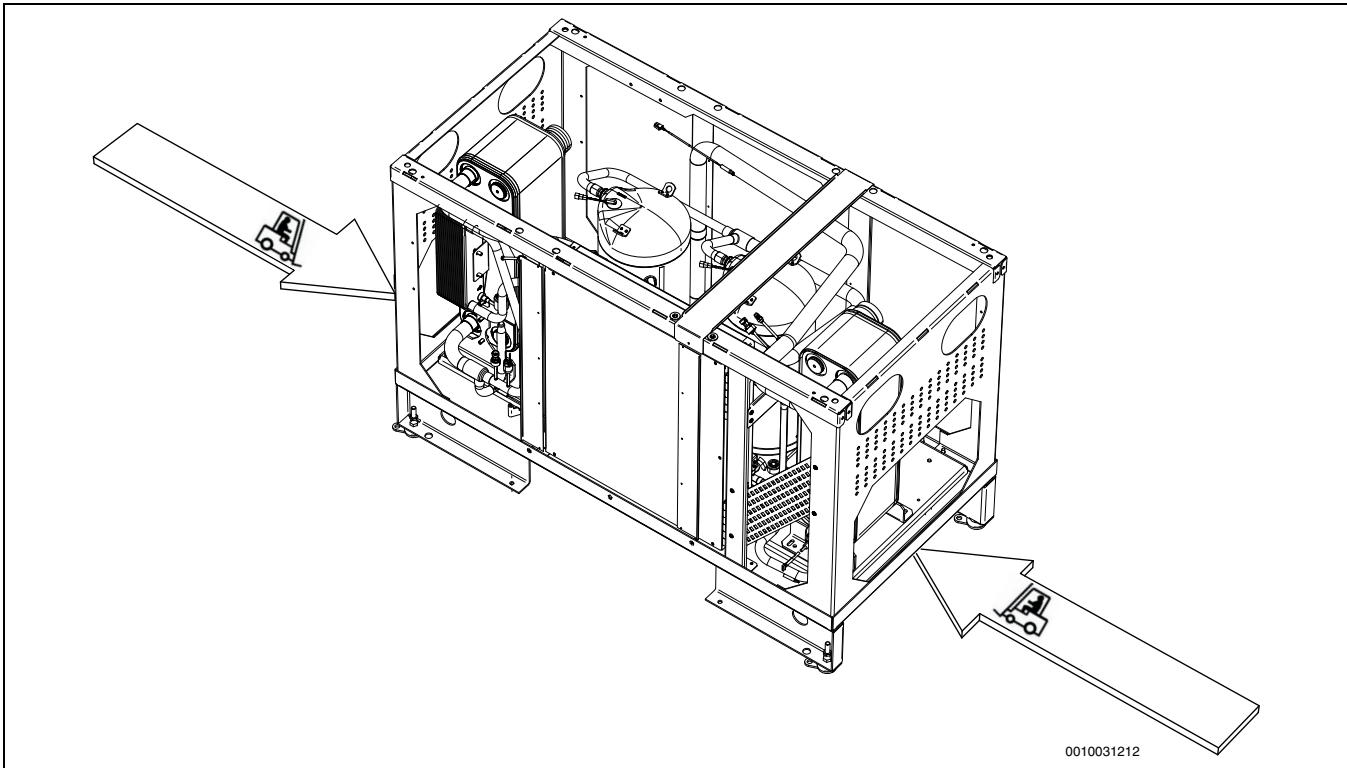
Bild 8 Beispiel für den Transport von Wärmepumpen
