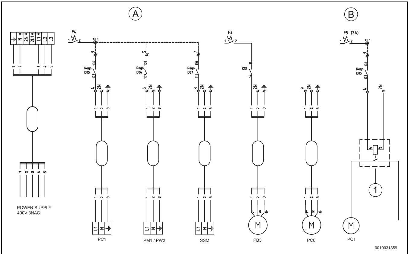
Bild 23 Anschlussplan der externen Anschlüsse
