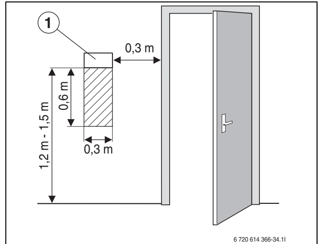
Bild 13 Empfohlener Montageort für Raumtemperaturfühler
