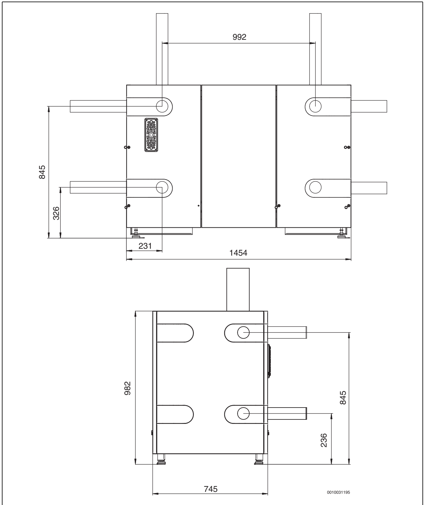
Bild 4 Abmessungen der Wärmepumpe
