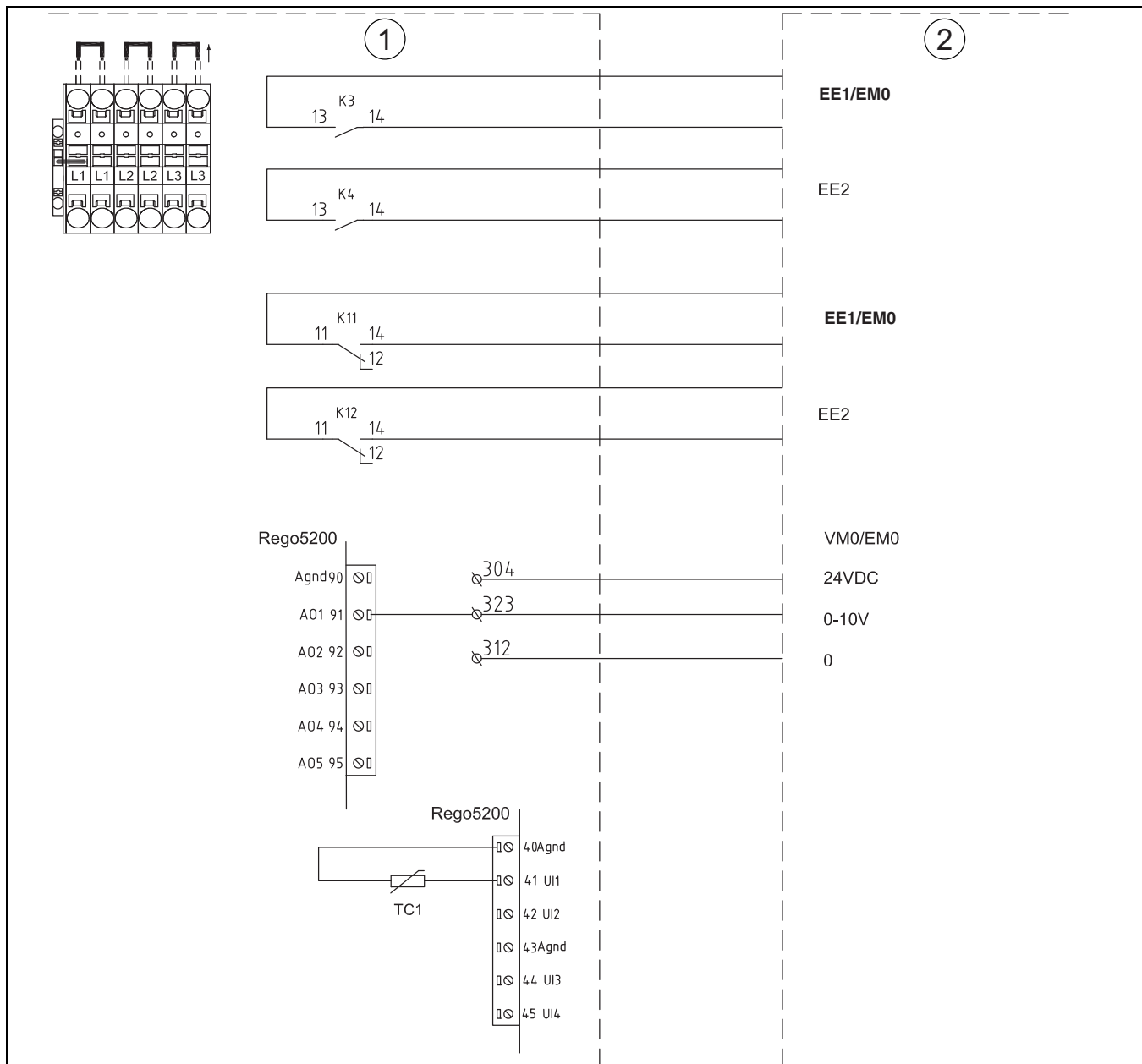
Bild 32 Anschluss des externen Zuheizers mit Mischer (22–80 kW)
