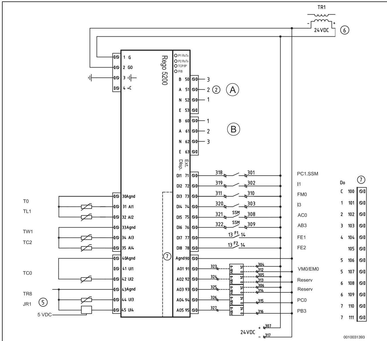
Bild 28 Schaltplan mit Steuerungssicherung
