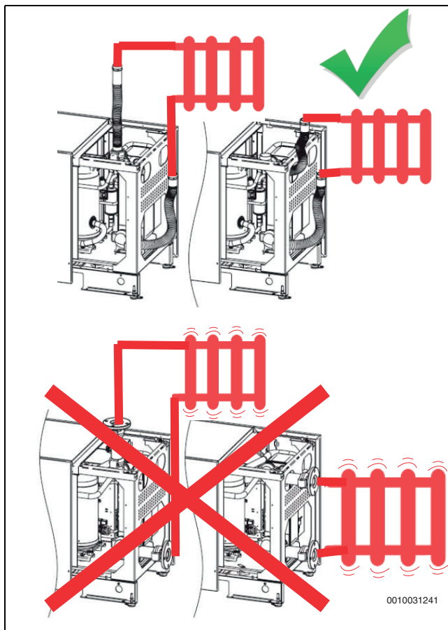
Bild 15 Schwingungsdämpfung an den Leitungsanbindungen der Heizungsanlage
