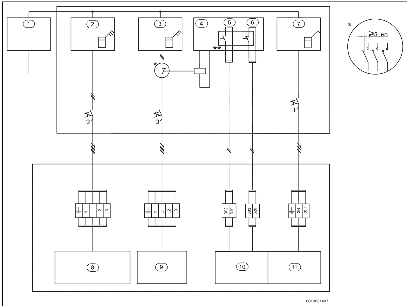
Bild 38 EVU Typ 3 mit Abschaltung von Kompressor und Elektro-Heizeinsatz
