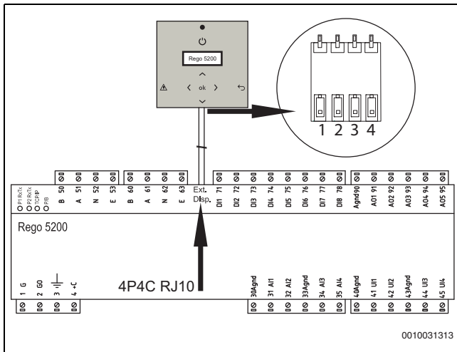
Bild 20 Überblick Klemmenkasten
