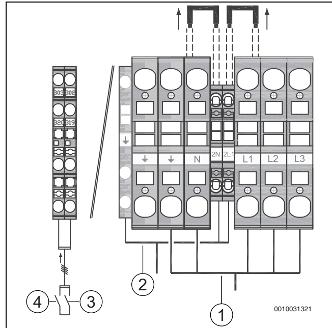
Bild 22 Belegung bei Stromversorgung im Niedertarif
