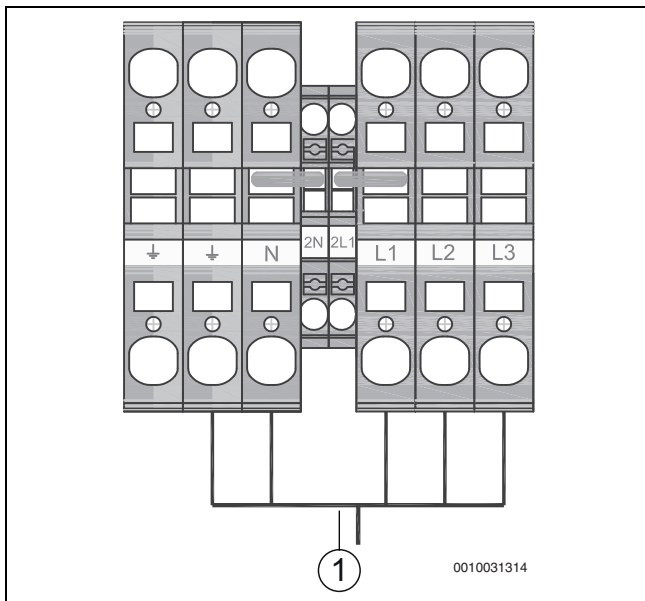
Bild 21 Stromversorgung in Standardausführung
