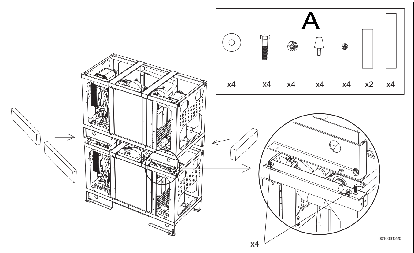
Bild 10 Stapeln von zwei Wärmepumpen
