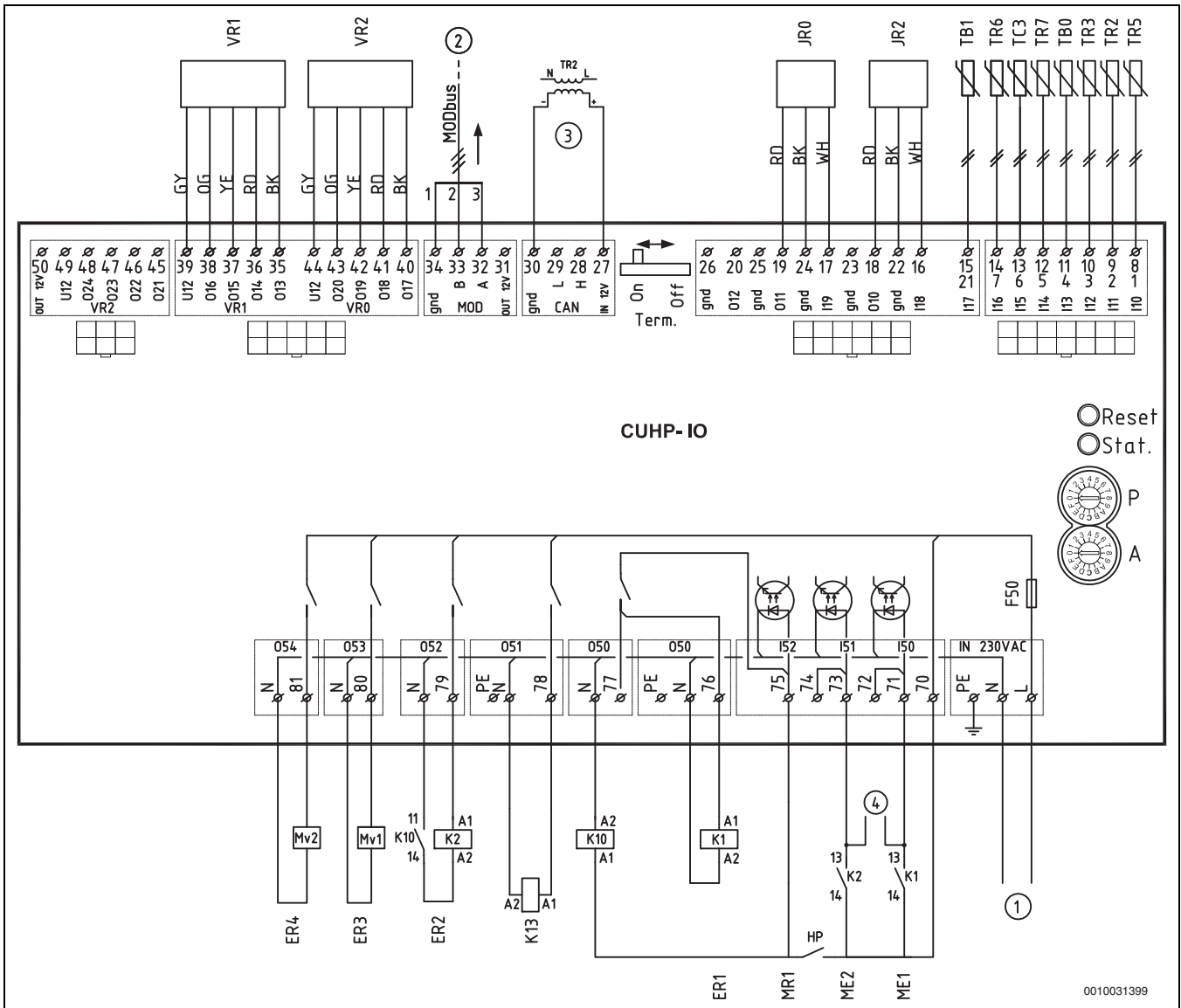
Bild 29 Schaltplan, Wärmepumpe mit Schütz
