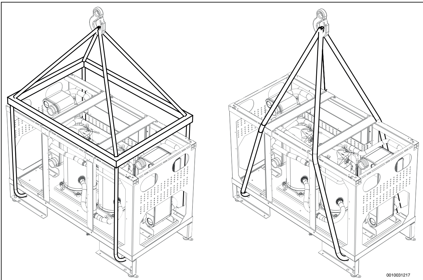
Bild 9 Beispiel für den Transport von Wärmepumpen
