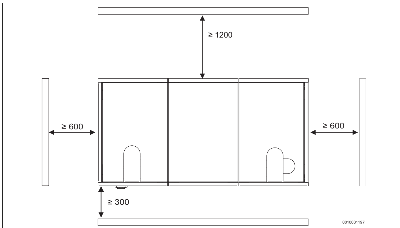
Bild 5 Mindestabstände rund um die Wärmepumpe
