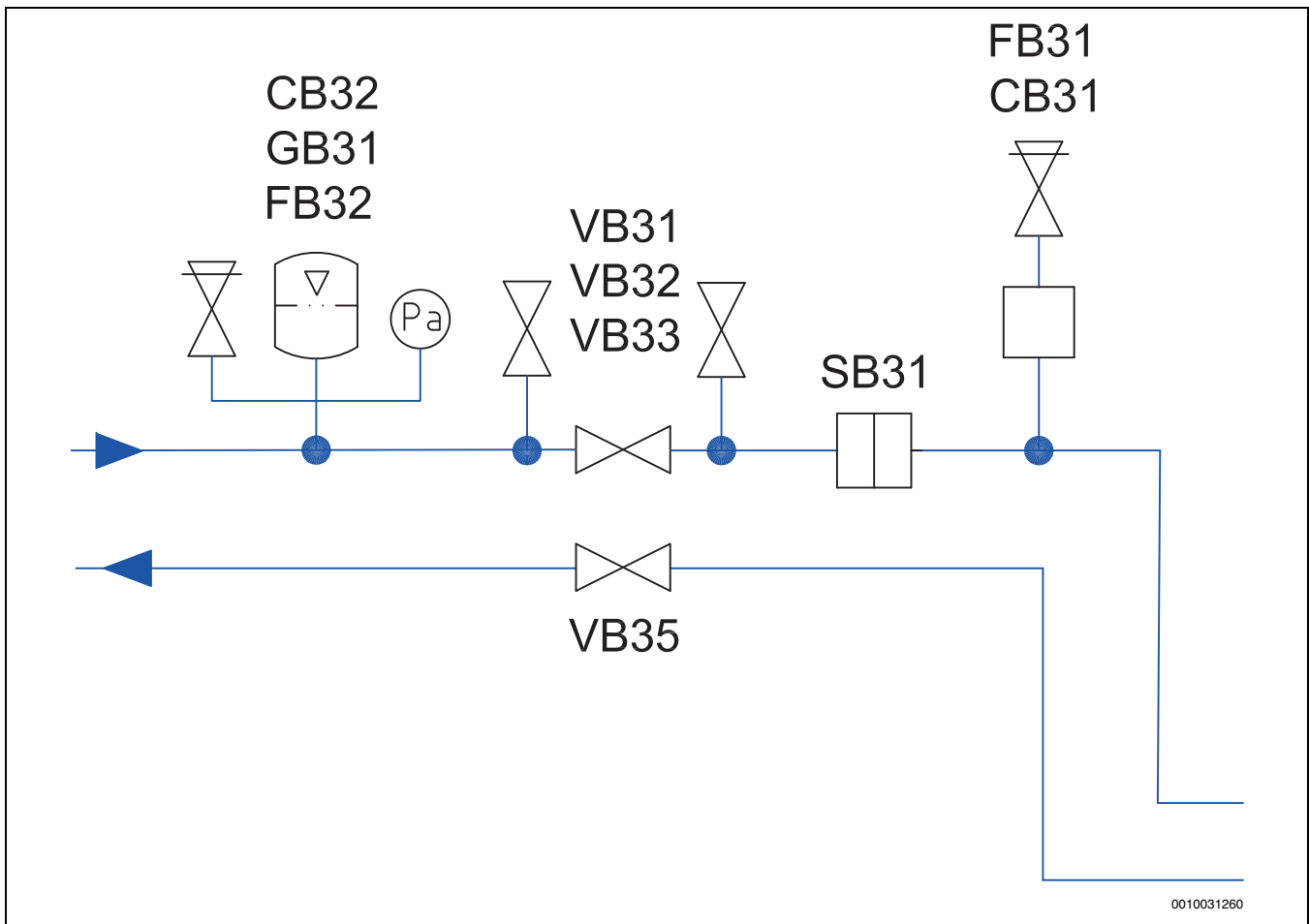
Bild 17 Quellenkreis
