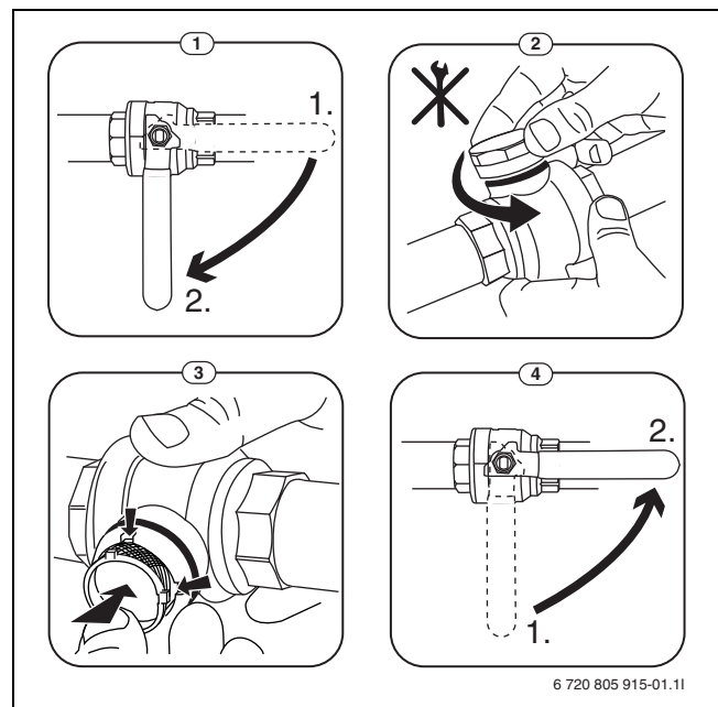
Bild 16 Siebreinigung
