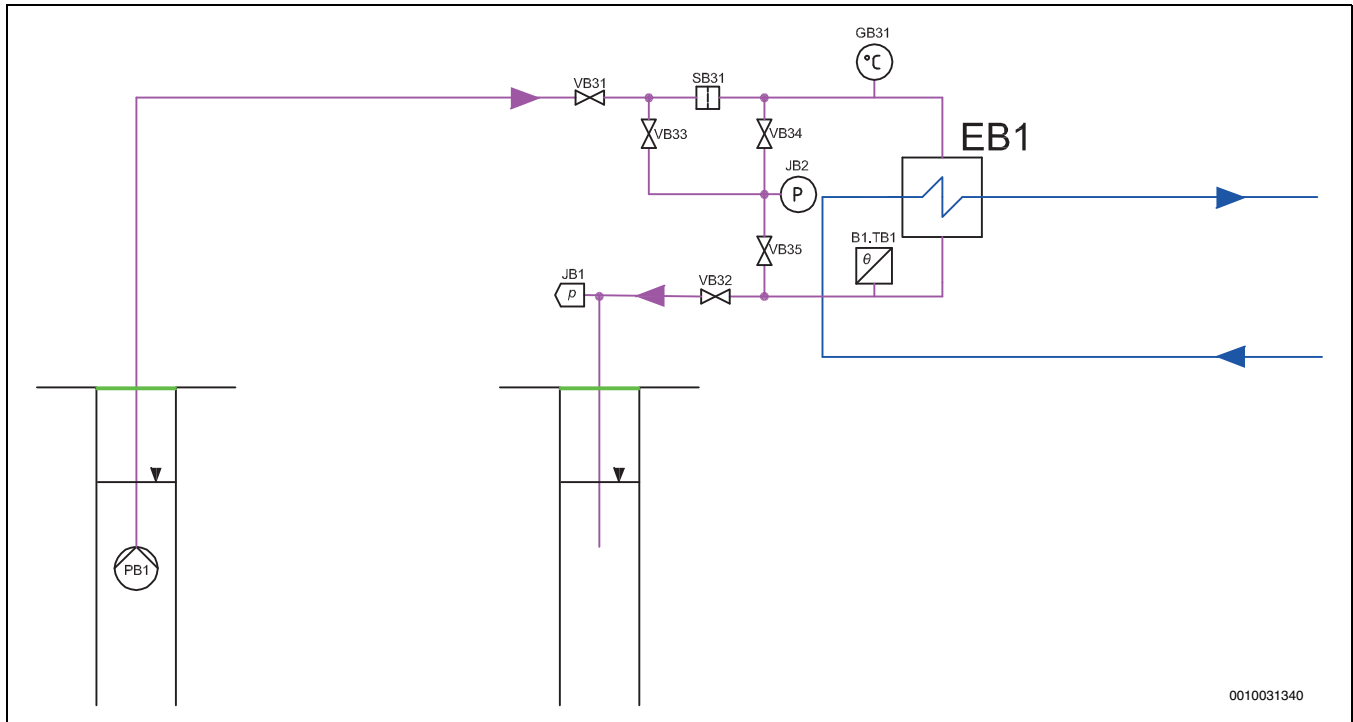
Bild 39 Grundwassersystem
