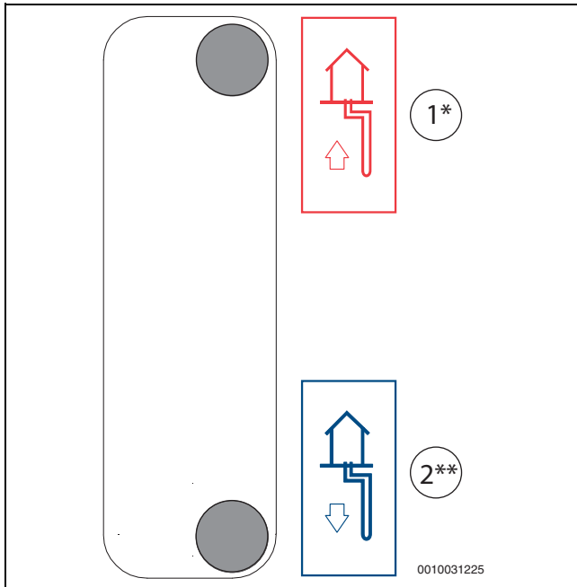
Bild 11 Solekreisanschlüsse der Wärmepumpe
