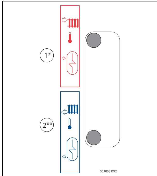
Bild 12 Heizungsanlagenanschlüsse der Wärmepumpe
