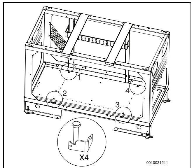
Bild 7 Transportsicherungen, Wärmepumpe
