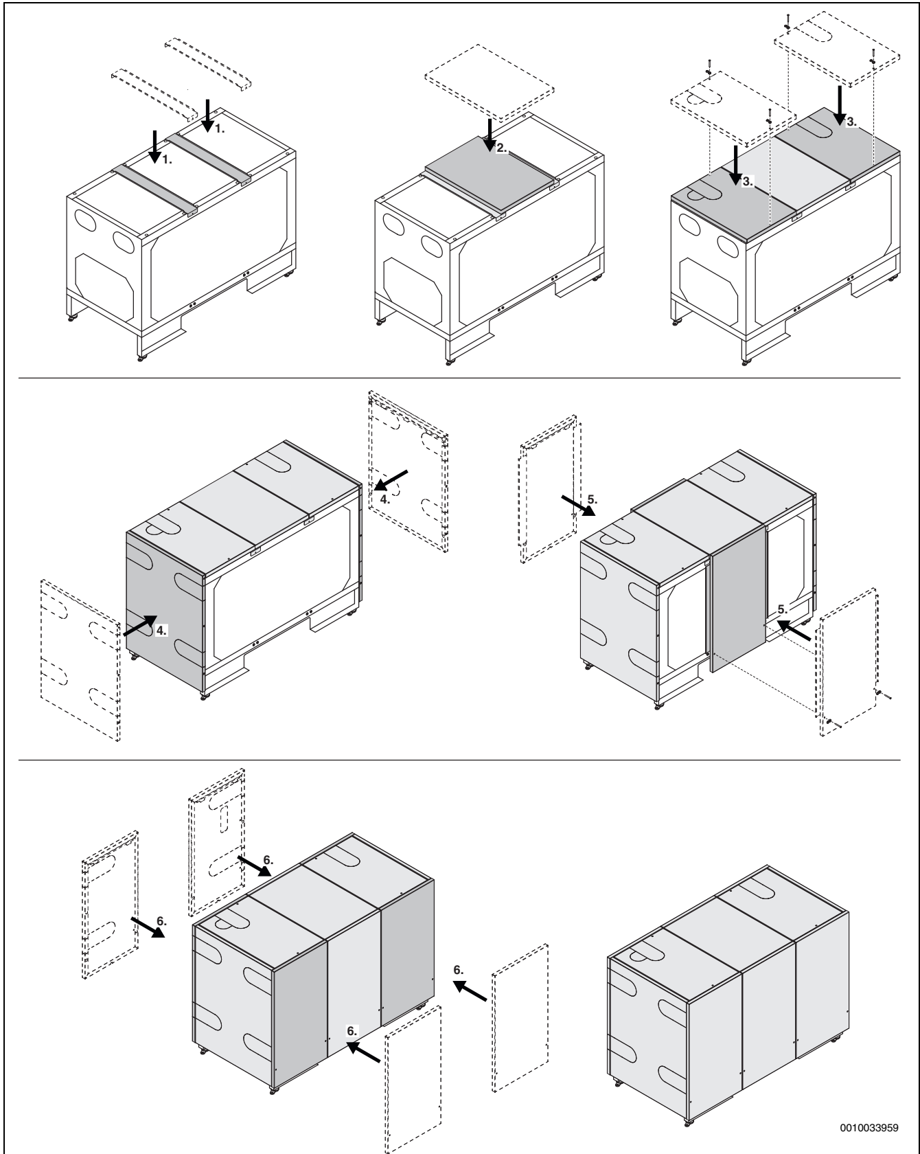
Bild 14 Montage der Blenden
