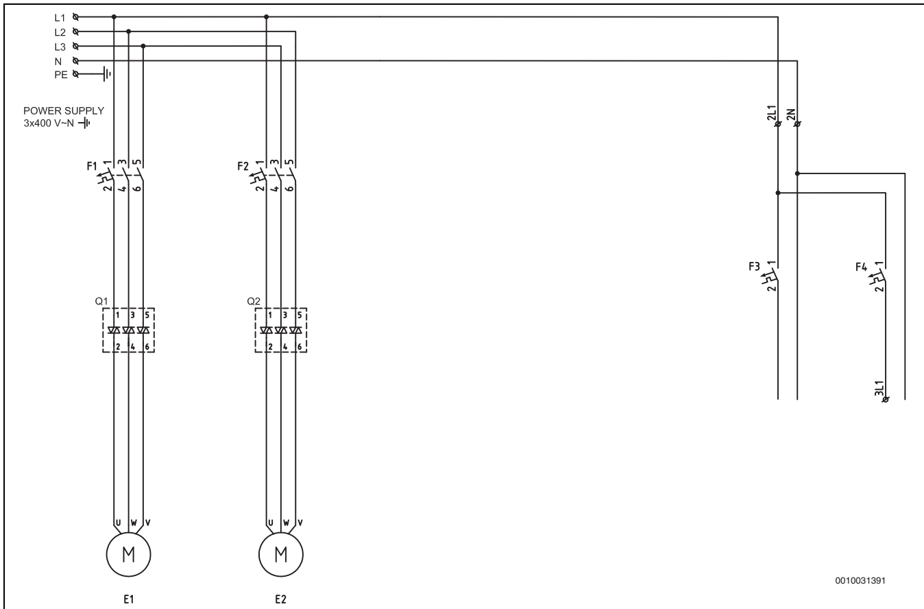
Bild 26 Betriebsschaltplan, Anlaufstrombegrenzer
