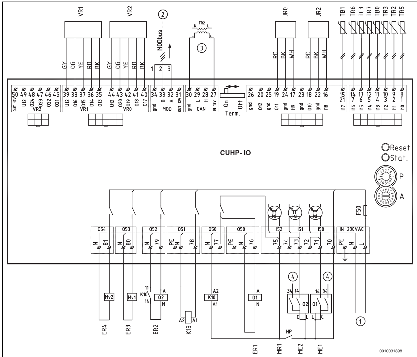
Bild 30 Schaltplan, Wärmepumpe mit Anlaufstrombegrenzer
