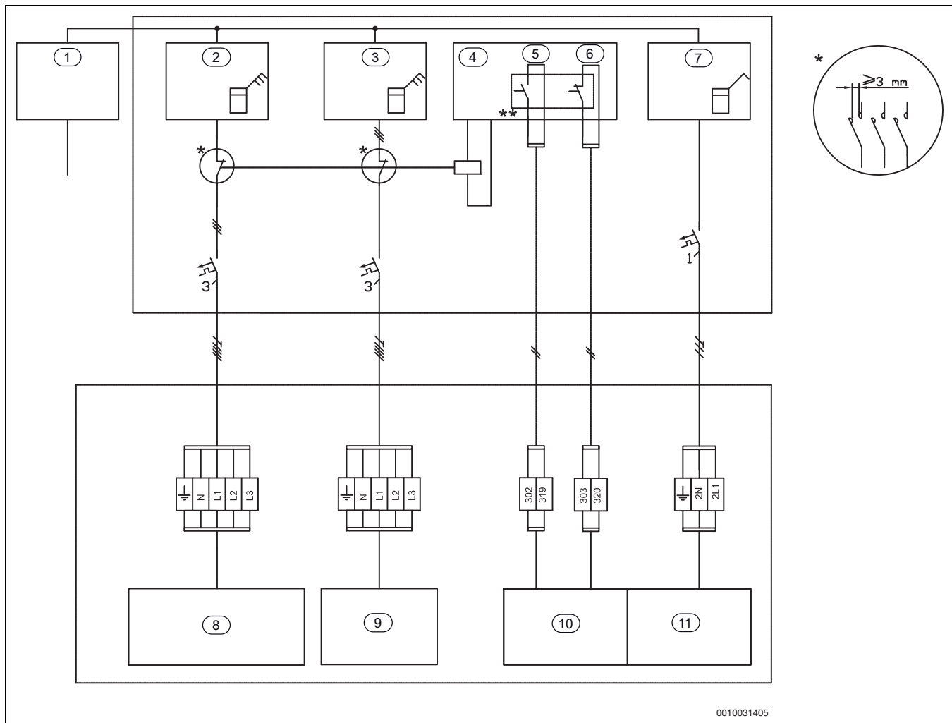
Bild 36 EVU Typ 1 mit Abschaltung des Elektro-Heizeinsatzes
