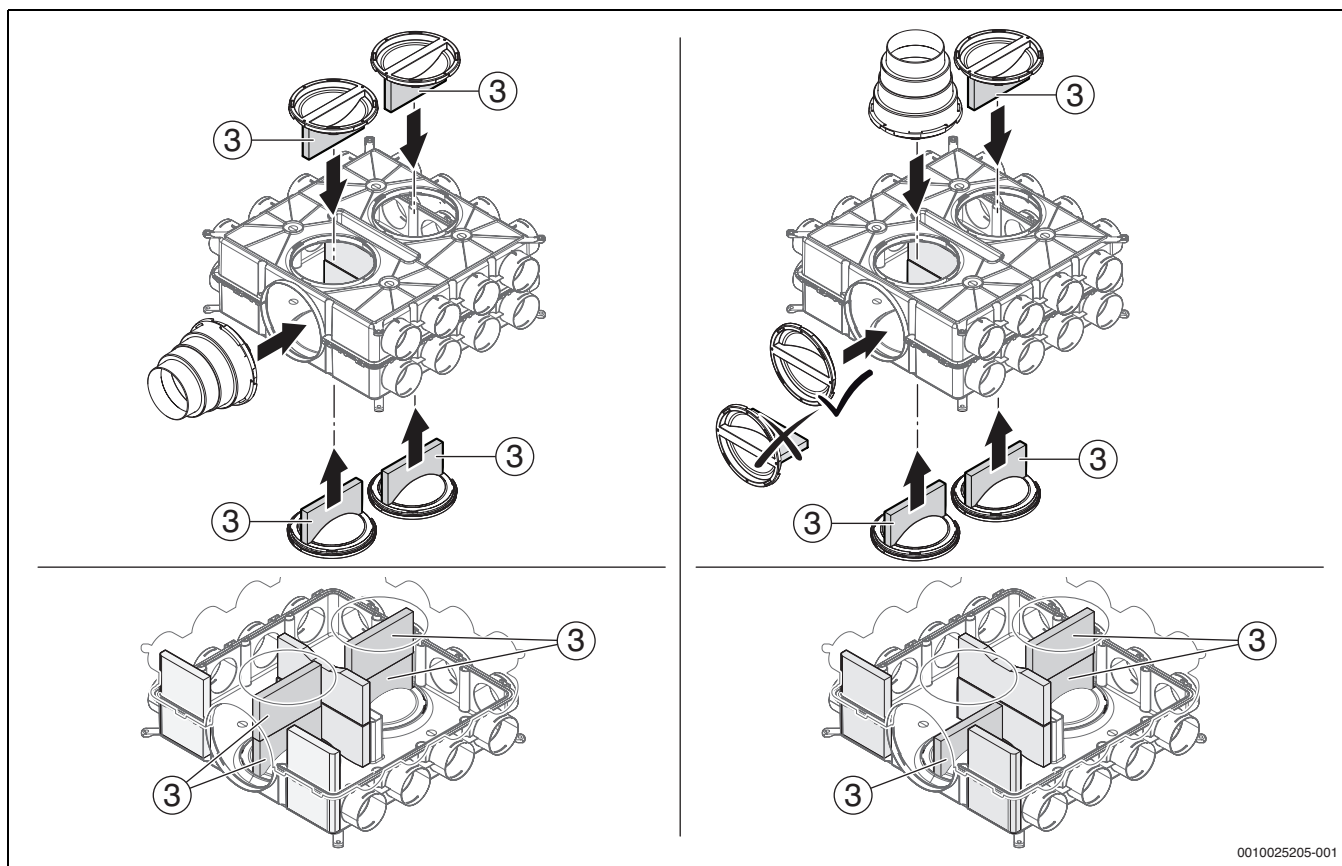
Bild 117 Montage Schalldämmset SDE VK 160
