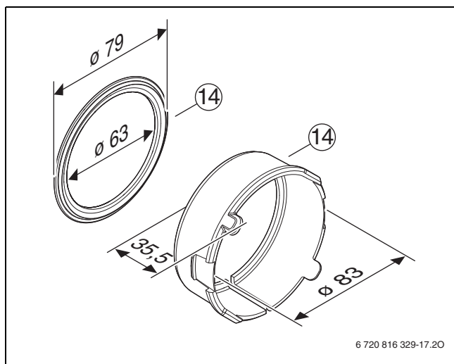
Bild 144 RRD 75 (Maße in mm)
