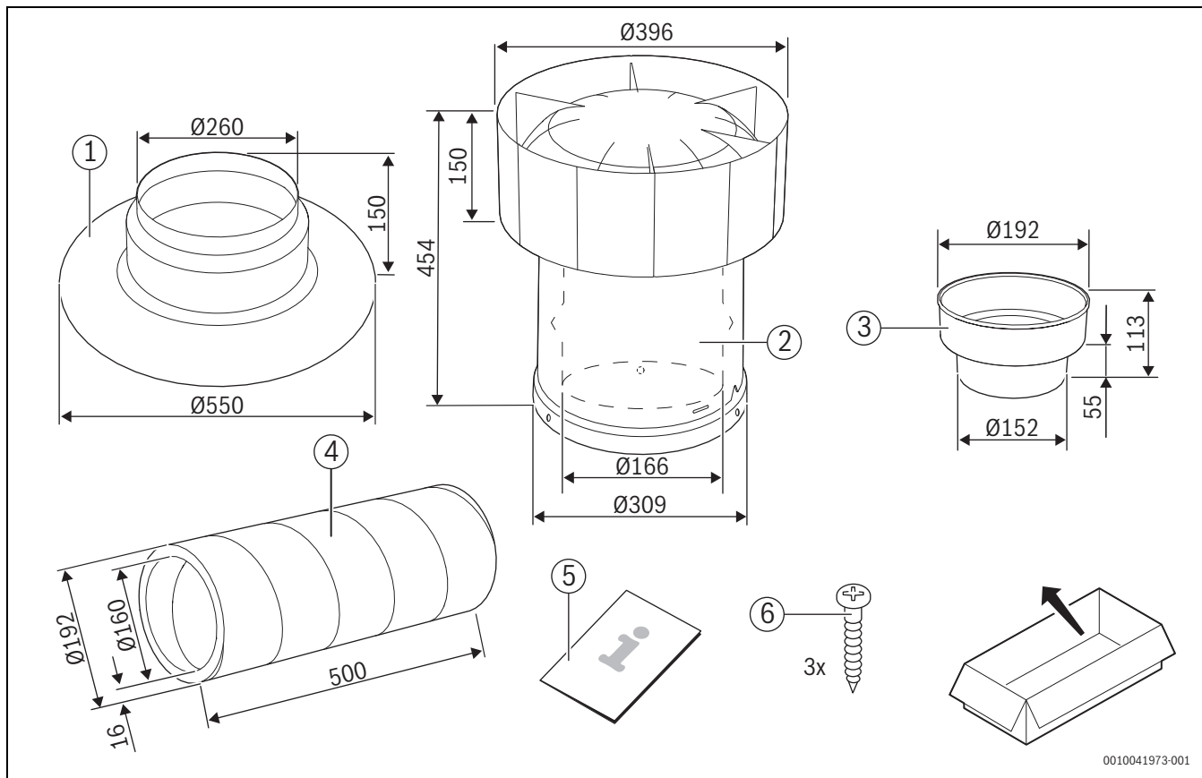
Bild 77 Lieferumfang und Maße DDF-F 160
