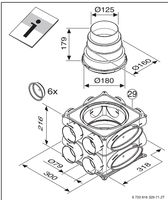
Bild 113 VK 125-2V (Maße in mm)
