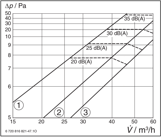
Bild 198 Strömungsgeräusche bei verschiedenen Volumenströmen – Abluft
