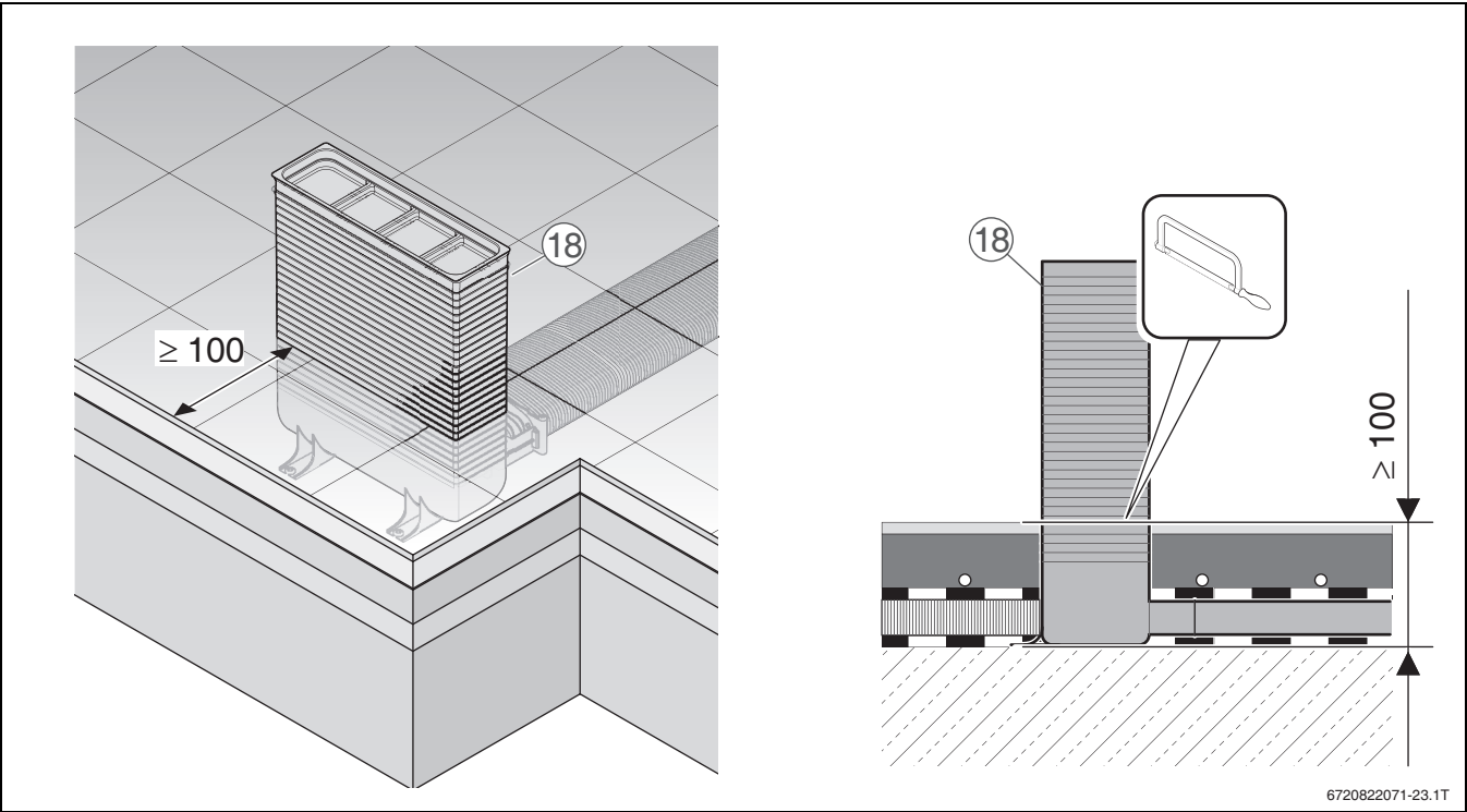
Bild 171 RRU 75-2: Einsatzbeispiel (Maße in mm)
