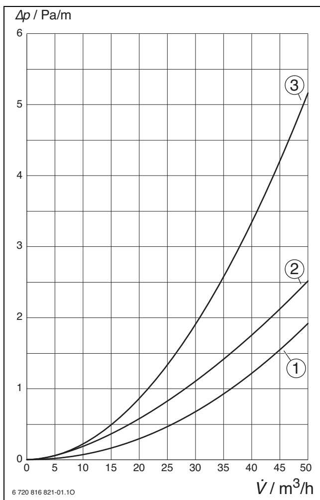
Bild 151 Druckverlust Flachkanal FK 140
