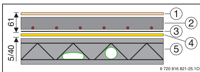
Bild 98 Flach-/Rundkanal in Rohbetondecke (Maße in mm)
