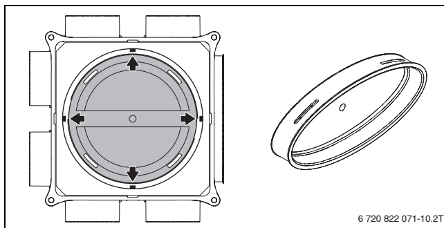
Bild 105 Revisionsdeckel
