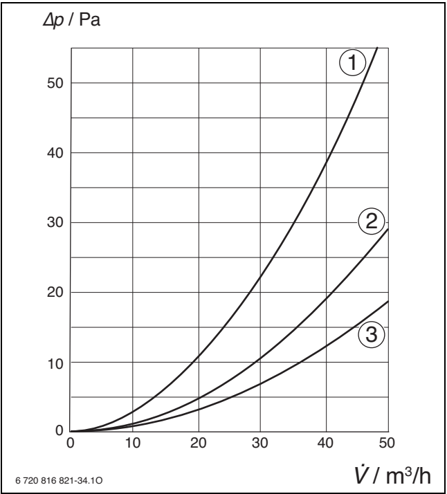
Bild 200 Druckverlust bei Verwendung als Abluftventil
