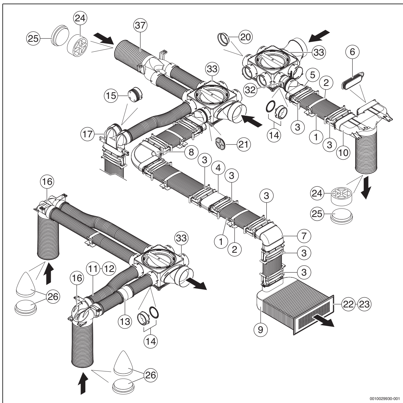
Bild 103 Luftverteiler mit VK 125-1S, beispielhafte Luftkanalführung
