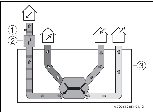
Bild 45 Lüftungsgerät mit elektrischem Nachheizregister
