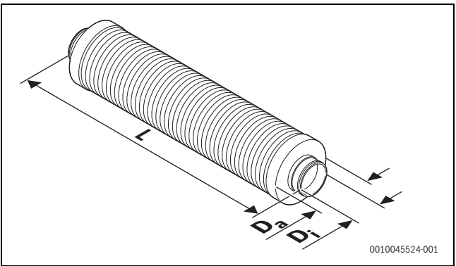
Bild 92 Schalldämpfer SDF... (Maße in mm)
