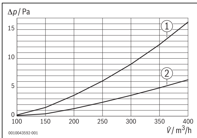
Bild 62 Druckverlust
