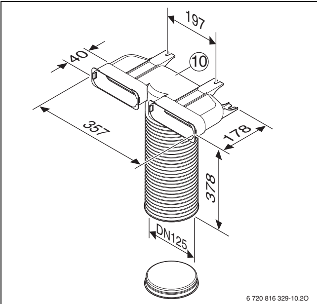
Bild 156 FKU 140-3 (Maße in mm)
