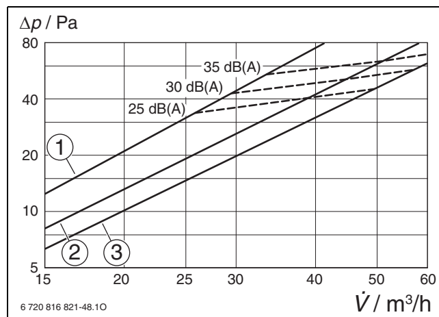
Bild 203 Strömungsgeräusche bei verschiedenen Volumenströmen
