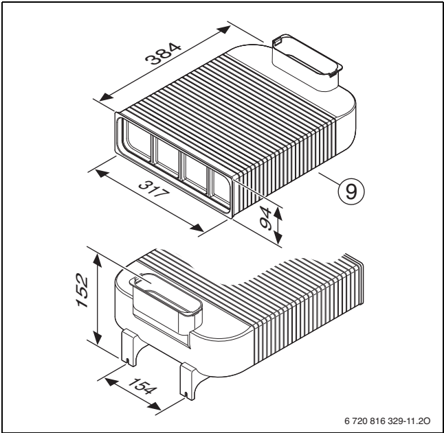
Bild 168 FKU 140-2 (Maße in mm)
