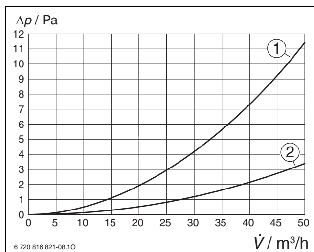
Bild 159 Druckverlust FKU 140-3 – Abluft
