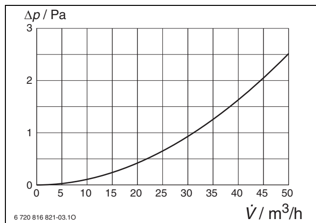
Bild 153 Druckverlust FKB 140-1
