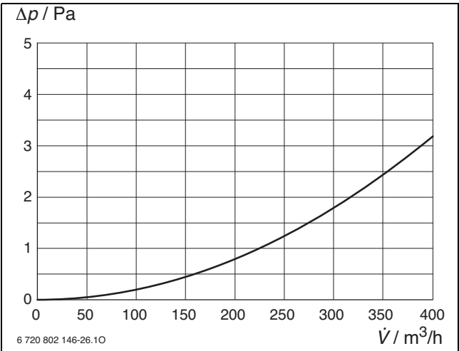
Bild 67 Druckverlust BEPP 160-1
