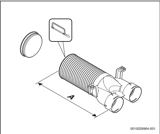
Bild 141 Kürzung Ventilanschluss RRU 75-5
