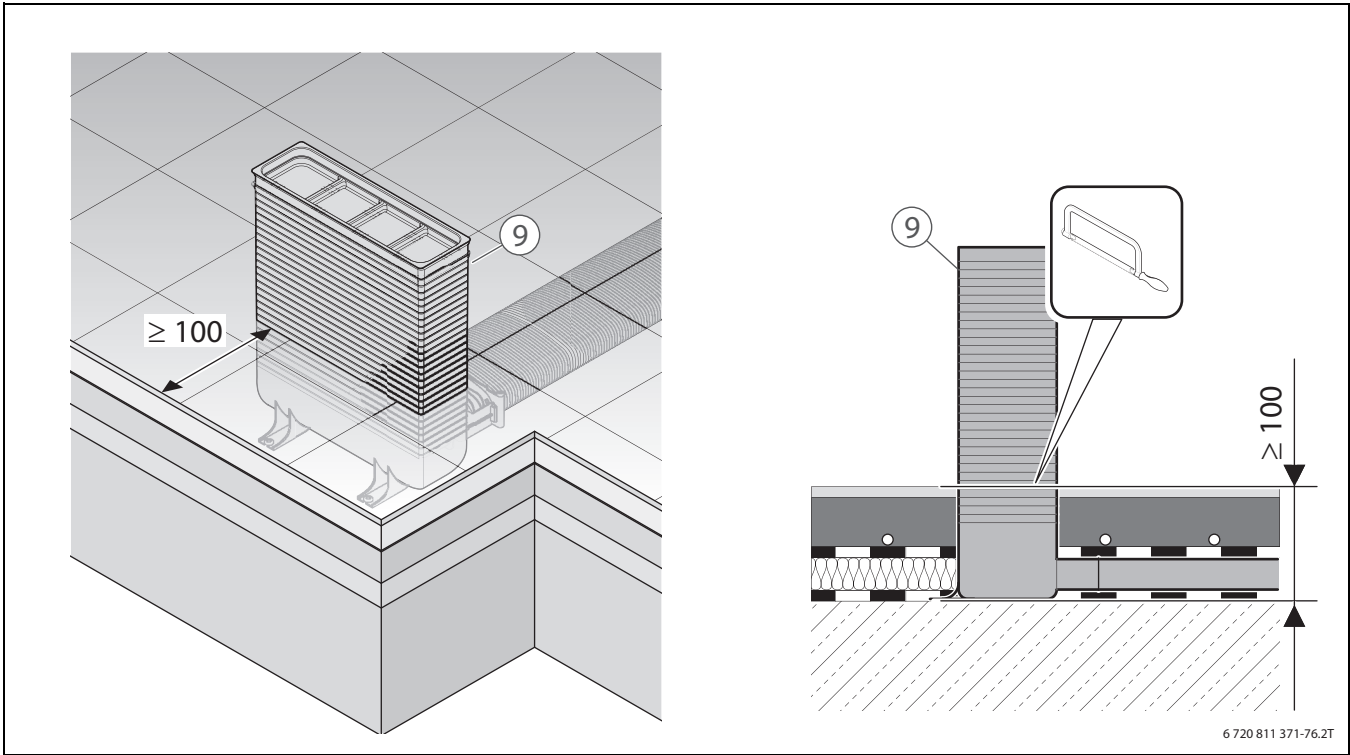
Bild 169 FKU 140-2: Einsatzbeispiel (Maße in mm)
