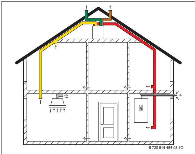
Bild 213 Vent 5000 C und raumluftunabhängige Feuerstätte
