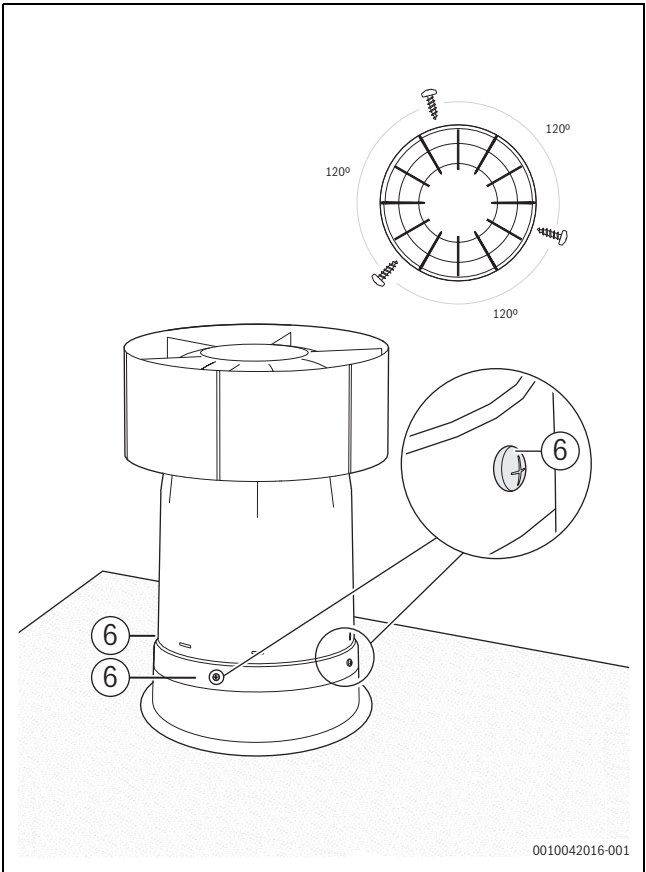
Bild 78 DDF-F 160 montiert
