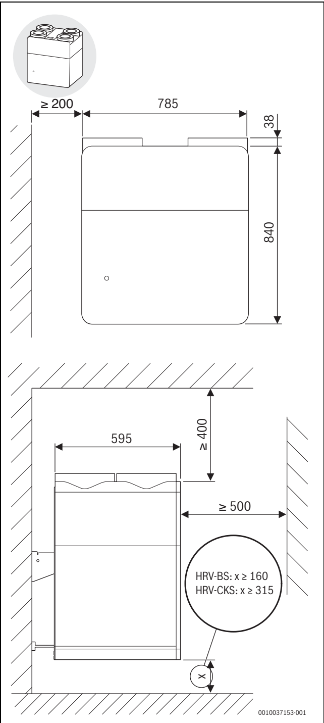
Bild 33 Abmessungen und Mindestabstände Wand- installation V5001C... - Mindestabstände wenn Anschlussstutzen senkrecht
