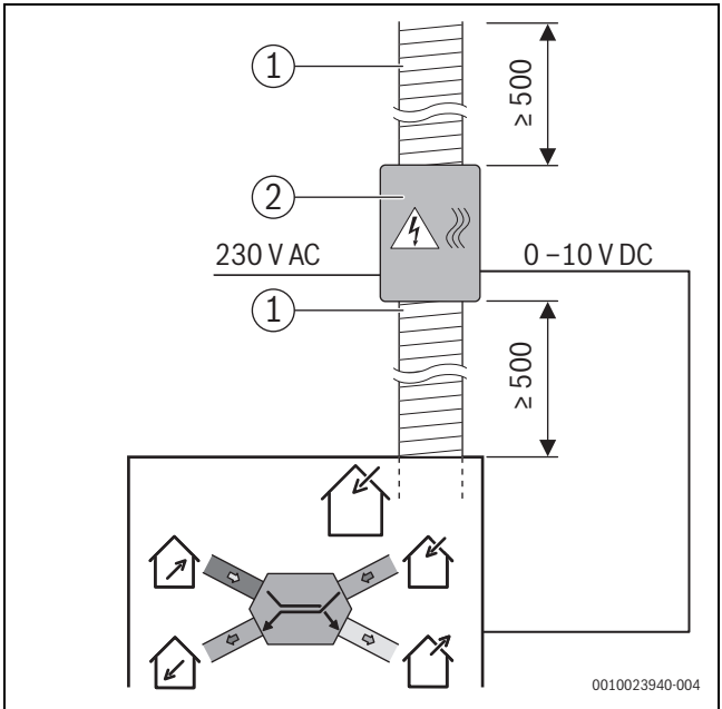
Bild 46 Position zusätzliches Vorheizregister HRE 160-1200
