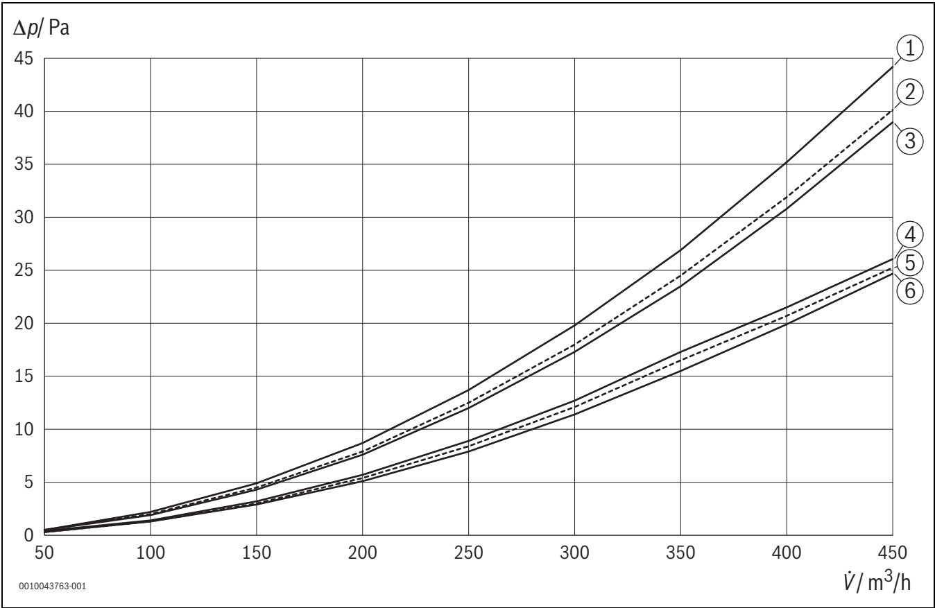
Bild 76 Druckverluste Dachdurchführung DDF-S 160
