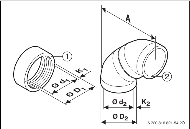
Bild 66 Steckverbinder CEPP 160-3 ... und Bogen BEPP 160-1
