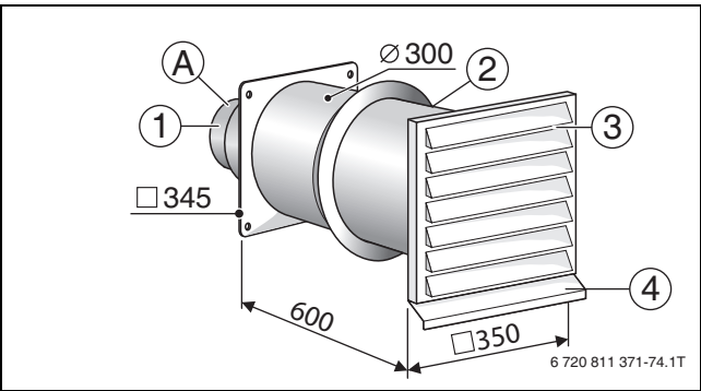
Bild 83 Abmessungen Wanddurchführung WG 160/1 (Maße in mm)
