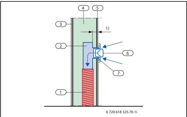
Bild 176 Einbaubeispiel Abluftventil AV 125
