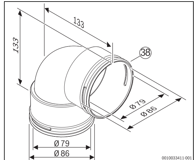
Bild 135 RRB 75-2 (Maße in mm)
