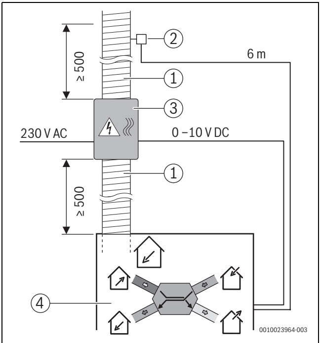
Bild 47 Position Nachheizregister HRE-A 160-1200
