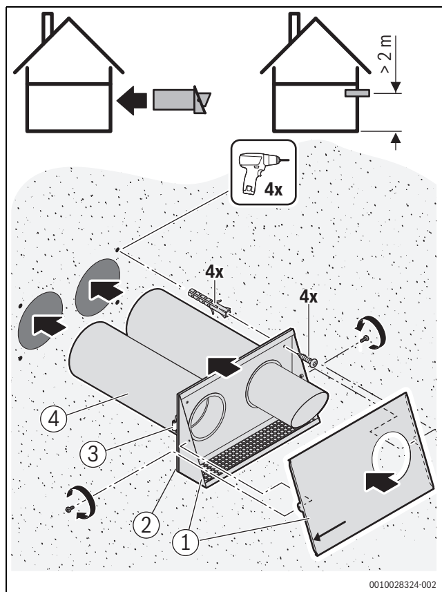
Bild 71 Montagebeispiel
