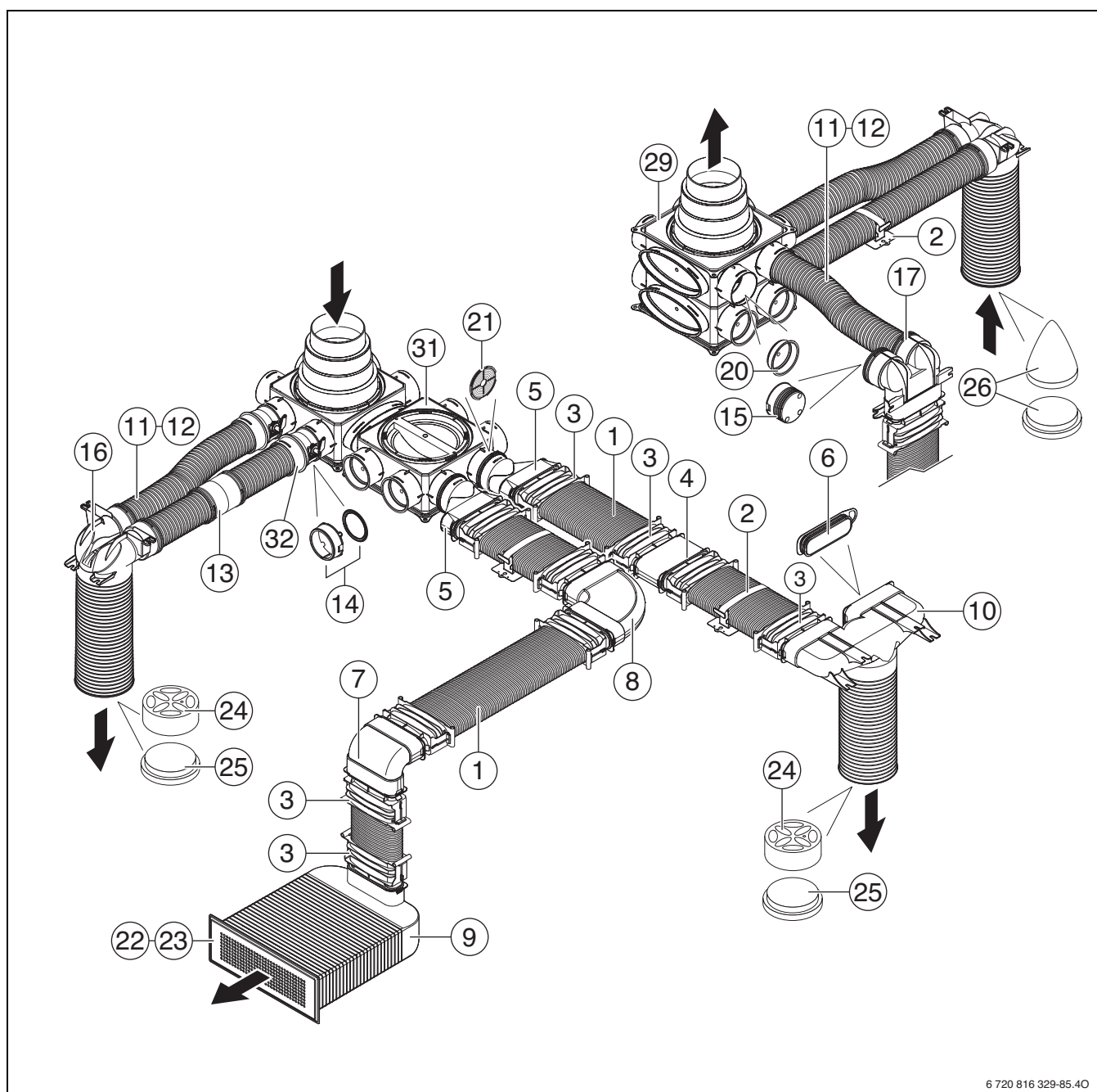
Bild 101 Luftverteiler mit VK 125-2V und VK 125-2H, beispielhafte Luftkanalführung
