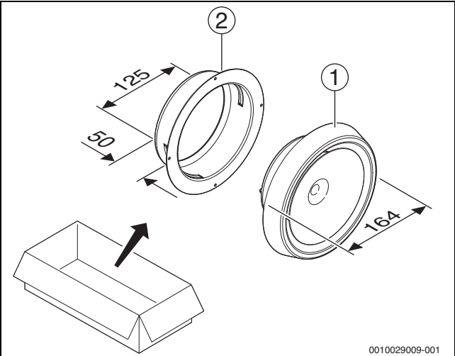
Bild 181 ZU 125 (Maße in mm)
