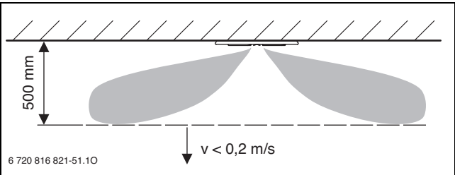
Bild 207 Wurfweite und Strömungsgeschwindigkeit
