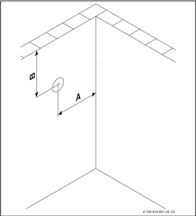
Bild 175 Mindestabstände bei Wandinstallation bei Verwendung eines Umlenkstücks
