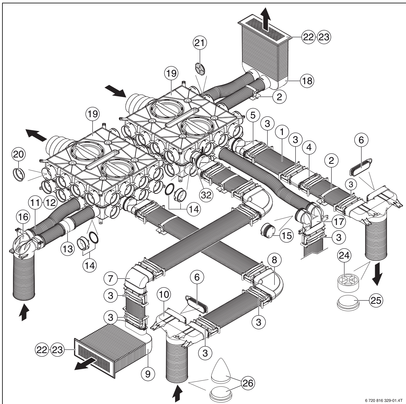
Bild 100 Luftverteiler mit VK 160, beispielhafte Luftkanalführung
