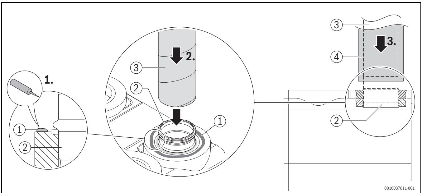
Bild 54 Wickelfalzrohr und Dämmung montieren
