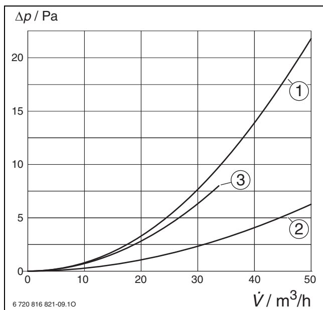
Bild 119 Zusätzlicher Druckverlust je Strang nach Kanalart
