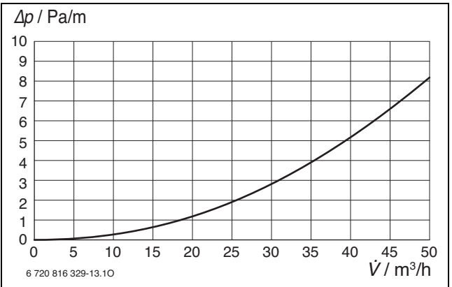
Bild 133 Druckverlust Rundkanal RR 75-1/2 – gerade
