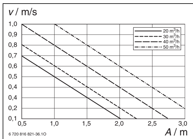
Bild 202 Wurfweite bei verschiedenen Volumenströmen
