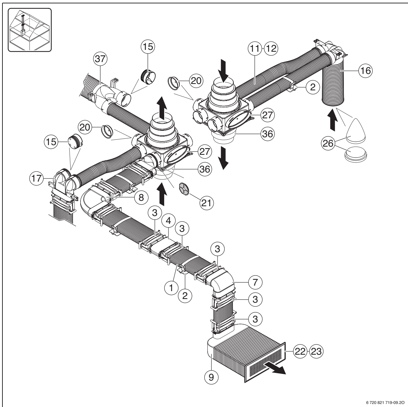
Bild 104 Luftverteiler als Etagenverteiler, beispielhafte Luftkanalführung
