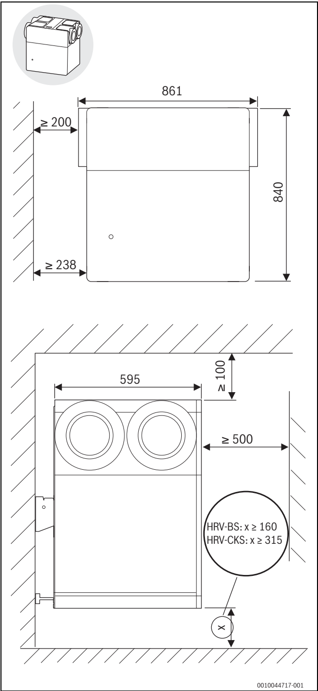
Bild 34 Abmessungen und Mindestabstände Wand- installation V5001C... - Mindestabstände wenn Anschlussstutzen waagerecht
