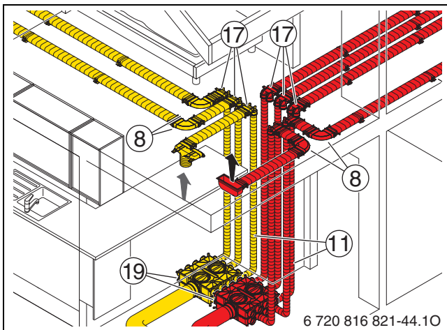
Bild 95 Luftverteilung-Kanalsystem
