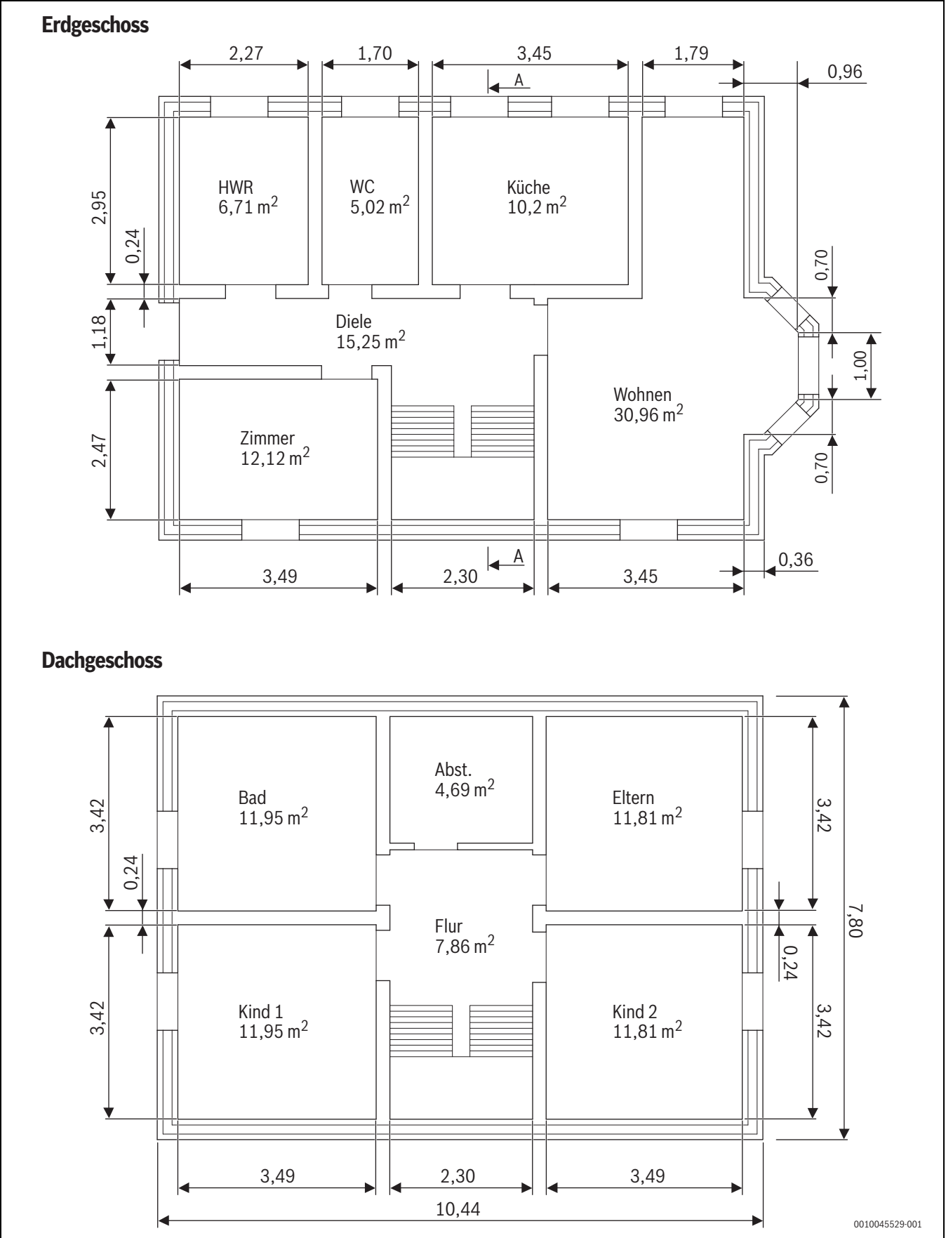
Bild 226 Beispielauslegung - Grundriss (Maße in m)
