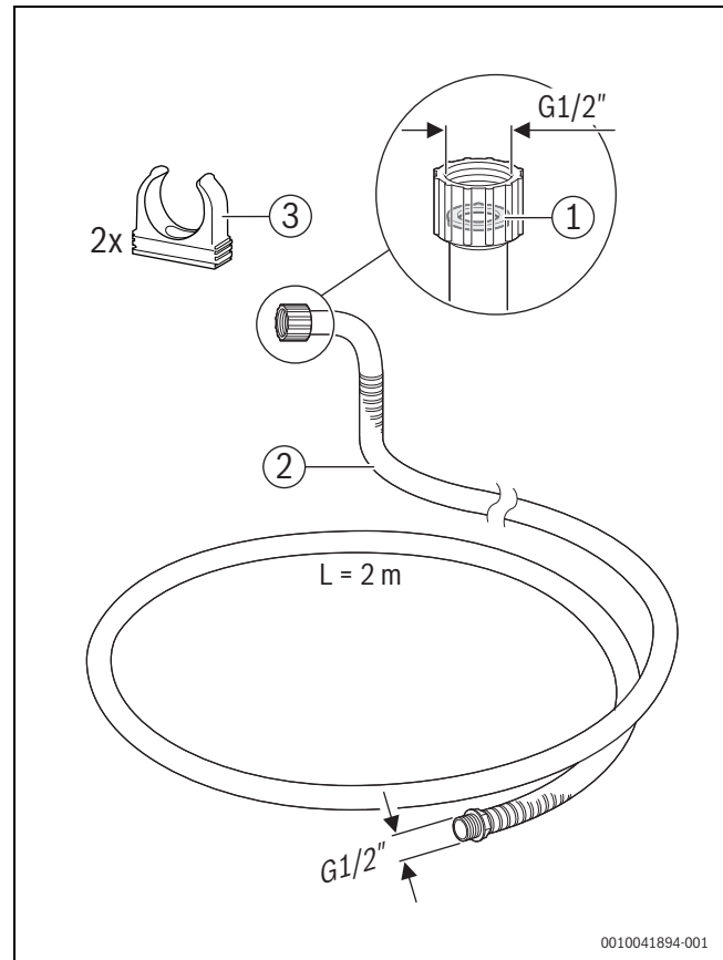
Bild 27 Schlauchsiphon-Set
