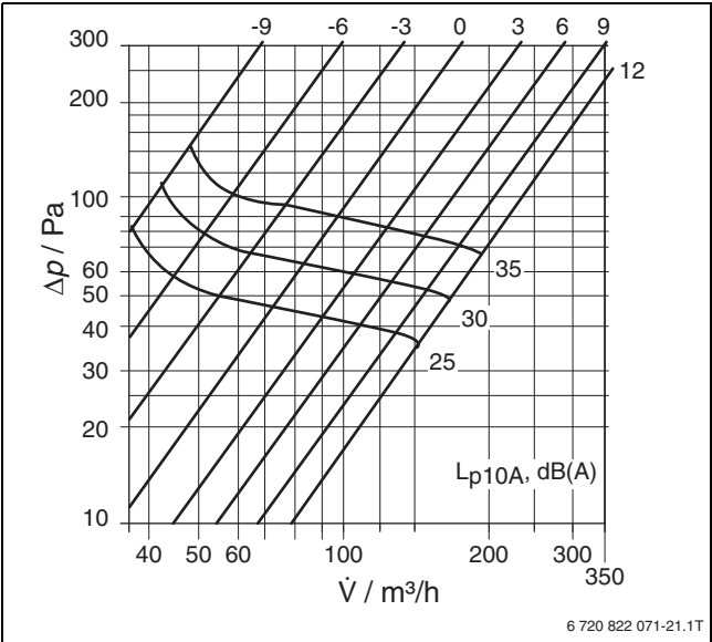
Bild 184 Strömungsgeräusche ZU 125 bei Stellung des Ventilkonus S
