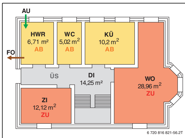
Bild 3 Aufteilung Lüftungsbereiche
