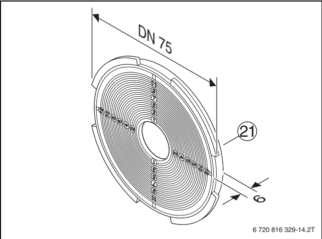
Bild 122 VKD (Maße in mm)
