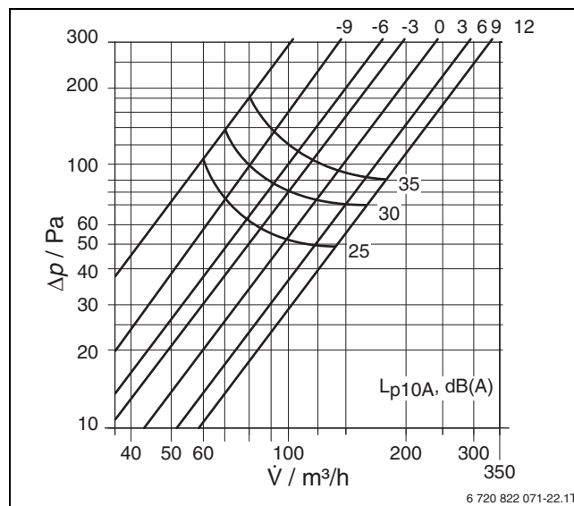
Bild 188 Strömungsgeräusche AV 125 bei Stellung des Ventilkonus S
