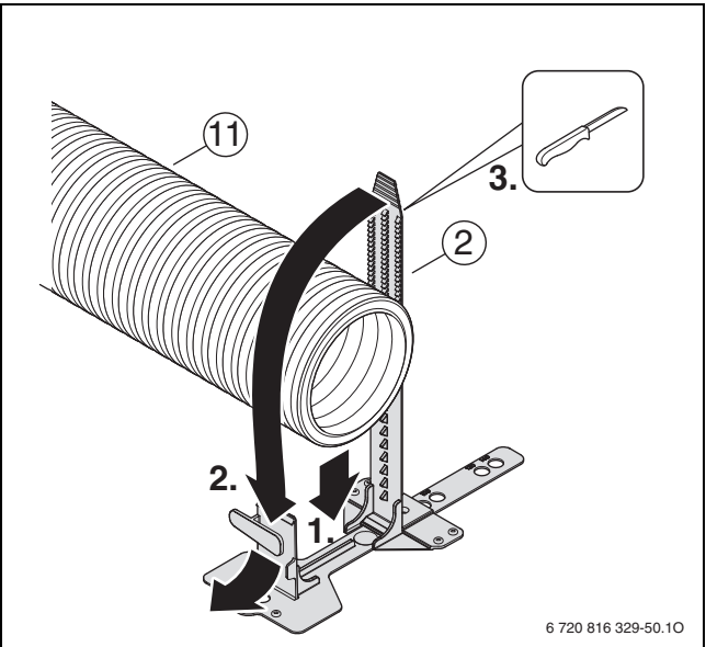
Bild 132 RR 75-1/2 + FKH 140
