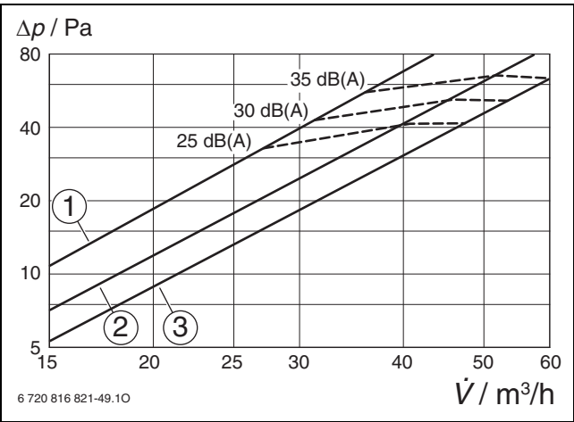
Bild 206 Strömungsgeräusche bei verschiedenen Volumenströmen
