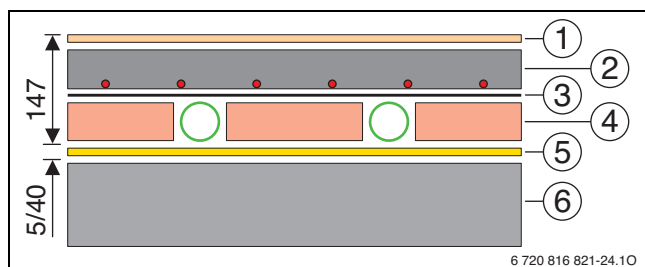
Bild 97 Rundkanal auf Rohbetondecke (Maße in mm)
