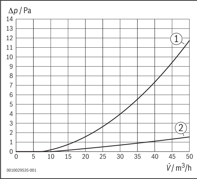
Bild 142 Druckverlust RRU 75-5 – Zuluft
