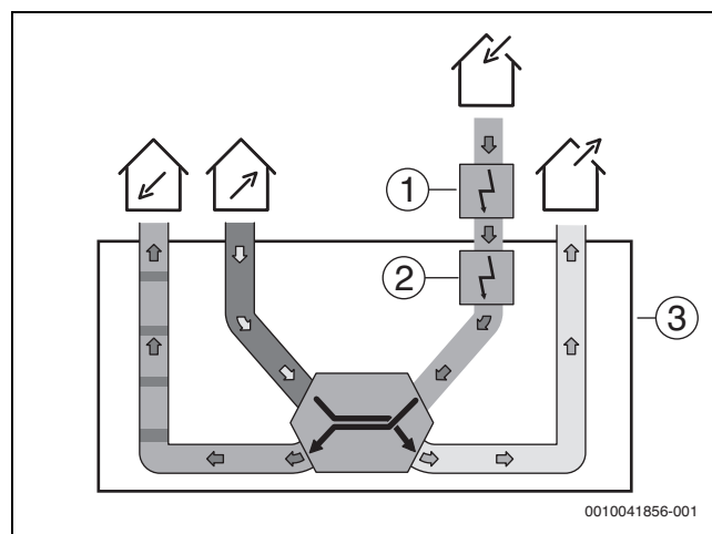
Bild 43 Lüftungsgerät mit zusätzlichem elektrischen Vorheizregister
