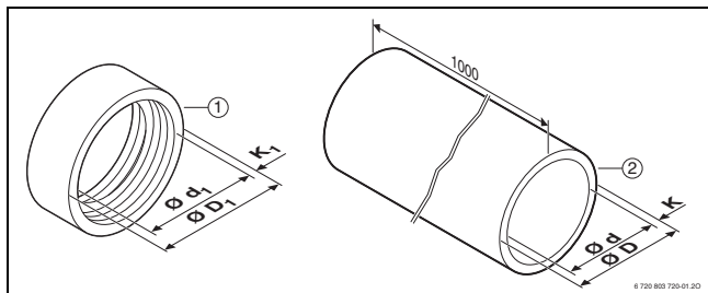
Bild 68 Steckverbinder CEPP 160-3 und Rohr DEPP 160-3
