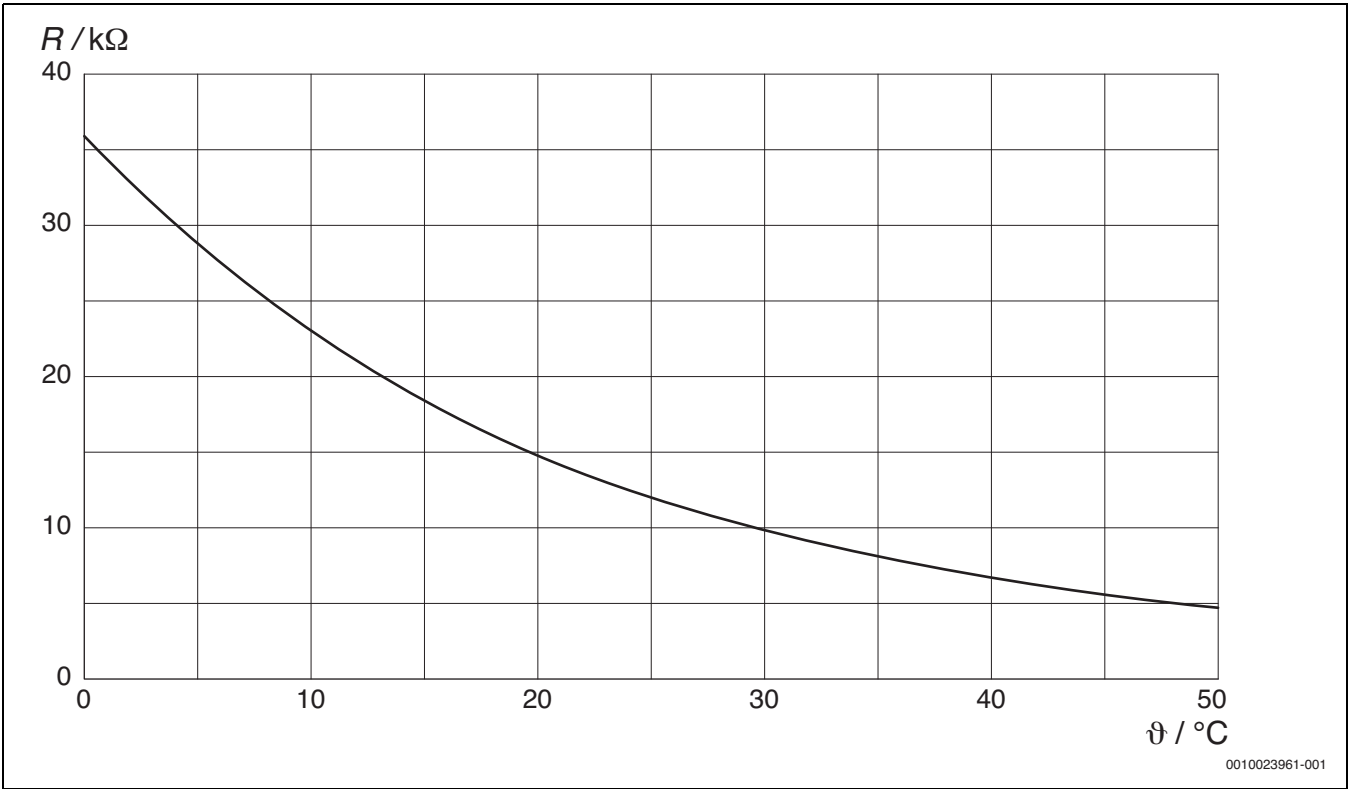
Bild 51 Widerstandskennlinie Temperaturfühler
