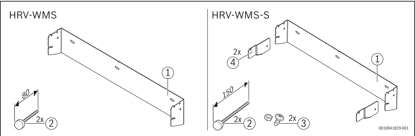
Bild 16 Lieferumfang HRV-WMS/HRV-WMS-S
