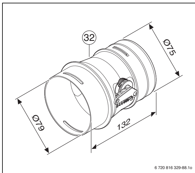
Bild 126 VKD-E (Maße in mm)
