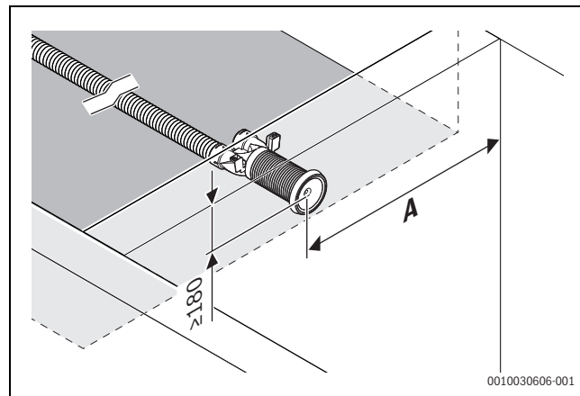
Bild 179 Mindestabstände bei Wandinstallation bei Verwendung von geradem Ventilanschluss RRU 75-5
