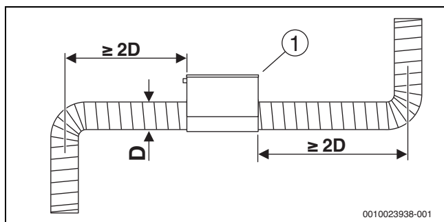
Bild 49 Abstand Heizregister – Bogen
