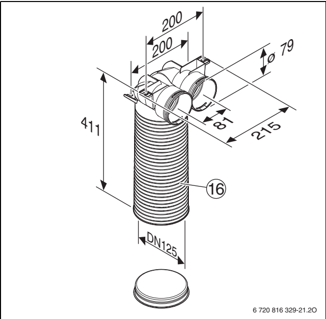
Bild 136 RRU 75-4 (Maße in mm)
