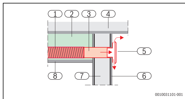
Bild 180 Einbaubeispiel Zuluftventil ZU 125
