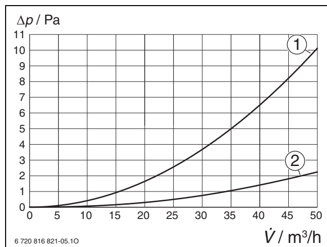
Bild 158 Druckverlust FKU 140-3 – Zuluft
