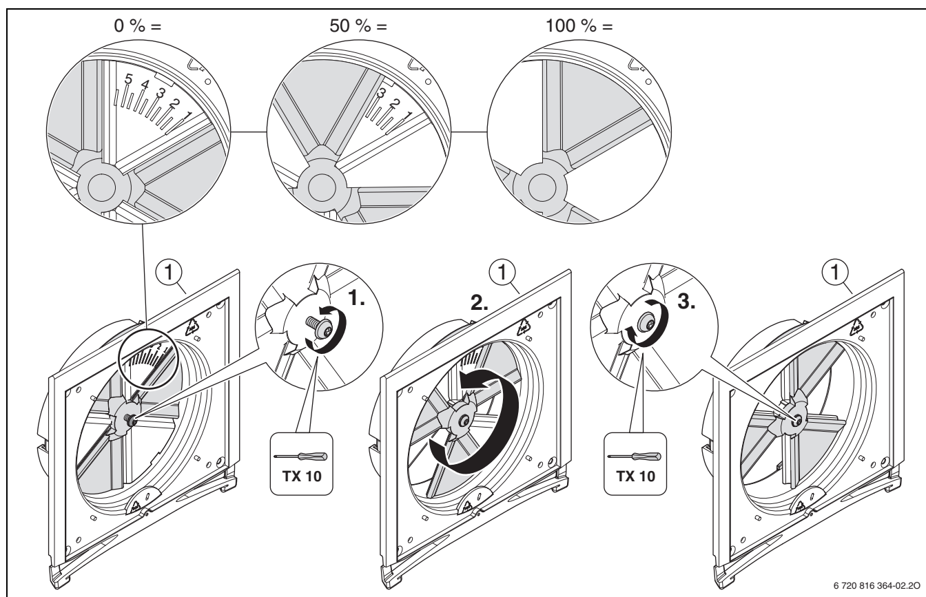
Bild 193 Einstellen der Drosselblende
