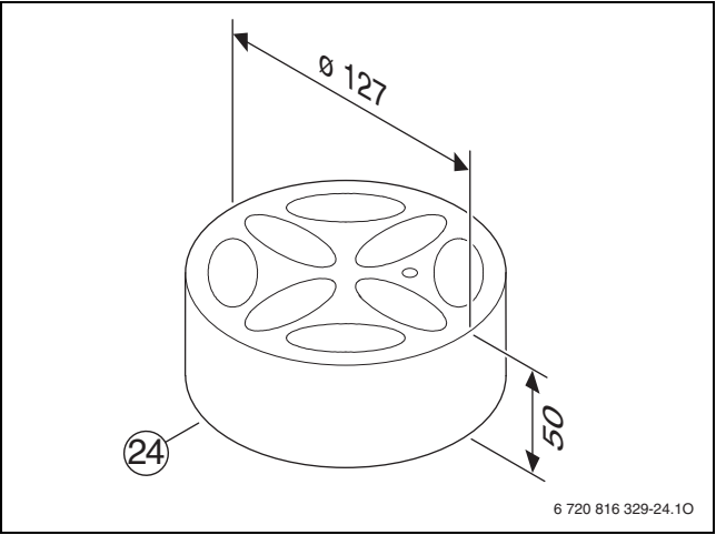
Bild 189 SDE (Maße in mm)
