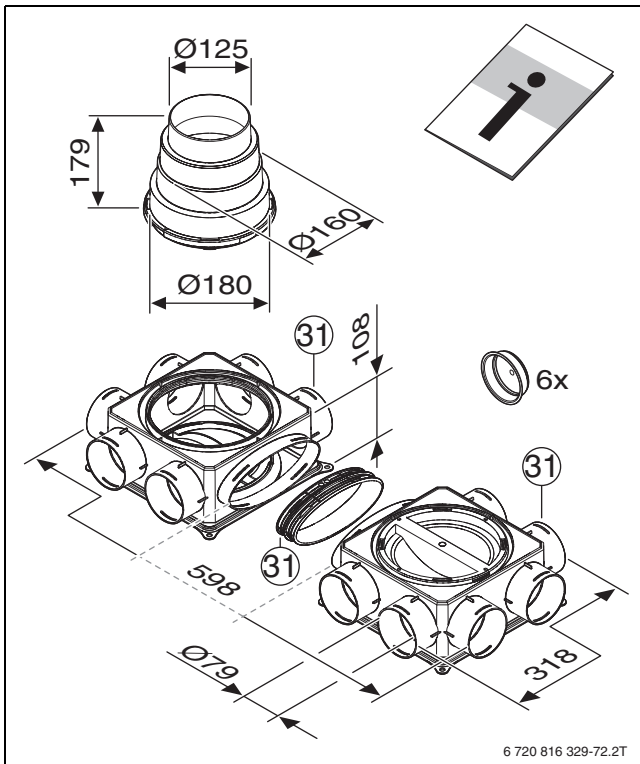
Bild 112 VK 125-2H (Maße in mm)
