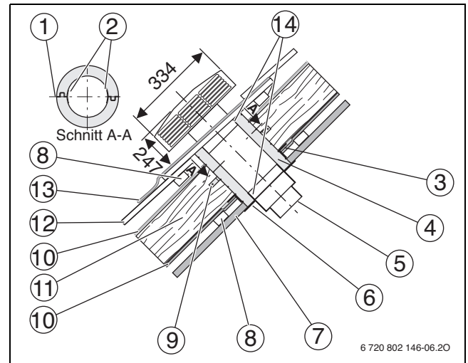
Bild 81 Schnitt Skizze Einbau Dachdurchführung DDF 160/1 (Maße in mm)
