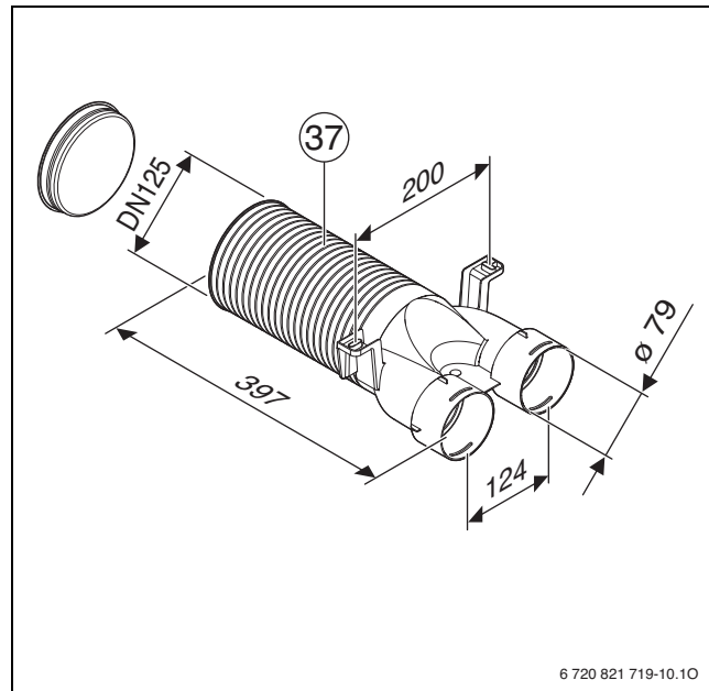
Bild 140 RRU 75-5 (Maße in mm)
