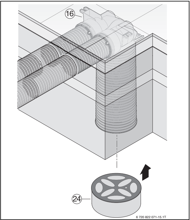
Bild 190 SDE – Anwendungsbeispiel
