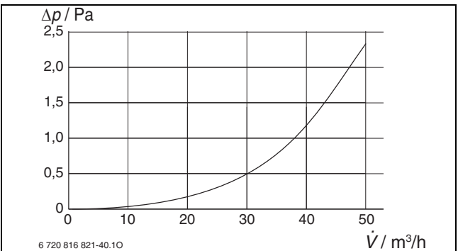
Bild 191 Druckverlust SDE
