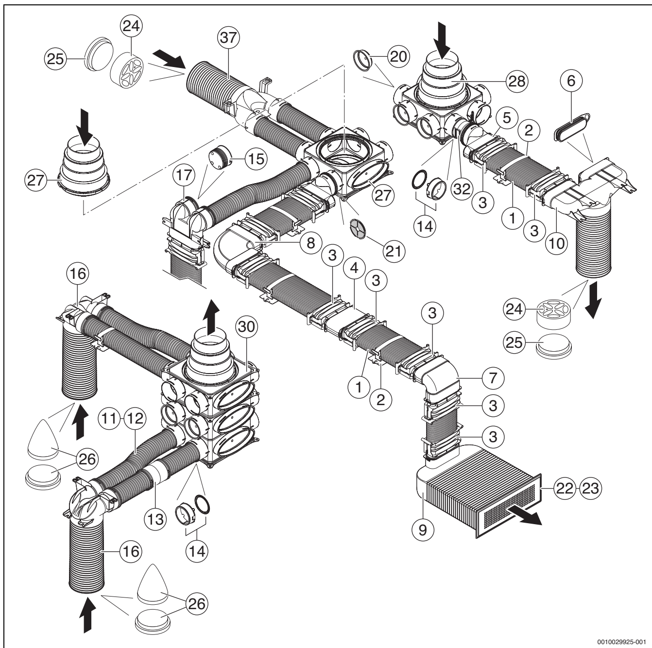
Bild 102 Luftverteiler mit VK 125-1, VK 125-1-8 und VK 125-3V, beispielhafte Luftkanalführung
