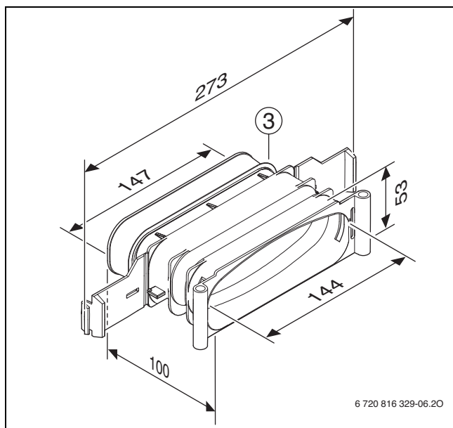
Bild 162 FKV 140-3 (Maße in mm)
