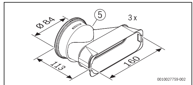
Bild 129 FKV 140-5 (Maße in mm)
