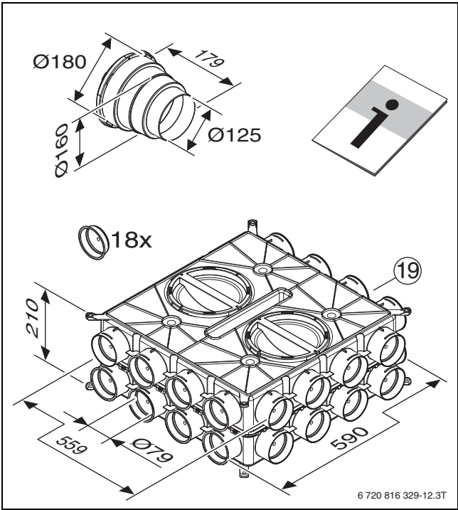
Bild 108 VK 160 (Maße in mm)
