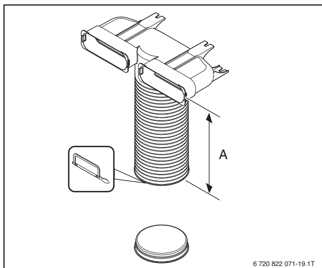
Bild 157 Kürzung Umlenkstück FKU 140-3 (Maße in mm)
