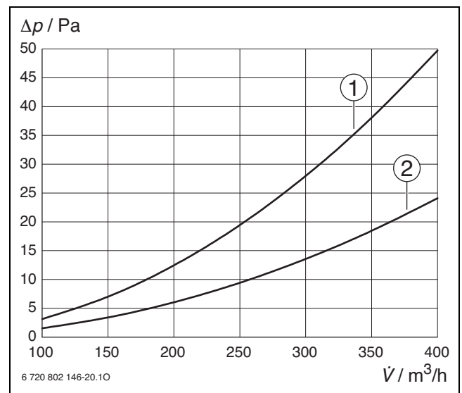
Bild 82 Druckverluste Dachdurchführung DDF 160/1 Anschluss DN 160
