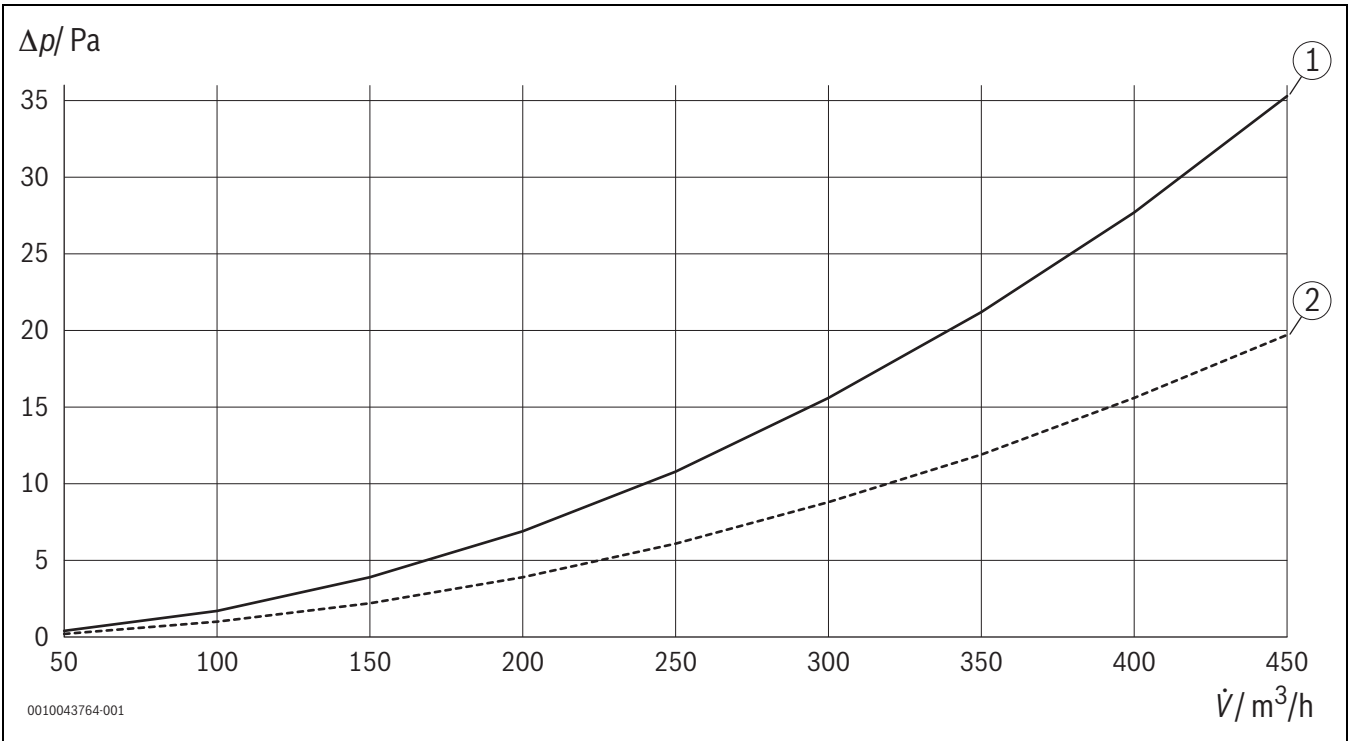
Bild 79 Druckverluste Dachdurchführung DDF-F 160
