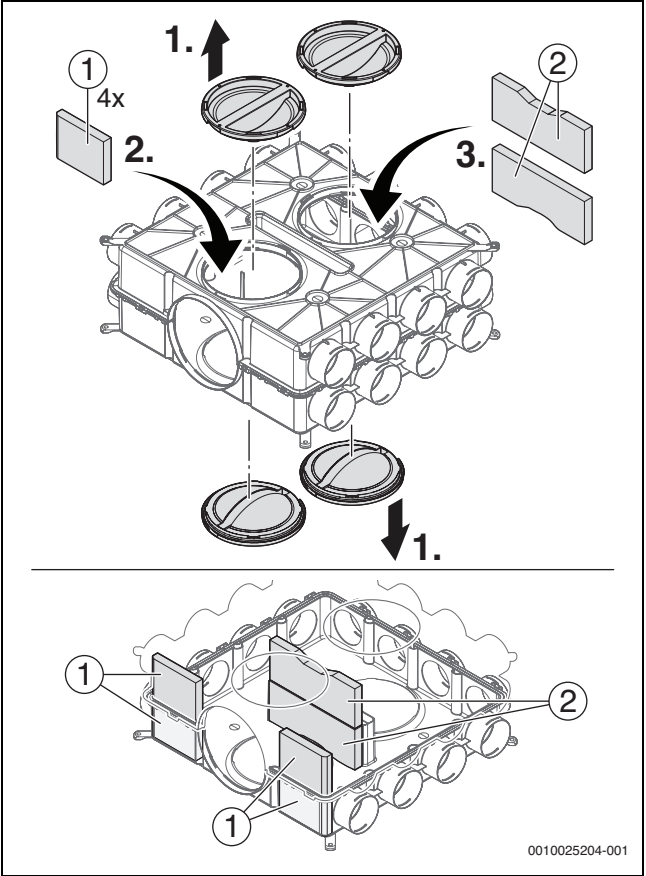
Bild 116 Montage Schalldämmset SDE VK 160
