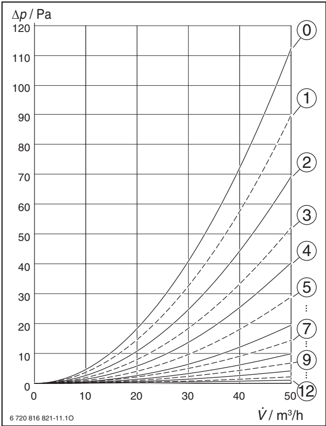
Bild 125 Druckverlust Volumenstrombegrenzer VKD
