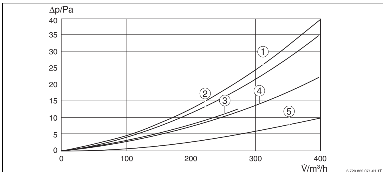
Bild 118 Druckverluste Luftverteilerkasten VK ... je Kasten (zusätzlicher Druckverlust nach Kanalart berücksichtigen → Bild 119)
