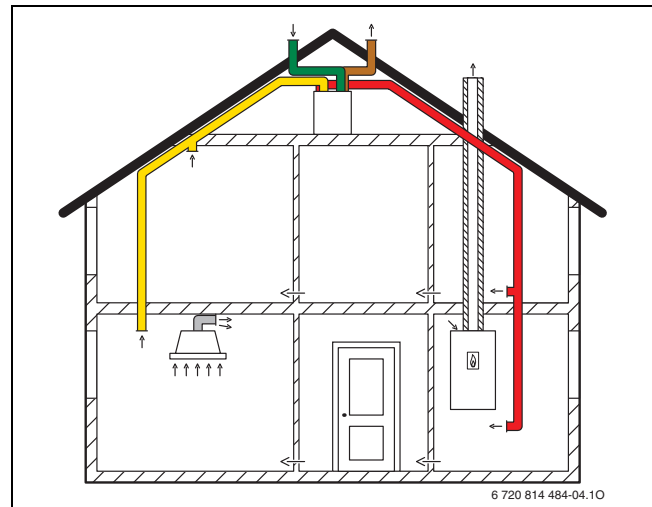
Bild 214 Vent 5000 C und raumluftabhängige Feuerstätte
