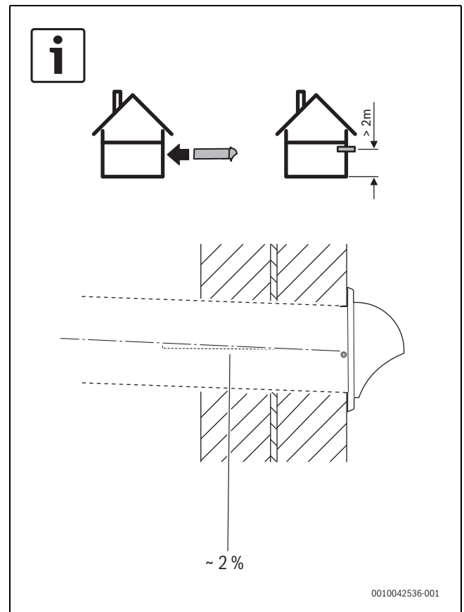
Bild 88 Einbausituation
