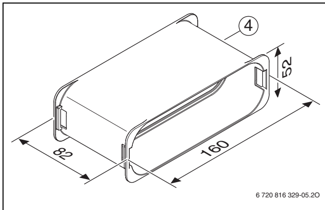
Bild 165 FKV 140-2 (Maße in mm)
