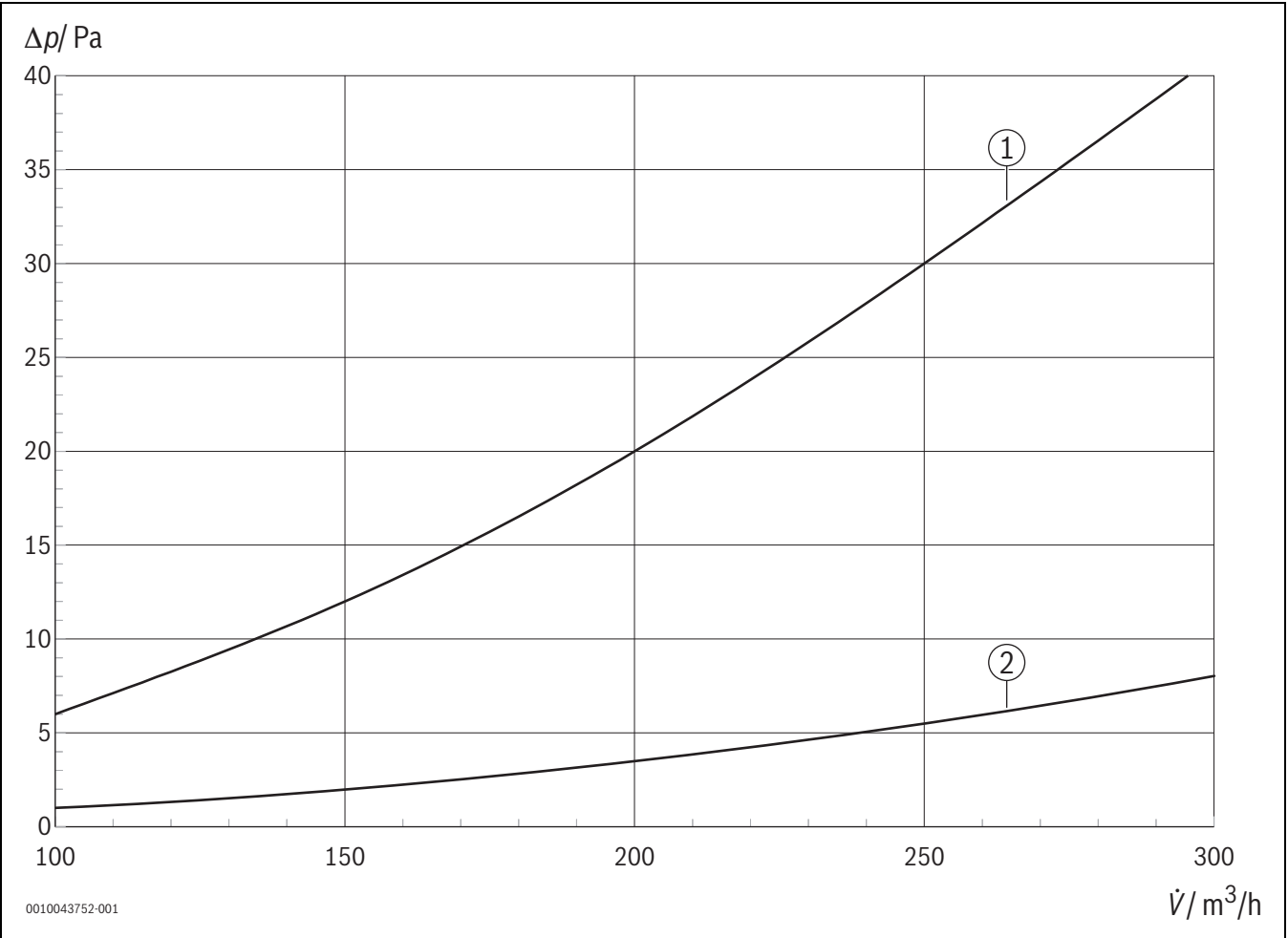
Bild 73 Druckverluste Außen- und Fortluftelement WGE 160-2
