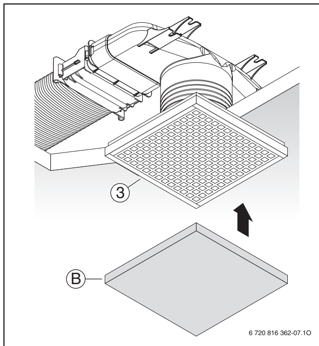
Bild 212 Blende
