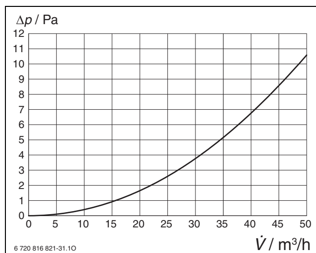
Bild 173 Druckverlust FKU 140-2 mit Luftgitter AG/...
