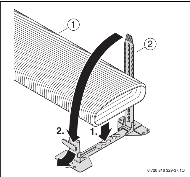
Bild 150 Flachkanal montieren
