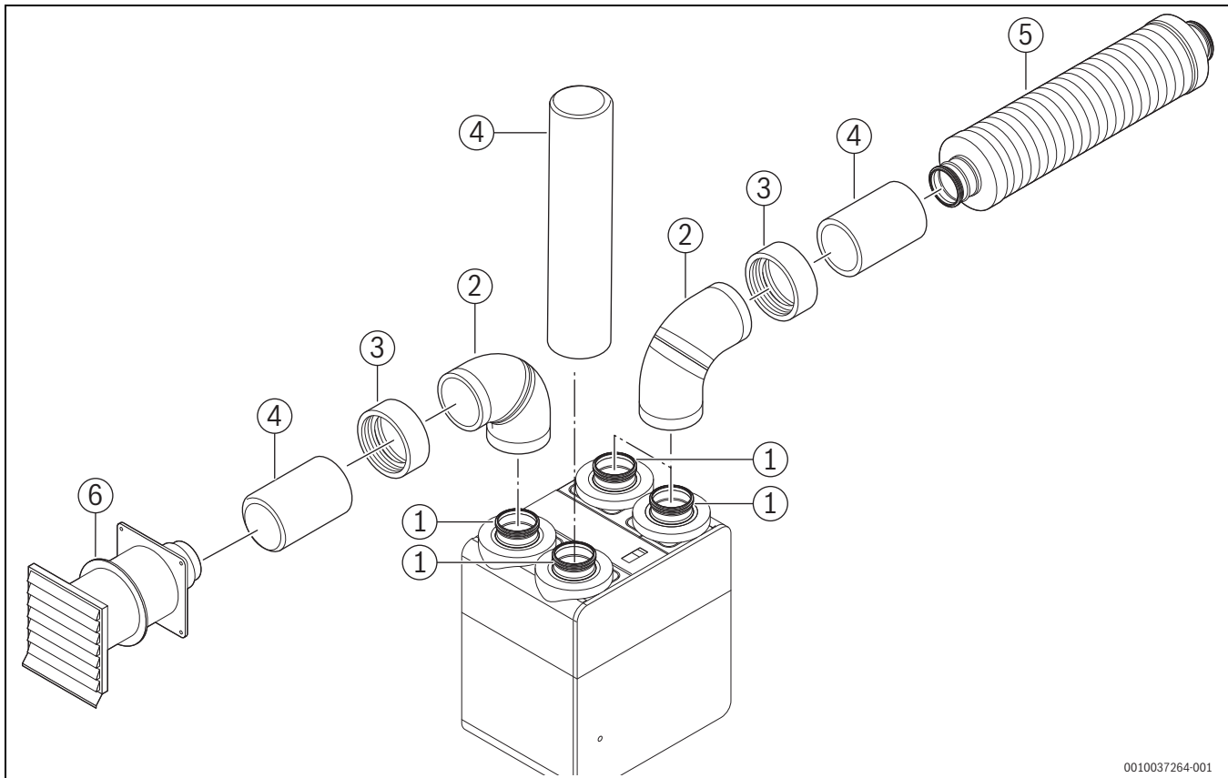
Bild 58 Anschluss Luftkanalsystem Variante 1
