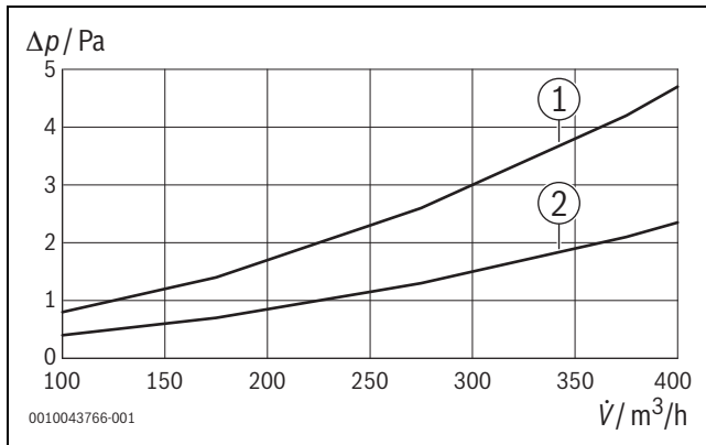
Bild 94 Druckverluste Schalldämpfung SDF...
