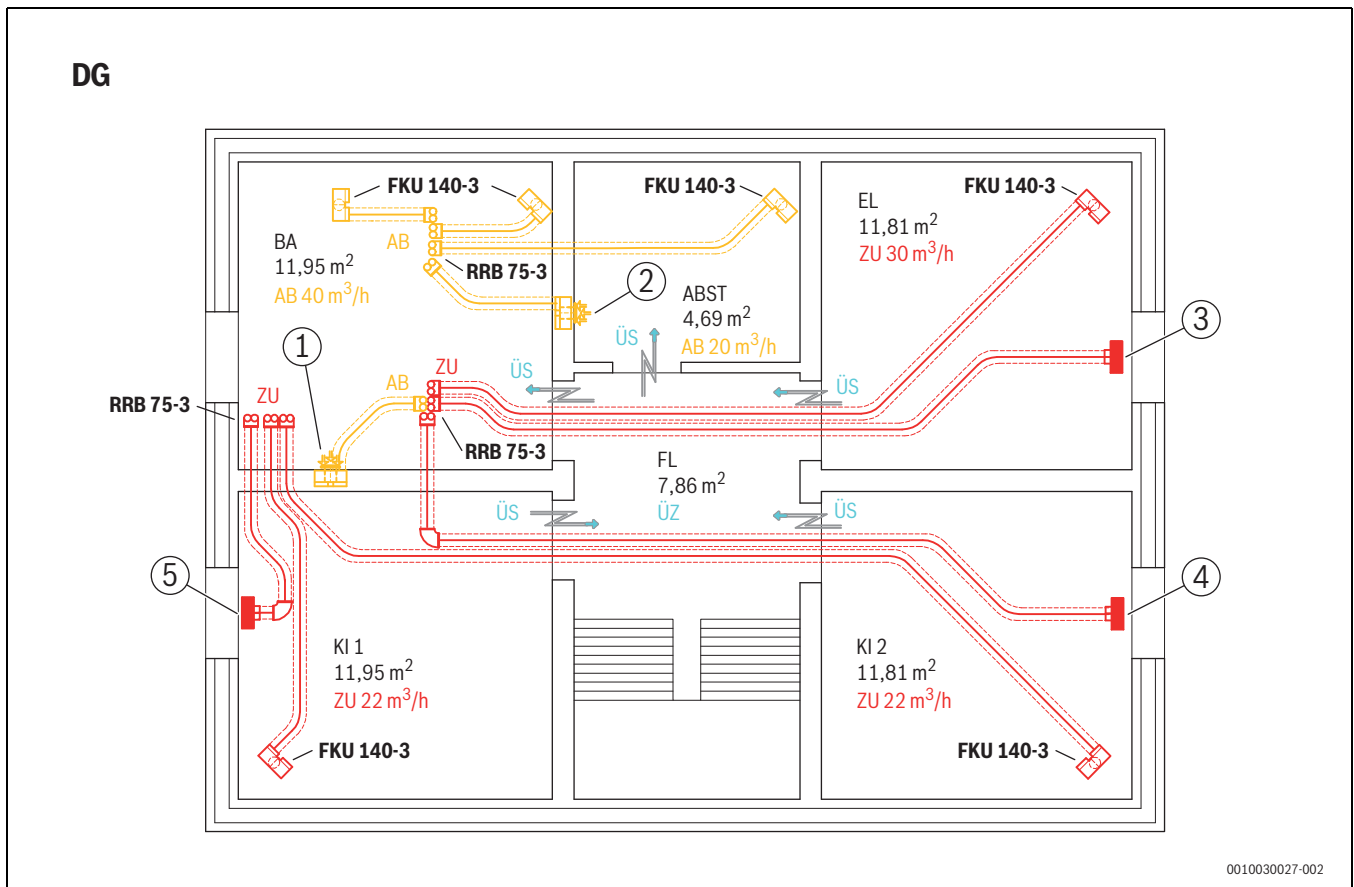
Bild 230 Grundriss Dachgeschoss mit Lüftungsinstallation
