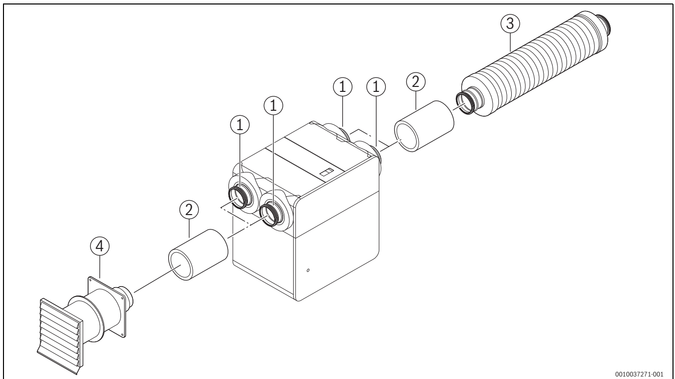
Bild 59 Anschluss Luftkanalsystem Variante 2
