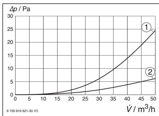
Bild 174 Druckverlust RRU 75-2 mit Luftgitter AG/...
