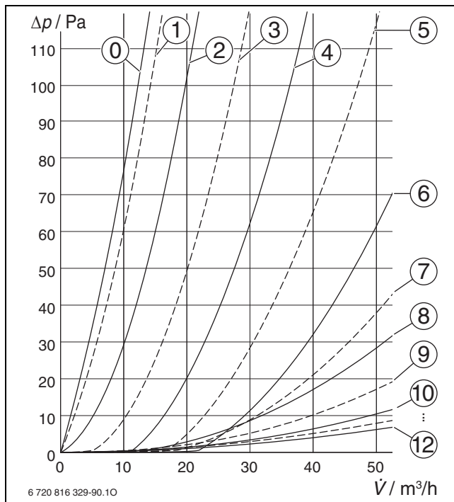
Bild 128 Druckverlust Volumenstromdrossel VKD-E
