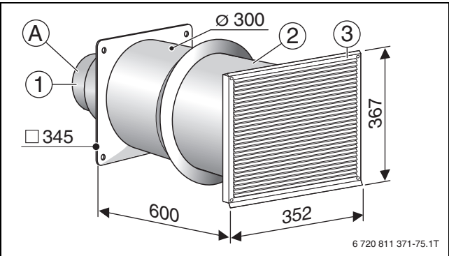
Bild 84 Abmessungen Wanddurchführung WGE 160-2 (Maße in mm)
