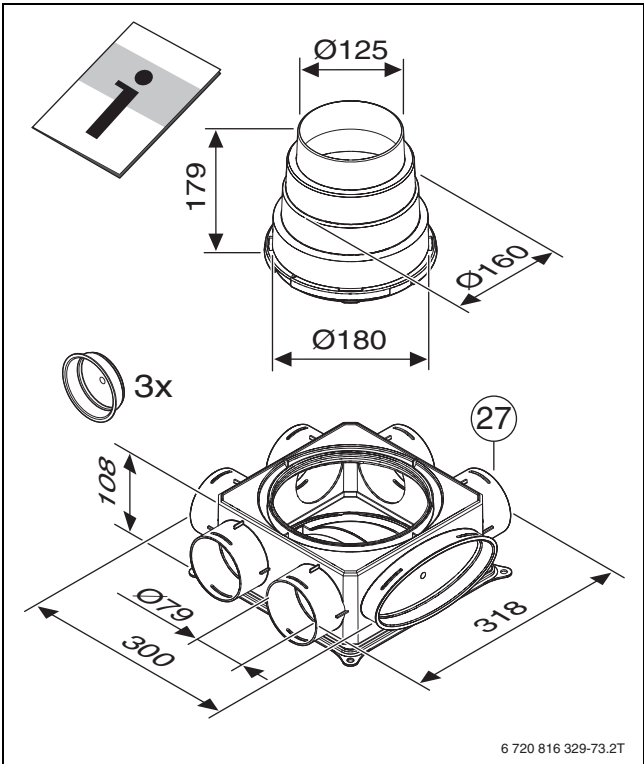
Bild 109 VK 125-1 (Maße in mm)
