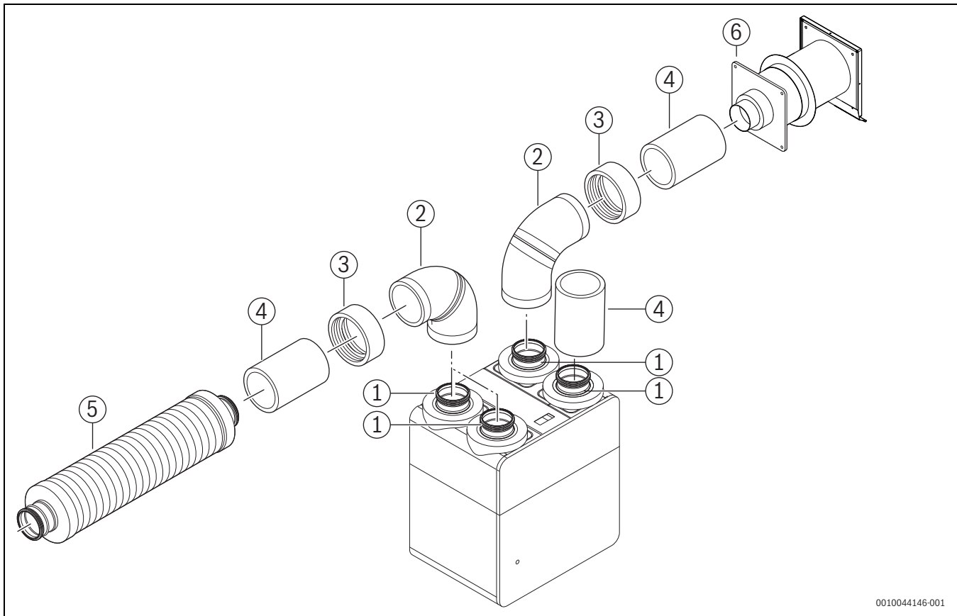
Bild 60 Anschluss Luftkanalsystem Variante 3
