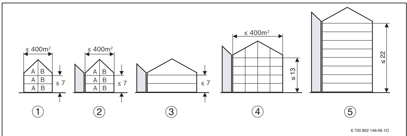
Bild 221 Gebäudeklassen (Maße in m)
