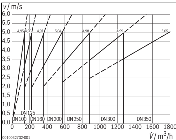
Bild 220 Überschlägige Auslegung von Luftleitungen in Abhängigkeit vom Luftvolumenstrom für Luftgeschwindigkeiten \leq 5 m/s
