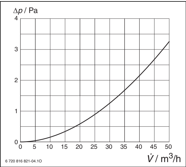
Bild 155 Druckverlust FKB 140-2
