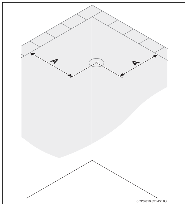
Bild 177 Mindestabstände bei Deckeninstallation
