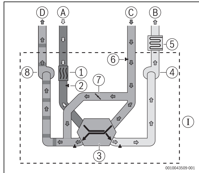
Bild 7 Funktionsprinzip
