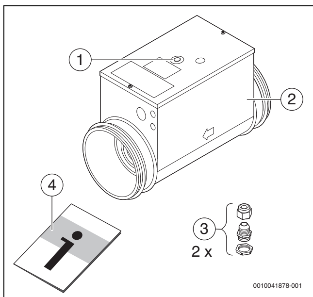
Bild 42 Lieferumfang zusätzliches Vorheizregister HRE 160-1200
