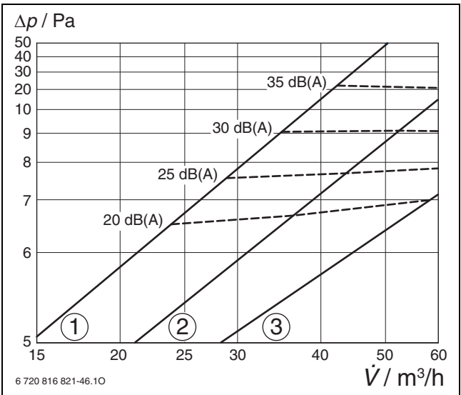
Bild 197 Strömungsgeräusche bei verschiedenen Volumenströmen – Zuluft
