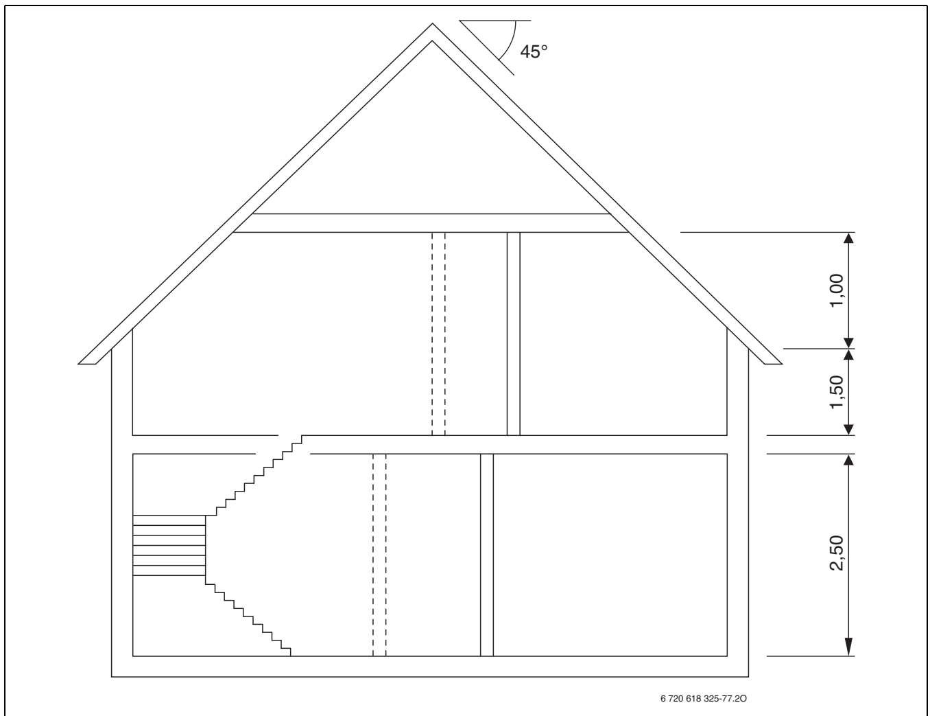
Bild 227 Beispielauslegung - Schnitt (Maße in m)
