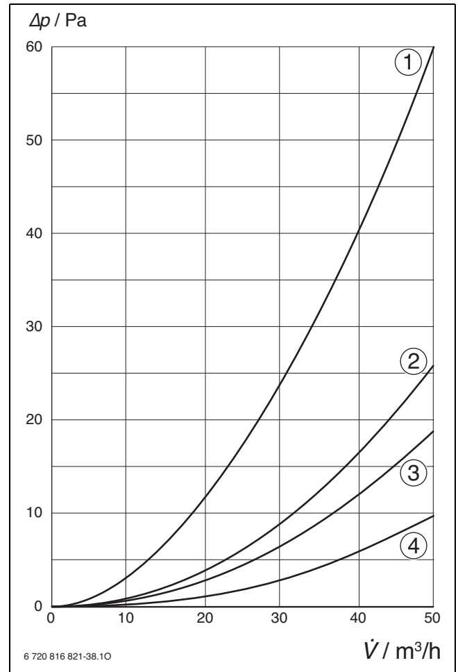
Bild 211 Druckverlust AV 125/K
