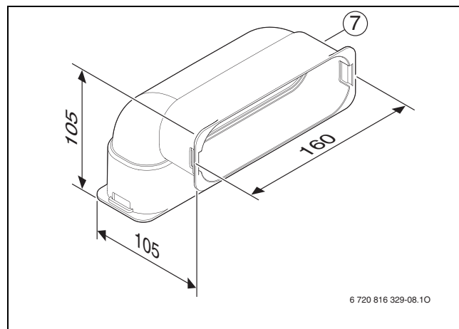
Bild 152 FKB 140-1 (Maße in mm)
