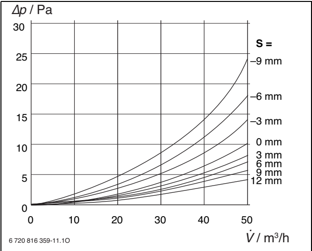
Bild 183 Druckverlust ZU 125
