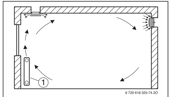
Bild 218 Luftführung im Raum
