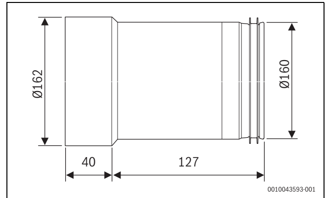
Bild 63 Maße
