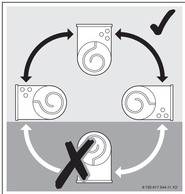
Bild 48 Einbaulagen Heizregister
