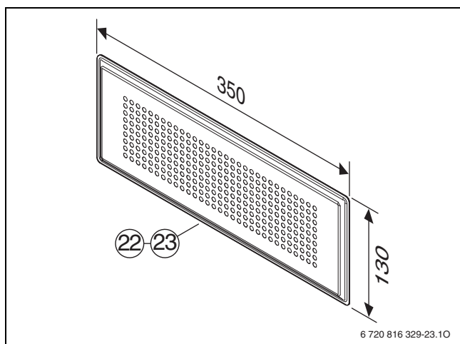
Bild 172 AG/W, AG/E (Maße in mm)
