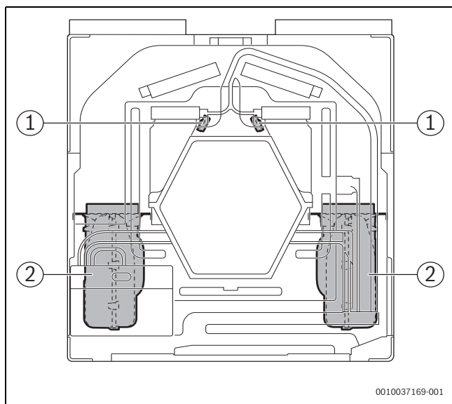
Bild 32 Position der Fühler im Gerät
