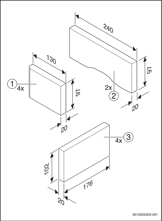
Bild 115 Lieferumfang und Abmessungen Schalldämmset SDE VK 160 (Maße in mm)
