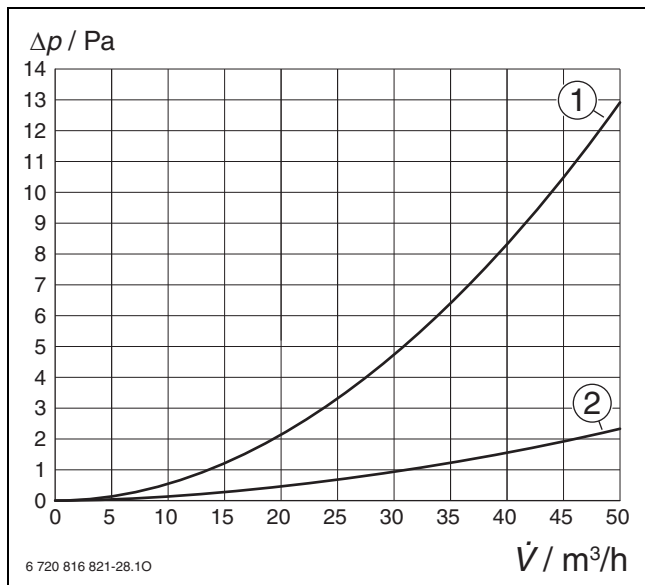
Bild 138 Druckverlust RRU 75-4 – Zuluft
