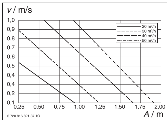
Bild 196 Wurfweite bei verschiedenen Volumenströmen
