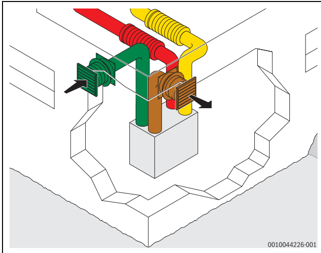
Bild 53 Hauptleitungen
