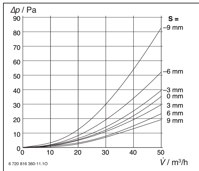
Bild 187 Druckverlust AV 125
