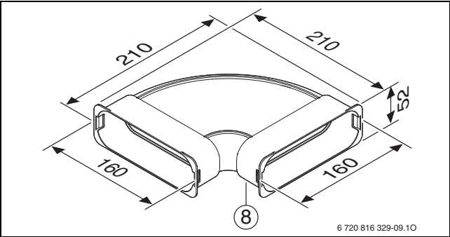
Bild 154 FKB 140-2 (Maße in mm)
