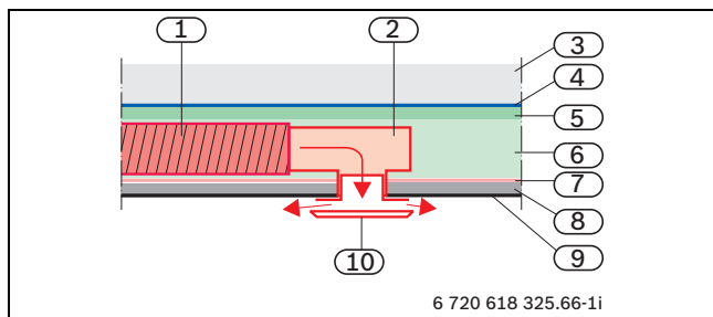
Bild 178 Einbaubeispiel Zuluftventil ZU 125
