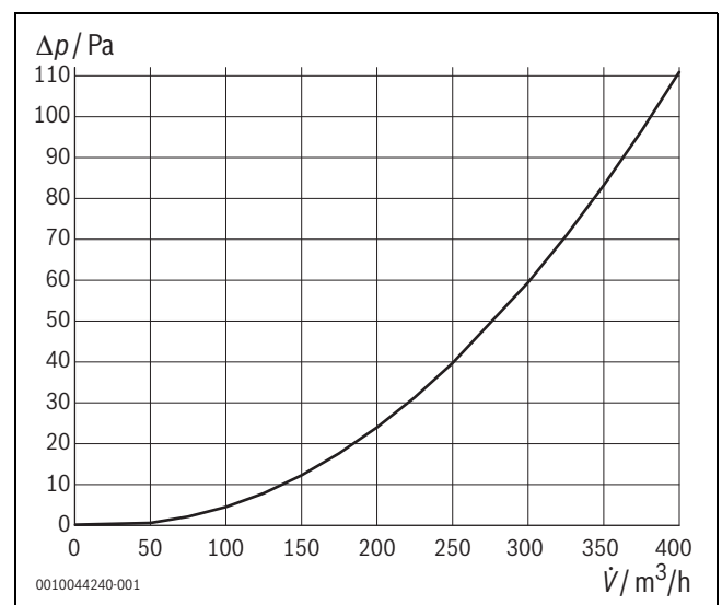
Bild 89 Druckverlust Kugelauslass WGK 160
