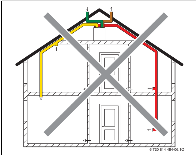
Bild 216 Vent 5000 C im Mehrfamilienhaus
