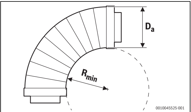
Bild 93 Kleinsten Biegeradius Schalldämpfer SDF...
