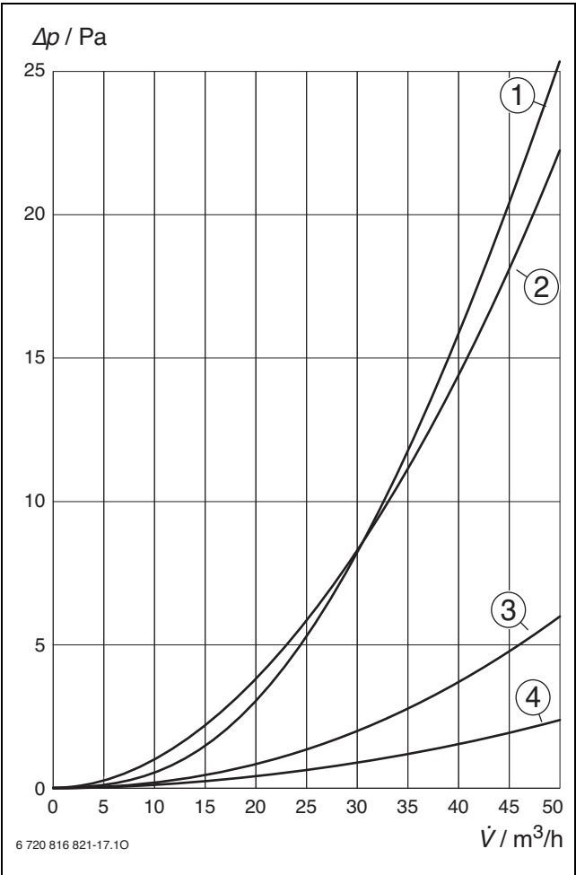
Bild 161 Druckverlust Verbinder 90° RRB 75-3
