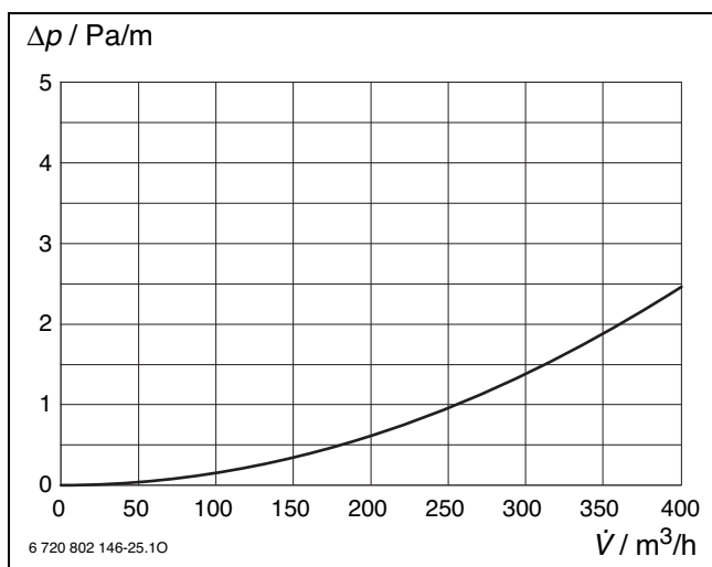
Bild 69 Druckverlust DEPP 160-3
