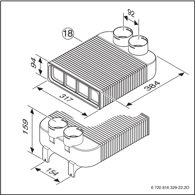
Bild 170 RRU 75-2 (Maße in mm)
