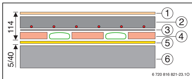
Bild 96 Flachkanal auf Rohbetondecke (Maße in mm)
