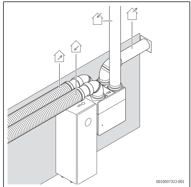
Bild 57 Variante 3: Geräteanschlüsse senkrecht - Luftführung Variante A
