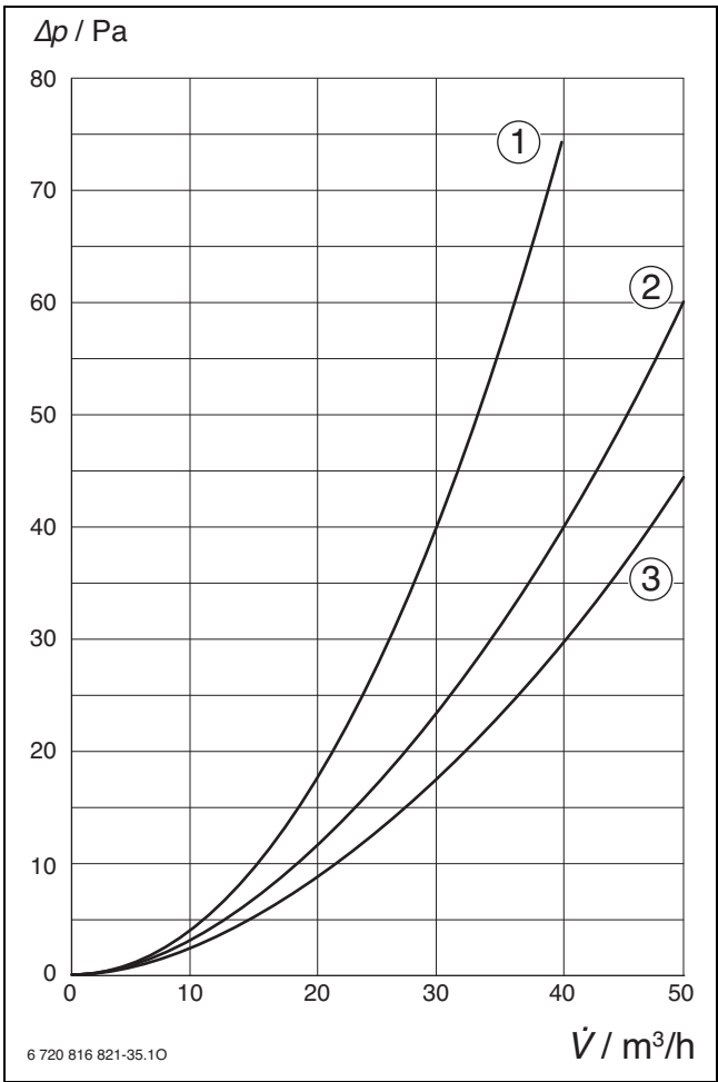
Bild 208 Druckverlust
