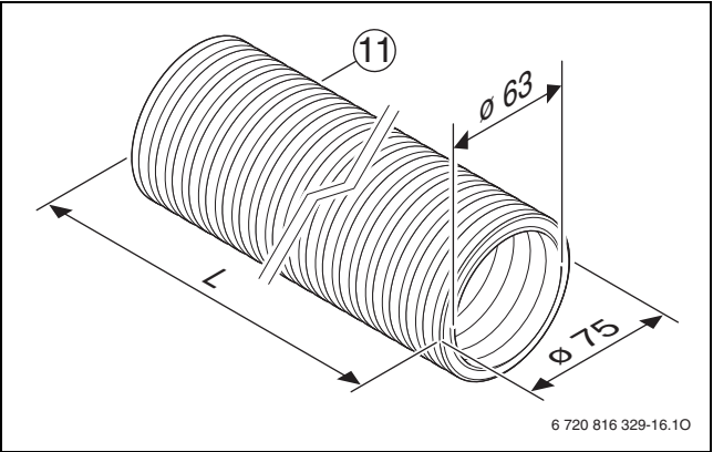
Bild 131 RR 75-1/2 (Maße in mm)
