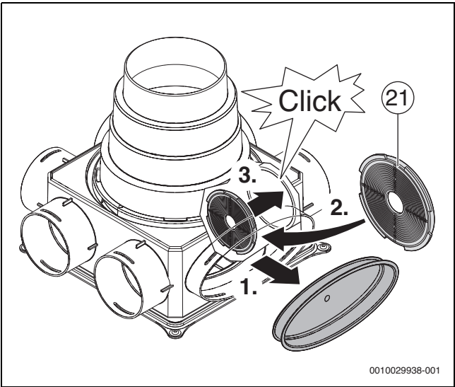
Bild 124 VKD + VK 125-1/VK 125-2V/VK 125-3V
