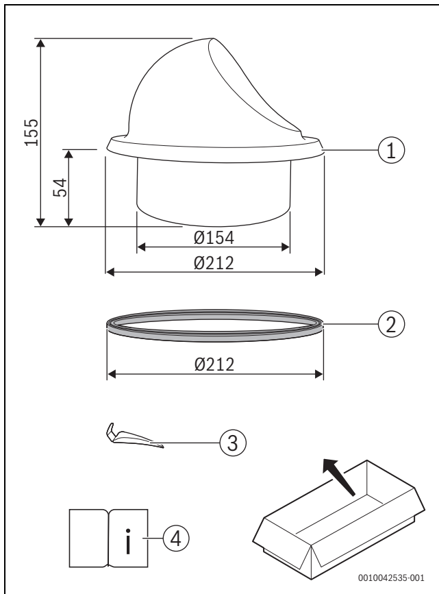
Bild 87 Lieferumfang WGK 160
