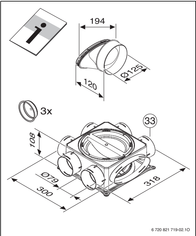
Bild 111 VK 125-1S (Maße in mm)
