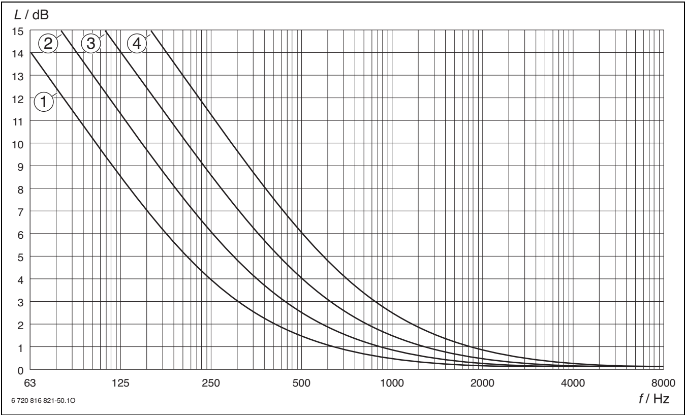
Bild 194 Pegelsenkung am offenen Kanalende nach VDI 2081
