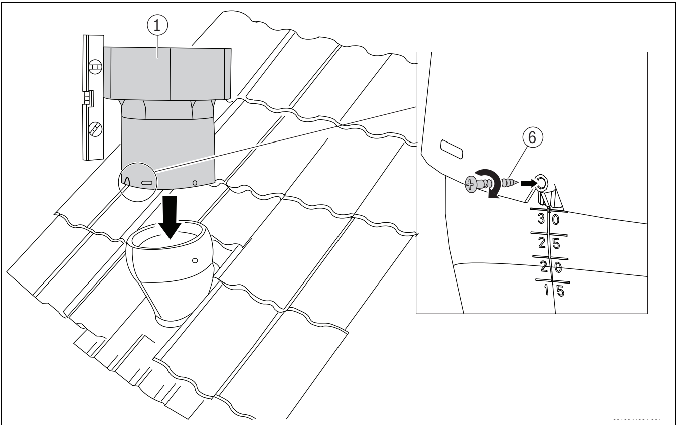
Bild 75 Montage DDF-S 160
