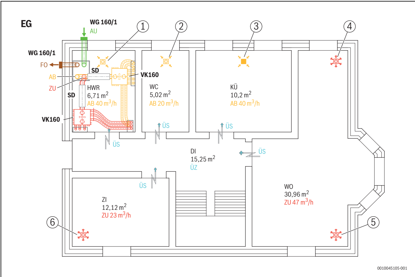
Bild 229 Grundriss Erdgeschoss mit Lüftungsinstallation
