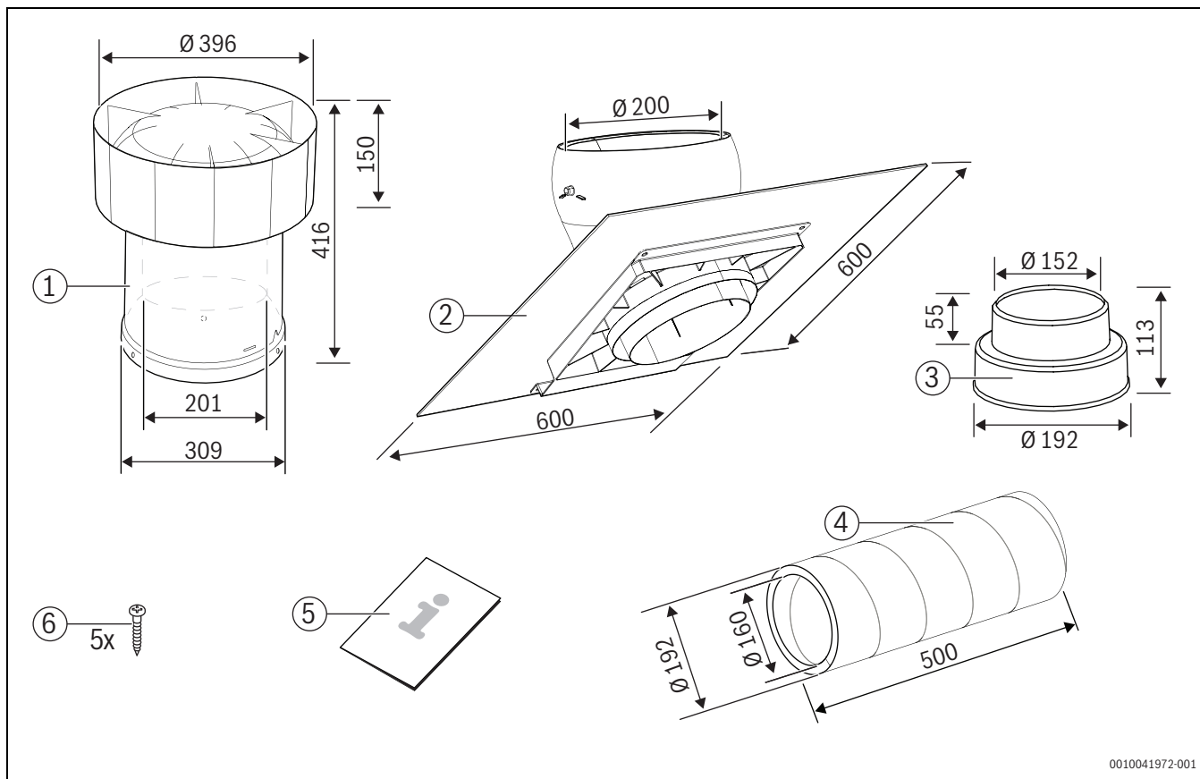
Bild 74 Lieferumfang und Maße DDF-S 160
