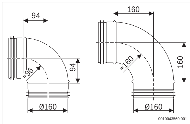
Bild 61 Maße
