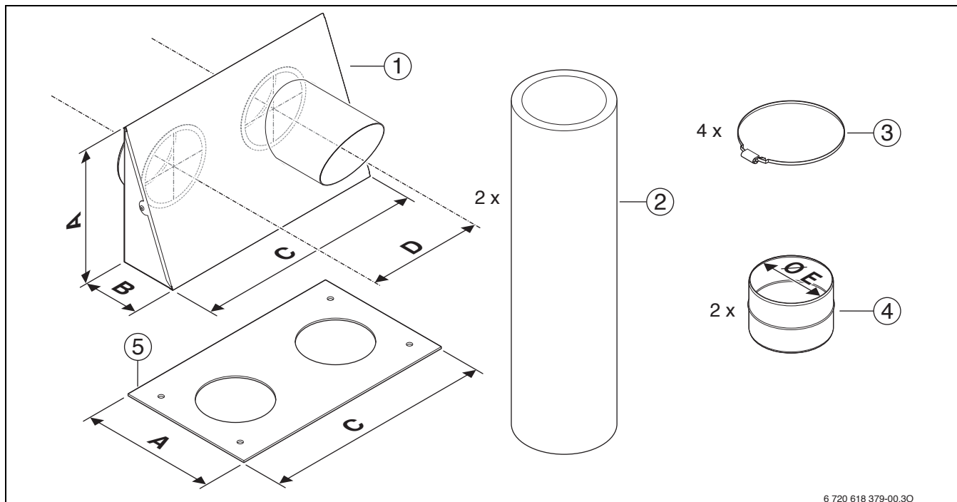
Bild 72 Abmessungen Außen- und Fortluftelement WGE 160-2
