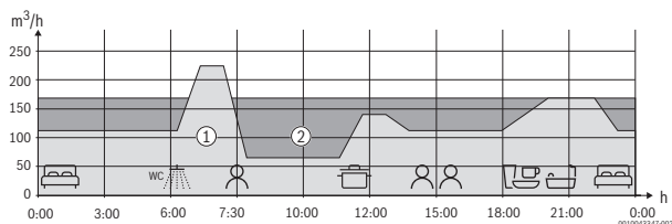
Bild 10 Beispielhafter Vergleich der bedarfsgeregelten/ manuellen Lüftung
