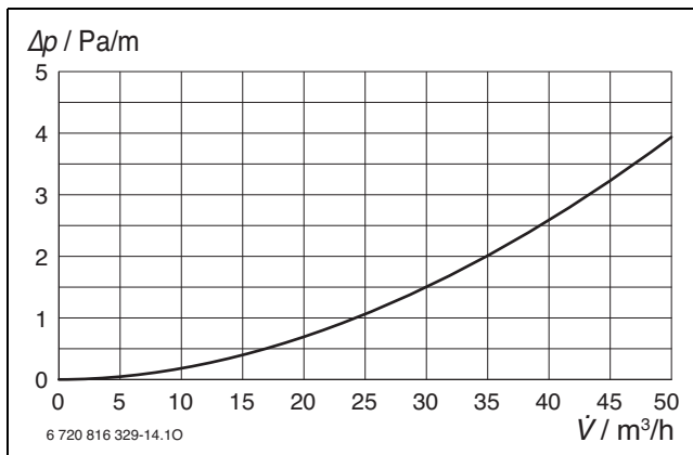
Bild 134 zusätzlicher Druckverlust pro 90°-Bogen Rundkanal RR 75-1/2 – gebogen mit Radius 150 mm
