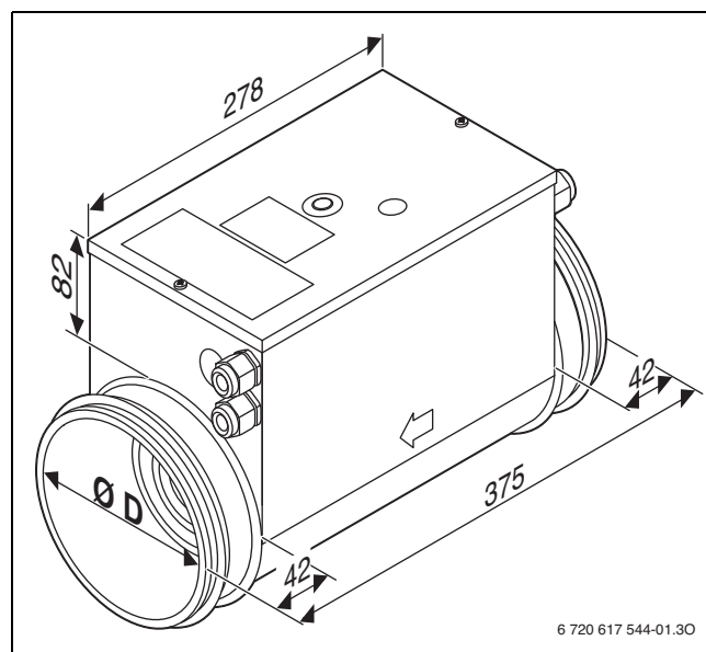
Bild 50 Einbaumaße der Heizregister (Maße in mm)
