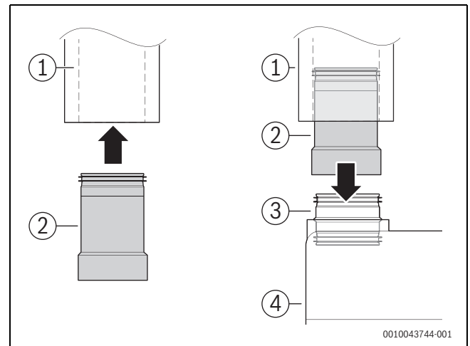
Bild 64 Montage
