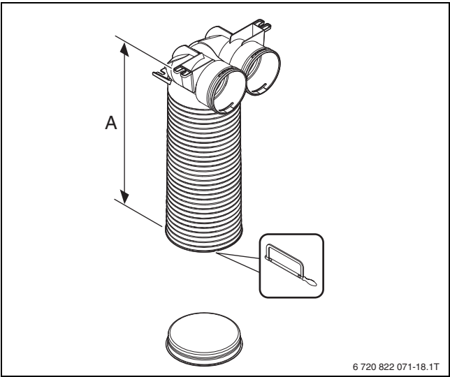
Bild 137 Kürzung Umlenkstück RRU 75-4
