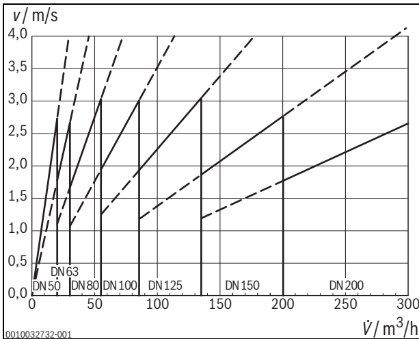
Bild 219 Überschlägige Auslegung von Luftleitungen in Abhängigkeit vom Luftvolumenstrom für Luftgeschwindigkeiten \leq 3 m/s
