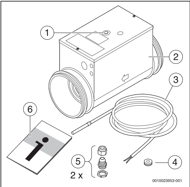
Bild 44 Lieferumfang Nachheizregister HRE-A 160-1200
