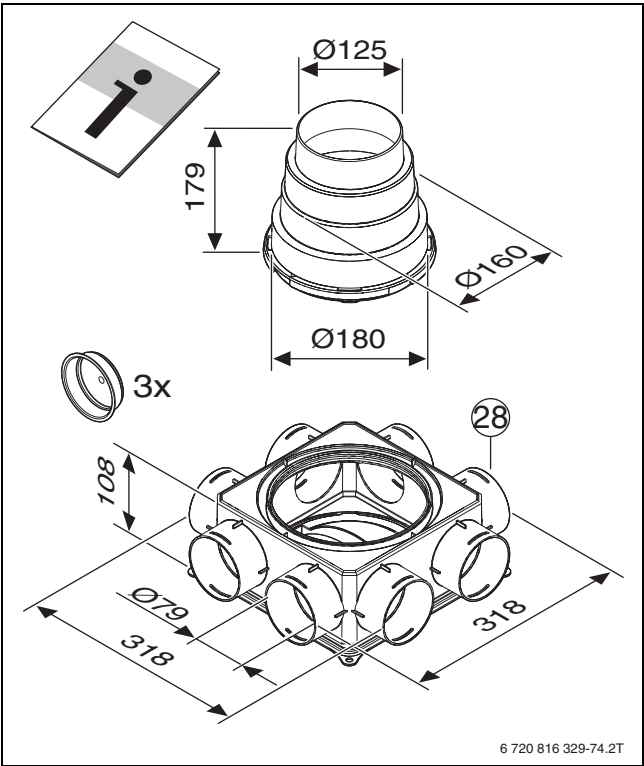
Bild 110 VK 125-1-8 (Maße in mm)
