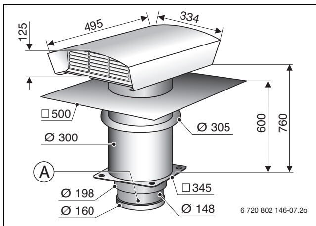
Bild 80 Abmessungen Dachdurchführung DDF 160/1 (Maße in mm)
