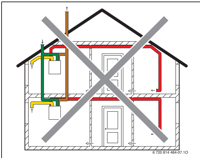
Bild 217 Vent 5000 C und Sammelleitungen für Fort-Außenluft
