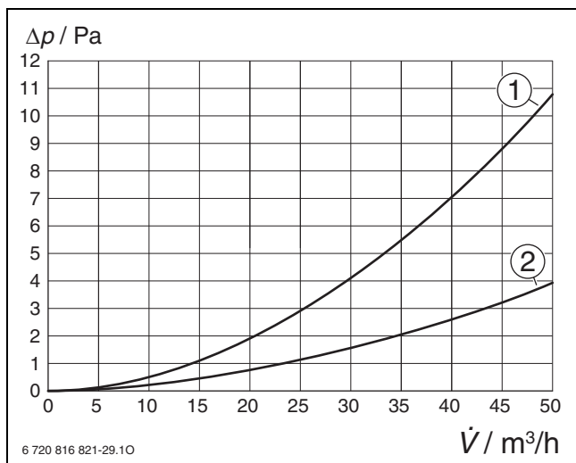
Bild 139 Druckverlust RRU 75-4 – Abluft
