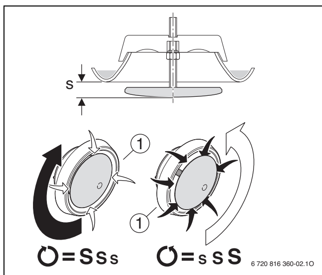
Bild 186 Luftmengen-Feineinstellung
