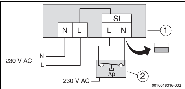
Bild 13 Anschluss Differenzdruckwächter an der Anschlussklemme SI
