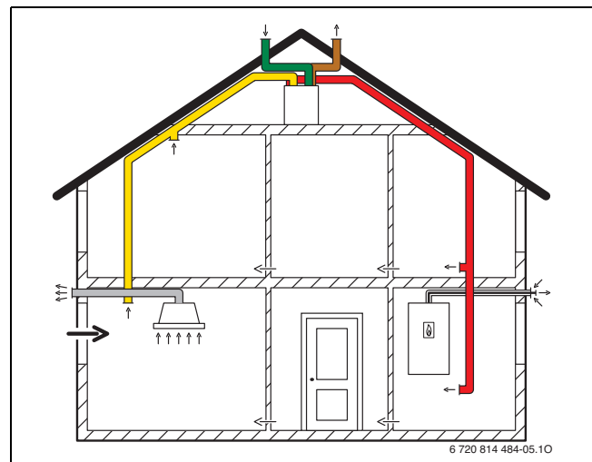
Bild 215 Vent 5000 C und Dunstabzugshaube im Abluftbetrieb
