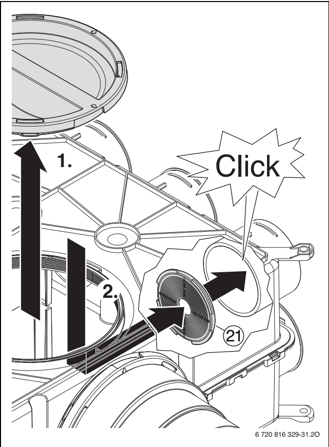
Bild 123 VKD + VK 160/VK 125...
