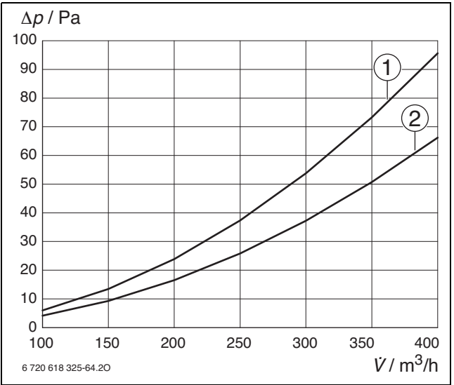
Bild 85 Druckverluste Wanddurchführung WG 160/1, mit Anschluss DN 160
