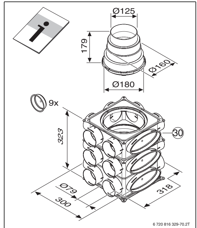
Bild 114 VK 125-3V (Maße in mm)
