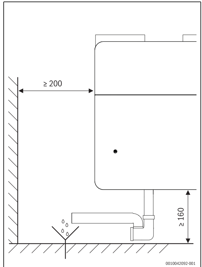
Bild 30 Mindestabstände V5001C mit Kugelsiphon HRV-BS
