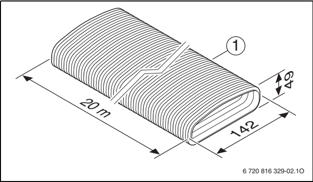
Bild 149 Flachkanal FK 140 (Maße in mm)
