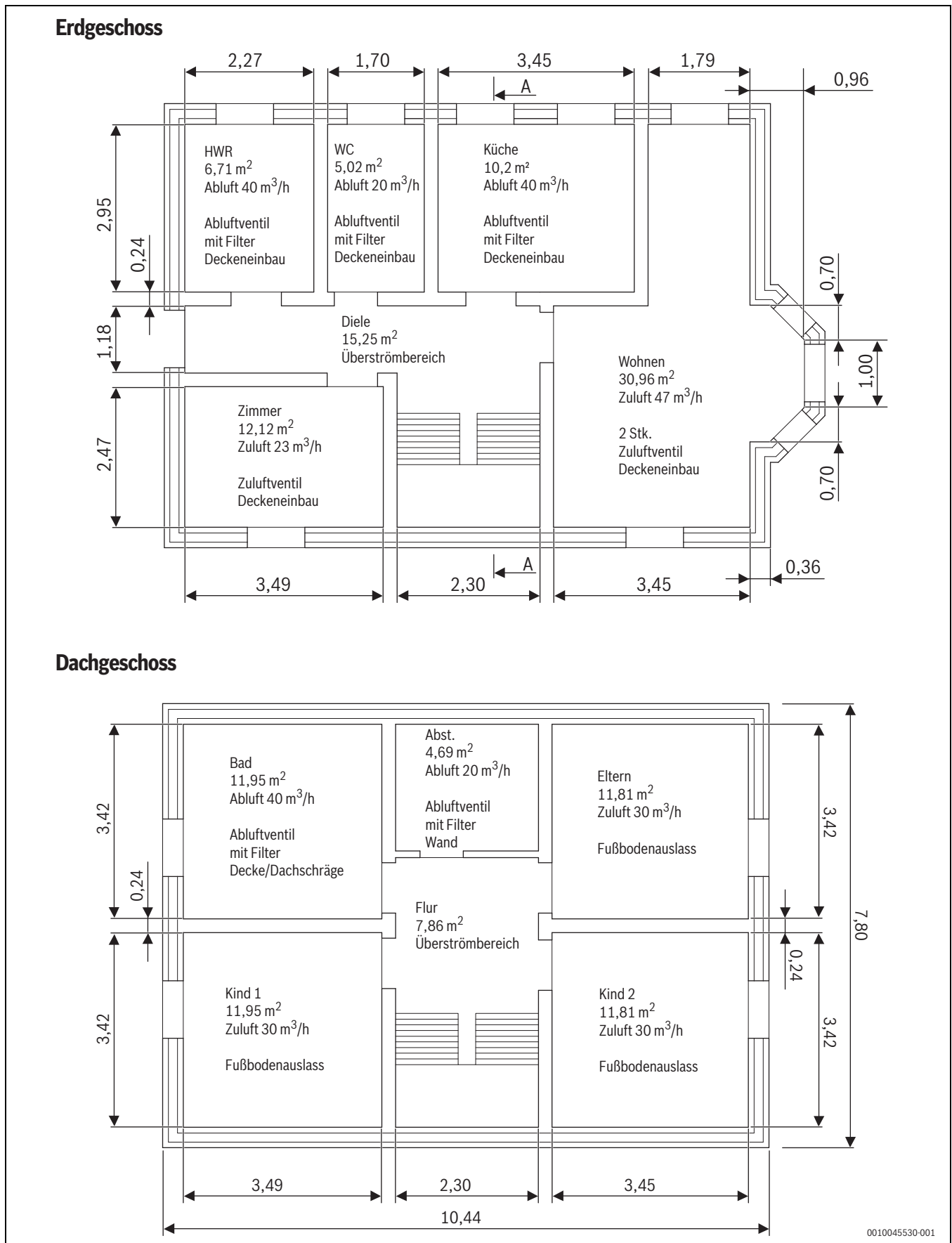
Bild 228 Grundriss (Maße in m)
