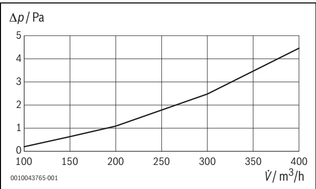
Bild 91 Druckverluste Schalldämpfung SD...
