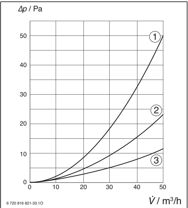
Bild 199 Druckverlust bei Verwendung als Zuluftventil
