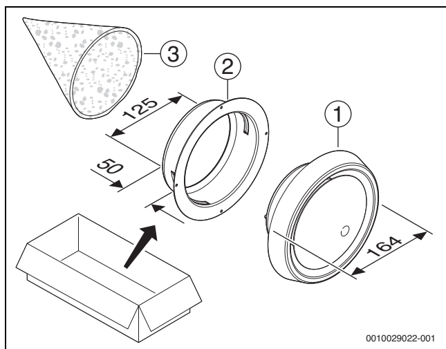
Bild 185 Lieferumfang AV 125 (Maße in mm)
