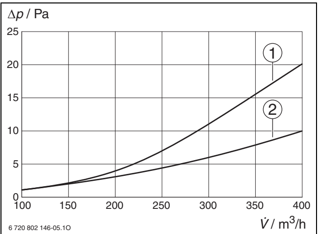
Bild 86 Druckverluste Wanddurchführung WGE 160-2, mit Anschluss DN 160
