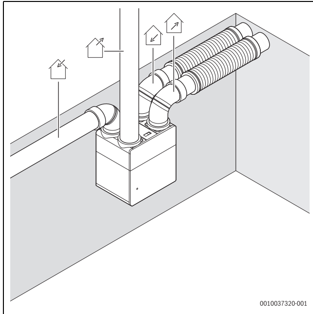
Bild 55 Variante 1: Geräteanschlüsse senkrecht - Luftführung Variante B
