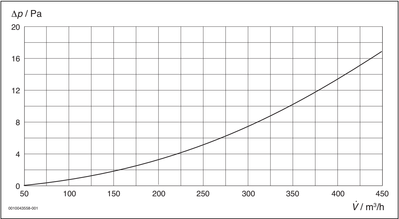
Bild 52 Kennlinie Druckverlust/Volumenstrom
