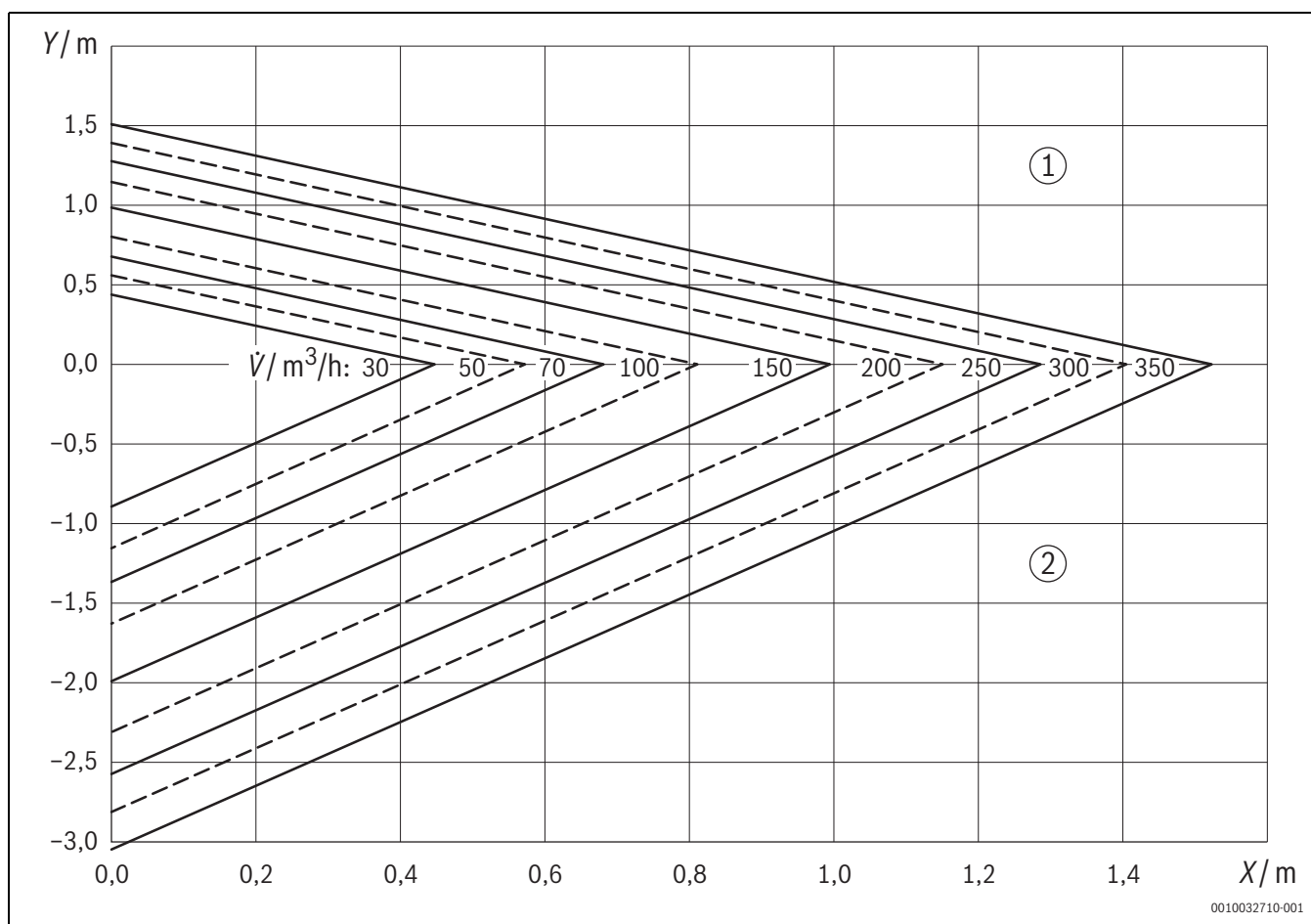
Bild 70 Mindestabstände AU-FO
