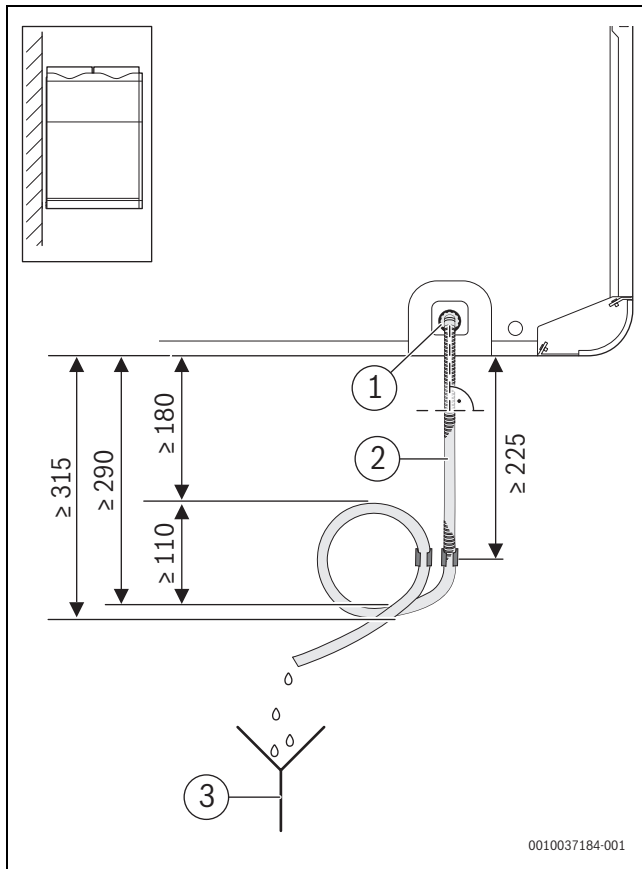
Bild 28 Siphon - Wandinstallation
