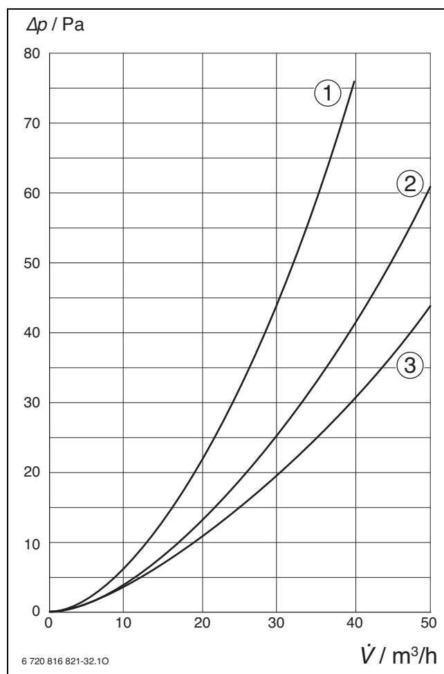
Bild 204 Druckverlust
