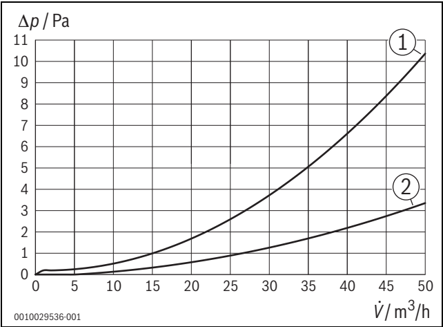
Bild 143 Druckverlust RRU 75-5 – Abluft
