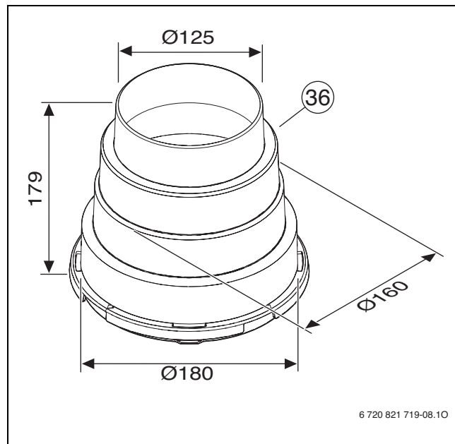
Bild 121 VKH (Maße in mm)
