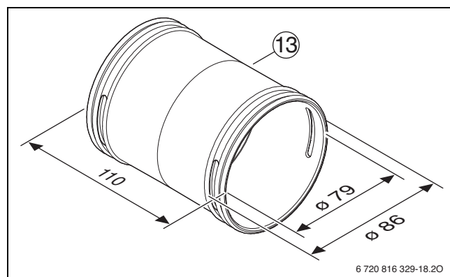
Bild 146 RRV 75-2 (Maße in mm)
