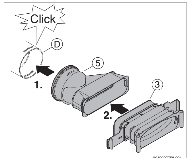
Bild 130 Verteilerkasten/VKD-E + FKV 140-5 + FKV 140-3
