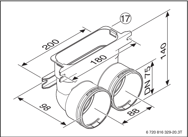
Bild 160 RRB 75-3 (Maße in mm)
