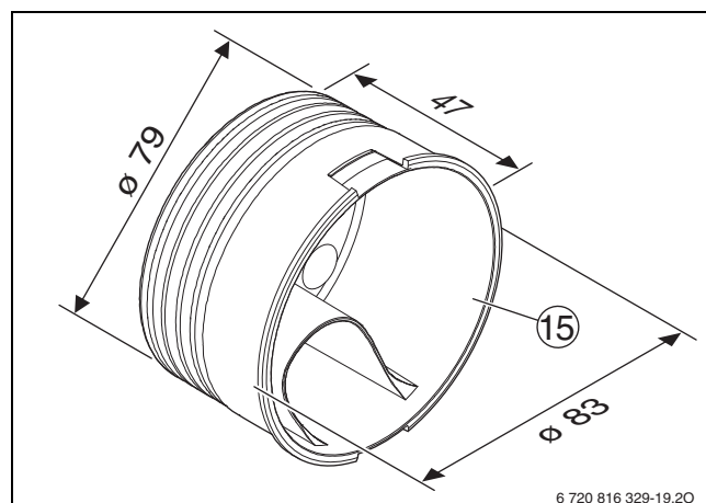
Bild 147 RRS 75 (Maße in mm)
