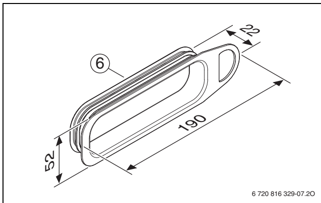
Bild 166 FKS 140 (Maße in mm)
