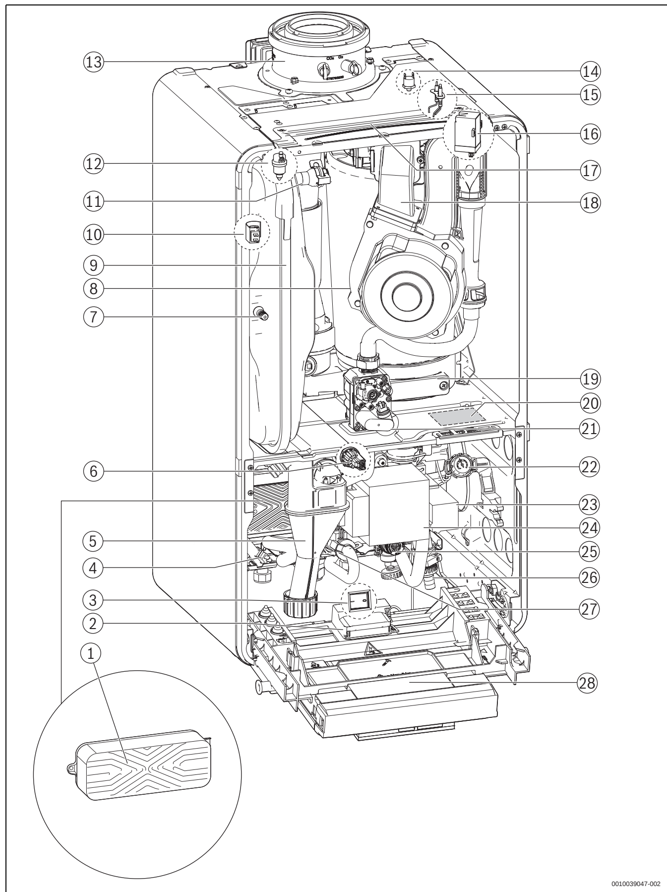
Bild 18 Produktübersicht Kombigerät
