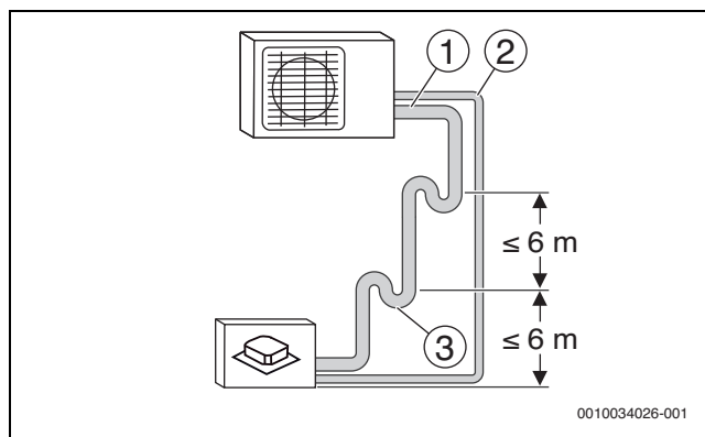
Bild 14 Höhenunterschied Installation Ölbogen
