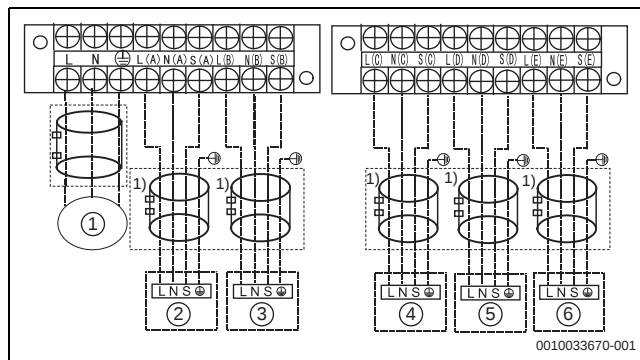
Bild 22 Verdrahtungsschema Außeneinheit mit 5 Inneneinheiten
