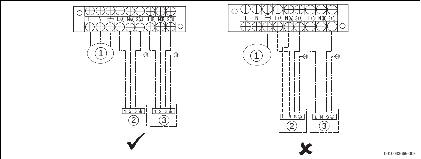
Bild 18 Verdrahtungsschema
