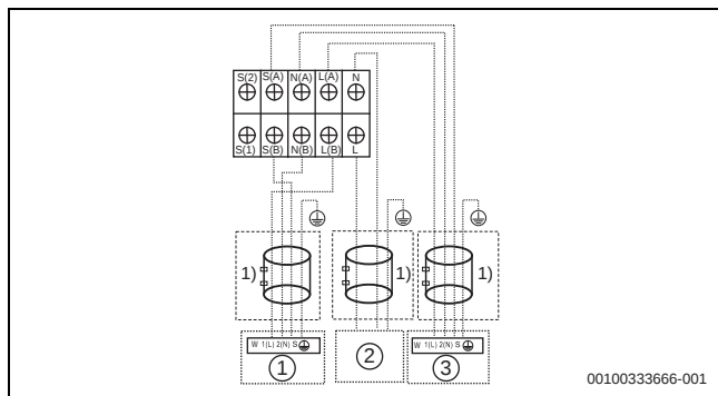
Bild 19 Verdrahtungsschema Außeneinheit mit 2 Inneneinheiten
