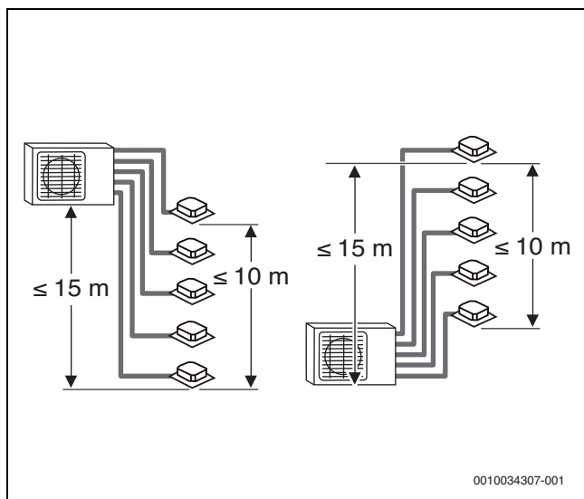
Bild 13 Maximale Höhen
