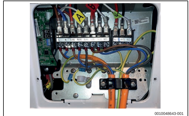
Bild 16 Elektrischer Anschluss
