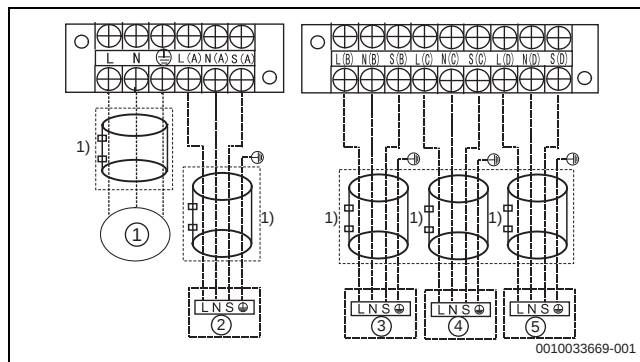
Bild 21 Verdrahtungsschema Außeneinheit mit 4 Inneneinheiten
