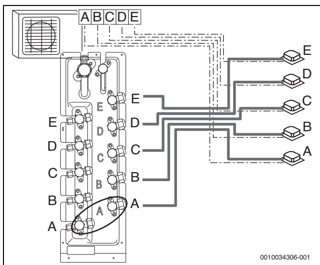
Bild 15 Übersicht Anschlussklemmen
