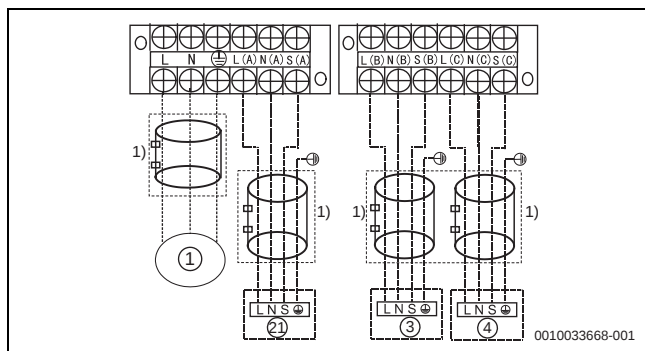
Bild 20 Verdrahtungsschema Außeneinheit mit 3 Inneneinheiten
