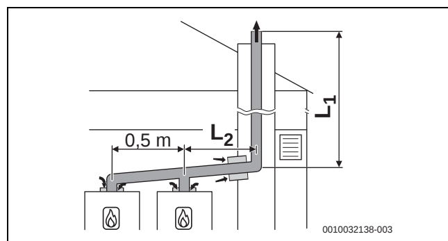
Bild 56 Kaskade mit 2 Geräten:
