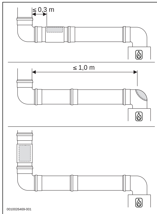
Bild 35 Anordnung der unteren Prüföffnung
