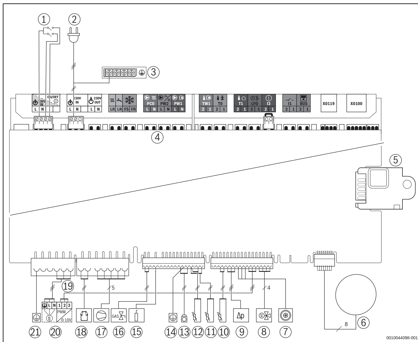
Bild 18 Elektrische Verdrahtung
