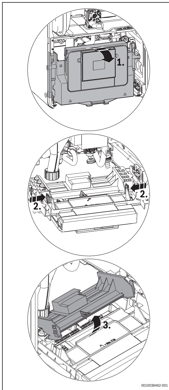
Bild 23 Abdeckung aufklappen
