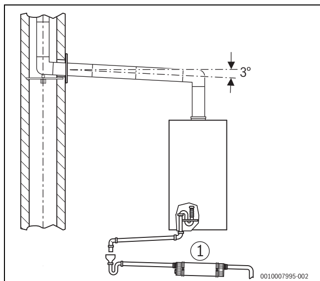
Bild 22 Kondensatschlauch aus dem Gas-Brennwertgerät und eine Kondensatableitung über die Neutralisationseinrichtung
