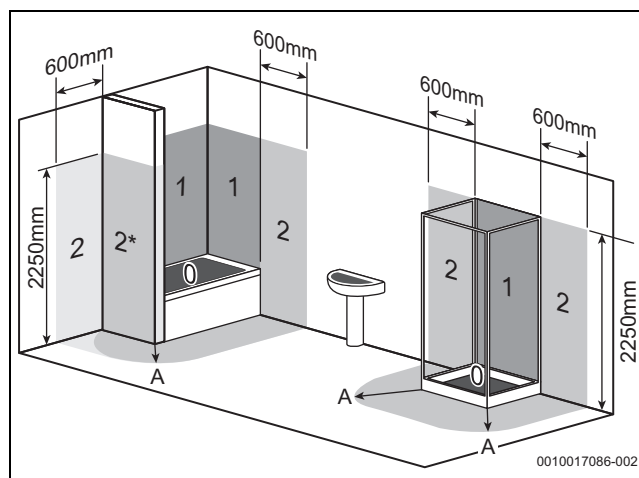
Bild 19 Schutzbereiche (Beispieldarstellung)
