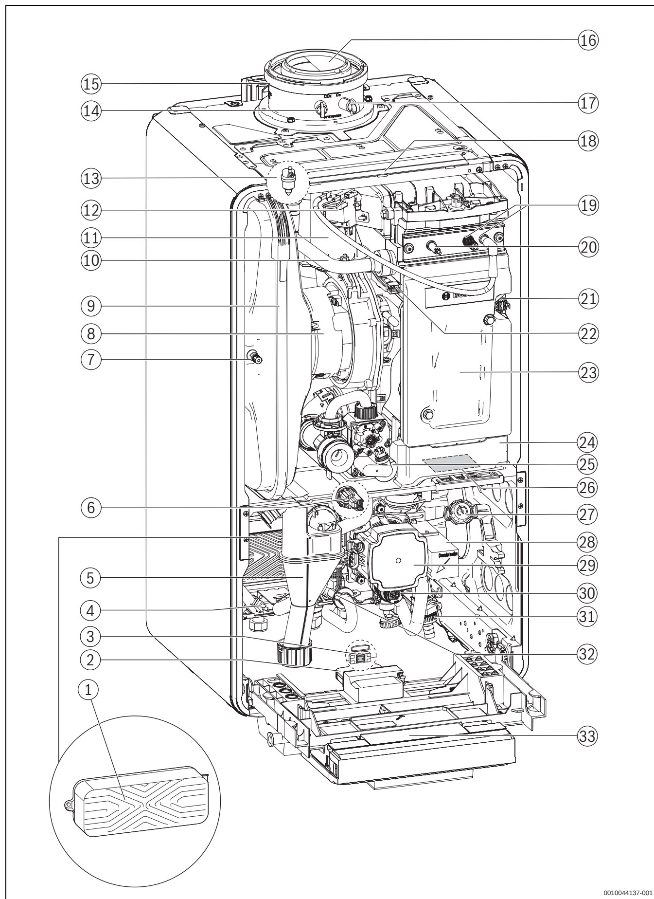
Bild 13 Produktübersicht Kombigerät
