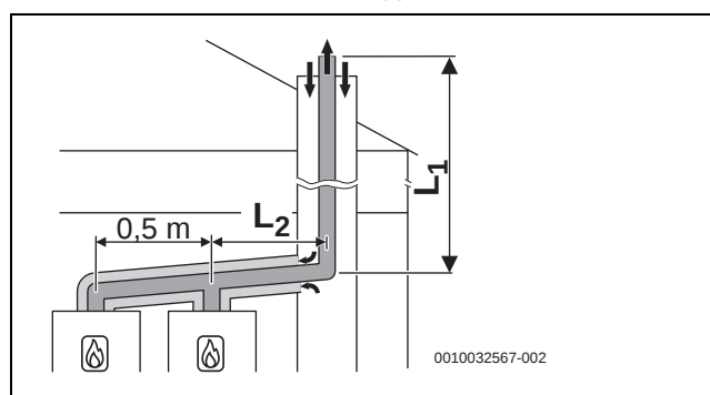
Bild 57 Kaskade mit 2 Geräten:
