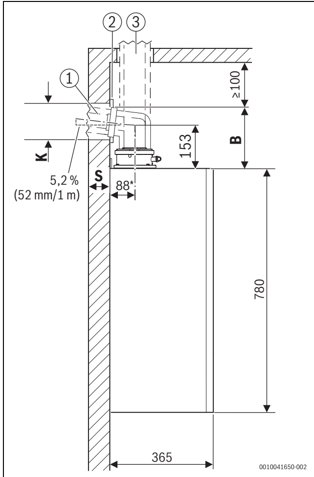
Bild 15 Seitenansicht (mm)
