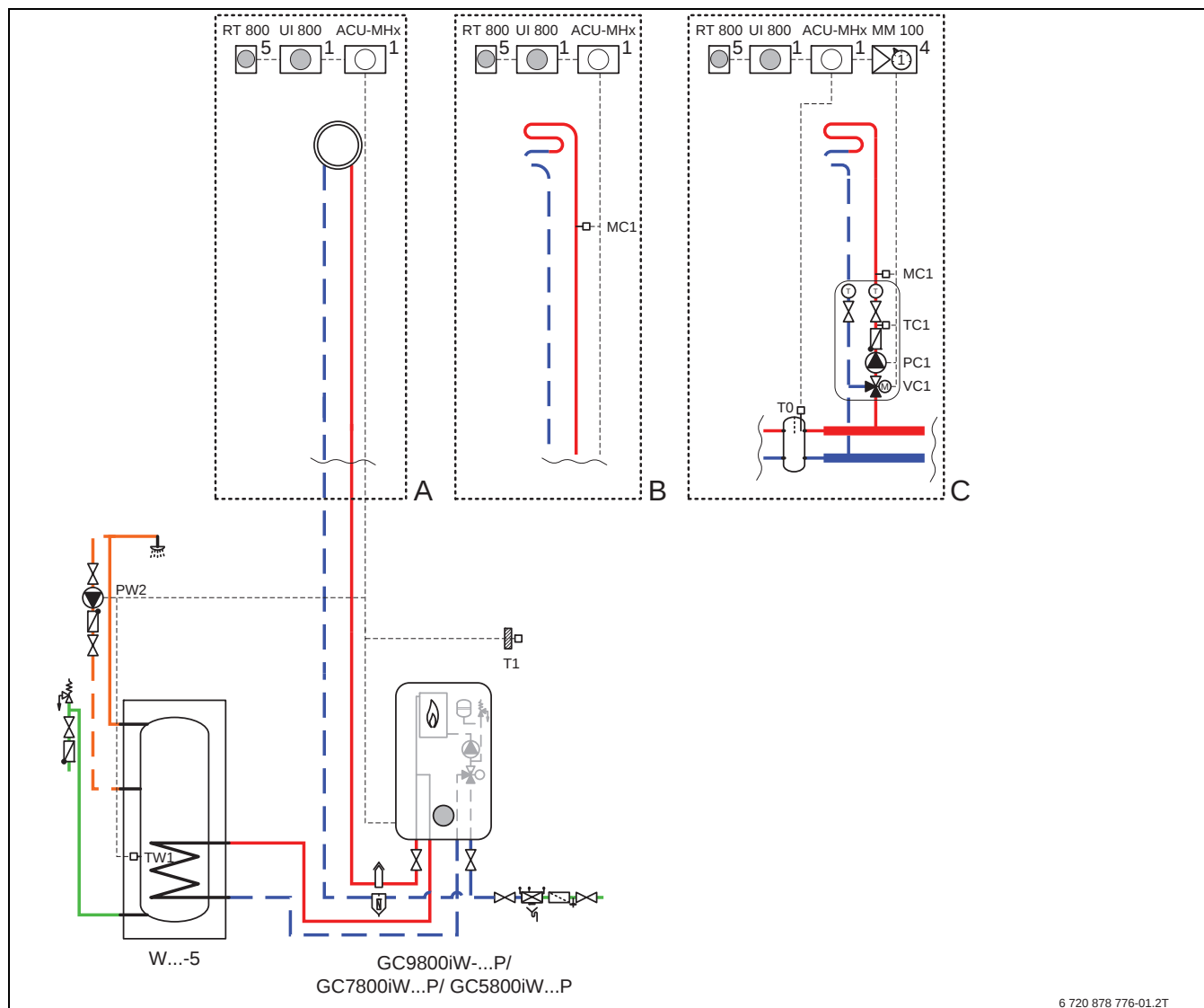
Bild 3 Anlagenschema mit Regelung (unverbindliche Prinzipdarstellung), Abkürzungsverzeichnis → Seite 8
