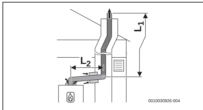
Bild 50 Flexible Abgasführung im Schacht nach B 53p mit raumluftabhängiger Luftzufuhr am Gerät und konzentrischem Verbindungsstück zwischen Aufstellraum und Schacht
