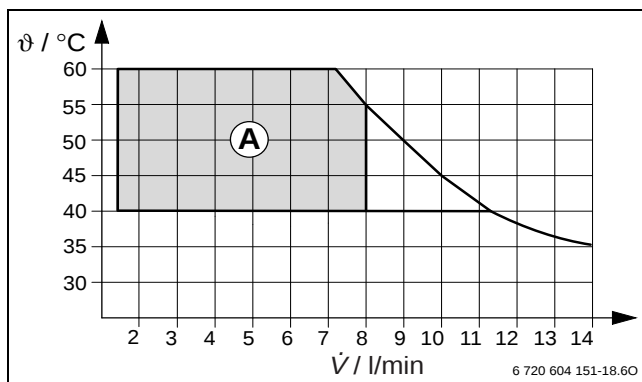
Bild 32 Warmwasseraustritt
