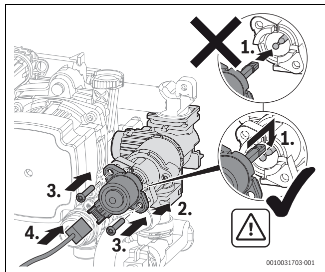
Bild 54 Motor am 3-Wege-Ventil einbauen (Variante mit Schrauben)
