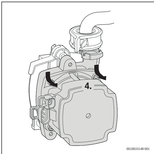
Bild 35 Heizungspumpe abnehmen
