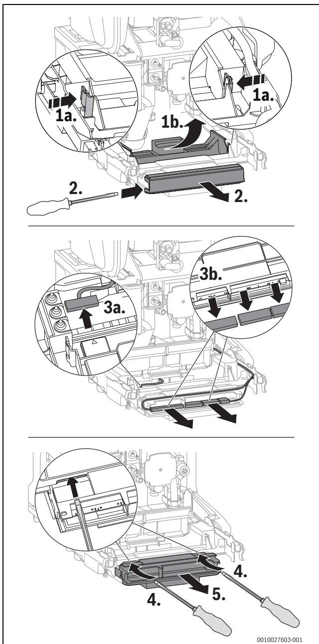
Bild 45 Steuergerät herausnehmen
