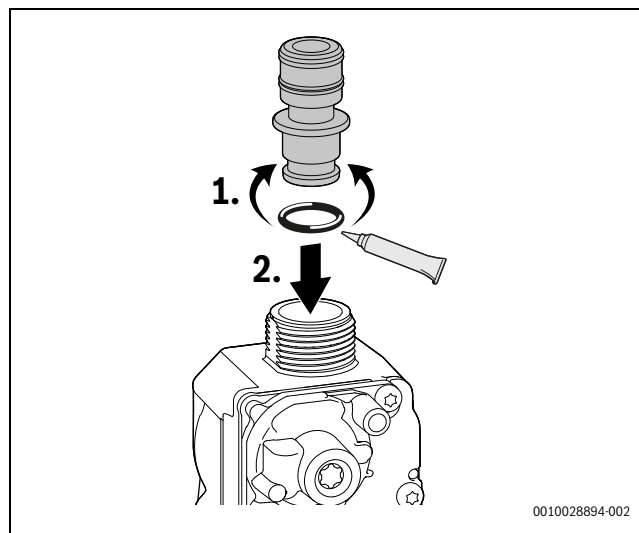
Bild 43 Gasdrossel einsetzen
