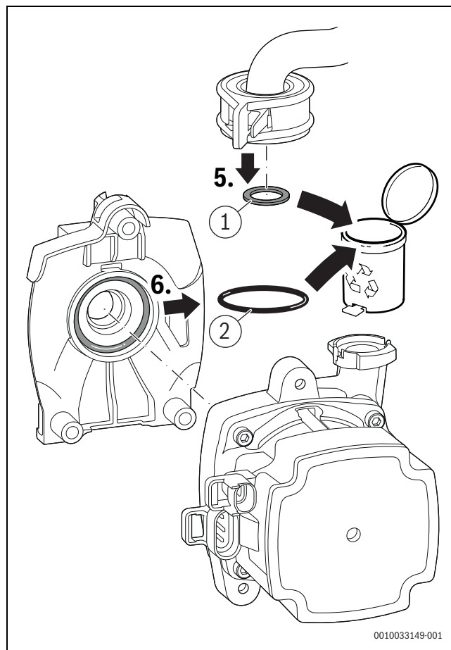
Bild 36 Dichtungen entsorgen
