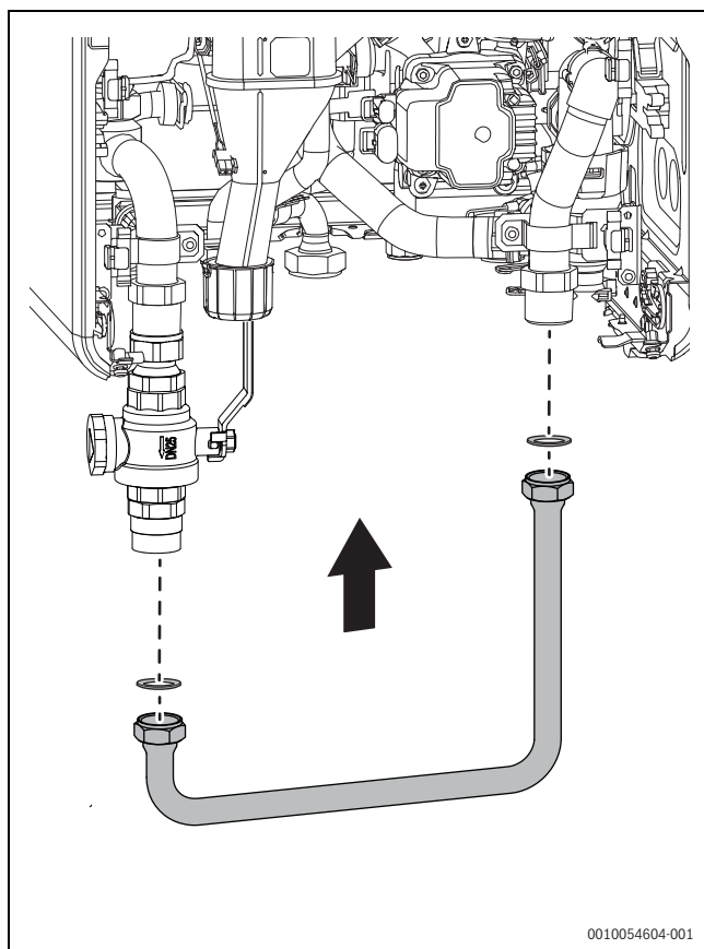
Bild 47 Bypassleitung installieren
