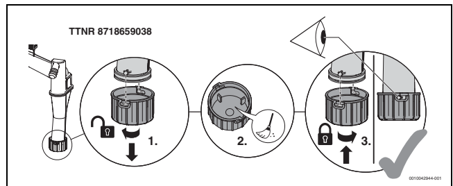
Bild 93 Schmutzfänger reinigen
