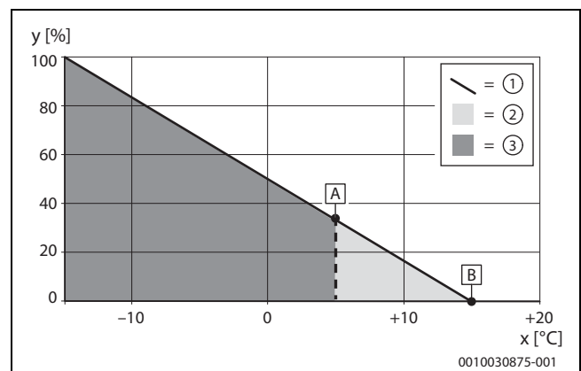
Bild 9 Außentemperatur alternativ
