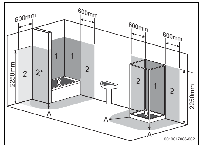
Bild 37 Schutzbereiche (Beispieldarstellung)
