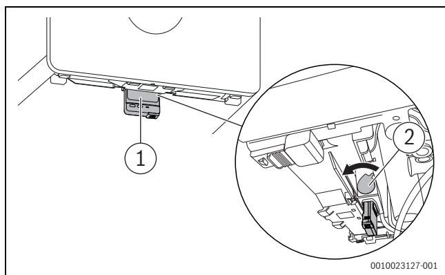
Bild 68 Connect-Key sichern
