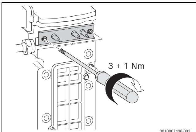
Bild 78 Elektroden-Set montieren
