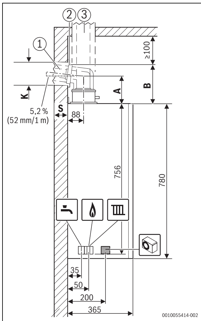
Bild 2 Seitenansicht (mm)
