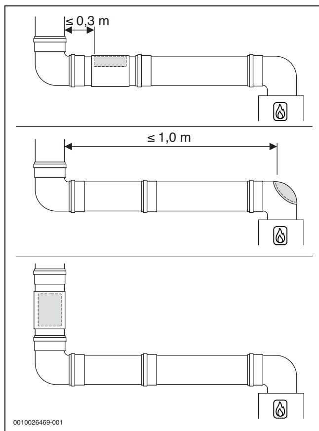
Bild 11 Anordnung der unteren Prüfföffnung
