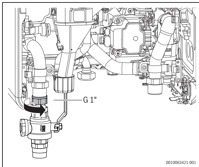
Bild 46 Partikelfilter befestigen
