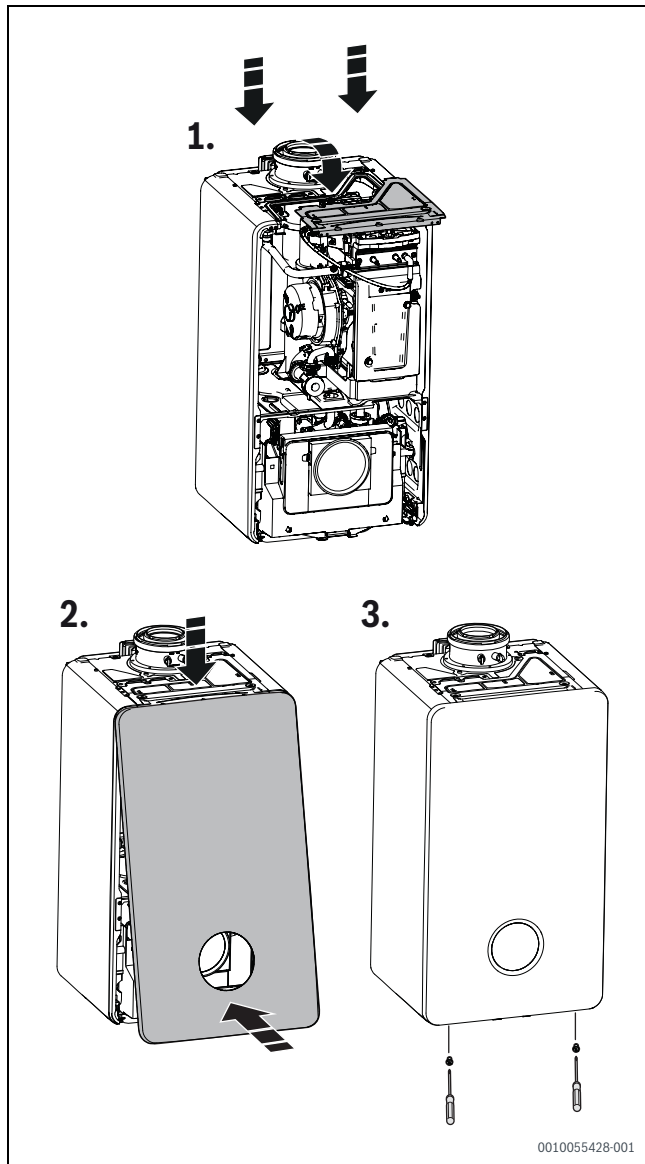
Bild 71 Verkleidung montieren
