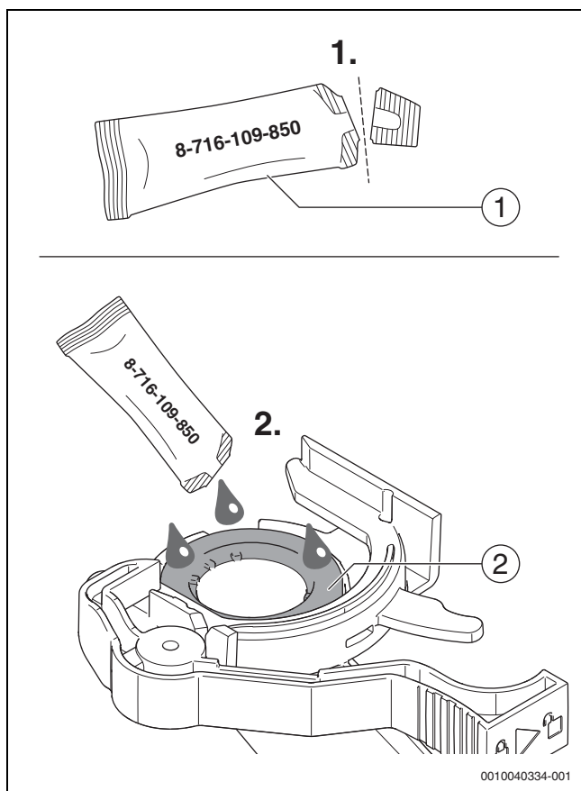
Bild 95 Dichtung schmieren
