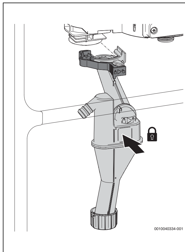
Bild 56 Siphon installieren
