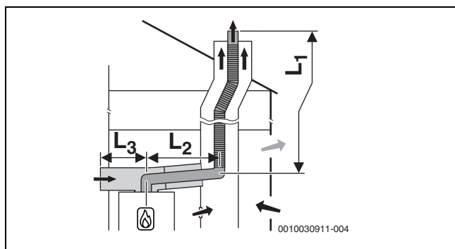
Bild 21 Flexible Abgasführung nach C 53x im Schacht und Luft-Abgas-Führung mit separater Luftzufuhr und konzentrischer Abgasableitung im Aufstellraum
