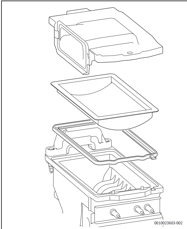
Bild 84 Brenner
