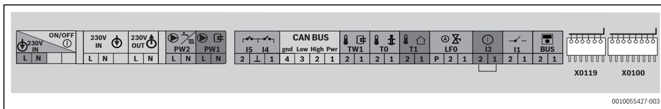
Bild 66 Klemmleiste für externes Zubehör
