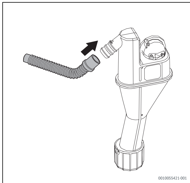
Bild 57 Kondensatschlauch anbringen
