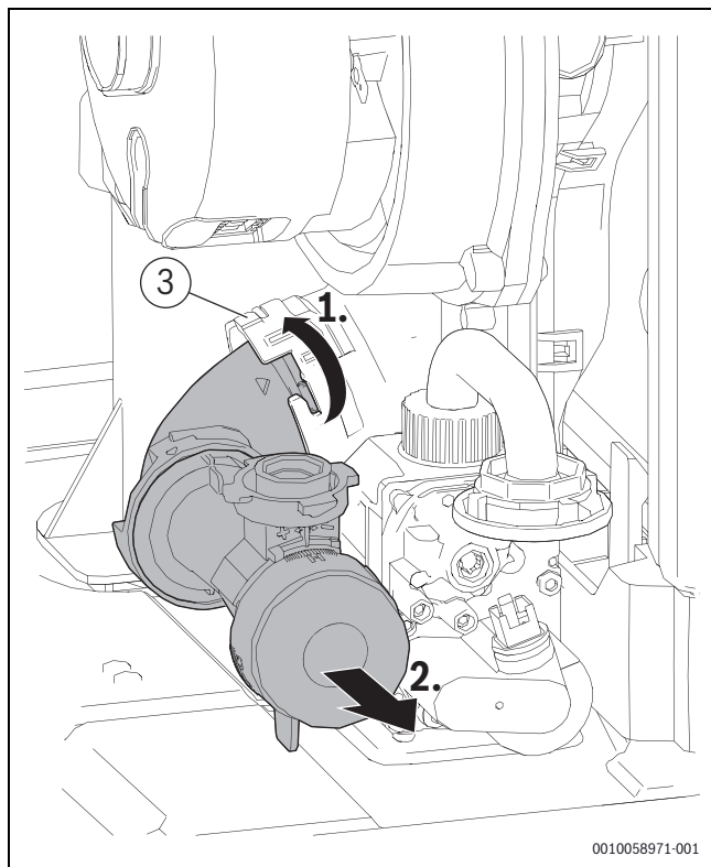
Bild 81 Einstelldüse ausbauen
