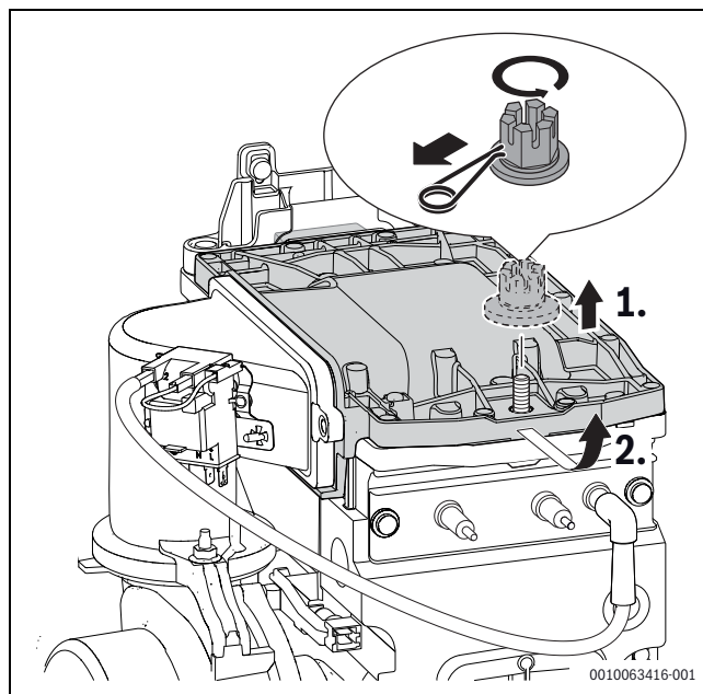
Bild 83 Brennerdeckel ausbauen
