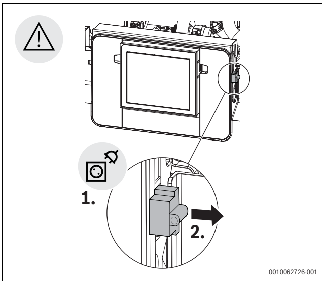
Bild 62 Demontage des Kodiersteckers
