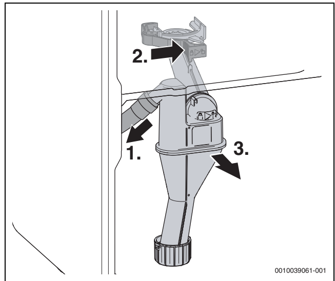
Bild 92 Siphon demontieren
