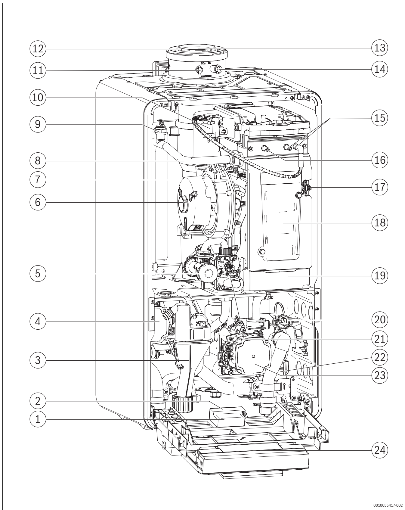
Bild 5 Produktübersicht
