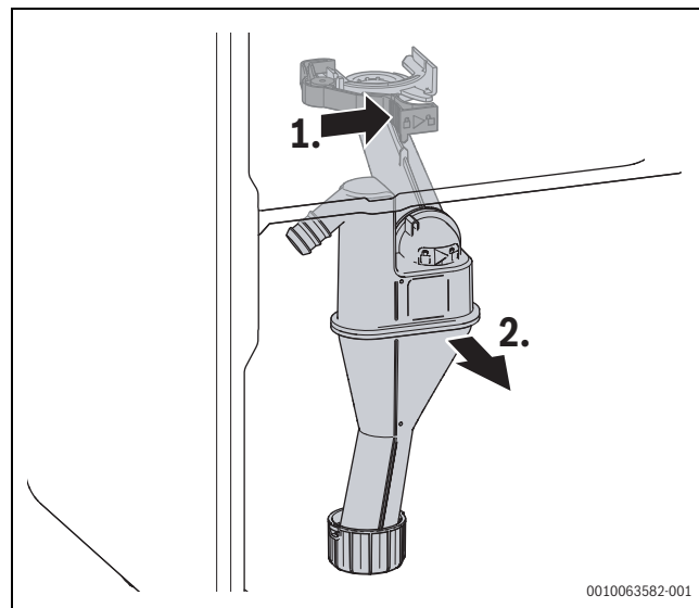
Bild 55 Siphon demontieren
