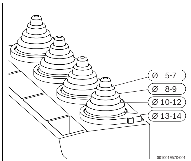
Bild 65 Zugentlastung an Kabeldurchmesser anpassen
