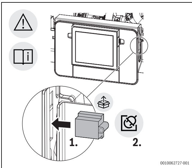
Bild 63 Demontage des Kodiersteckers
