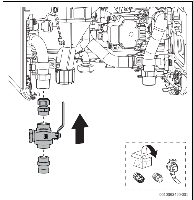
Bild 45 Partikelfilter installieren
