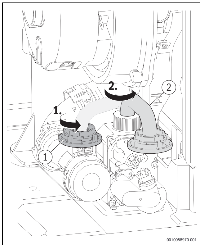
Bild 80 Verriegelung der Einstelldüse öffnen
