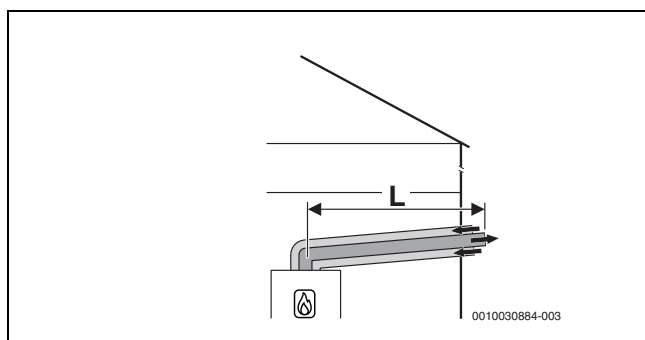
Bild 15 Horizontale konzentrische Luft-Abgas-Führung nach C 13x durch die Außenwand
