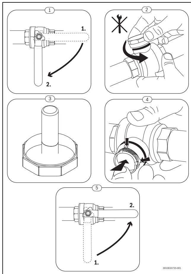
Bild 97 Siebreinigung
