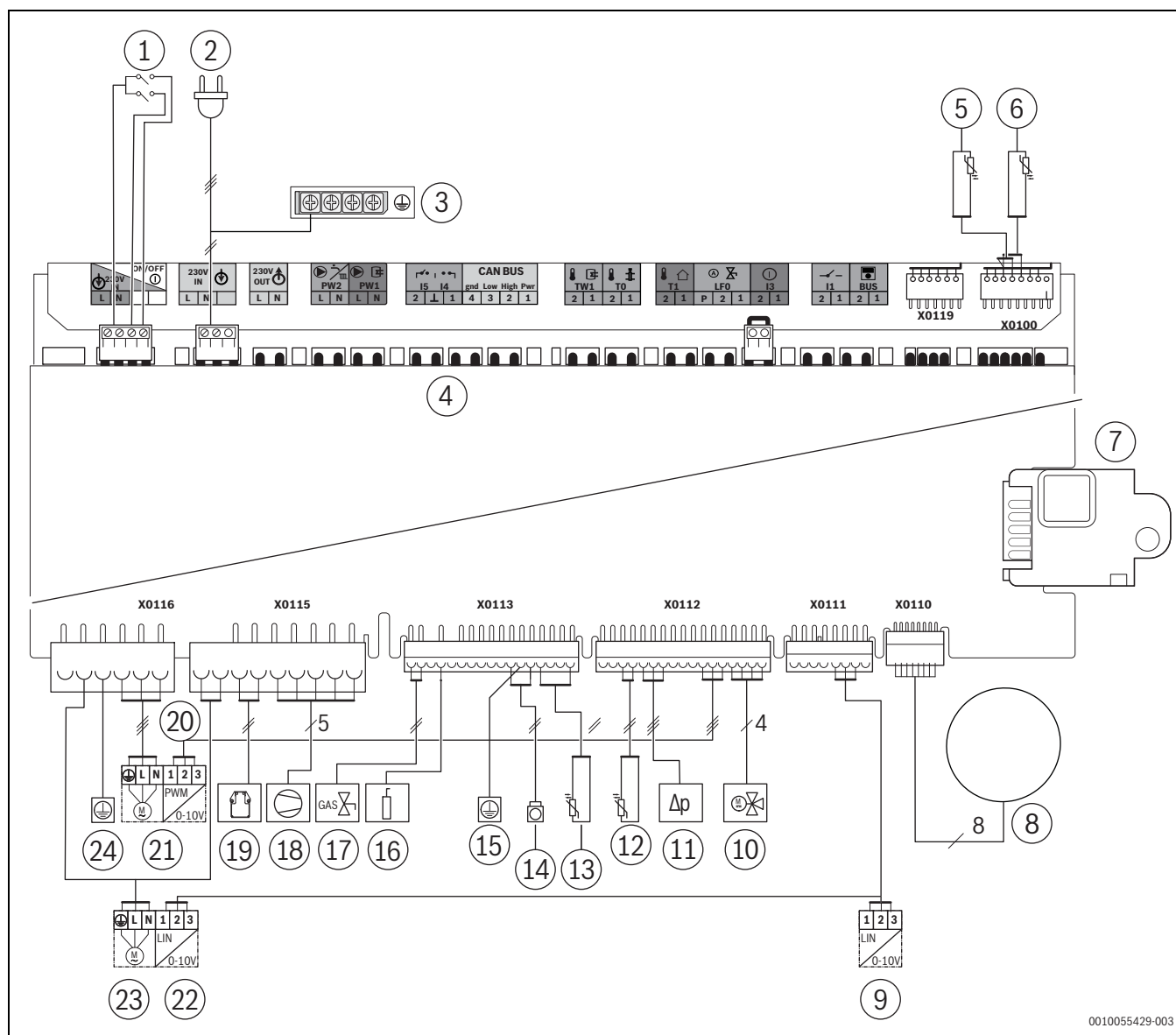
Bild 103 Elektrische Verdrahtung
