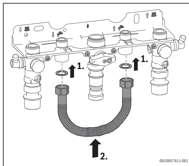
Bild 50 Warmwasser-Bypassleitung (7107800) installieren
