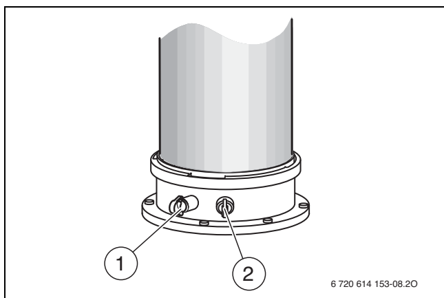
Bild 77 Abgassensstutzen und Verbrennungsluft-Messstutzen
