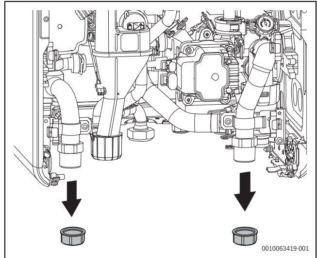
Bild 44 Kappen abnehmen
