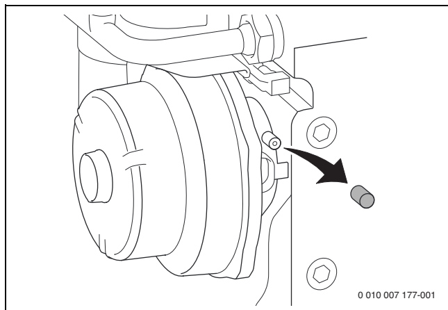
Bild 87 Messstutzen an der Mischeinrichtung
