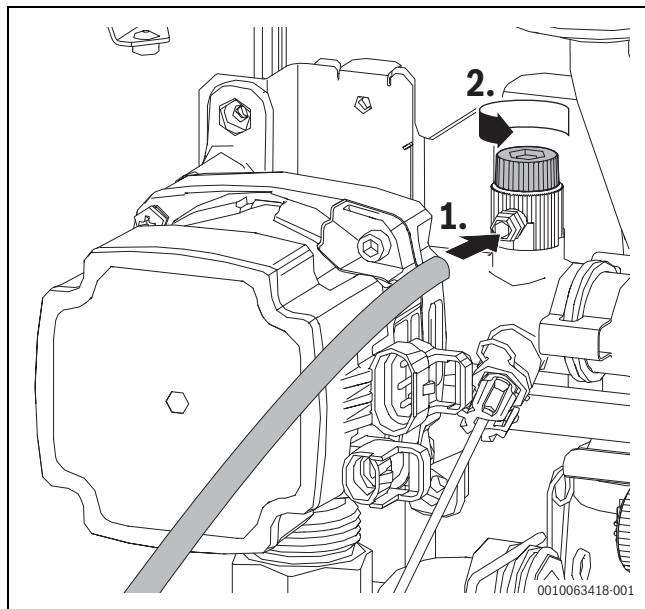
Bild 61 Manuelle Entlüftung der Hybridpumpe
