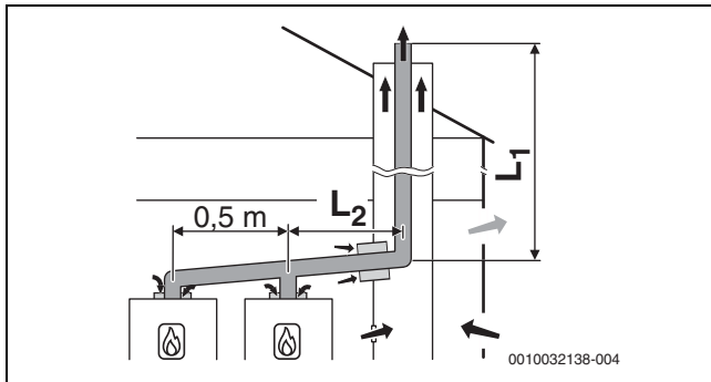
Bild 35 Kaskade mit 2 Geräten: Starre Abgasführung im Schacht nach B 53P mit raumluftabhängiger Luftzufuhr am Gerät und einwandiger Abgasleitung im Aufstellraum; Hinterlüftungsöffnung im Schacht
