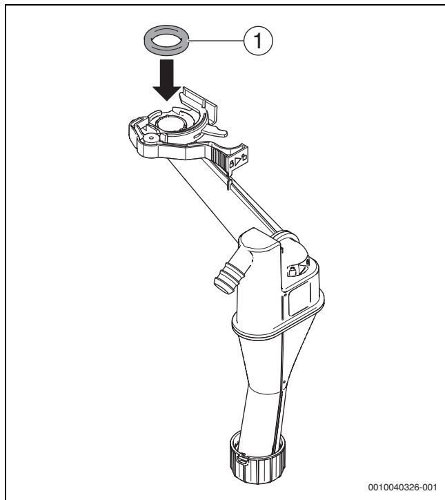
Bild 94 Dichtung in den Siphon einsetzen
