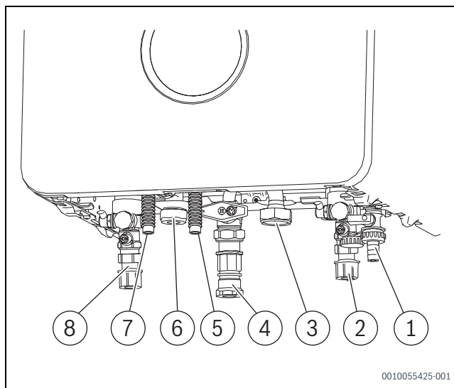
Bild 60 Gas- und wasserseitige Anschlüsse (Zubehör)
