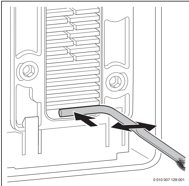
Bild 91 Kondensatwanne reinigen
