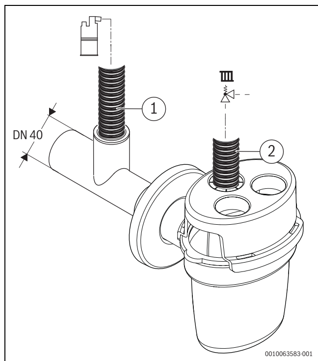
Bild 58 Kondensatschlauch und Schläuche der Sicherheitsventile am Siphon anbringen
