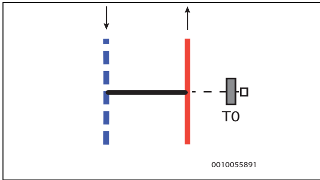
Bild 33 Bypass, gerade Ausführung
