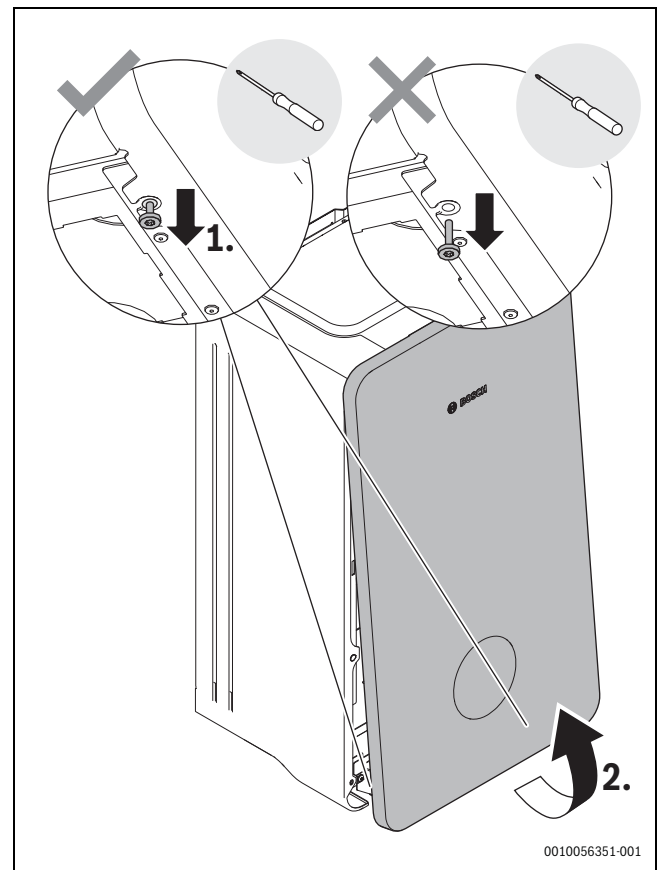
Bild 11 Abdeckung abnehmen
