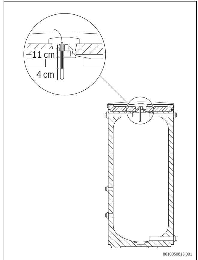
Bild 51 Platzierung des Vorlauftemperaturfühlers T0
