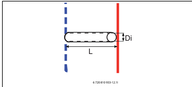
Bild 25 Detailansicht Bypass
