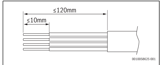
Bild 48 Abisolierung CAN-BUS
