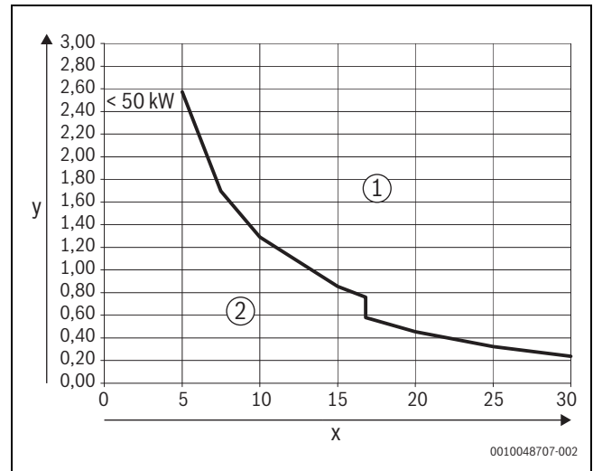
Bild 8 Wärmeerzeuger < 50 kW - 100 kW
