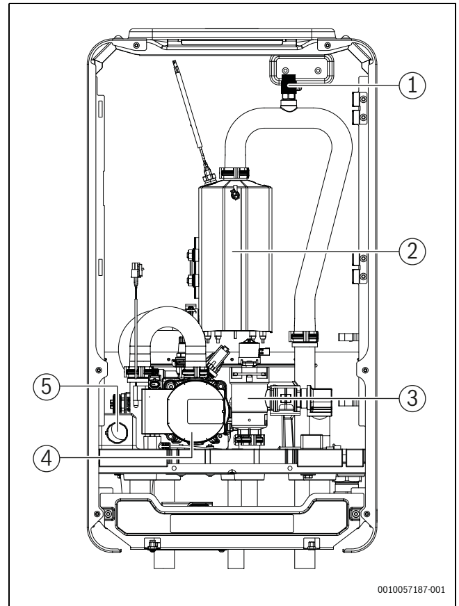
Bild 5 Komponenten
