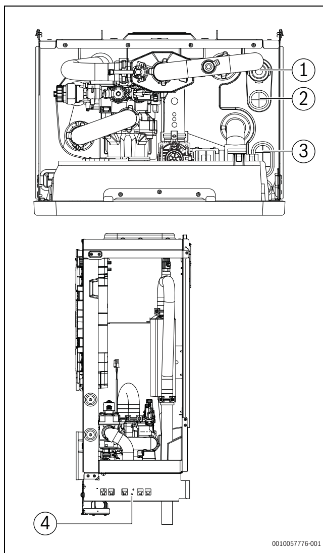
Bild 37 Kabelverschraubung und -durchführungen zur Inneneinheit (Netzanschluss, Zubehör und Niederspannung)
