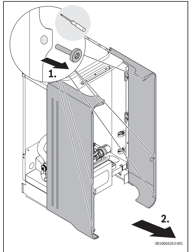
Bild 13 Seitliche Abdeckungen demontieren
