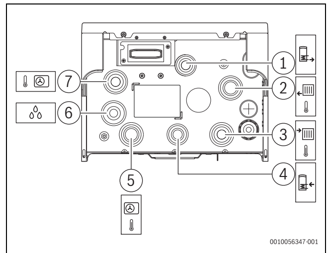
Bild 6 Rohranschlüsse
