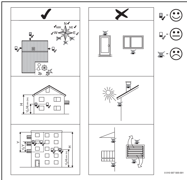
Bild 43 Installationsort Außentemperaturfühler
