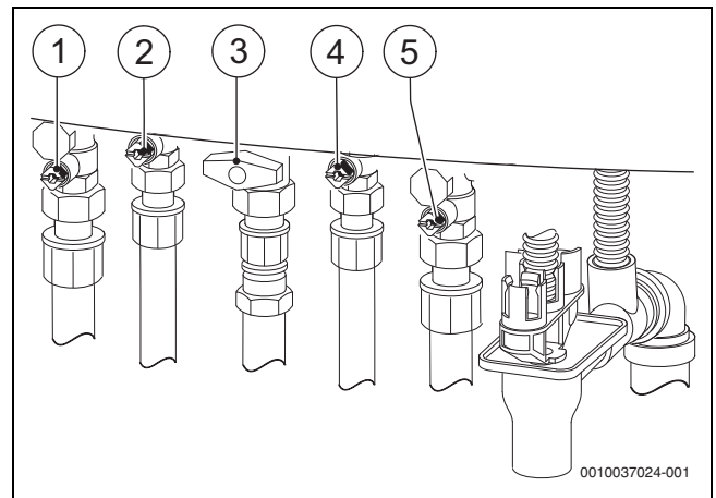
Bild 45 Gas- und wasserseitige Anschlüsse (vertikal)
