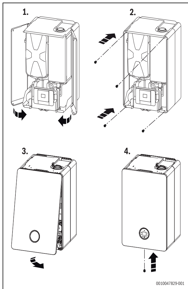
Bild 49 Verkleidung montieren
