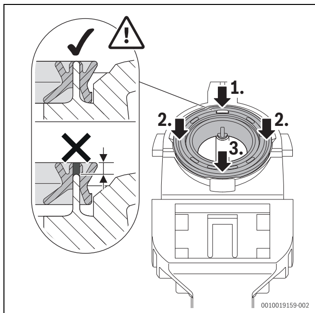
Bild 76 Dichtung andrücken
