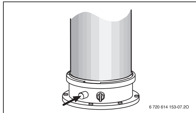
Bild 55 Stopfen abnehmen
