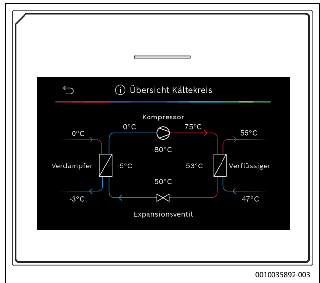
Bild 10 Übersicht Kühlkreis
